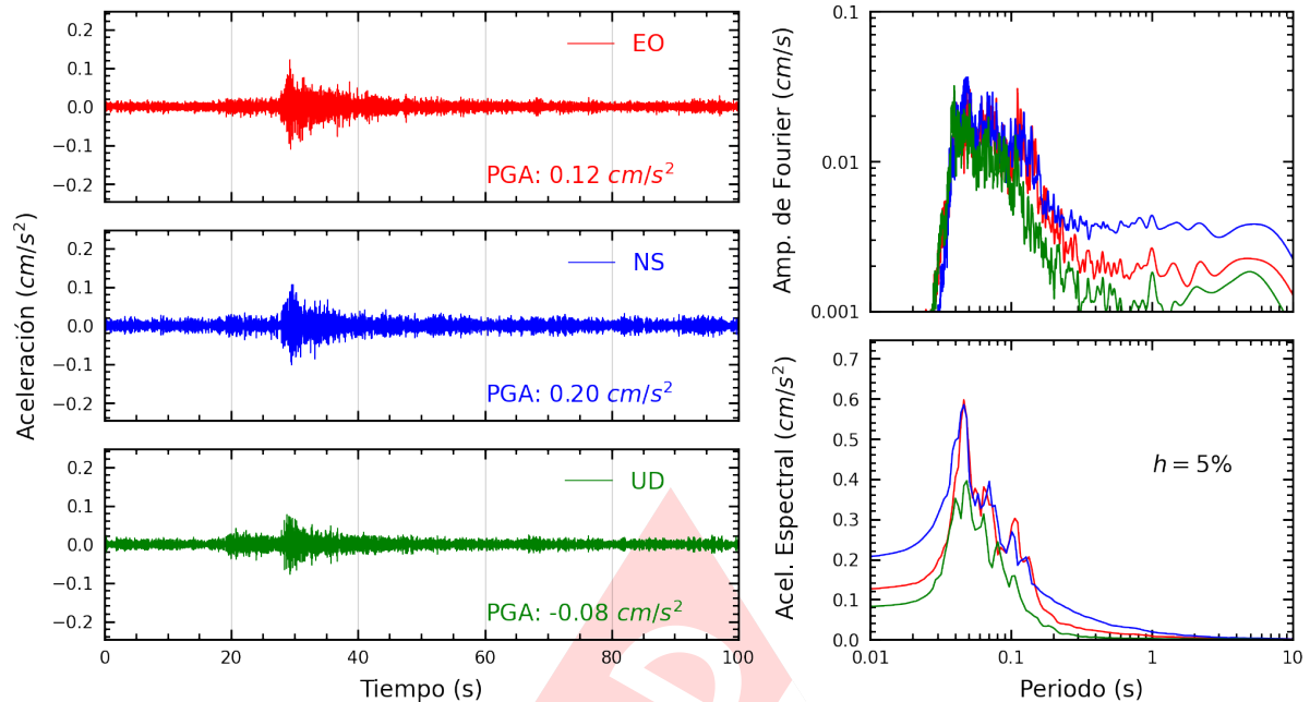
Figura A.3: Registros tiempo-historia, espectros de Fourier y de respuesta en las direcciones EO, NS y vertical de la estación ATARJ. Sismo de Chilca, Cañete - Lima del 2024-05-04, 20:29:16 (Hora local)
