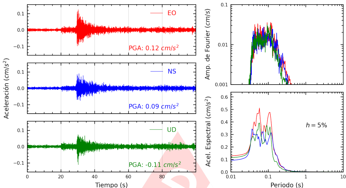
Figura A.5: Registros tiempo-historia, espectros de Fourier y de respuesta en las direcciones EO, NS y vertical de la estación JALV2. Sismo de Chilca, Cañete - Lima del 2024-05-04, 20:29:16 (Hora local)
