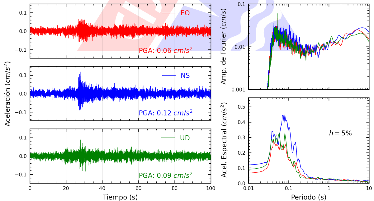
Figura A.8: Registros tiempo-historia, espectros de Fourier y de respuesta en las direcciones EO, NS y vertical de la estación SERVI. Sismo de Chilca, Cañete - Lima del 2024-05-04, 20:29:16 (Hora local)
