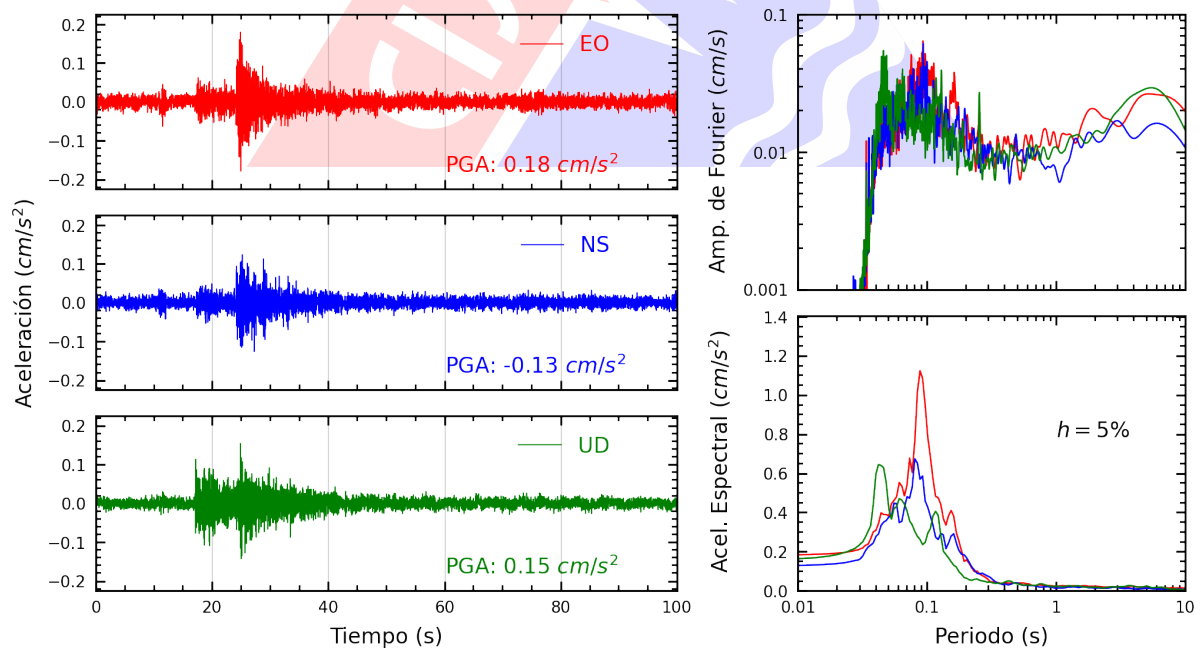
Figura A.4: Registros tiempo-historia, espectros de Fourier y de respuesta en las direcciones EO, NS y vertical de la estación USILP. Sismo de Chilca, Cañete - Lima del 2024-05-04, 20:29:16 (Hora local)
