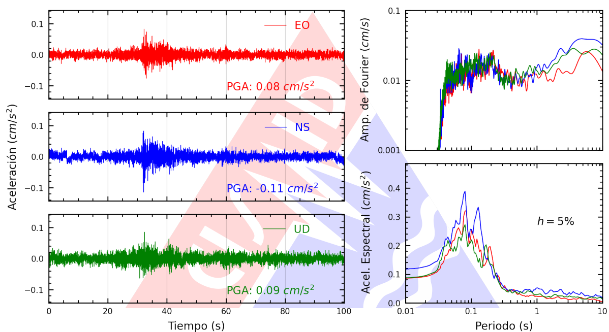
Figura A.9: Registros tiempo-historia, espectros de Fourier y de respuesta en las direcciones EO, NS y vertical de la estación VHAYA. Sismo de Chilca, Cañete - Lima del 2024-05-04, 20:29:16 (Hora local)
