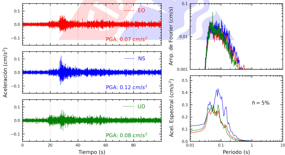
Figura A.6: Registros tiempo-historia, espectros de Fourier y de respuesta en las direcciones EO, NS y vertical de la estación SERV2. Sismo de Chilca, Cañete - Lima del 2024-05-04, 20:29:16 (Hora local)
