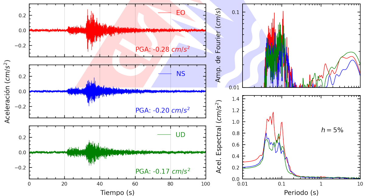
Figura A.2: Registros tiempo-historia, espectros de Fourier y de respuesta en las direcciones EO, NS y vertical de la estación AMORE. Sismo de Chilca, Cañete - Lima del 2024-05-04, 20:29:16 (Hora local)
