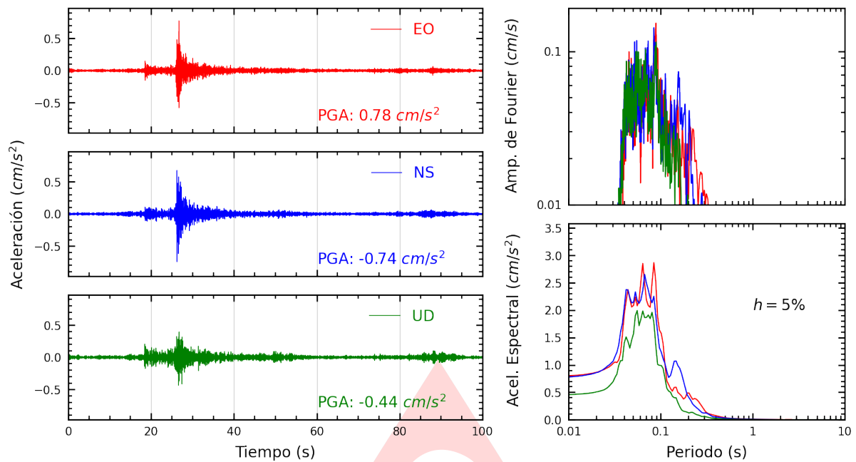
Figura A.1: Registros tiempo-historia, espectros de Fourier y de respuesta en las direcciones EO, NS y vertical de la estación ASIA. Sismo de Chilca, Cañete - Lima del 2024-05-04, 20:29:16 (Hora local)
