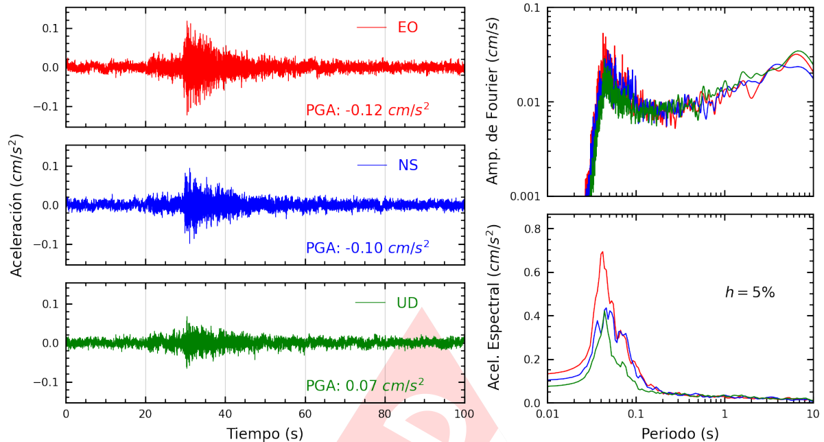
Figura A.7: Registros tiempo-historia, espectros de Fourier y de respuesta en las direcciones EO, NS y vertical de la estación UCSS. Sismo de Chilca, Cañete - Lima del 2024-05-04, 20:29:16 (Hora local)
