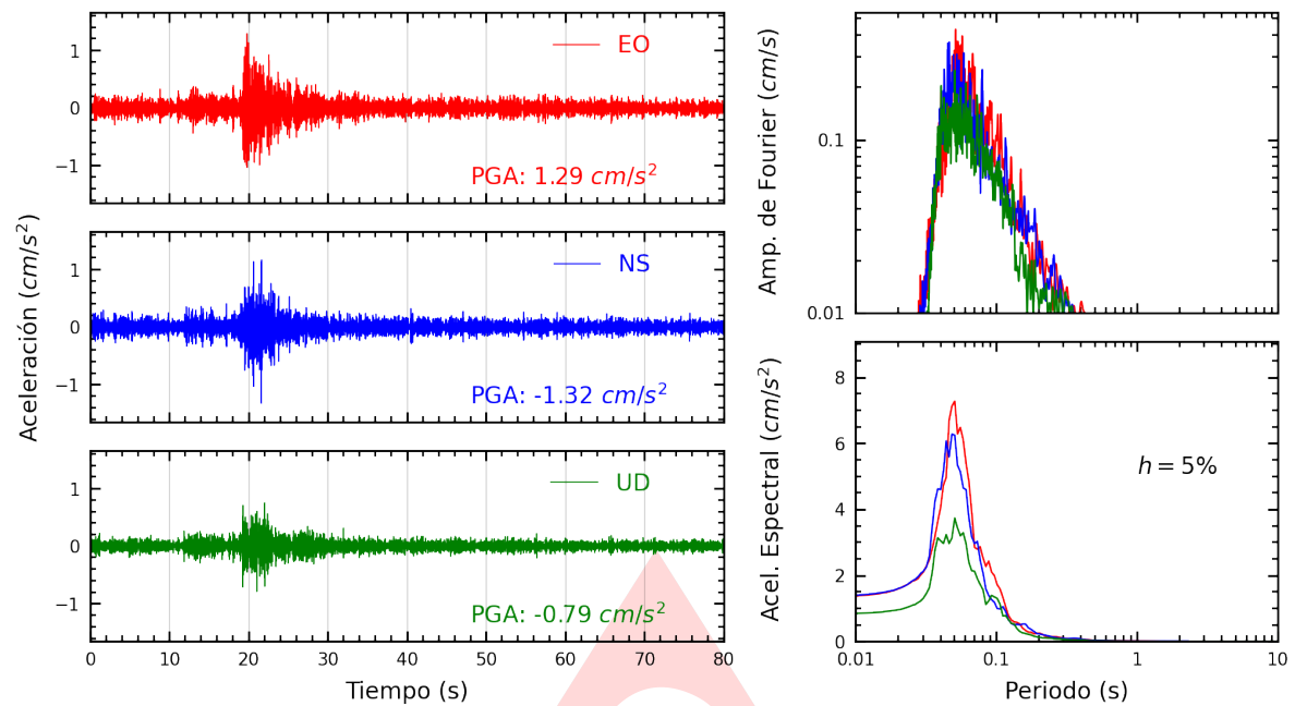
Figura A.1: Registros tiempo-historia, espectros de Fourier y de respuesta en las direcciones EO, NS y vertical de la estación UNTEL. Sismo de Chilca, Cañete - Lima del 2024-05-04, 22:01:40 (Hora local)
