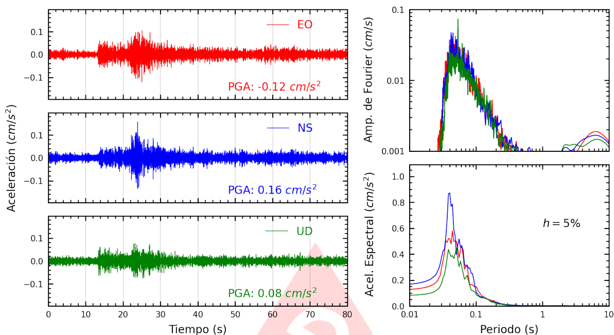
Figura A.17: Registros tiempo-historia, espectros de Fourier y de respuesta en las direcciones EO, NS y vertical de la estación BORJA. Sismo de Chilca, Cañete - Lima del 2024-05-04, 22:01:40 (Hora local)
