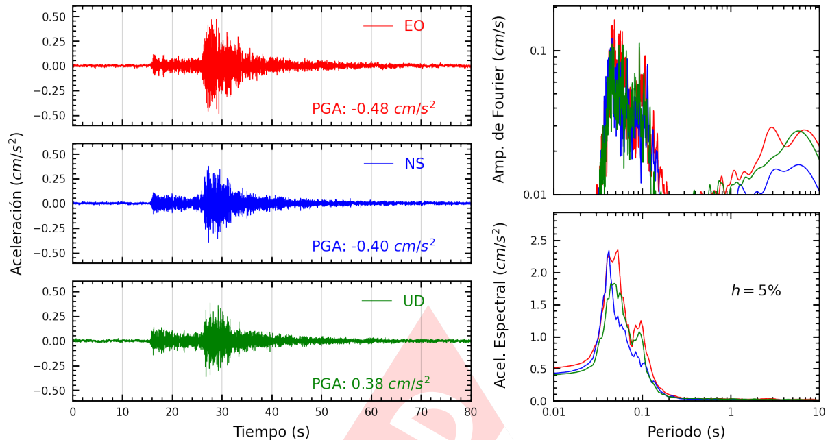
Figura A.5: Registros tiempo-historia, espectros de Fourier y de respuesta en las direcciones EO, NS y vertical de la estación AMORE. Sismo de Chilca, Cañete - Lima del 2024-05-04, 22:01:40 (Hora local)
