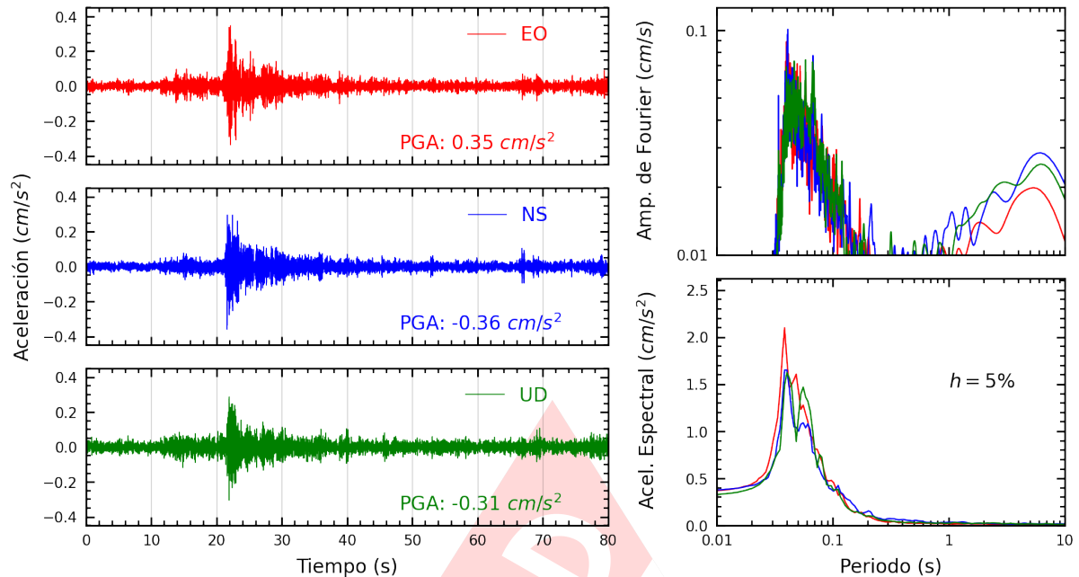
Figura A.7: Registros tiempo-historia, espectros de Fourier y de respuesta en las direcciones EO, NS y vertical de la estación USMP. Sismo de Chilca, Cañete - Lima del 2024-05-04, 22:01:40 (Hora local)
