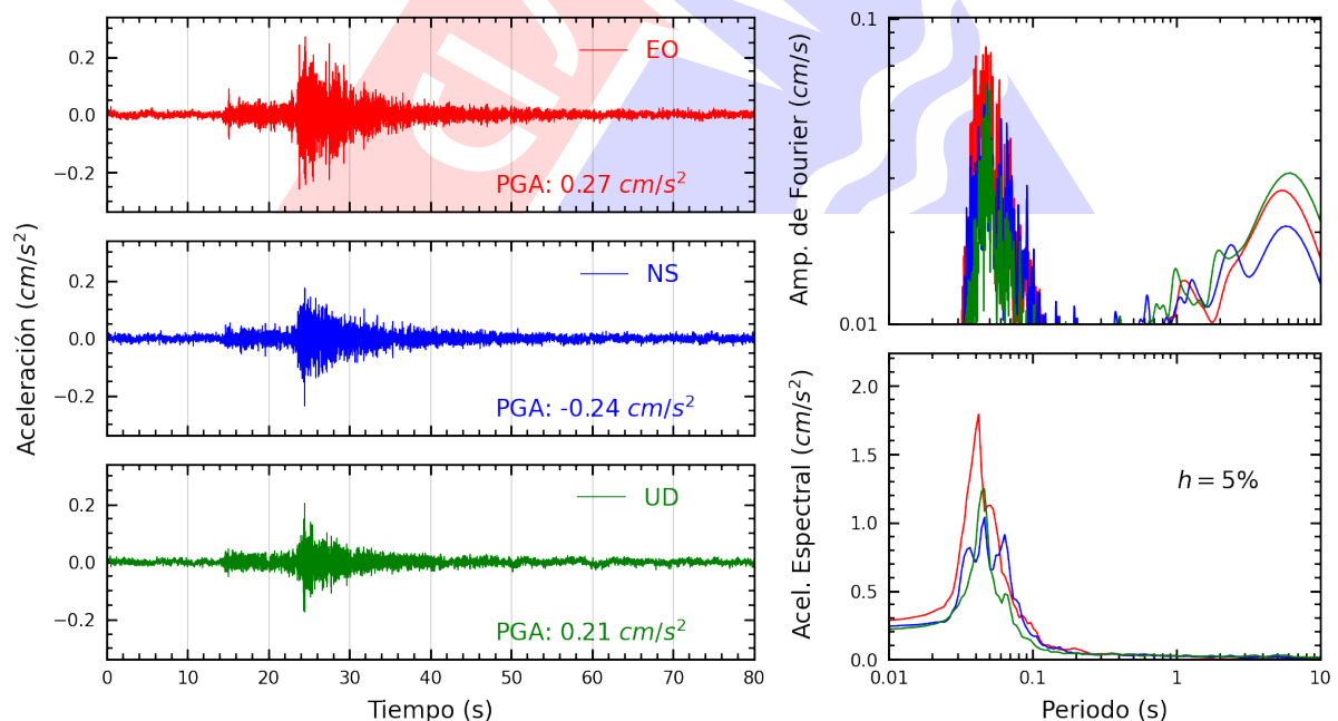
Figura A.10: Registros tiempo-historia, espectros de Fourier y de respuesta en las direcciones EO, NS y vertical de la estación UCSS. Sismo de Chilca, Cañete - Lima del 2024-05-04, 22:01:40 (Hora local)
