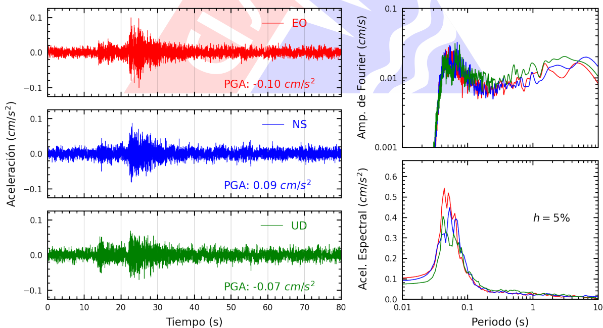
Figura A.18: Registros tiempo-historia, espectros de Fourier y de respuesta en las direcciones EO, NS y vertical de la estación UNFV. Sismo de Chilca, Cañete - Lima del 2024-05-04, 22:01:40 (Hora local)
