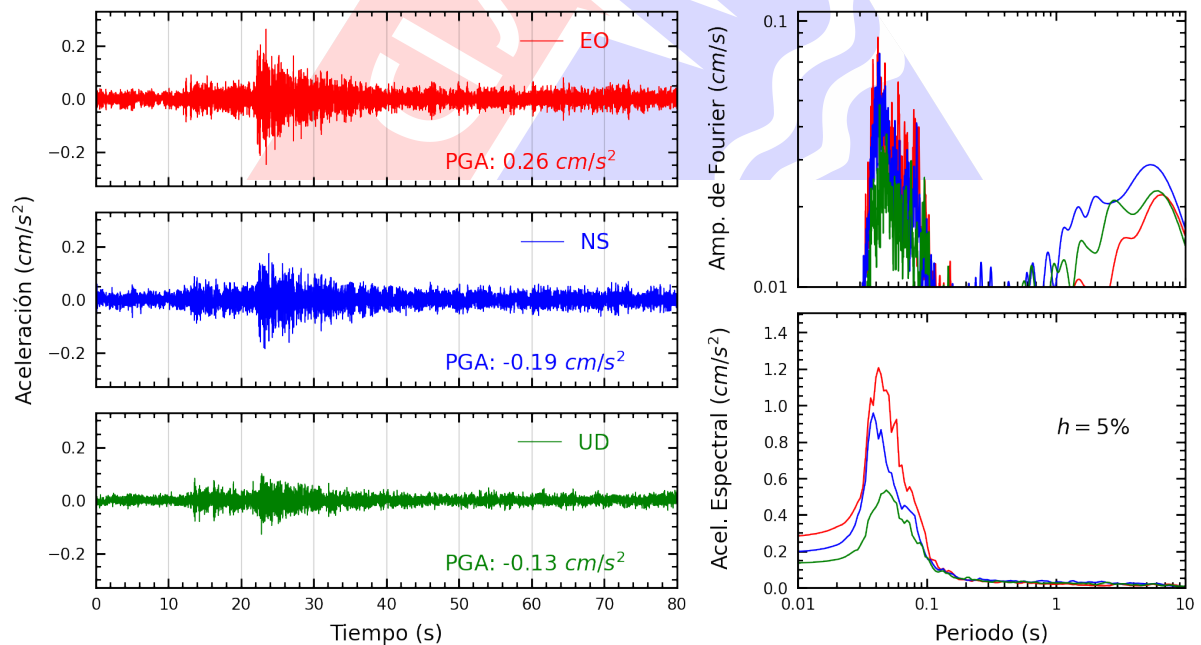
Figura A.12: Registros tiempo-historia, espectros de Fourier y de respuesta en las direcciones EO, NS y vertical de la estación CEPRE. Sismo de Chilca, Cañete - Lima del 2024-05-04, 22:01:40 (Hora local)
