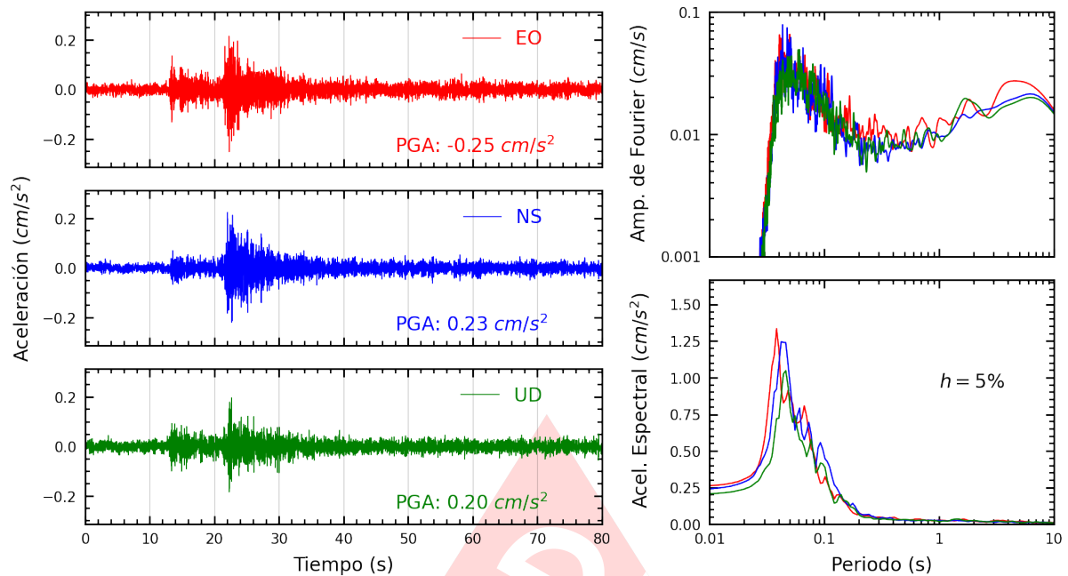
Figura A.13: Registros tiempo-historia, espectros de Fourier y de respuesta en las direcciones EO, NS y vertical de la estación IMCA. Sismo de Chilca, Cañete - Lima del 2024-05-04, 22:01:40 (Hora local)
