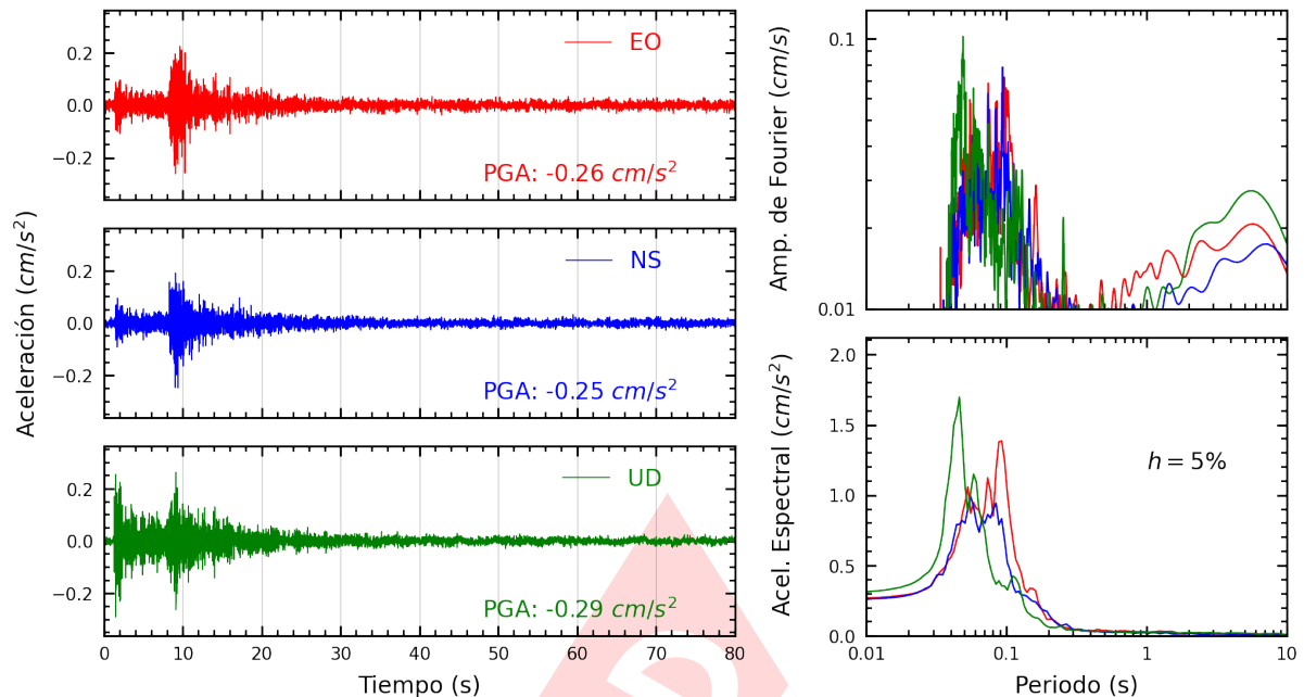
Figura A.9: Registros tiempo-historia, espectros de Fourier y de respuesta en las direcciones EO, NS y vertical de la estación USILP. Sismo de Chilca, Cañete - Lima del 2024-05-04, 22:01:40 (Hora local)
