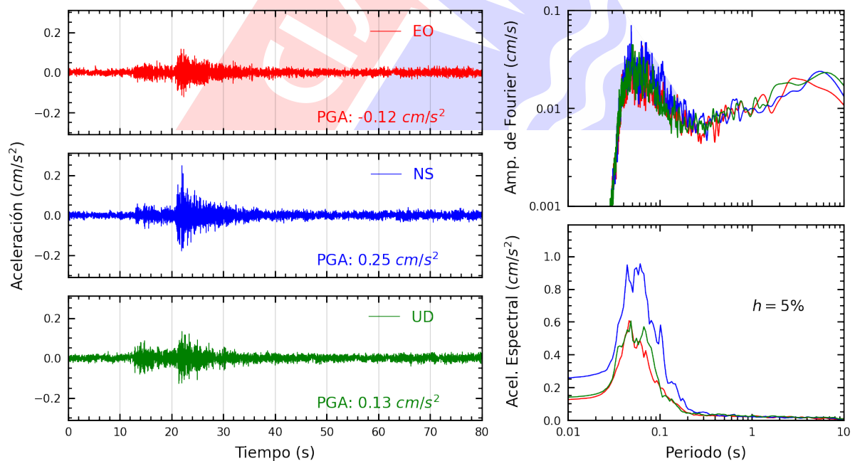
Figura A.14: Registros tiempo-historia, espectros de Fourier y de respuesta en las direcciones EO, NS y vertical de la estación SERVI. Sismo de Chilca, Cañete - Lima del 2024-05-04, 22:01:40 (Hora local)
