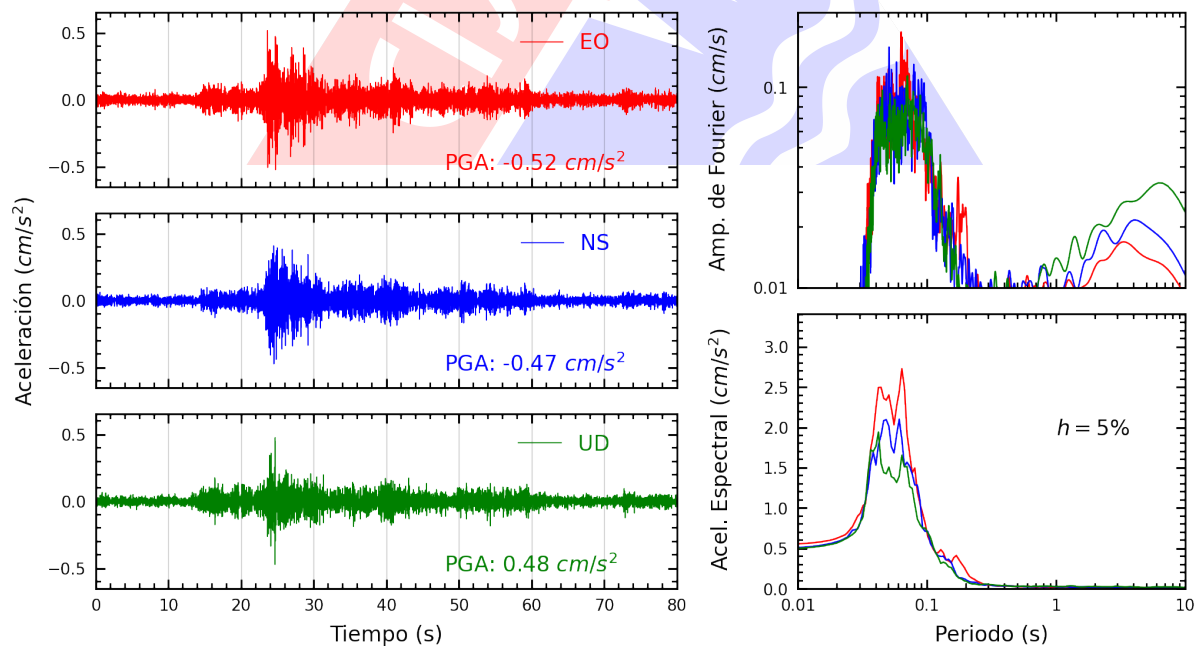
Figura A.4: Registros tiempo-historia, espectros de Fourier y de respuesta en las direcciones EO, NS y vertical de la estación INDEP. Sismo de Chilca, Cañete - Lima del 2024-05-04, 22:01:40 (Hora local)
