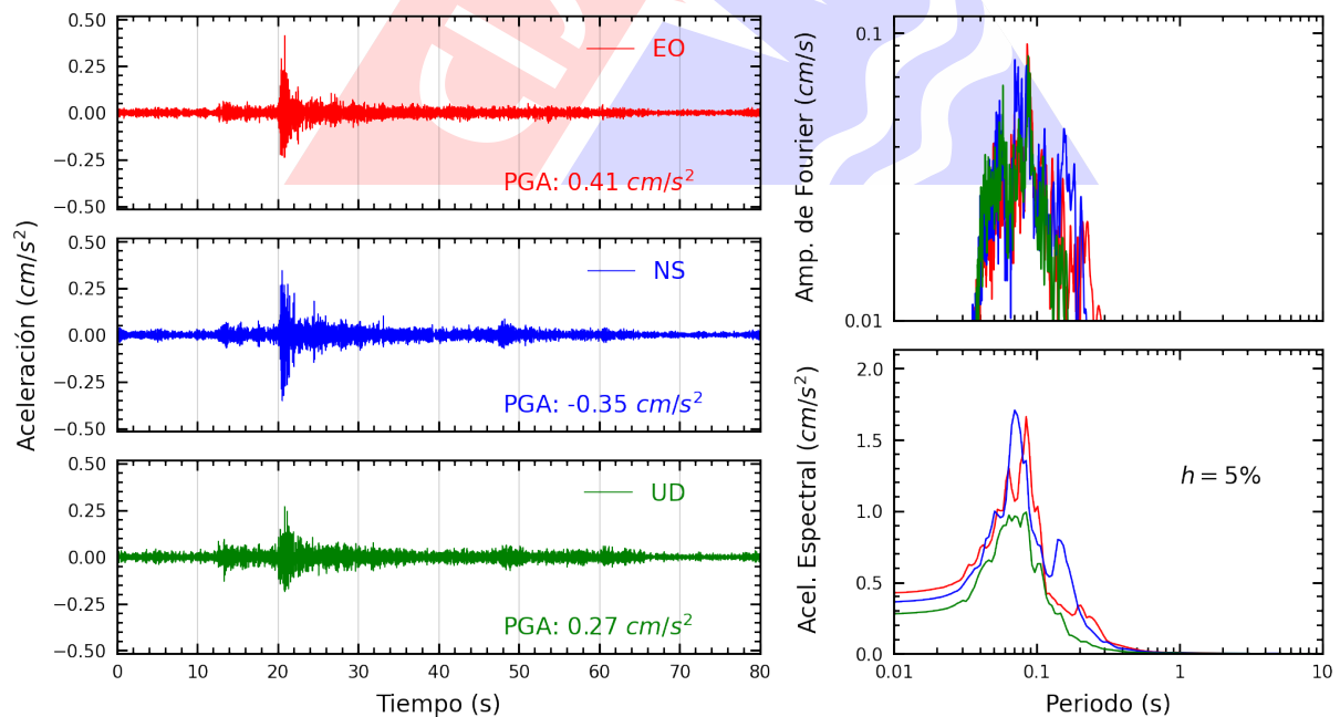
Figura A.6: Registros tiempo-historia, espectros de Fourier y de respuesta en las direcciones EO, NS y vertical de la estación ASIA. Sismo de Chilca, Cañete - Lima del 2024-05-04, 22:01:40 (Hora local)
