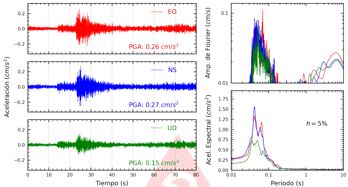
Figura A.11: Registros tiempo-historia, espectros de Fourier y de respuesta en las direcciones EO, NS y vertical de la estación FICPE. Sismo de Chilca, Cañete - Lima del 2024-05-04, 22:01:40 (Hora local)
