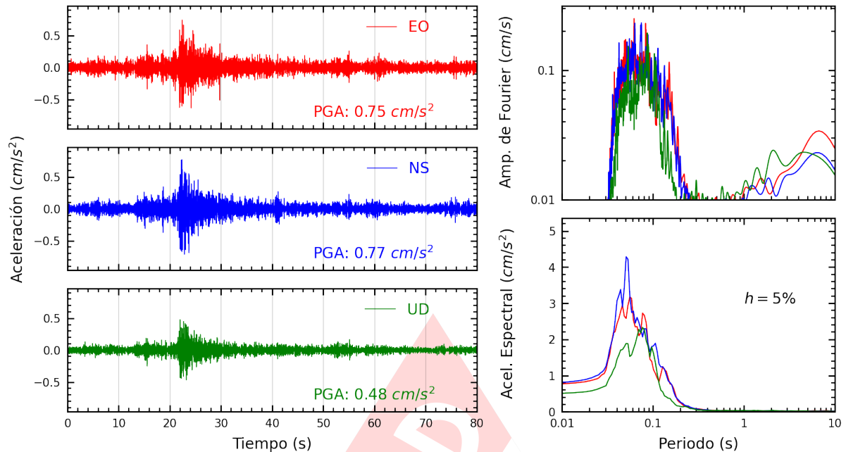
Figura A.3: Registros tiempo-historia, espectros de Fourier y de respuesta en las direcciones EO, NS y vertical de la estación USILM. Sismo de Chilca, Cañete - Lima del 2024-05-04, 22:01:40 (Hora local)
