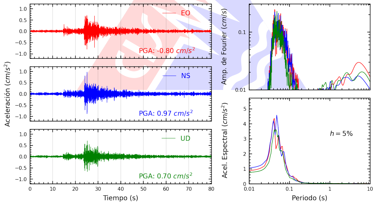
Figura A.2: Registros tiempo-historia, espectros de Fourier y de respuesta en las direcciones EO, NS y vertical de la estación JOSEO. Sismo de Chilca, Cañete - Lima del 2024-05-04, 22:01:40 (Hora local)
