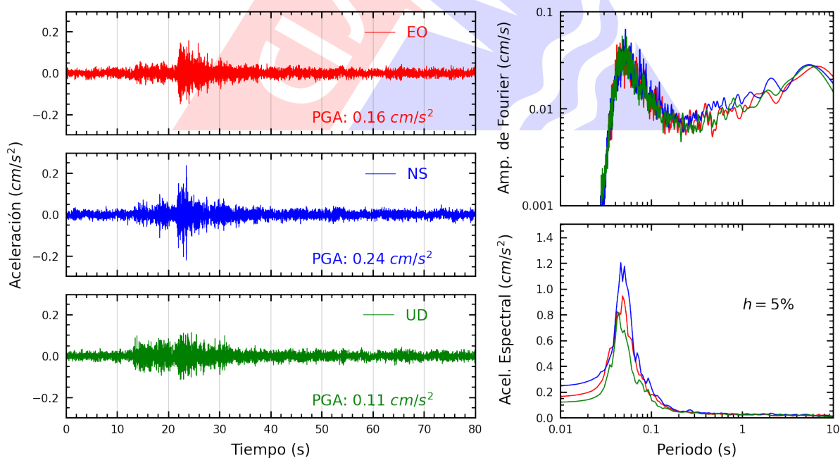
Figura A.16: Registros tiempo-historia, espectros de Fourier y de respuesta en las direcciones EO, NS y vertical de la estación CENEP. Sismo de Chilca, Cañete - Lima del 2024-05-04, 22:01:40 (Hora local)
