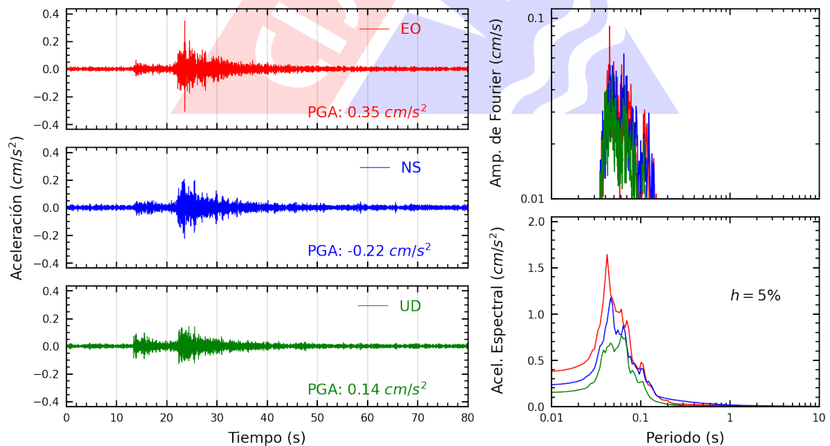
Figura A.8: Registros tiempo-historia, espectros de Fourier y de respuesta en las direcciones EO, NS y vertical de la estación ATARJ. Sismo de Chilca, Cañete - Lima del 2024-05-04, 22:01:40 (Hora local)
