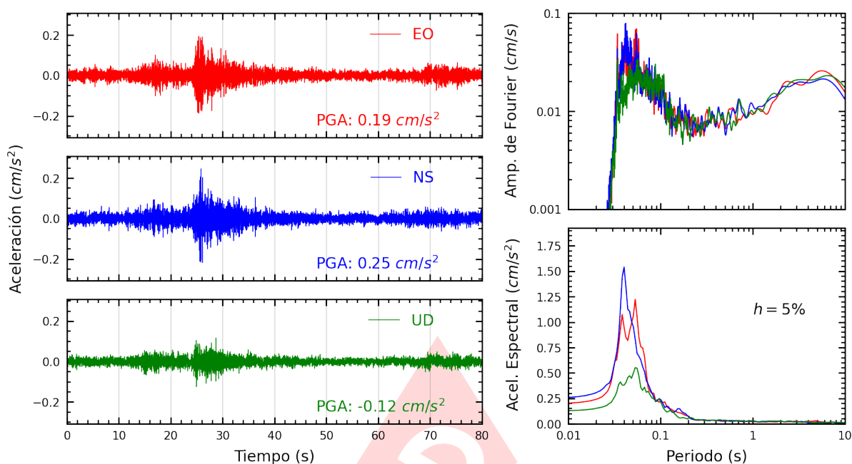
Figura A.15: Registros tiempo-historia, espectros de Fourier y de respuesta en las direcciones EO, NS y vertical de la estación COMAS. Sismo de Chilca, Cañete - Lima del 2024-05-04, 22:01:40 (Hora local)
