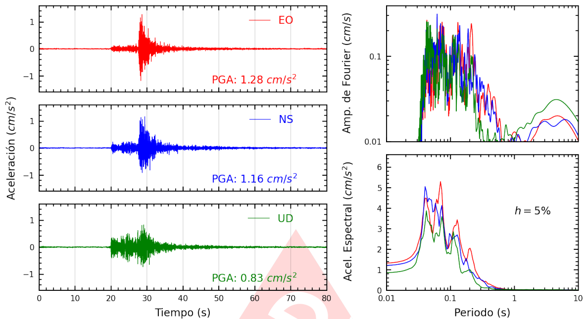
Figura A.25: Registros tiempo-historia, espectros de Fourier y de respuesta en las direcciones EO, NS y vertical de la estación VHAYA. Sismo de Provincia Constitucional del Callao , Callao - Lima del 2024-05-04, 22:17:27 (Hora local)
