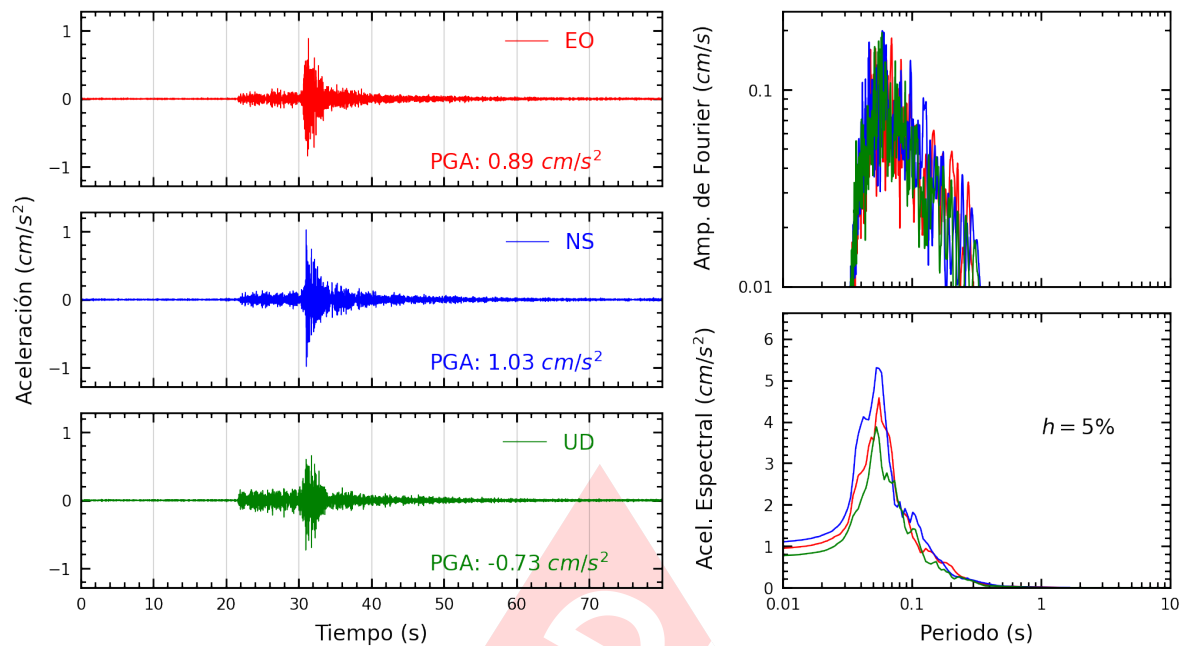
Figura A.29: Registros tiempo-historia, espectros de Fourier y de respuesta en las direcciones EO, NS y vertical de la estación SERV2. Sismo de Provincia Constitucional del Callao , Callao - Lima del 2024-05-04, 22:17:27 (Hora local)
