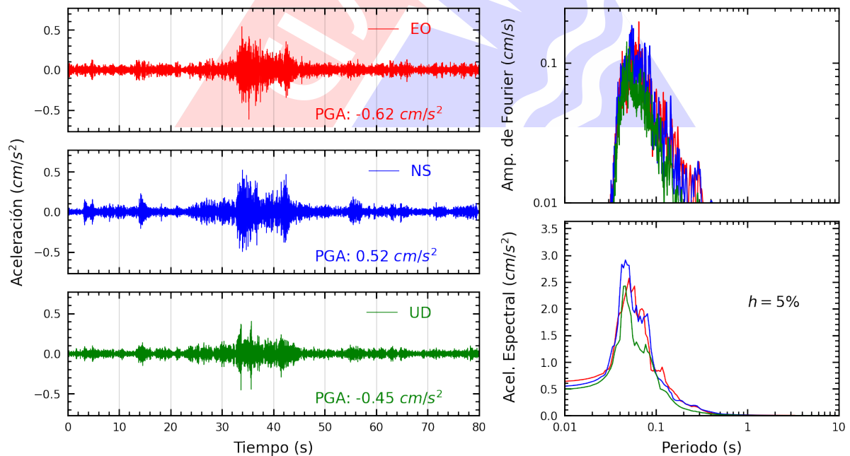
Figura A.32: Registros tiempo-historia, espectros de Fourier y de respuesta en las direcciones EO, NS y vertical de la estación PACHA. Sismo de Provincia Constitucional del Callao , Callao - Lima del 2024-05-04, 22:17:27 (Hora local)
