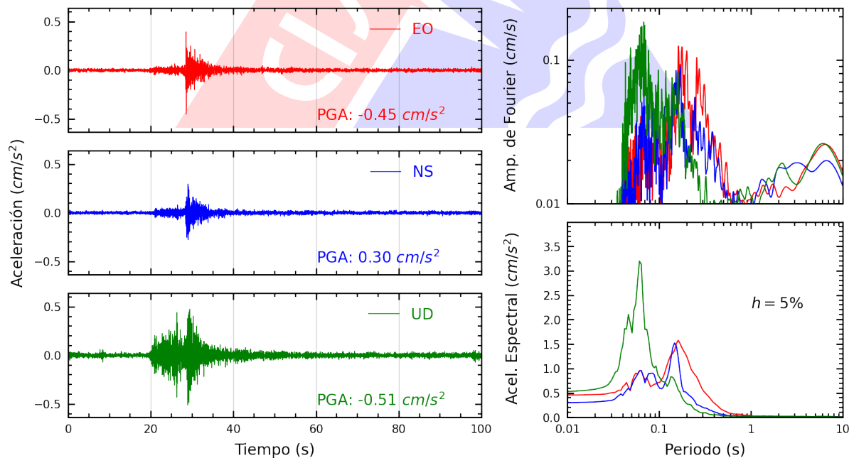
Figura A.34: Registros tiempo-historia, espectros de Fourier y de respuesta en las direcciones EO, NS y vertical de la estación ACAPU. Sismo de Provincia Constitucional del Callao , Callao - Lima del 2024-05-04, 22:17:27 (Hora local)
