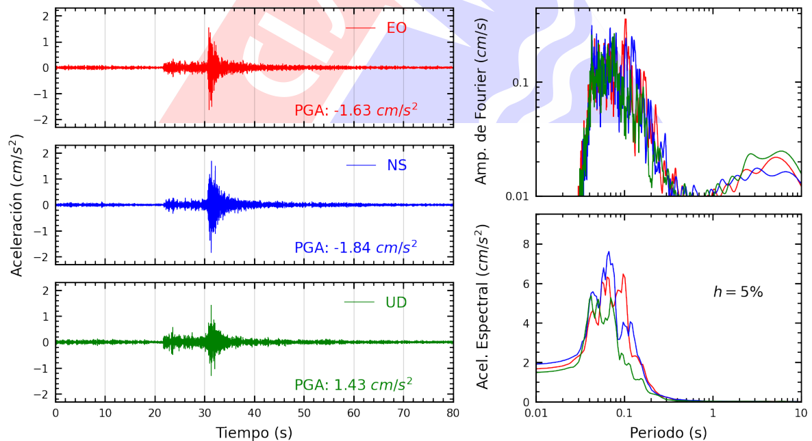
Figura A.20: Registros tiempo-historia, espectros de Fourier y de respuesta en las direcciones EO, NS y vertical de la estación URPE. Sismo de Provincia Constitucional del Callao , Callao - Lima del 2024-05-04, 22:17:27 (Hora local)
