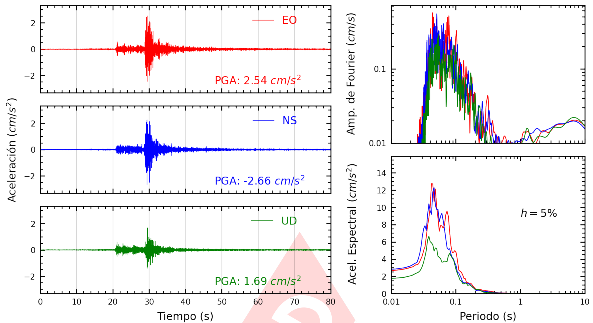
Figura A.15: Registros tiempo-historia, espectros de Fourier y de respuesta en las direcciones EO, NS y vertical de la estación FICPE. Sismo de Provincia Constitucional del Callao , Callao - Lima del 2024-05-04, 22:17:27 (Hora local)
