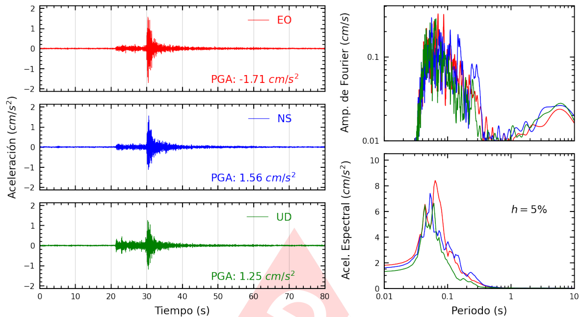
Figura A.21: Registros tiempo-historia, espectros de Fourier y de respuesta en las direcciones EO, NS y vertical de la estación CENEP. Sismo de Provincia Constitucional del Callao , Callao - Lima del 2024-05-04, 22:17:27 (Hora local)
