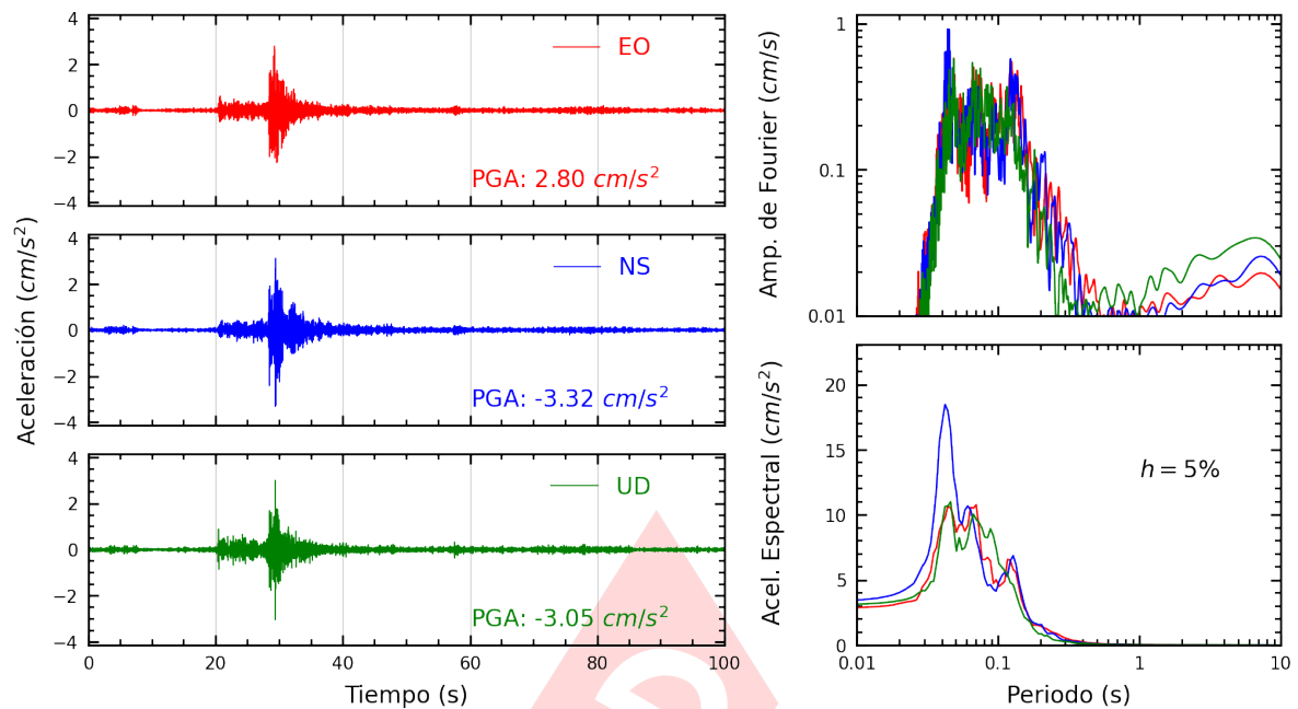
Figura A.7: Registros tiempo-historia, espectros de Fourier y de respuesta en las direcciones EO, NS y vertical de la estación CARAB. Sismo de Provincia Constitucional del Callao , Callao - Lima del 2024-05-04, 22:17:27 (Hora local)
