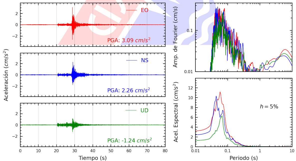
Figura A.8: Registros tiempo-historia, espectros de Fourier y de respuesta en las direcciones EO, NS y vertical de la estación COMAS. Sismo de Provincia Constitucional del Callao , Callao - Lima del 2024-05-04, 22:17:27 (Hora local)
