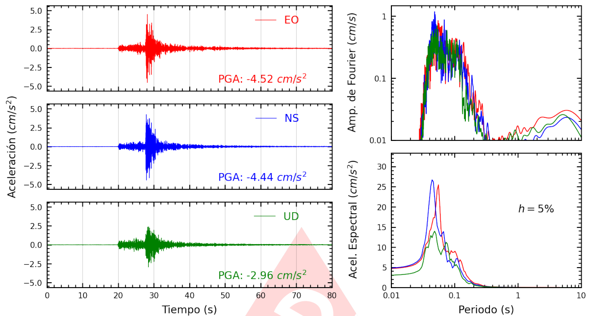
Figura A.5: Registros tiempo-historia, espectros de Fourier y de respuesta en las direcciones EO, NS y vertical de la estación AMORE. Sismo de Provincia Constitucional del Callao , Callao - Lima del 2024-05-04, 22:17:27 (Hora local)
