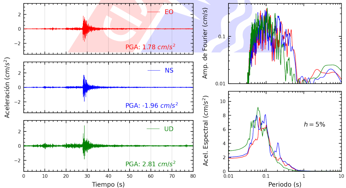
Figura A.12: Registros tiempo-historia, espectros de Fourier y de respuesta en las direcciones EO, NS y vertical de la estación MDPP. Sismo de Provincia Constitucional del Callao , Callao - Lima del 2024-05-04, 22:17:27 (Hora local)
