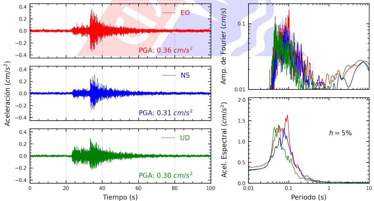
Figura A.36: Registros tiempo-historia, espectros de Fourier y de respuesta en las direcciones EO, NS y vertical de la estación USILP. Sismo de Provincia Constitucional del Callao , Callao - Lima del 2024-05-04, 22:17:27 (Hora local)
