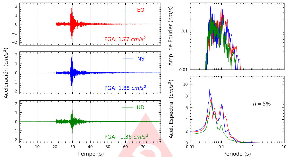
Figura A.19: Registros tiempo-historia, espectros de Fourier y de respuesta en las direcciones EO, NS y vertical de la estación JALV2. Sismo de Provincia Constitucional del Callao , Callao - Lima del 2024-05-04, 22:17:27 (Hora local)
