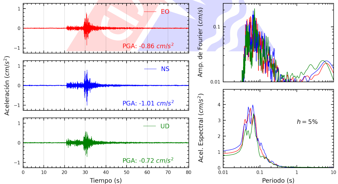
Figura A.30: Registros tiempo-historia, espectros de Fourier y de respuesta en las direcciones EO, NS y vertical de la estación UNFV. Sismo de Provincia Constitucional del Callao , Callao - Lima del 2024-05-04, 22:17:27 (Hora local)
