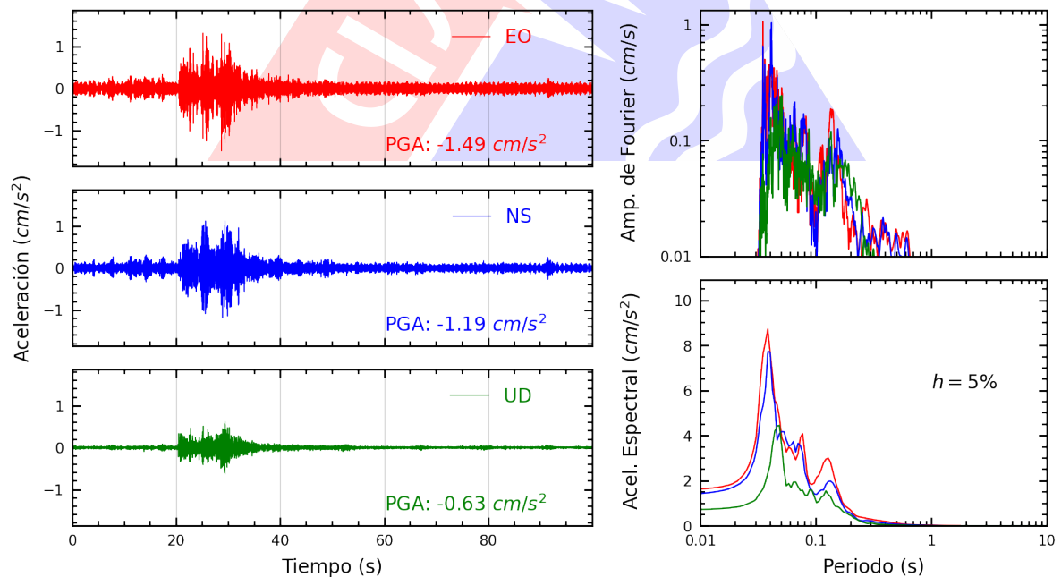
Figura A.24: Registros tiempo-historia, espectros de Fourier y de respuesta en las direcciones EO, NS y vertical de la estación DHN2. Sismo de Provincia Constitucional del Callao , Callao - Lima del 2024-05-04, 22:17:27 (Hora local)
