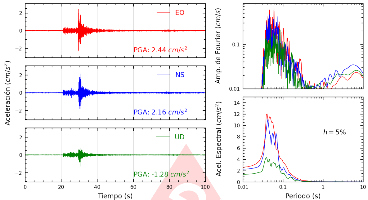
Figura A.17: Registros tiempo-historia, espectros de Fourier y de respuesta en las direcciones EO, NS y vertical de la estación CEPRE. Sismo de Provincia Constitucional del Callao , Callao - Lima del 2024-05-04, 22:17:27 (Hora local)
