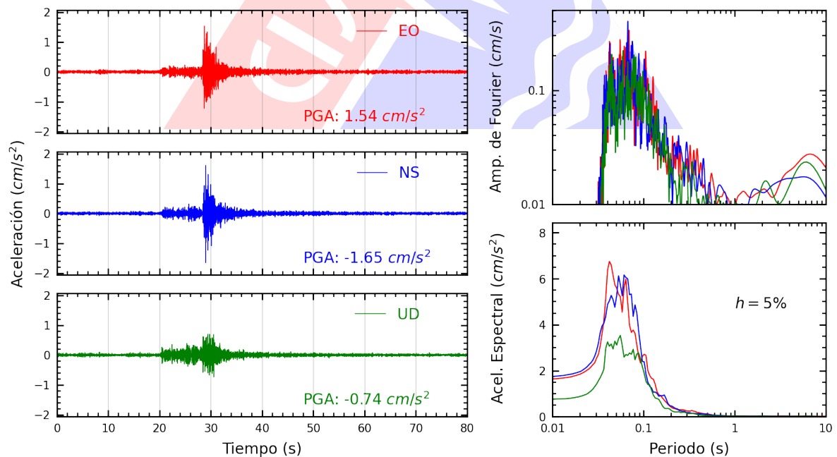
Figura A.22: Registros tiempo-historia, espectros de Fourier y de respuesta en las direcciones EO, NS y vertical de la estación MADRE. Sismo de Provincia Constitucional del Callao , Callao - Lima del 2024-05-04, 22:17:27 (Hora local)
