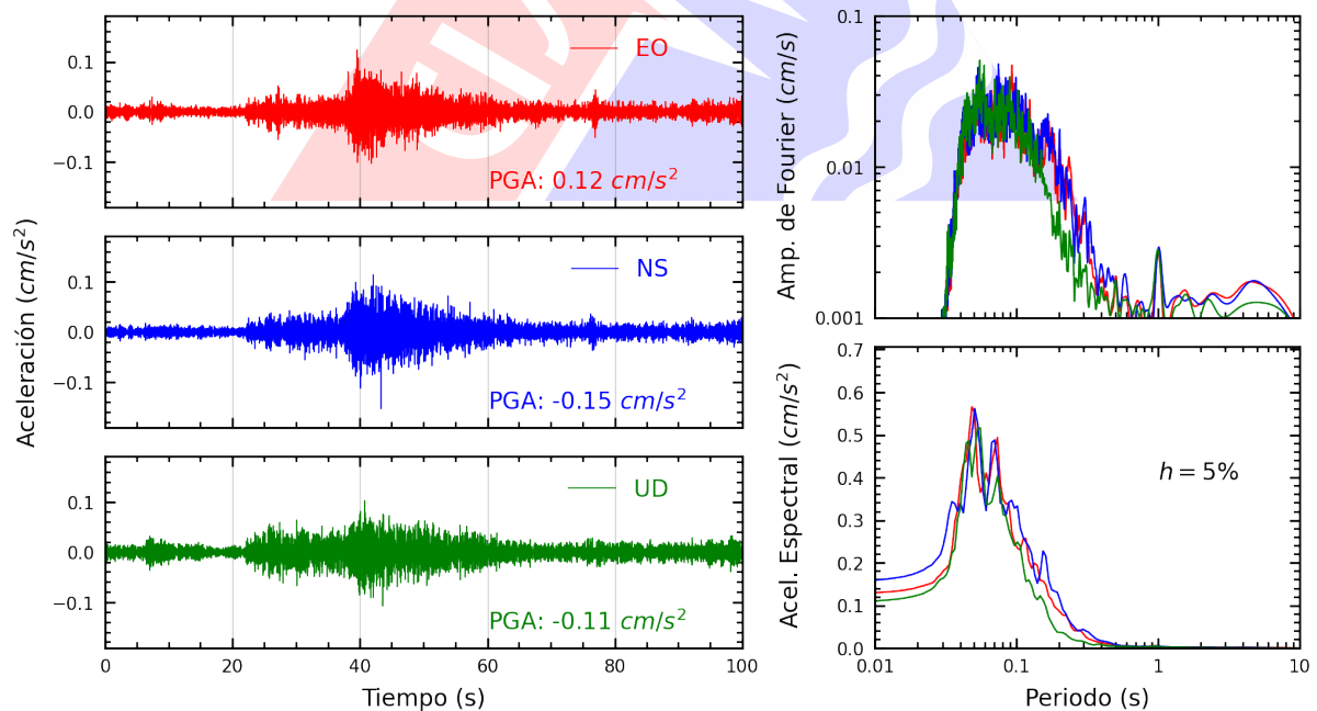
Figura A.38: Registros tiempo-historia, espectros de Fourier y de respuesta en las direcciones EO, NS y vertical de la estación ASIA. Sismo de Provincia Constitucional del Callao , Callao - Lima del 2024-05-04, 22:17:27 (Hora local)
