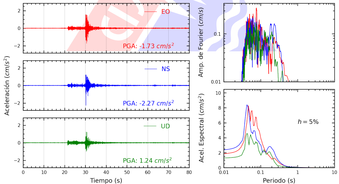
Figura A.18: Registros tiempo-historia, espectros de Fourier y de respuesta en las direcciones EO, NS y vertical de la estación BORJA. Sismo de Provincia Constitucional del Callao , Callao - Lima del 2024-05-04, 22:17:27 (Hora local)
