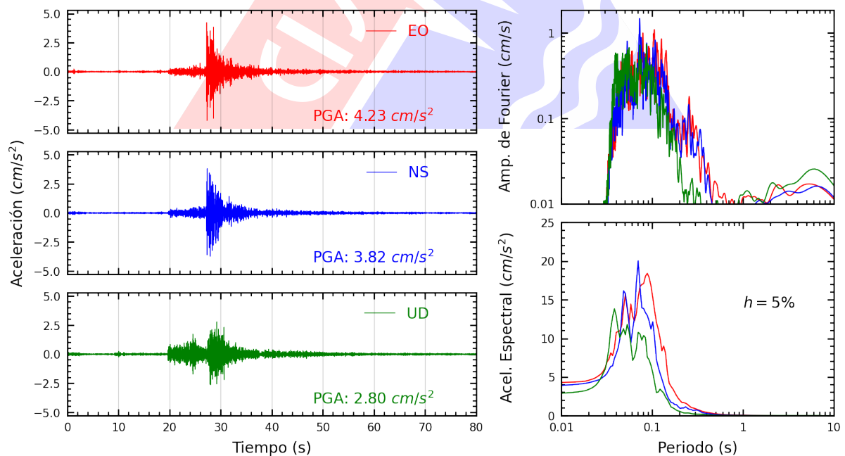
Figura A.6: Registros tiempo-historia, espectros de Fourier y de respuesta en las direcciones EO, NS y vertical de la estación ANCON. Sismo de Provincia Constitucional del Callao , Callao - Lima del 2024-05-04, 22:17:27 (Hora local)
