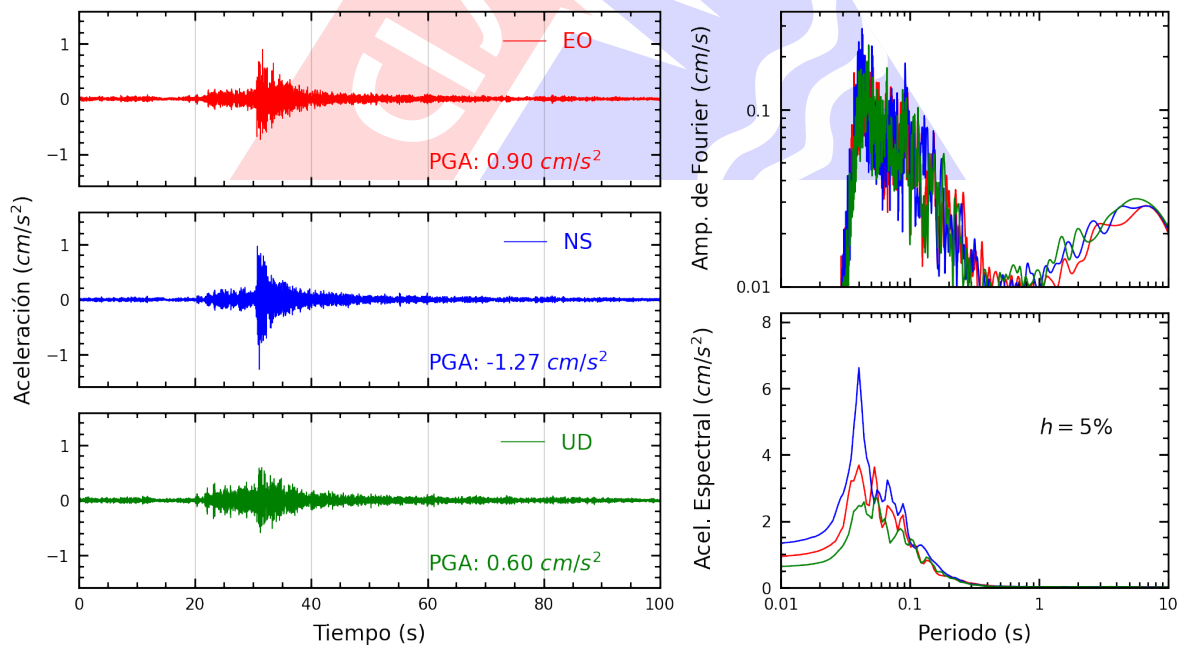
Figura A.26: Registros tiempo-historia, espectros de Fourier y de respuesta en las direcciones EO, NS y vertical de la estación USMP. Sismo de Provincia Constitucional del Callao , Callao - Lima del 2024-05-04, 22:17:27 (Hora local)
