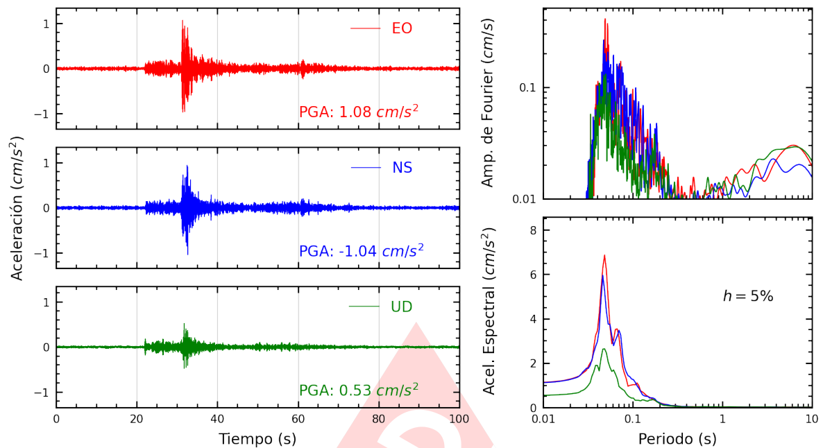
Figura A.27: Registros tiempo-historia, espectros de Fourier y de respuesta en las direcciones EO, NS y vertical de la estación UPCVI. Sismo de Provincia Constitucional del Callao , Callao - Lima del 2024-05-04, 22:17:27 (Hora local)
