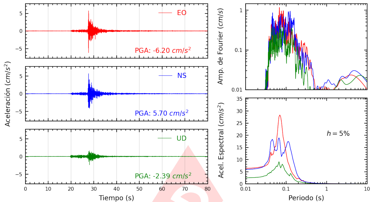
Figura A.3: Registros tiempo-historia, espectros de Fourier y de respuesta en las direcciones EO, NS y vertical de la estación DEFEN. Sismo de Provincia Constitucional del Callao , Callao - Lima del 2024-05-04, 22:17:27 (Hora local)
