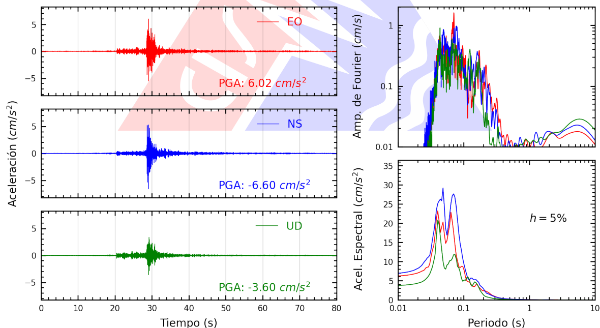
Figura A.2: Registros tiempo-historia, espectros de Fourier y de respuesta en las direcciones EO, NS y vertical de la estación INDEP. Sismo de Provincia Constitucional del Callao , Callao - Lima del 2024-05-04, 22:17:27 (Hora local)
