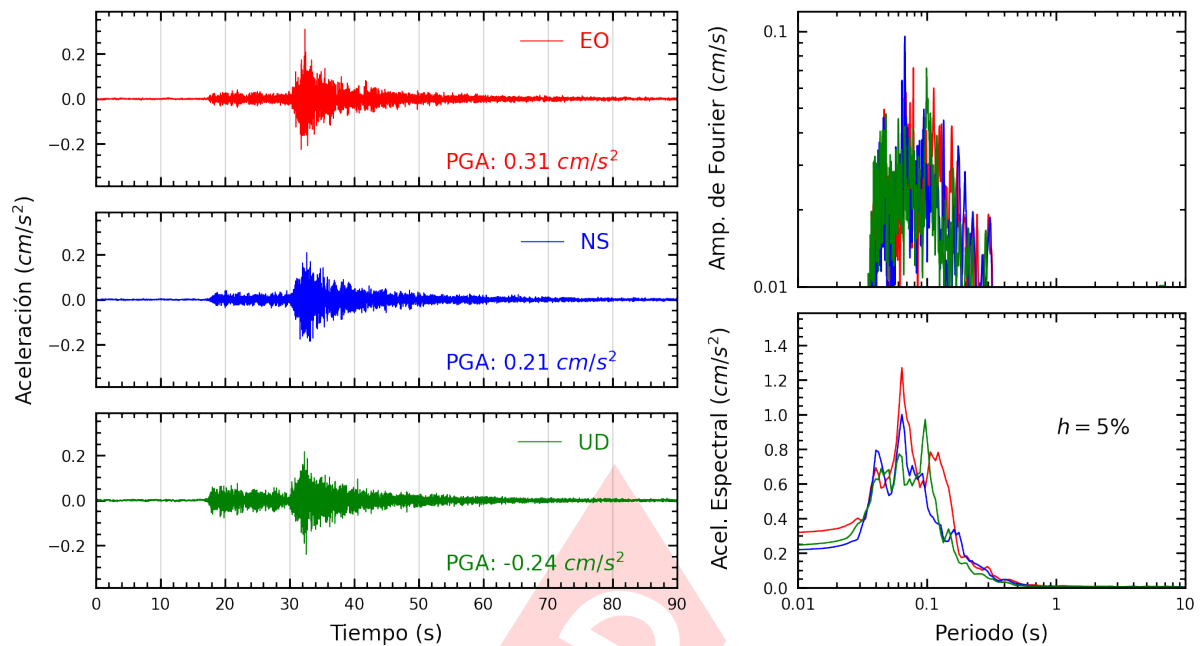
Figura A.37: Registros tiempo-historia, espectros de Fourier y de respuesta en las direcciones EO, NS y vertical de la estación CARAL. Sismo de Provincia Constitucional del Callao , Callao - Lima del 2024-05-04, 22:17:27 (Hora local)
