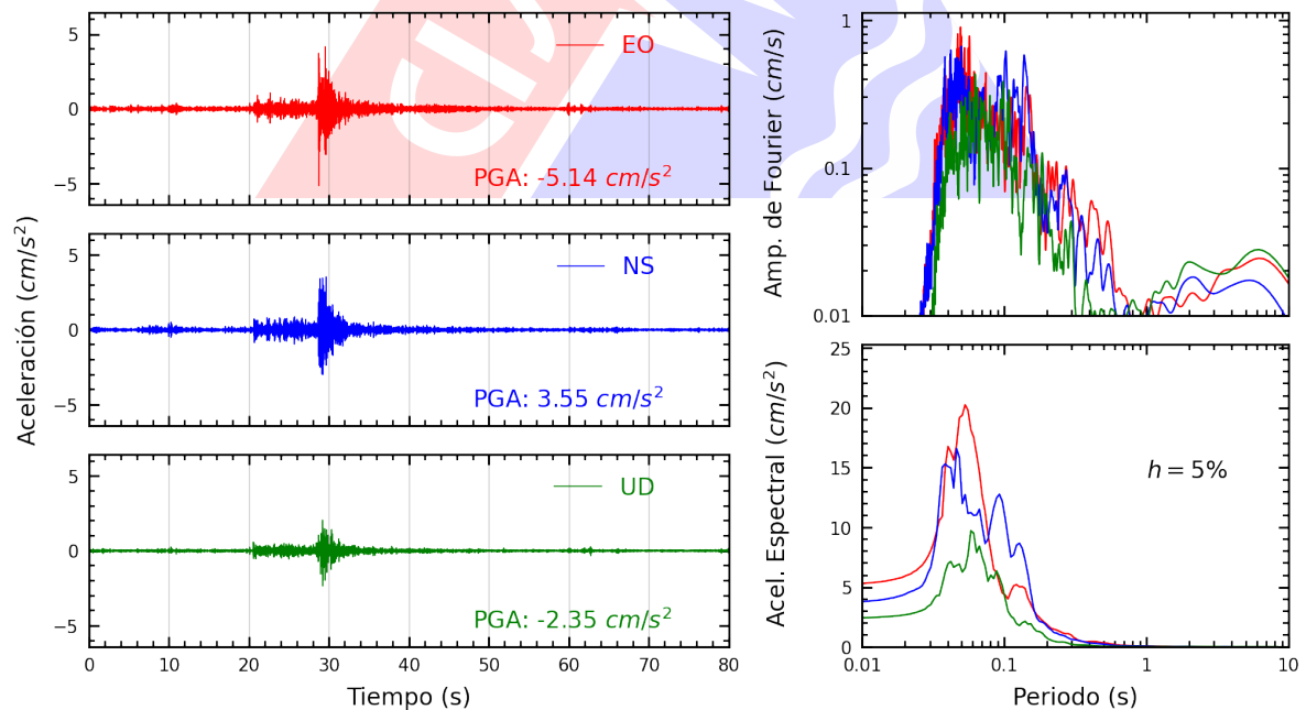
Figura A.4: Registros tiempo-historia, espectros de Fourier y de respuesta en las direcciones EO, NS y vertical de la estación OLIVO. Sismo de Provincia Constitucional del Callao , Callao - Lima del 2024-05-04, 22:17:27 (Hora local)
