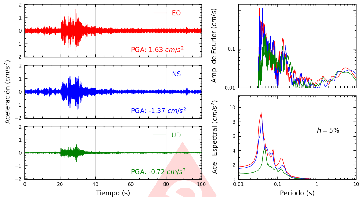
Figura A.23: Registros tiempo-historia, espectros de Fourier y de respuesta en las direcciones EO, NS y vertical de la estación DHNPE. Sismo de Provincia Constitucional del Callao , Callao - Lima del 2024-05-04, 22:17:27 (Hora local)
