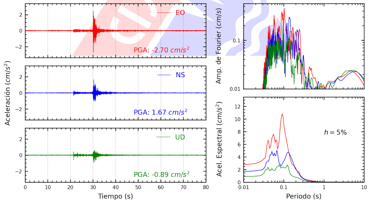
Figura A.14: Registros tiempo-historia, espectros de Fourier y de respuesta en las direcciones EO, NS y vertical de la estación INICT. Sismo de Provincia Constitucional del Callao , Callao - Lima del 2024-05-04, 22:17:27 (Hora local)
