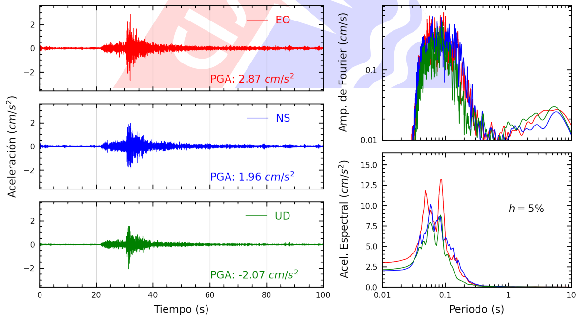
Figura A.10: Registros tiempo-historia, espectros de Fourier y de respuesta en las direcciones EO, NS y vertical de la estación USILM. Sismo de Provincia Constitucional del Callao , Callao - Lima del 2024-05-04, 22:17:27 (Hora local)
