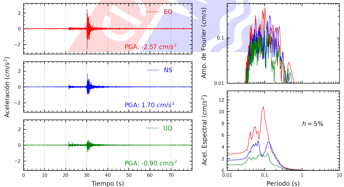
Figura A.16: Registros tiempo-historia, espectros de Fourier y de respuesta en las direcciones EO, NS y vertical de la estación INIC2. Sismo de Provincia Constitucional del Callao , Callao - Lima del 2024-05-04, 22:17:27 (Hora local)
