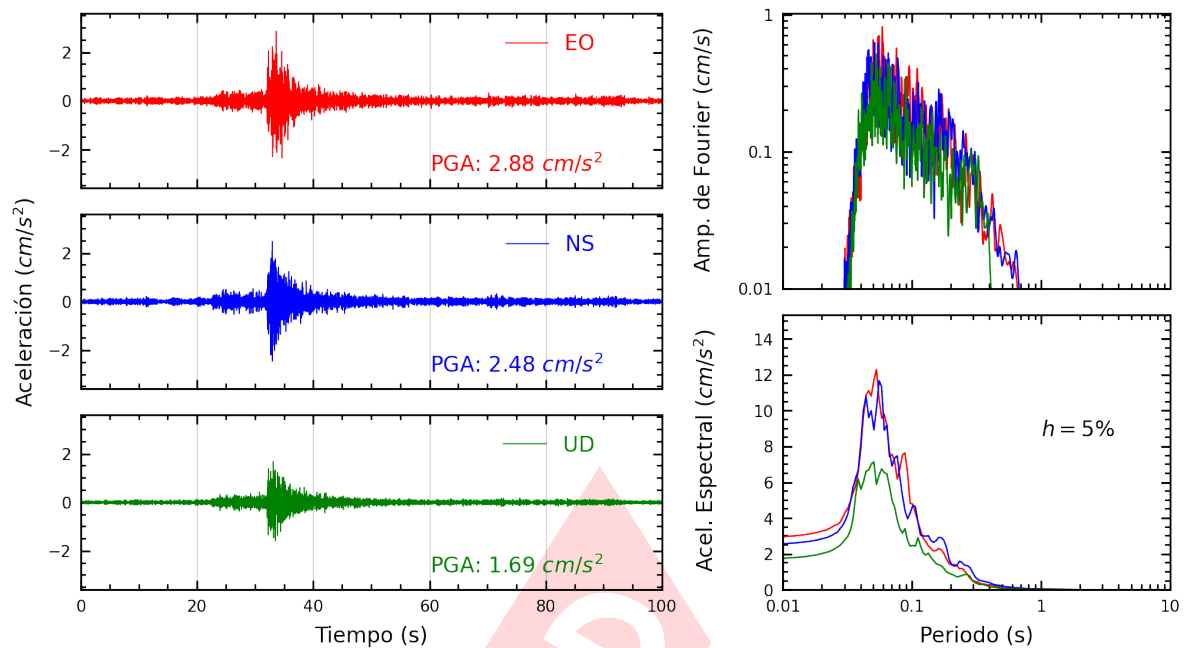
Figura A.9: Registros tiempo-historia, espectros de Fourier y de respuesta en las direcciones EO, NS y vertical de la estación UNTEL. Sismo de Provincia Constitucional del Callao , Callao - Lima del 2024-05-04, 22:17:27 (Hora local)
