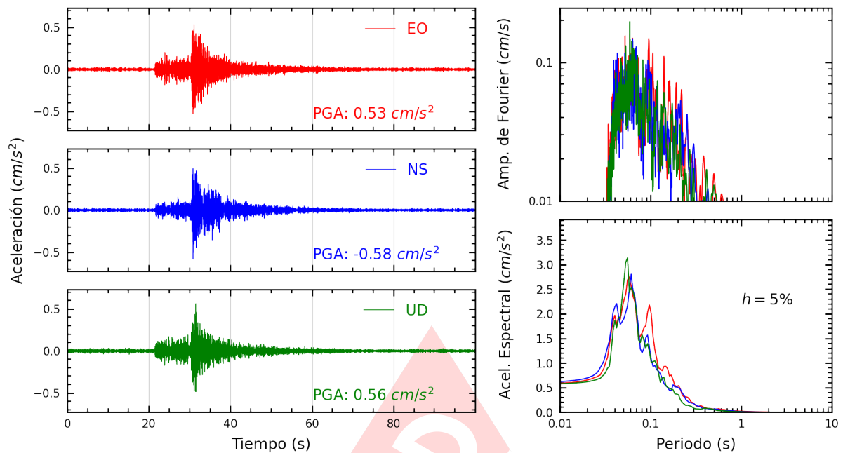
Figura A.33: Registros tiempo-historia, espectros de Fourier y de respuesta en las direcciones EO, NS y vertical de la estación IMCA2. Sismo de Provincia Constitucional del Callao , Callao - Lima del 2024-05-04, 22:17:27 (Hora local)
