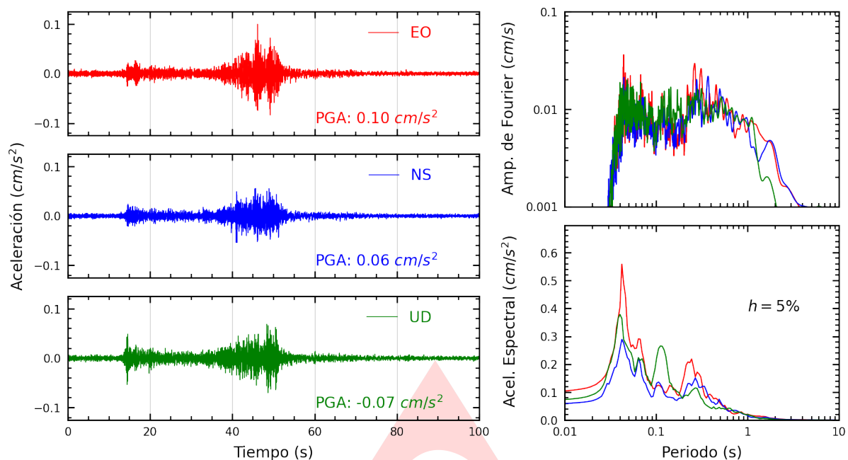
Figura A.1: Registros tiempo-historia, espectros de Fourier y de respuesta en las direcciones EO, NS y vertical de la estación UNCP. Sismo de Atalaya, Atalaya - Ucayali del 2024-05-07, 16:44:27 (Hora local)
