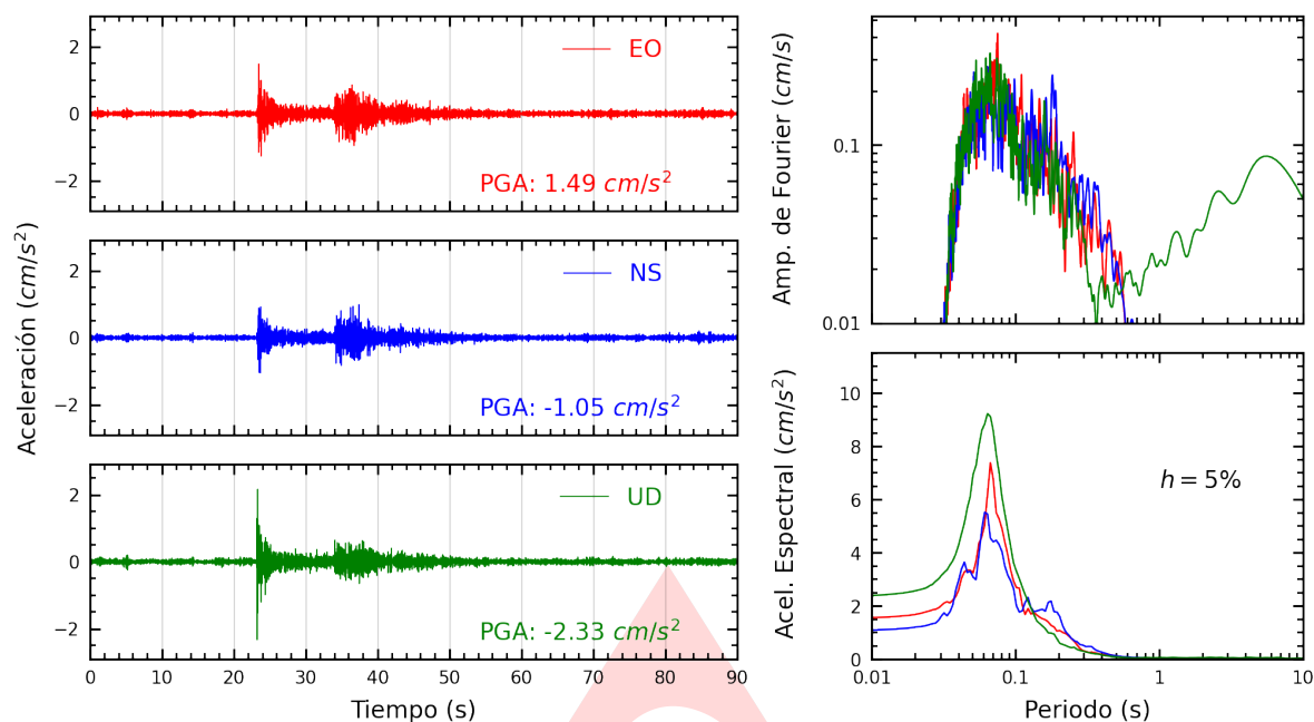
Figura A.1: Registros tiempo-historia, espectros de Fourier y de respuesta en las direcciones EO, NS y vertical de la estación SCARQ. Sismo de Mollendo, Islay - Arequipa del 2024-06-05, 12:14:28 (Hora local)
