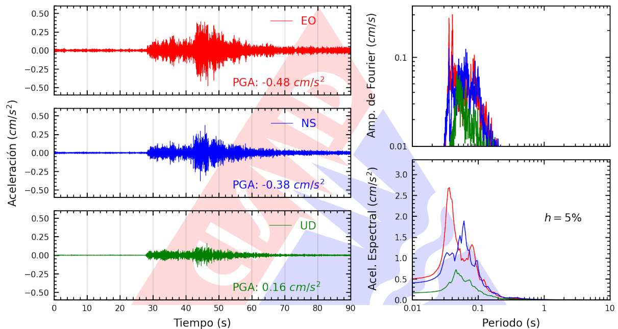
Figura A.3: Registros tiempo-historia, espectros de Fourier y de respuesta en las direcciones EO, NS y vertical de la estación UNAM. Sismo de Mollendo, Islay - Arequipa del 2024-06-05, 12:14:28 (Hora local)
