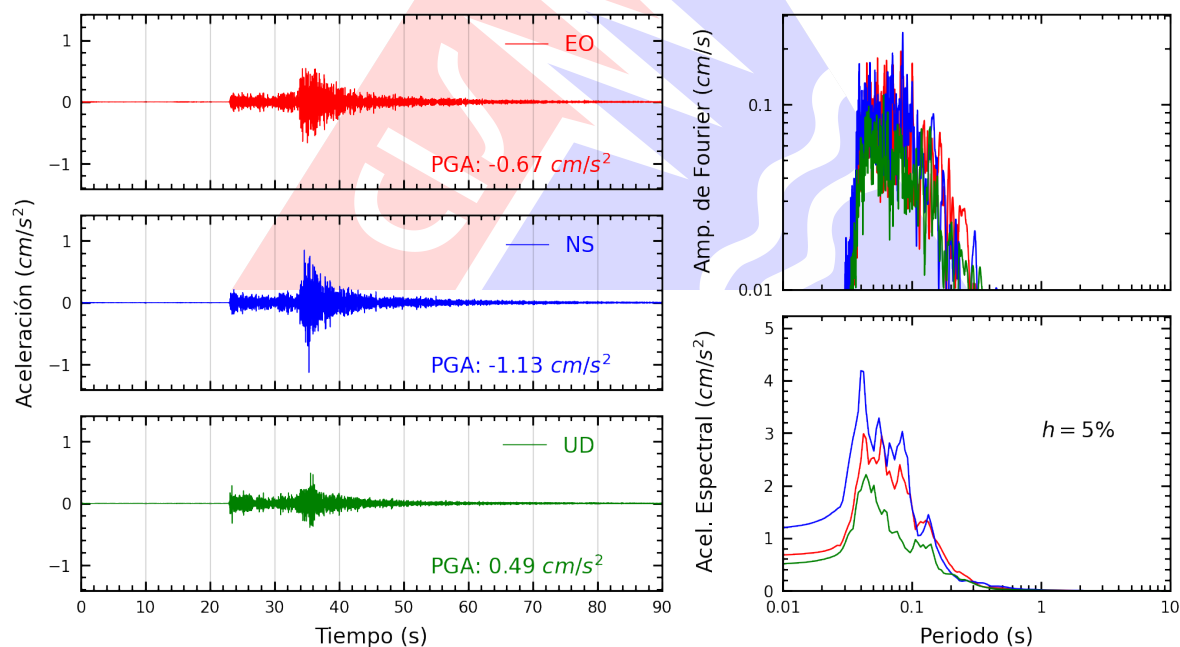
Figura A.2: Registros tiempo-historia, espectros de Fourier y de respuesta en las direcciones EO, NS y vertical de la estación UNSA2. Sismo de Mollendo, Islay - Arequipa del 2024-06-05, 12:14:28 (Hora local)
