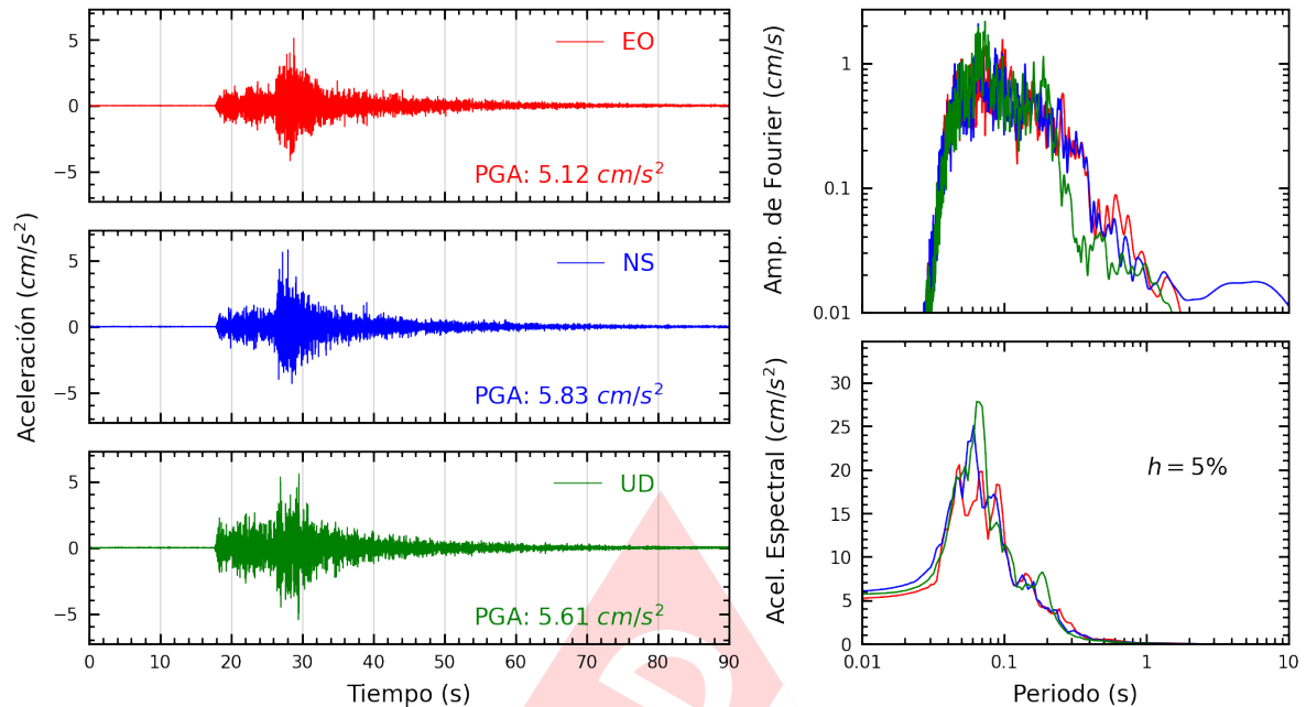
Figura A.3: Registros tiempo-historia, espectros de Fourier y de respuesta en las direcciones EO, NS y vertical de la estación SCTAC. Sismo de Tacna, Tacna - Tacna del 2024-06-07, 00:47:34 (Hora local)
