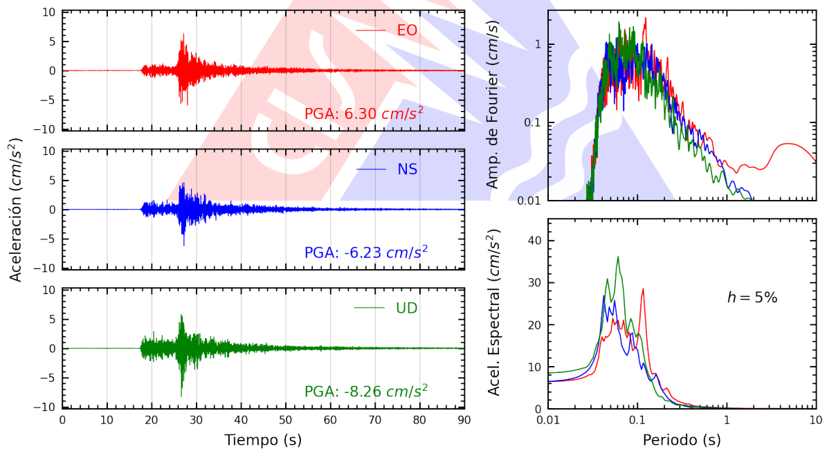
Figura A.2: Registros tiempo-historia, espectros de Fourier y de respuesta en las direcciones EO, NS y vertical de la estación UJBG3. Sismo de Tacna, Tacna - Tacna del 2024-06-07, 00:47:34 (Hora local)
