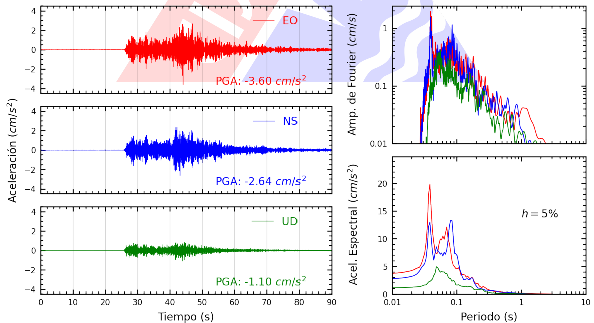
Figura A.4: Registros tiempo-historia, espectros de Fourier y de respuesta en las direcciones EO, NS y vertical de la estación UNAM. Sismo de Tacna, Tacna - Tacna del 2024-06-07, 00:47:34 (Hora local)
