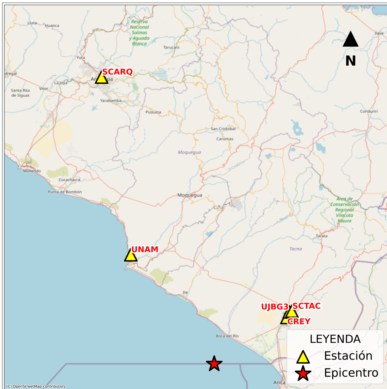
Figura 2: Mapa de ubicación de la(s) estación(es) acelerográfica(s) correspondiente(s) al Sismo de Tacna, Tacna - Tacna del 07 de junio de 2024 a las 00:47:34 (hora local)
