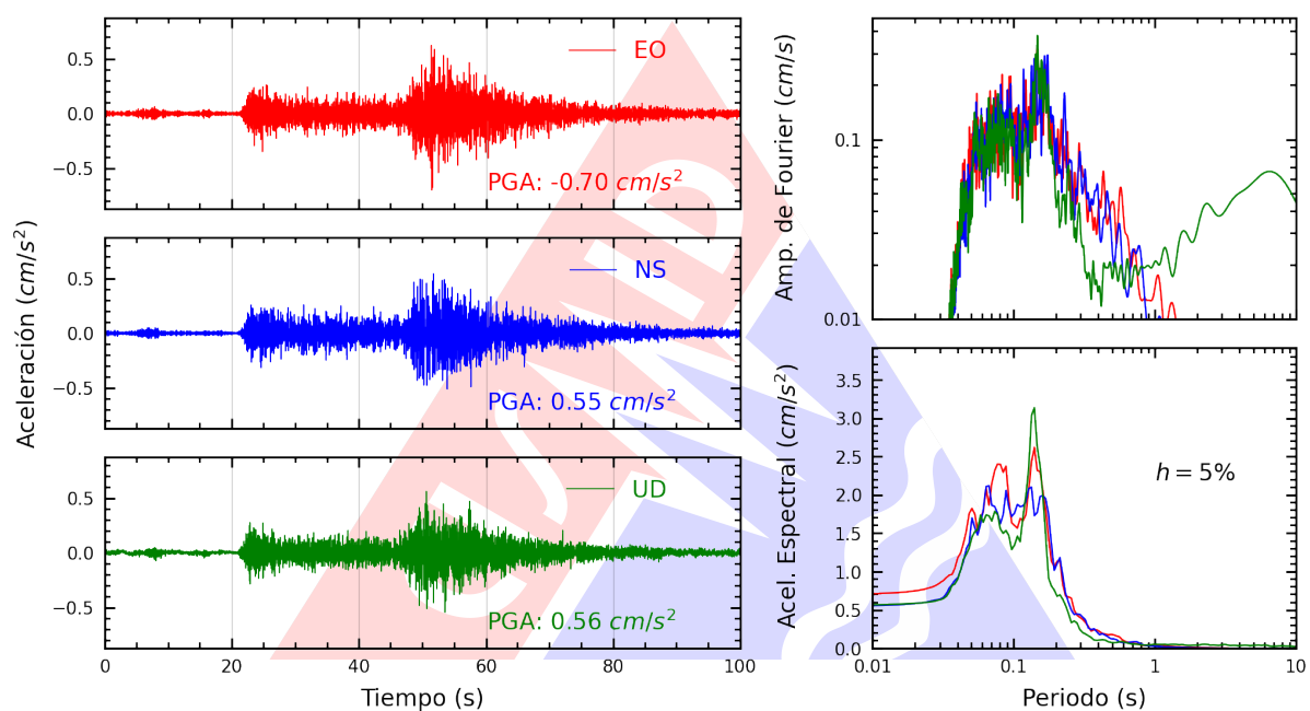
Figura A.5: Registros tiempo-historia, espectros de Fourier y de respuesta en las direcciones EO, NS y vertical de la estación SCARQ. Sismo de Tacna, Tacna - Tacna del 2024-06-07, 00:47:34 (Hora local)
