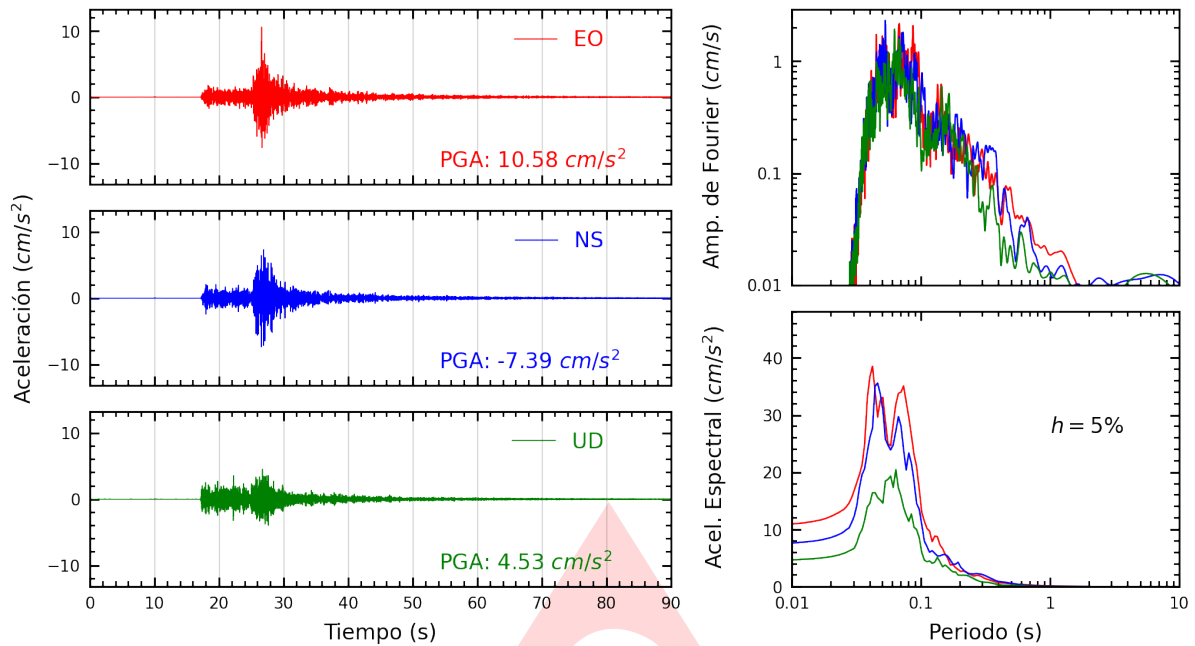
Figura A.1: Registros tiempo-historia, espectros de Fourier y de respuesta en las direcciones EO, NS y vertical de la estación CREY. Sismo de Tacna, Tacna - Tacna del 2024-06-07, 00:47:34 (Hora local)
