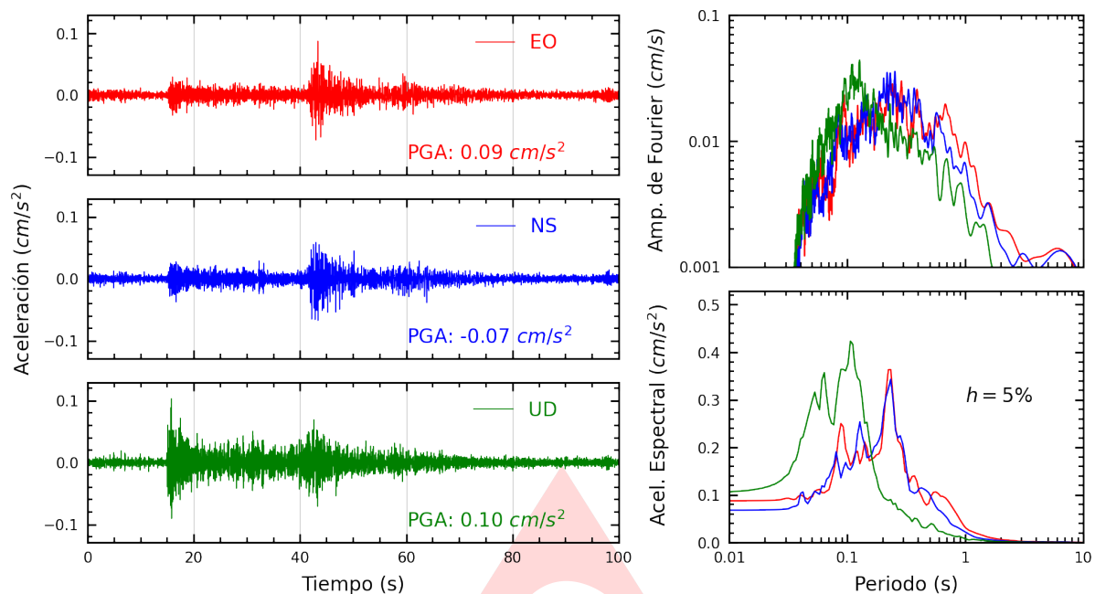
Figura A.1: Registros tiempo-historia, espectros de Fourier y de respuesta en las direcciones EO, NS y vertical de la estación UNIA. Sismo de Picota, Picota - San Martín del 2024-06-10, 07:51:29 (Hora local)
