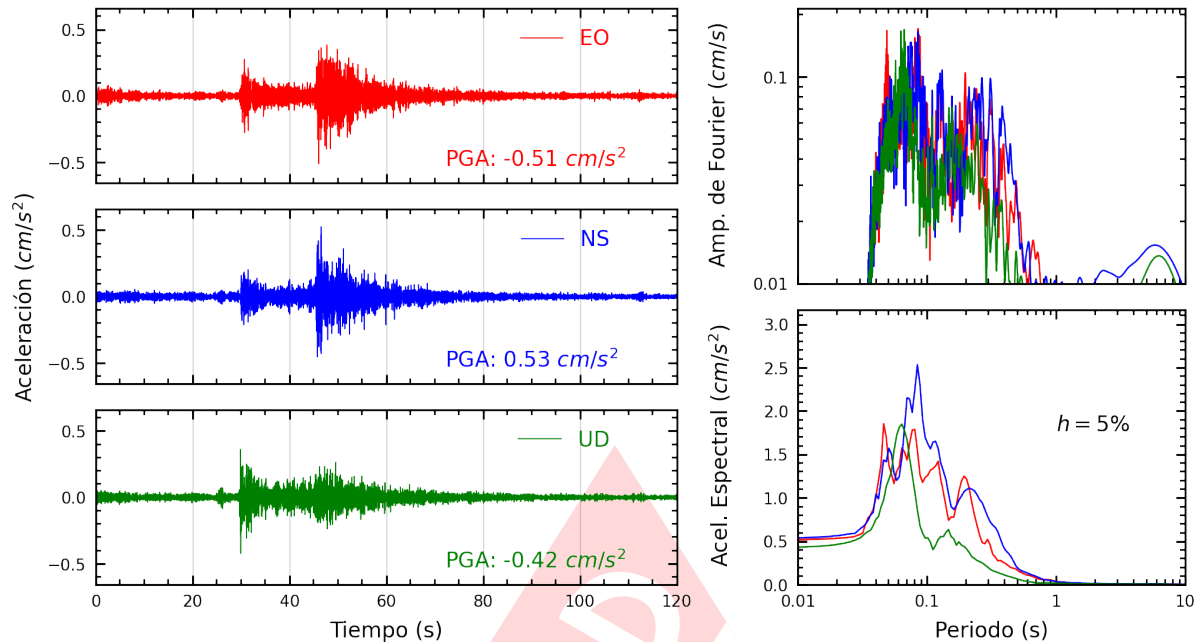
Figura A.3: Registros tiempo-historia, espectros de Fourier y de respuesta en las direcciones EO, NS y vertical de la estación CREY. Sismo de Calana, Tacna - Tacna del 2024-06-13, 15:56:18 (Hora local)
