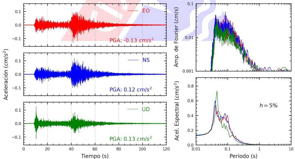
Figura A.4: Registros tiempo-historia, espectros de Fourier y de respuesta en las direcciones EO, NS y vertical de la estación UNSA2. Sismo de Calana, Tacna - Tacna del 2024-06-13, 15:56:18 (Hora local)
