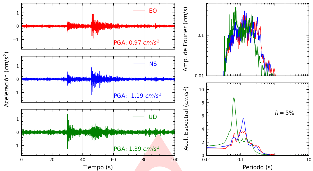
Figura A.1: Registros tiempo-historia, espectros de Fourier y de respuesta en las direcciones EO, NS y vertical de la estación SCTAC. Sismo de Calana, Tacna - Tacna del 2024-06-13, 15:56:18 (Hora local)
