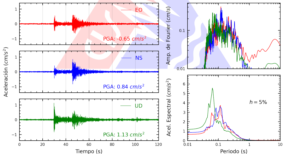
Figura A.2: Registros tiempo-historia, espectros de Fourier y de respuesta en las direcciones EO, NS y vertical de la estación UJBG3. Sismo de Calana, Tacna - Tacna del 2024-06-13, 15:56:18 (Hora local)
