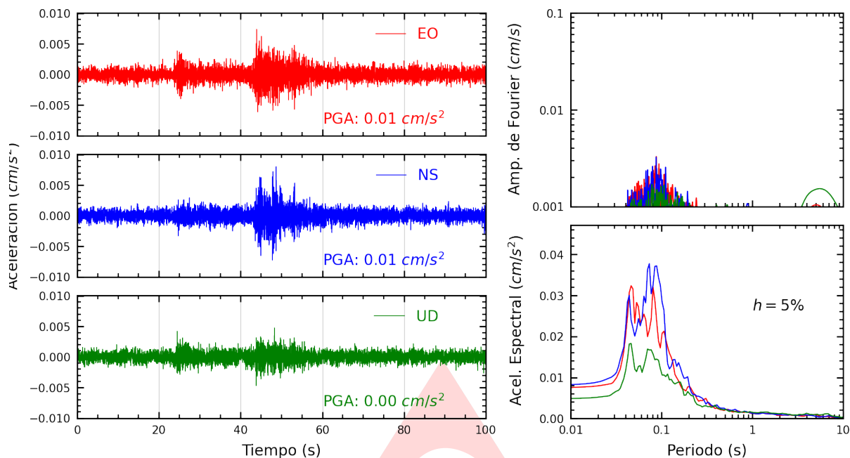
Figura A.1: Registros tiempo-historia, espectros de Fourier y de respuesta en las direcciones EO, NS y vertical de la estación UNSA2. Sismo de Chivay, Caylloma - Arequipa del 2024-06-13, 16:39:36 (Hora local)
