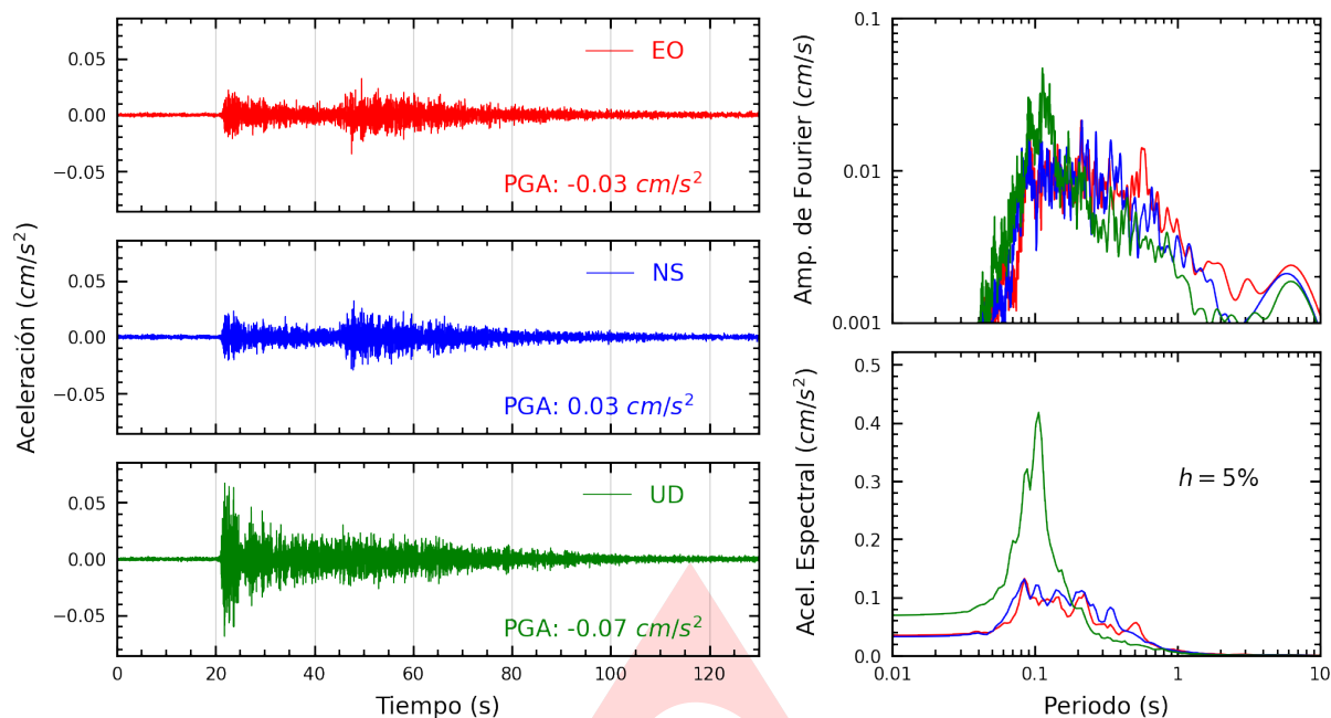
Figura A.1: Registros tiempo-historia, espectros de Fourier y de respuesta en las direcciones EO, NS y vertical de la estación UNIA. Sismo de Aucayacu, Leoncio Prado - Huanuco del 2024-06-14, 02:52:18 (Hora local)
