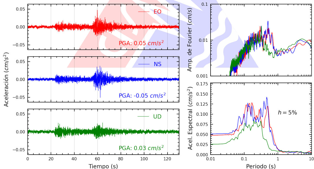
Figura A.2: Registros tiempo-historia, espectros de Fourier y de respuesta en las direcciones EO, NS y vertical de la estación CARAL. Sismo de Aucayacu, Leoncio Prado - Huanuco del 2024-06-14, 02:52:18 (Hora local)
