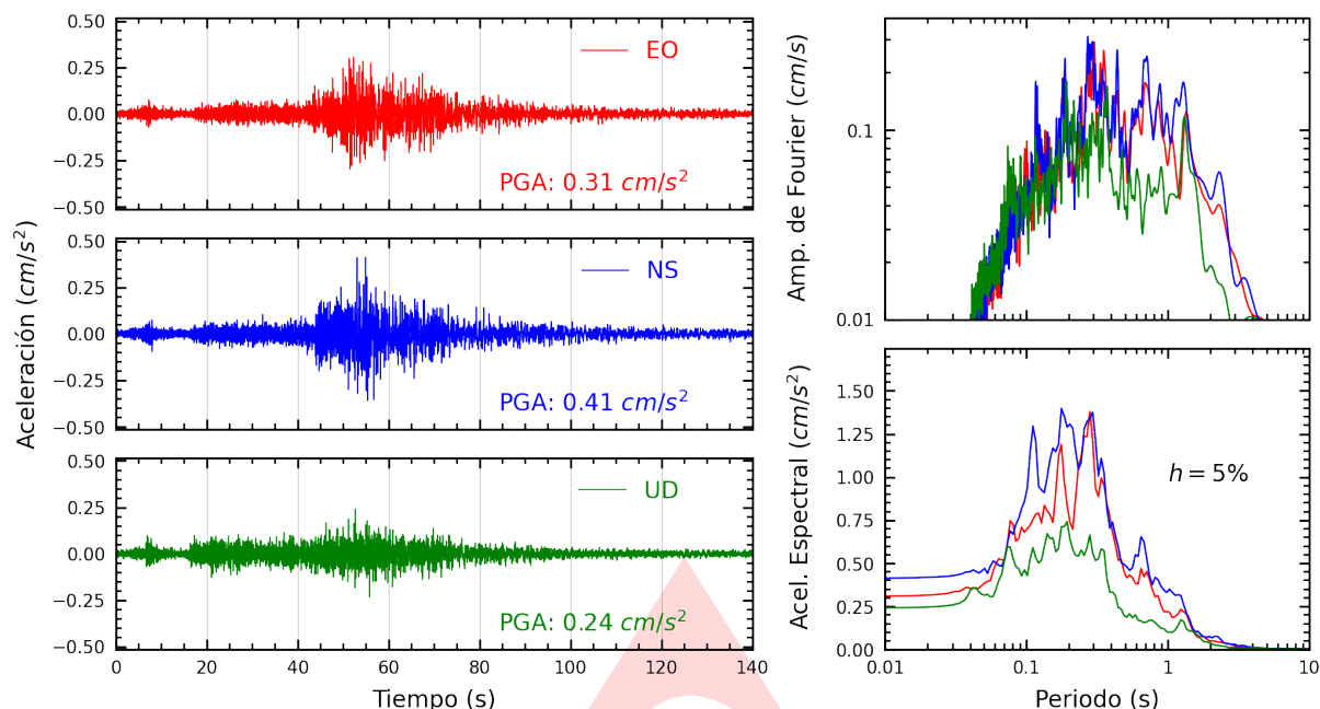
Figura A.1: Registros tiempo-historia, espectros de Fourier y de respuesta en las direcciones EO, NS y vertical de la estación UNICA. Sismo de Chala, Caraveli - Arequipa del 2024-06-16, 21:23:38 (Hora local)
