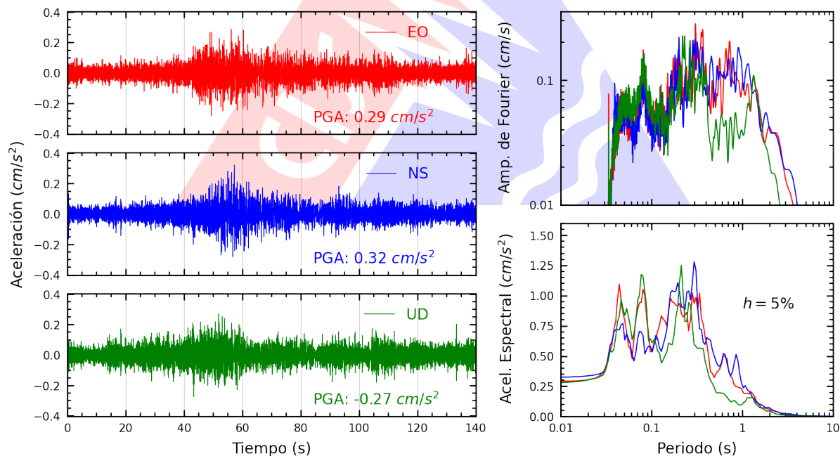
Figura A.2: Registros tiempo-historia, espectros de Fourier y de respuesta en las direcciones EO, NS y vertical de la estación SCICA. Sismo de Chala, Caraveli - Arequipa del 2024-06-16, 21:23:38 (Hora local)
