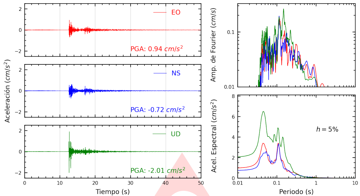
Figura A.1: Registros tiempo-historia, espectros de Fourier y de respuesta en las direcciones EO, NS y vertical de la estación UNCP. Sismo de Jauja, Jauja - Junín del 2024-06-18, 06:14:16 (Hora local)
