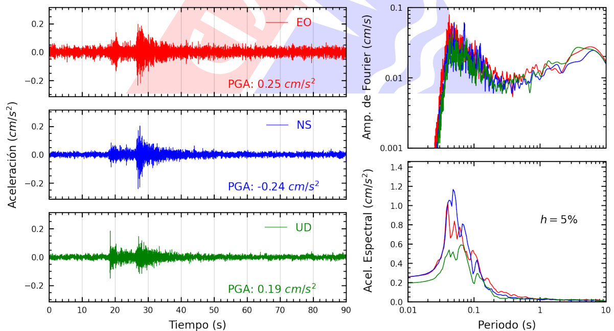
Figura A.20: Registros tiempo-historia, espectros de Fourier y de respuesta en las direcciones EO, NS y vertical de la estación INICT. Sismo de Chilca, Cañete - Lima del 2024-06-21, 02:25:56 (Hora local)
