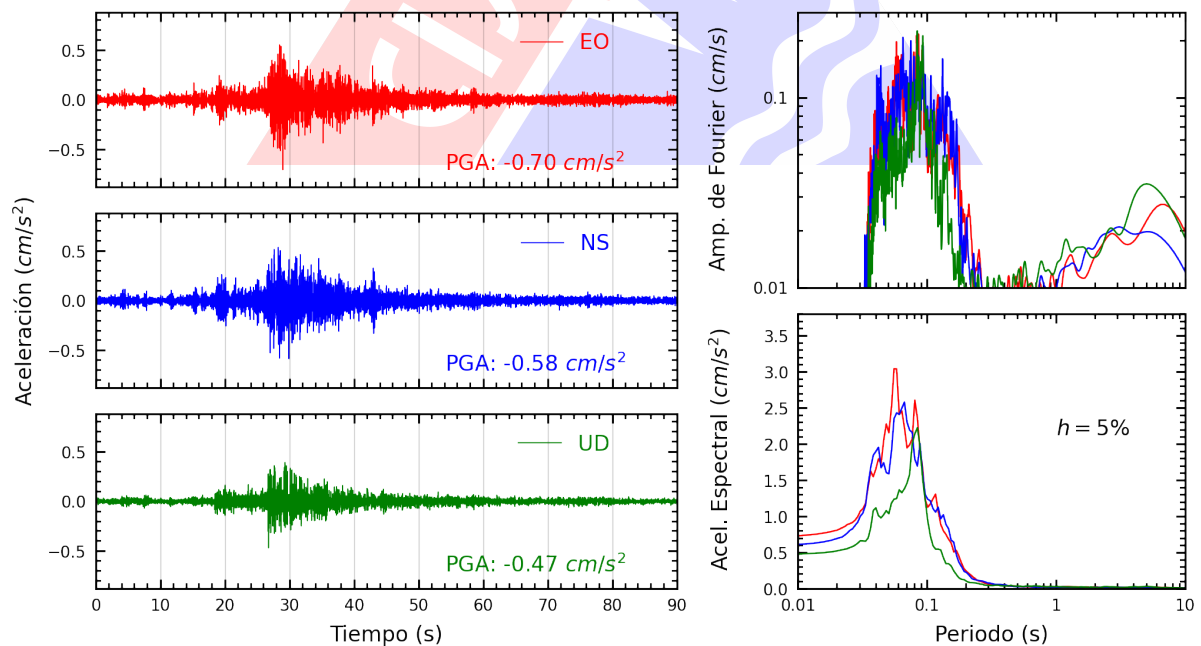
Figura A.4: Registros tiempo-historia, espectros de Fourier y de respuesta en las direcciones EO, NS y vertical de la estación USILM. Sismo de Chilca, Cañete - Lima del 2024-06-21, 02:25:56 (Hora local)
