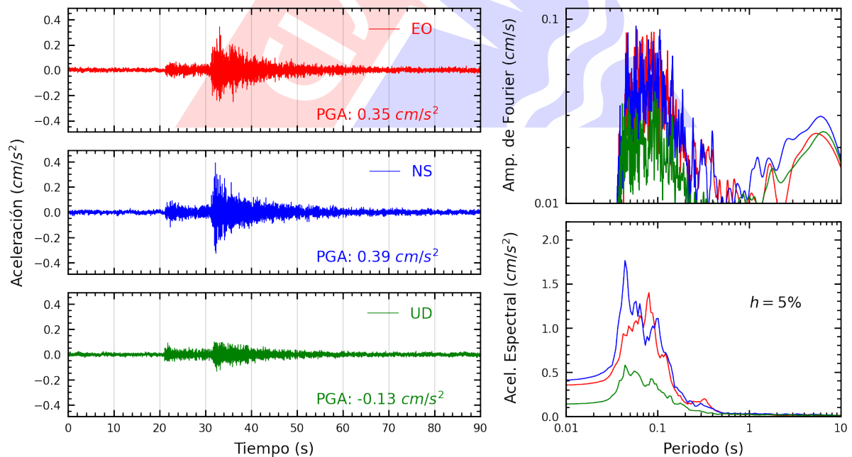
Figura A.14: Registros tiempo-historia, espectros de Fourier y de respuesta en las direcciones EO, NS y vertical de la estación DEFEN. Sismo de Chilca, Cañete - Lima del 2024-06-21, 02:25:56 (Hora local)
