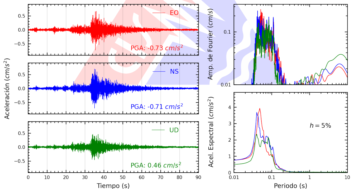
Figura A.2: Registros tiempo-historia, espectros de Fourier y de respuesta en las direcciones EO, NS y vertical de la estación SROSA. Sismo de Chilca, Cañete - Lima del 2024-06-21, 02:25:56 (Hora local)
