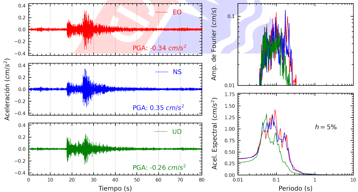
Figura A.16: Registros tiempo-historia, espectros de Fourier y de respuesta en las direcciones EO, NS y vertical de la estación SCCHO. Sismo de Chilca, Cañete - Lima del 2024-06-21, 02:25:56 (Hora local)
