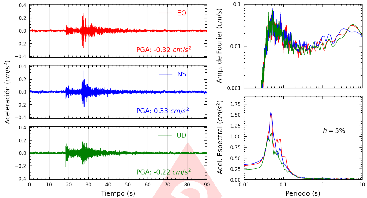
Figura A.17: Registros tiempo-historia, espectros de Fourier y de respuesta en las direcciones EO, NS y vertical de la estación CENEP. Sismo de Chilca, Cañete - Lima del 2024-06-21, 02:25:56 (Hora local)
