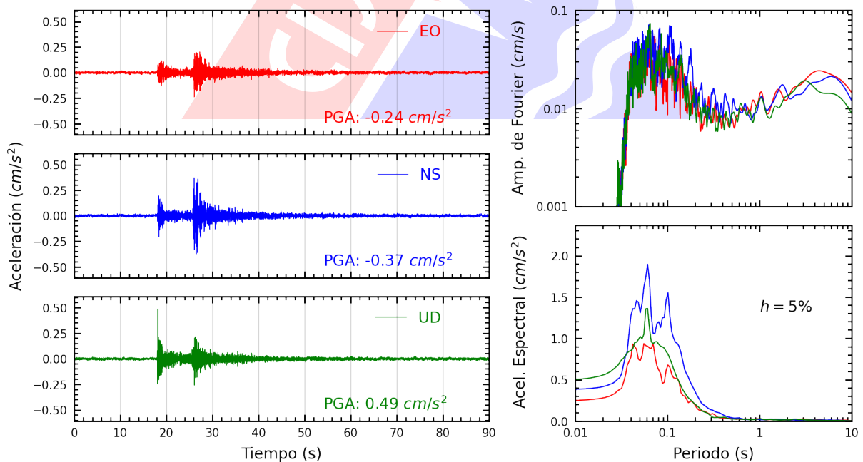
Figura A.8: Registros tiempo-historia, espectros de Fourier y de respuesta en las direcciones EO, NS y vertical de la estación SERVI. Sismo de Chilca, Cañete - Lima del 2024-06-21, 02:25:56 (Hora local)
