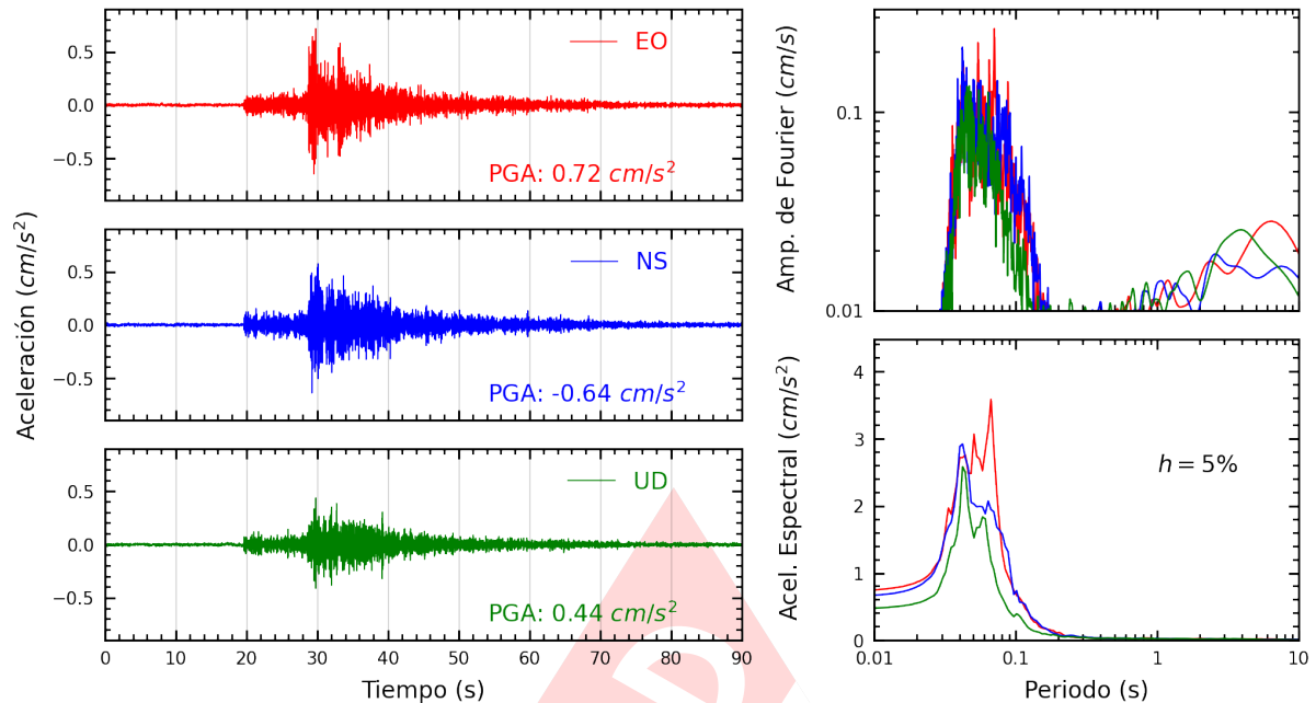
Figura A.3: Registros tiempo-historia, espectros de Fourier y de respuesta en las direcciones EO, NS y vertical de la estación JOSEO. Sismo de Chilca, Cañete - Lima del 2024-06-21, 02:25:56 (Hora local)
