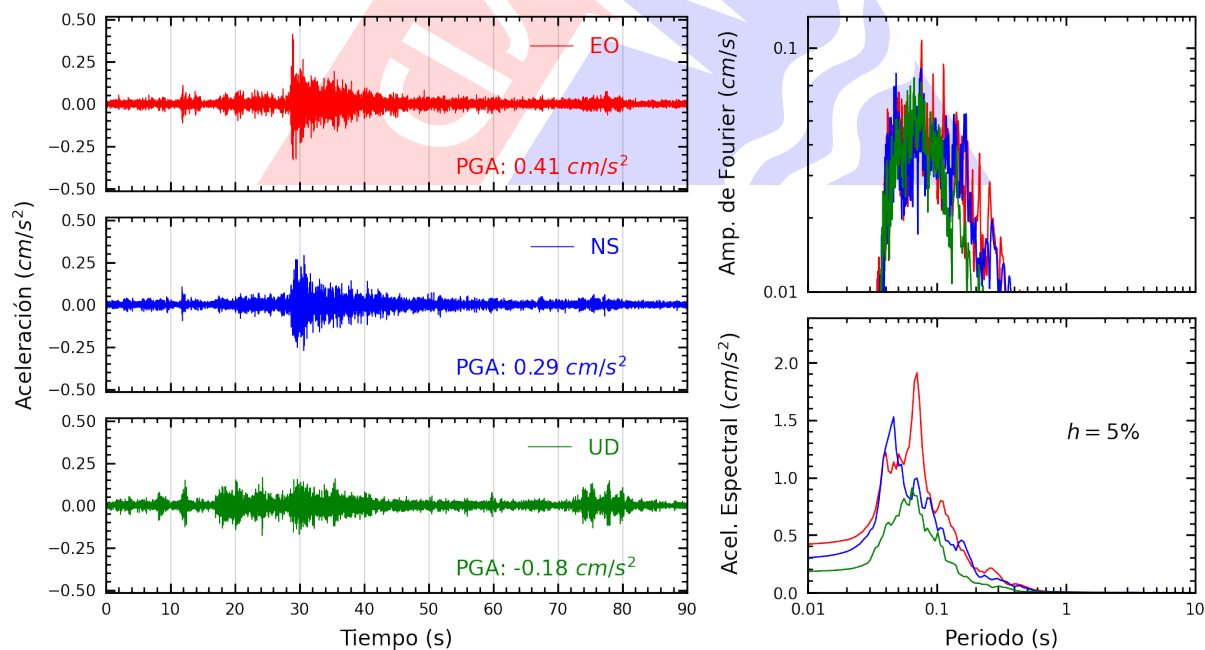
Figura A.12: Registros tiempo-historia, espectros de Fourier y de respuesta en las direcciones EO, NS y vertical de la estación SCOLI. Sismo de Chilca, Cañete - Lima del 2024-06-21, 02:25:56 (Hora local)
