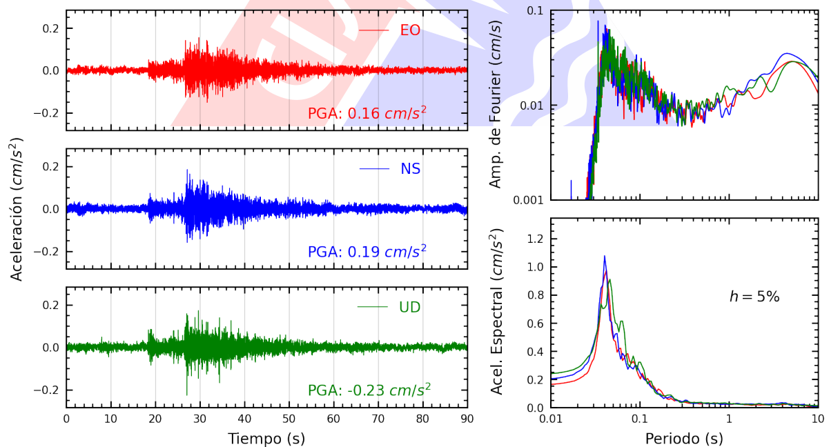
Figura A.22: Registros tiempo-historia, espectros de Fourier y de respuesta en las direcciones EO, NS y vertical de la estación USMP. Sismo de Chilca, Cañete - Lima del 2024-06-21, 02:25:56 (Hora local)
