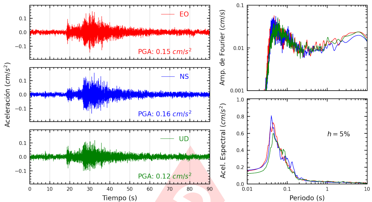
Figura A.25: Registros tiempo-historia, espectros de Fourier y de respuesta en las direcciones EO, NS y vertical de la estación IMCA. Sismo de Chilca, Cañete - Lima del 2024-06-21, 02:25:56 (Hora local)
