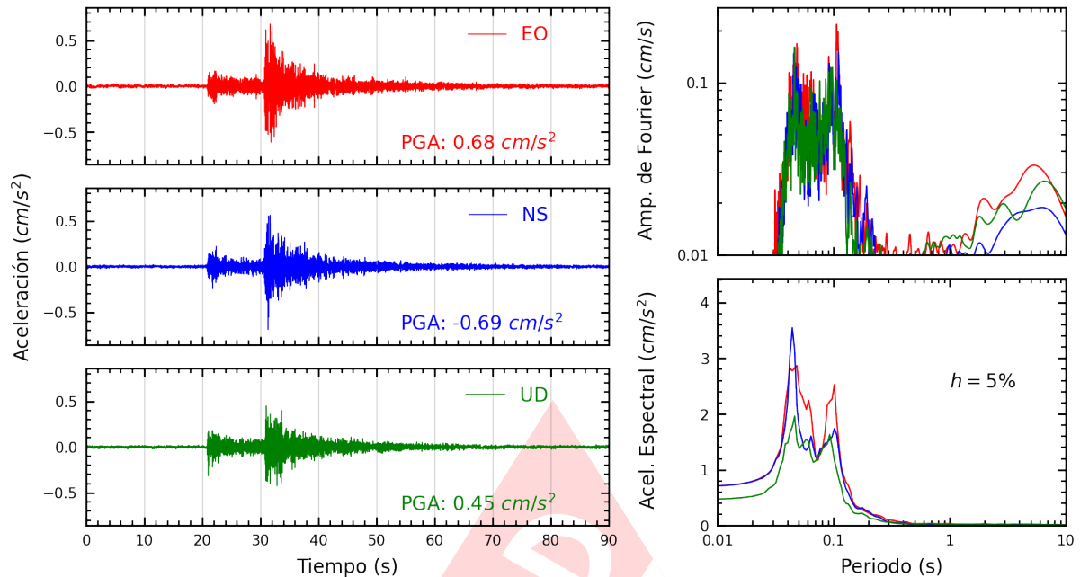
Figura A.5: Registros tiempo-historia, espectros de Fourier y de respuesta en las direcciones EO, NS y vertical de la estación AMORE. Sismo de Chilca, Cañete - Lima del 2024-06-21, 02:25:56 (Hora local)
