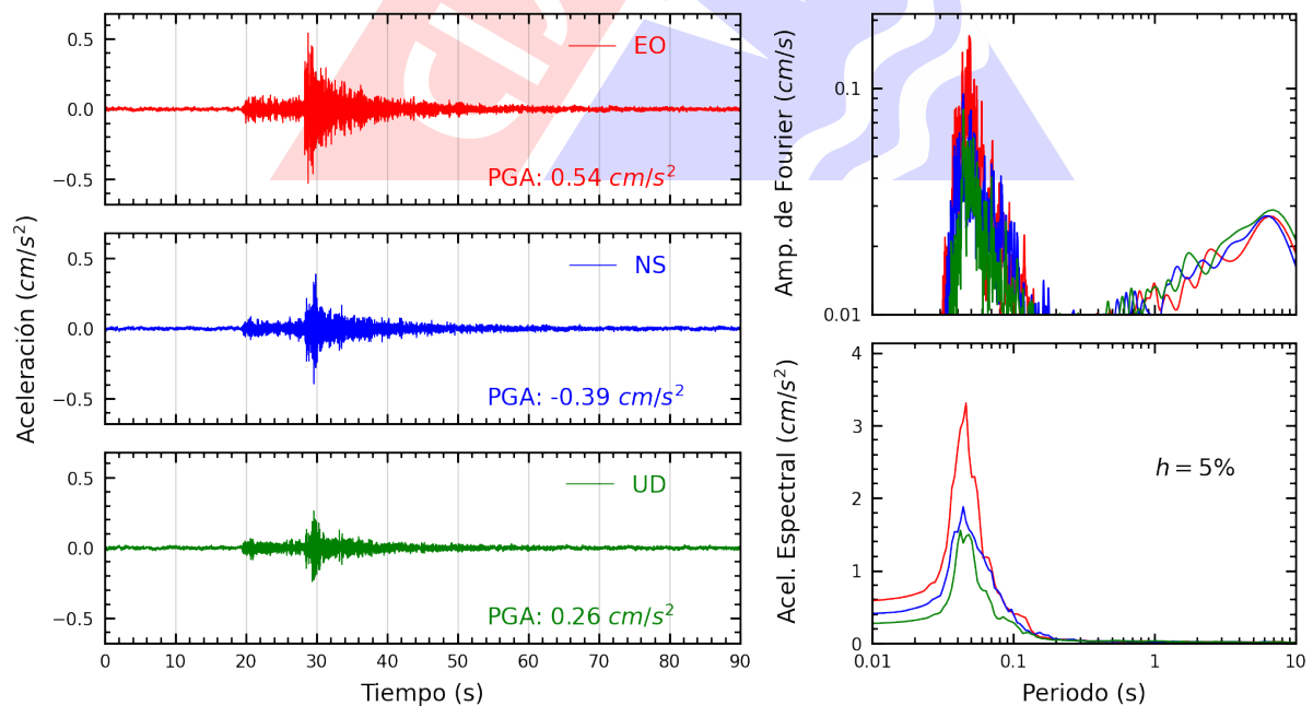
Figura A.6: Registros tiempo-historia, espectros de Fourier y de respuesta en las direcciones EO, NS y vertical de la estación UCSS. Sismo de Chilca, Cañete - Lima del 2024-06-21, 02:25:56 (Hora local)
