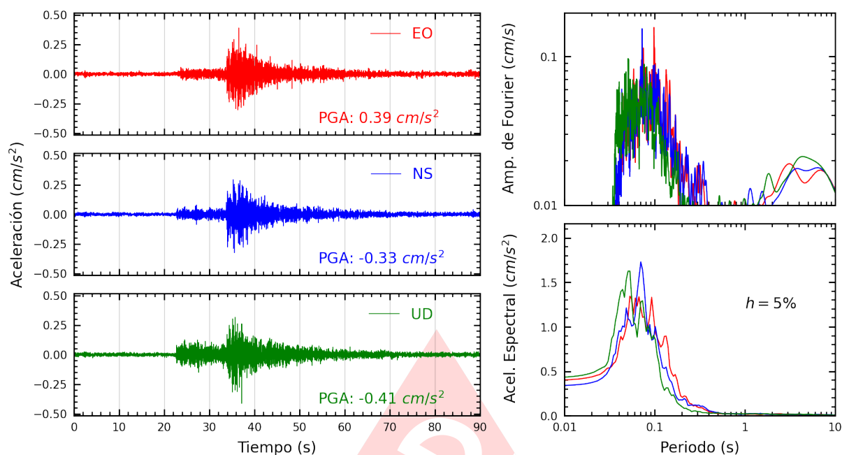
Figura A.11: Registros tiempo-historia, espectros de Fourier y de respuesta en las direcciones EO, NS y vertical de la estación ANCON. Sismo de Chilca, Cañete - Lima del 2024-06-21, 02:25:56 (Hora local)
