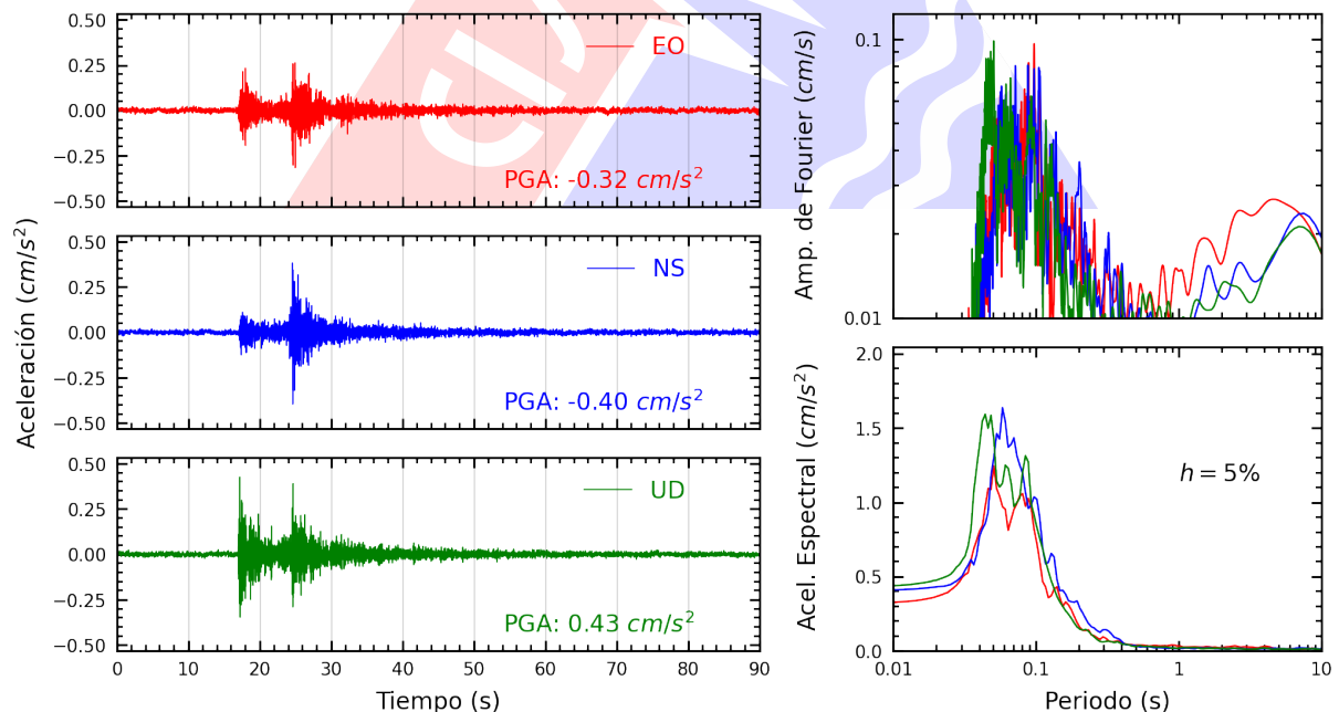
Figura A.10: Registros tiempo-historia, espectros de Fourier y de respuesta en las direcciones EO, NS y vertical de la estación USILP. Sismo de Chilca, Cañete - Lima del 2024-06-21, 02:25:56 (Hora local)
