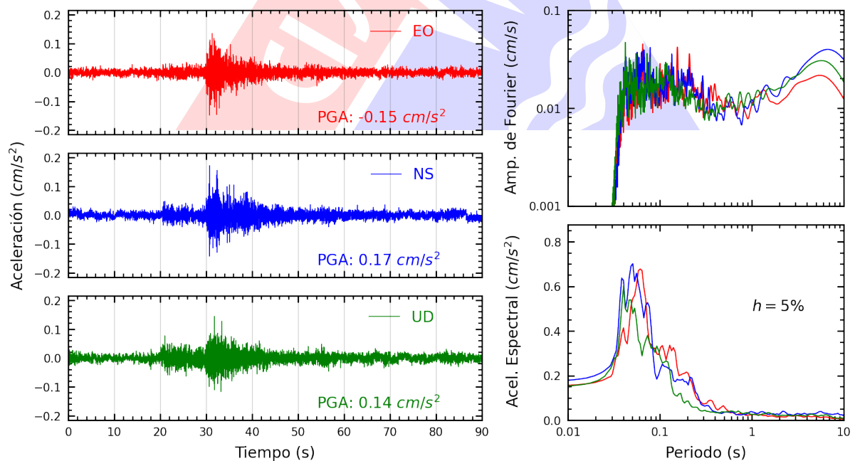
Figura A.24: Registros tiempo-historia, espectros de Fourier y de respuesta en las direcciones EO, NS y vertical de la estación VHAYA. Sismo de Chilca, Cañete - Lima del 2024-06-21, 02:25:56 (Hora local)
