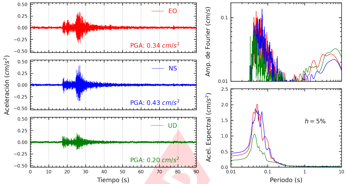
Figura A.9: Registros tiempo-historia, espectros de Fourier y de respuesta en las direcciones EO, NS y vertical de la estación UPCVI. Sismo de Chilca, Cañete - Lima del 2024-06-21, 02:25:56 (Hora local)
