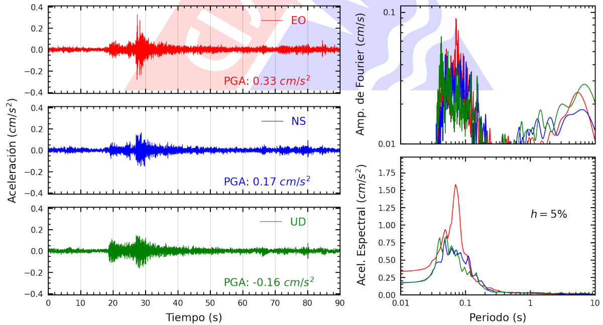
Figura A.18: Registros tiempo-historia, espectros de Fourier y de respuesta en las direcciones EO, NS y vertical de la estación UPCSM. Sismo de Chilca, Cañete - Lima del 2024-06-21, 02:25:56 (Hora local)
