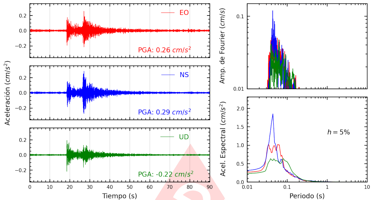
Figura A.19: Registros tiempo-historia, espectros de Fourier y de respuesta en las direcciones EO, NS y vertical de la estación BORJA. Sismo de Chilca, Cañete - Lima del 2024-06-21, 02:25:56 (Hora local)
