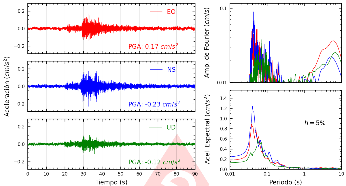
Figura A.21: Registros tiempo-historia, espectros de Fourier y de respuesta en las direcciones EO, NS y vertical de la estación COMAS. Sismo de Chilca, Cañete - Lima del 2024-06-21, 02:25:56 (Hora local)
