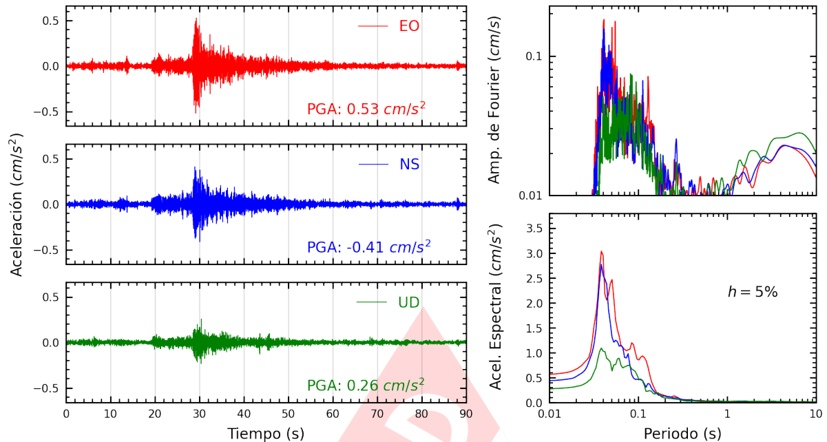
Figura A.7: Registros tiempo-historia, espectros de Fourier y de respuesta en las direcciones EO, NS y vertical de la estación OLIVO. Sismo de Chilca, Cañete - Lima del 2024-06-21, 02:25:56 (Hora local)
