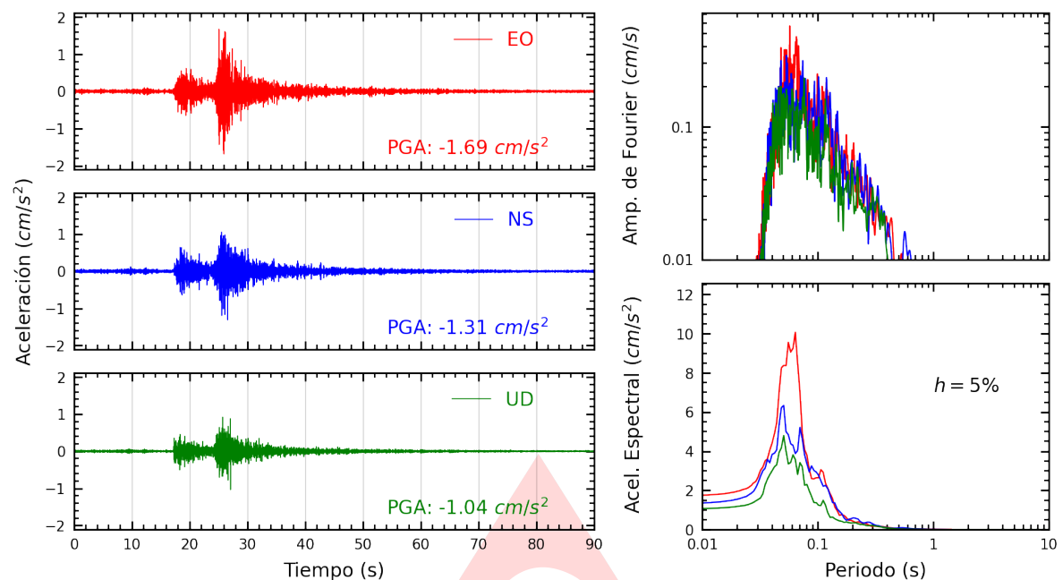
Figura A.1: Registros tiempo-historia, espectros de Fourier y de respuesta en las direcciones EO, NS y vertical de la estación UNTEL. Sismo de Chilca, Cañete - Lima del 2024-06-21, 02:25:56 (Hora local)
