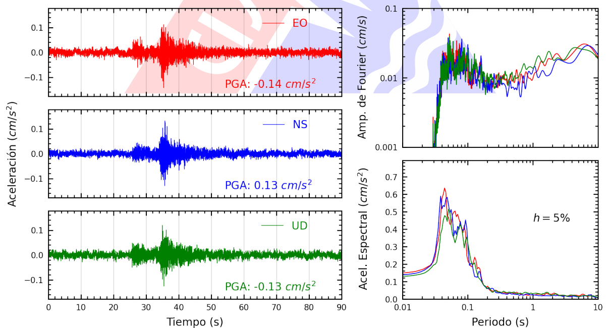
Figura A.26: Registros tiempo-historia, espectros de Fourier y de respuesta en las direcciones EO, NS y vertical de la estación UNMSM. Sismo de Chilca, Cañete - Lima del 2024-06-21, 02:25:56 (Hora local)
