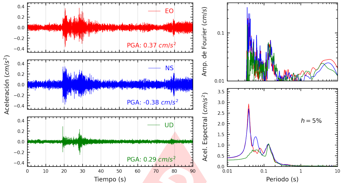
Figura A.15: Registros tiempo-historia, espectros de Fourier y de respuesta en las direcciones EO, NS y vertical de la estación DHNPE. Sismo de Chilca, Cañete - Lima del 2024-06-21, 02:25:56 (Hora local)
