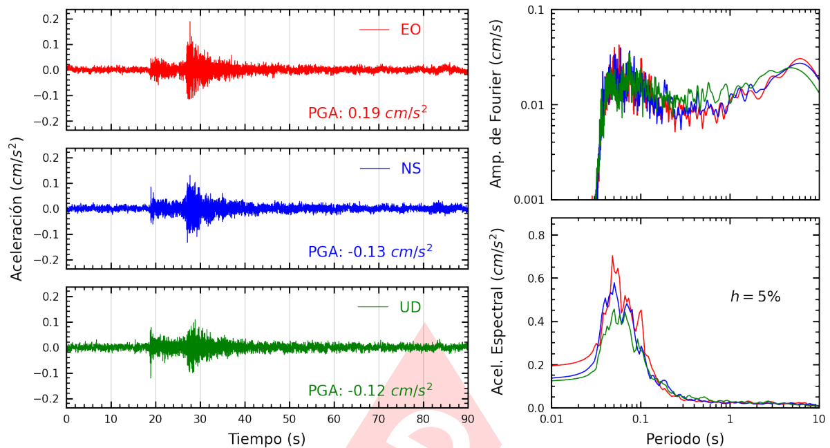
Figura A.23: Registros tiempo-historia, espectros de Fourier y de respuesta en las direcciones EO, NS y vertical de la estación UNFV. Sismo de Chilca, Cañete - Lima del 2024-06-21, 02:25:56 (Hora local)
