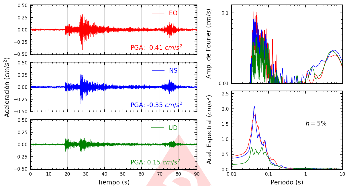
Figura A.13: Registros tiempo-historia, espectros de Fourier y de respuesta en las direcciones EO, NS y vertical de la estación CEPRE. Sismo de Chilca, Cañete - Lima del 2024-06-21, 02:25:56 (Hora local)
