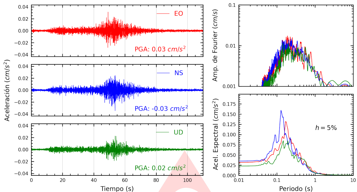
Figura A.1: Registros tiempo-historia, espectros de Fourier y de respuesta en las direcciones EO, NS y vertical de la estación UNSA2. Sismo de Yauca, Caraveli - Arequipa del 2024-08-02, 21:00:52 (Hora local)
