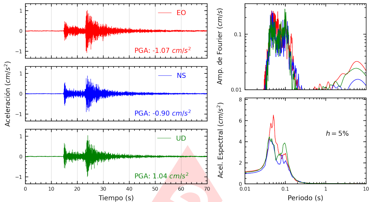
Figura A.13: Registros tiempo-historia, espectros de Fourier y de respuesta en las direcciones EO, NS y vertical de la estación AMORE. Sismo de Chilca, Cañete - Lima del 2024-08-04, 13:39:32 (Hora local)
