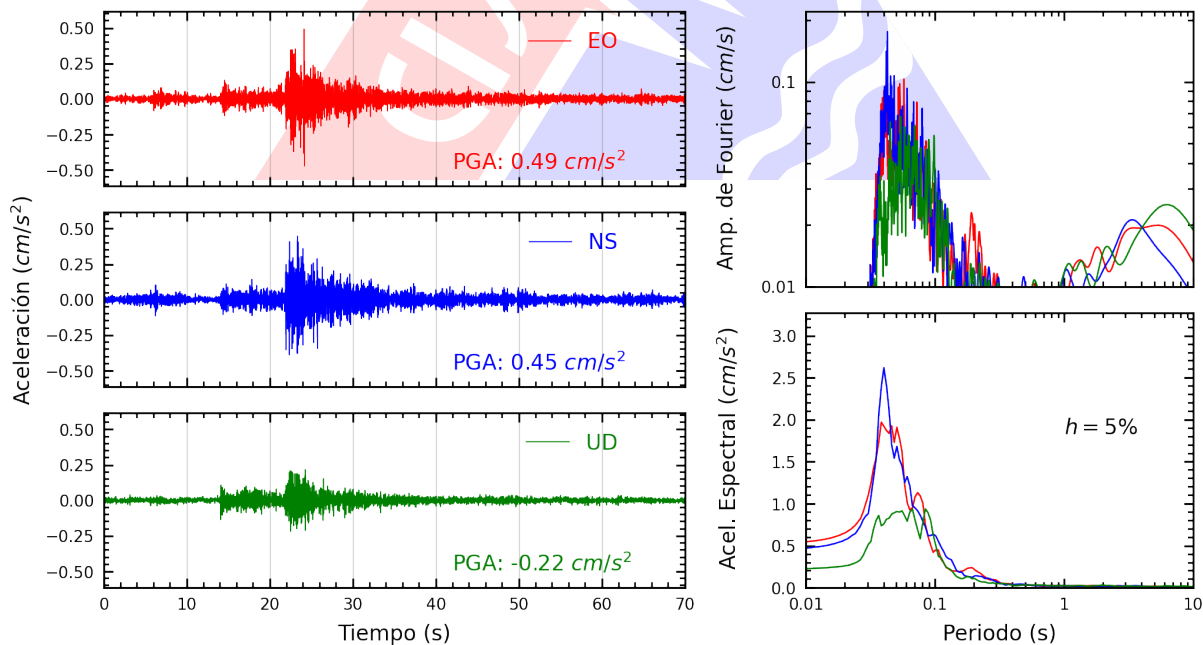
Figura A.26: Registros tiempo-historia, espectros de Fourier y de respuesta en las direcciones EO, NS y vertical de la estación COMAS. Sismo de Chilca, Cañete - Lima del 2024-08-04, 13:39:32 (Hora local)
