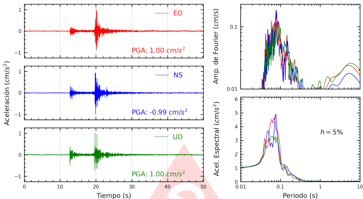
Figura A.15: Registros tiempo-historia, espectros de Fourier y de respuesta en las direcciones EO, NS y vertical de la estación UNMSM. Sismo de Chilca, Cañete - Lima del 2024-08-04, 13:39:32 (Hora local)
