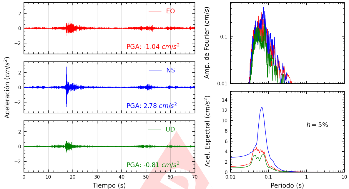
Figura A.3: Registros tiempo-historia, espectros de Fourier y de respuesta en las direcciones EO, NS y vertical de la estación PACHA. Sismo de Chilca, Cañete - Lima del 2024-08-04, 13:39:32 (Hora local)
