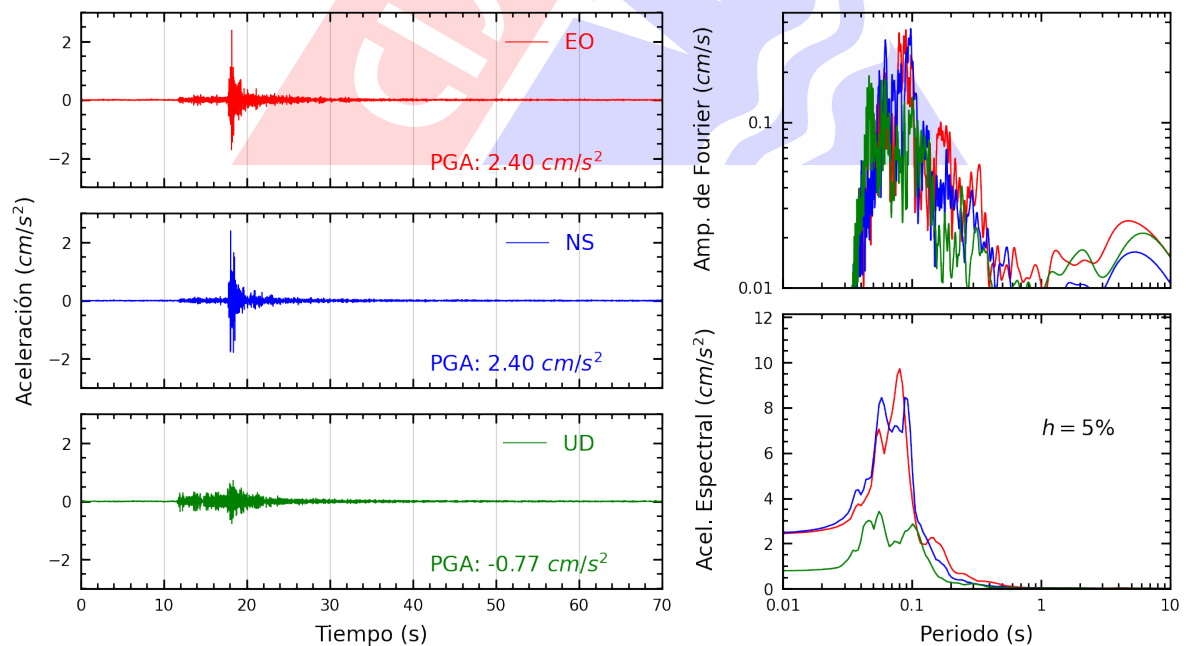
Figura A.4: Registros tiempo-historia, espectros de Fourier y de respuesta en las direcciones EO, NS y vertical de la estación USILP. Sismo de Chilca, Cañete - Lima del 2024-08-04, 13:39:32 (Hora local)
