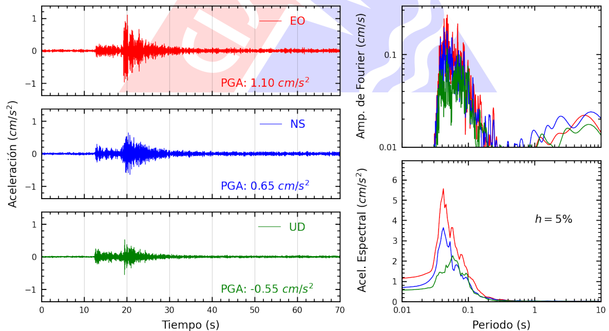
Figura A.12: Registros tiempo-historia, espectros de Fourier y de respuesta en las direcciones EO, NS y vertical de la estación CEPRE. Sismo de Chilca, Cañete - Lima del 2024-08-04, 13:39:32 (Hora local)
