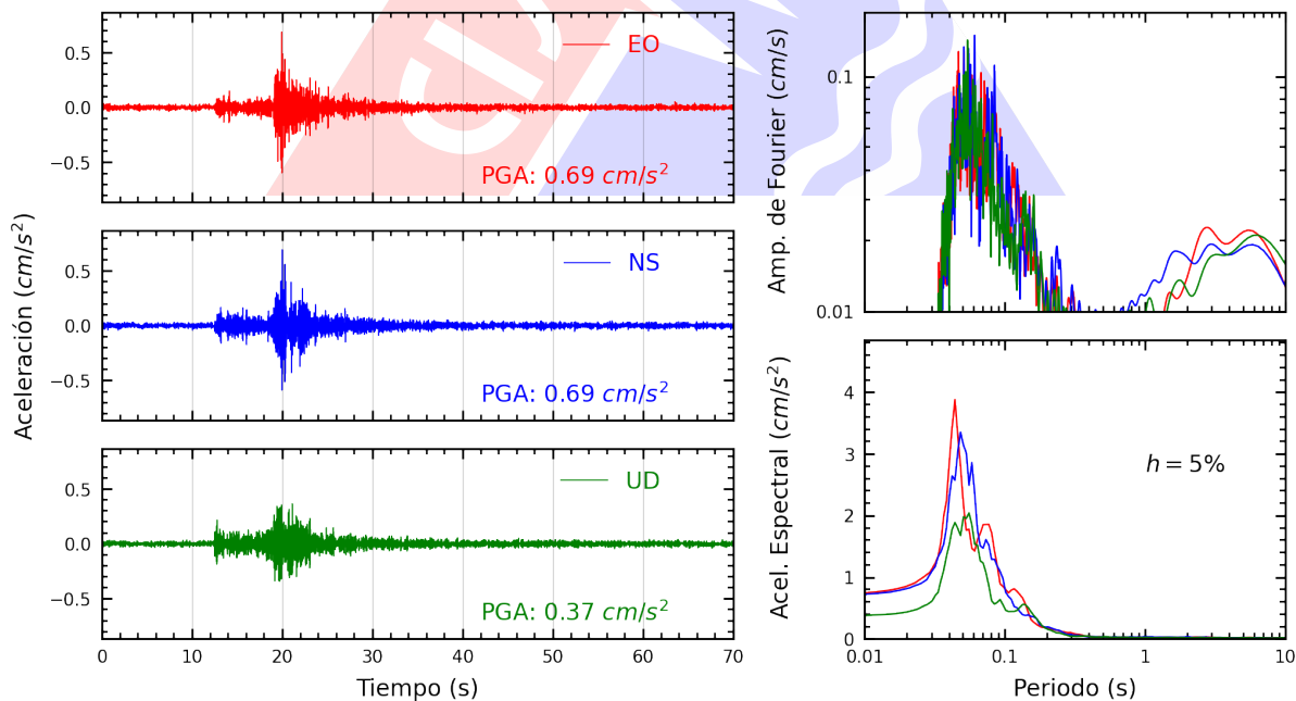
Figura A.22: Registros tiempo-historia, espectros de Fourier y de respuesta en las direcciones EO, NS y vertical de la estación CENEP. Sismo de Chilca, Cañete - Lima del 2024-08-04, 13:39:32 (Hora local)
