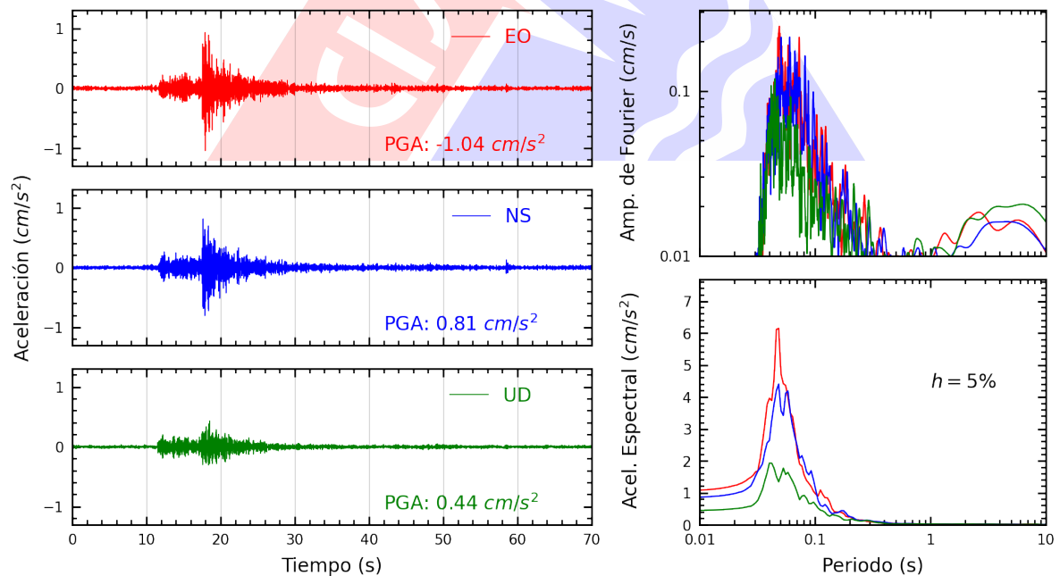
Figura A.14: Registros tiempo-historia, espectros de Fourier y de respuesta en las direcciones EO, NS y vertical de la estación UPCVI. Sismo de Chilca, Cañete - Lima del 2024-08-04, 13:39:32 (Hora local)
