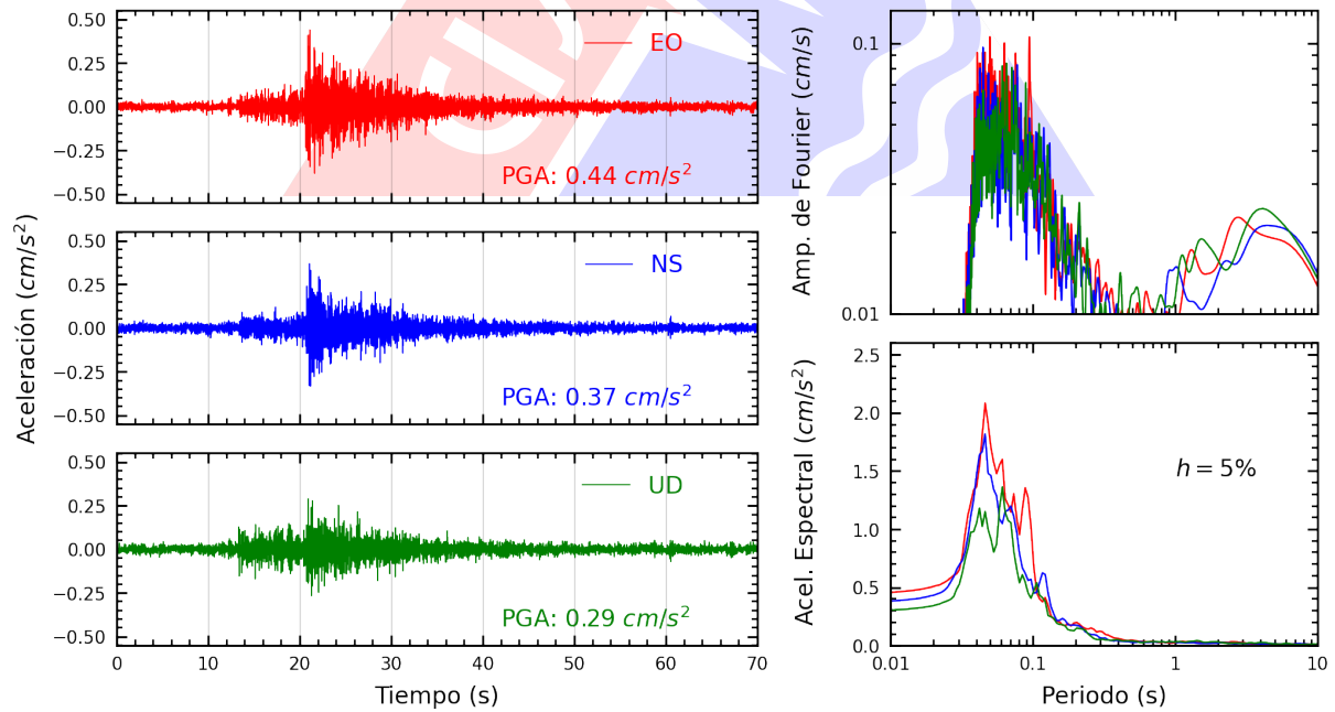
Figura A.28: Registros tiempo-historia, espectros de Fourier y de respuesta en las direcciones EO, NS y vertical de la estación UCVAT. Sismo de Chilca, Cañete - Lima del 2024-08-04, 13:39:32 (Hora local)
