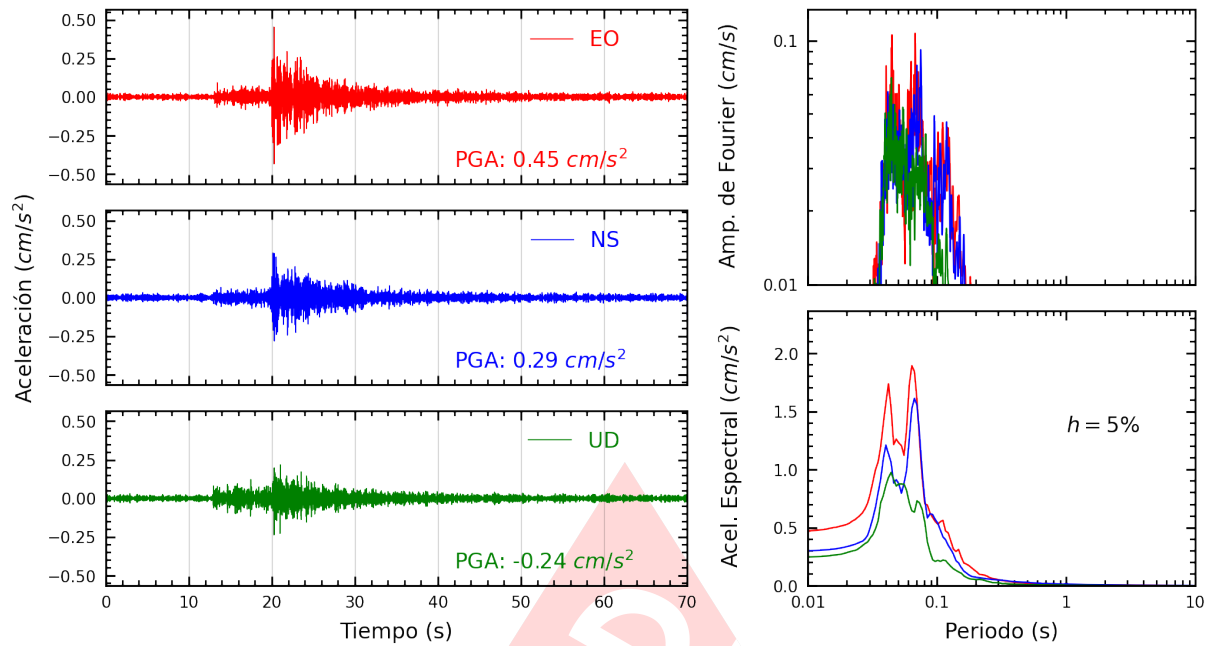
Figura A.27: Registros tiempo-historia, espectros de Fourier y de respuesta en las direcciones EO, NS y vertical de la estación ATARJ. Sismo de Chilca, Cañete - Lima del 2024-08-04, 13:39:32 (Hora local)
