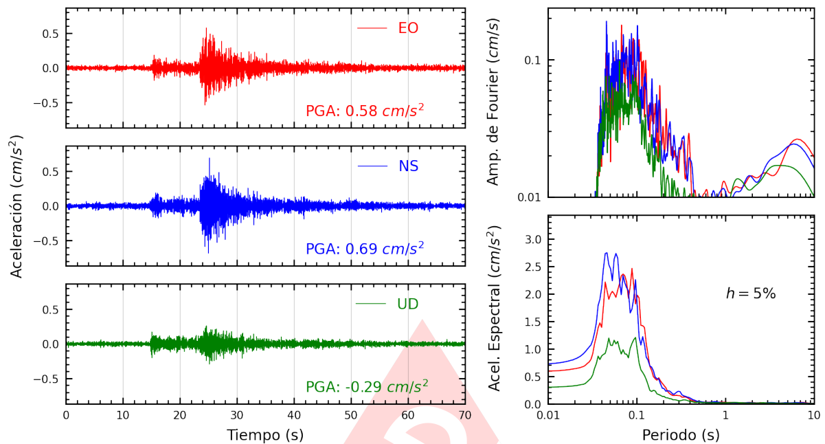
Figura A.23: Registros tiempo-historia, espectros de Fourier y de respuesta en las direcciones EO, NS y vertical de la estación DEFEN. Sismo de Chilca, Cañete - Lima del 2024-08-04, 13:39:32 (Hora local)
