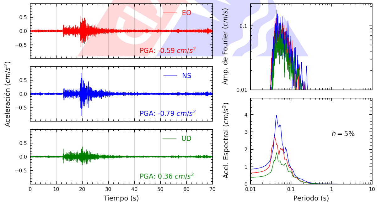
Figura A.18: Registros tiempo-historia, espectros de Fourier y de respuesta en las direcciones EO, NS y vertical de la estación BORJA. Sismo de Chilca, Cañete - Lima del 2024-08-04, 13:39:32 (Hora local)
