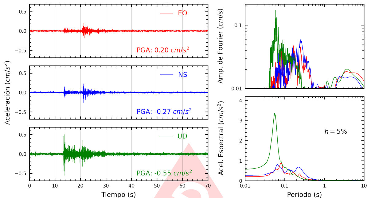
Figura A.25: Registros tiempo-historia, espectros de Fourier y de respuesta en las direcciones EO, NS y vertical de la estación ACAPU. Sismo de Chilca, Cañete - Lima del 2024-08-04, 13:39:32 (Hora local)
