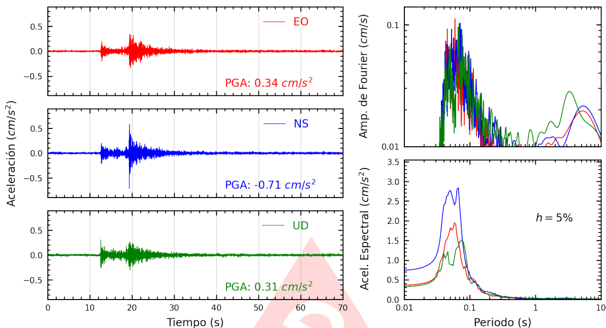
Figura A.21: Registros tiempo-historia, espectros de Fourier y de respuesta en las direcciones EO, NS y vertical de la estación UNFV. Sismo de Chilca, Cañete - Lima del 2024-08-04, 13:39:32 (Hora local)
