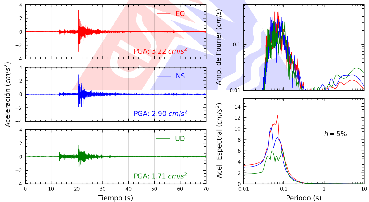
Figura A.2: Registros tiempo-historia, espectros de Fourier y de respuesta en las direcciones EO, NS y vertical de la estación INDEP. Sismo de Chilca, Cañete - Lima del 2024-08-04, 13:39:32 (Hora local)
