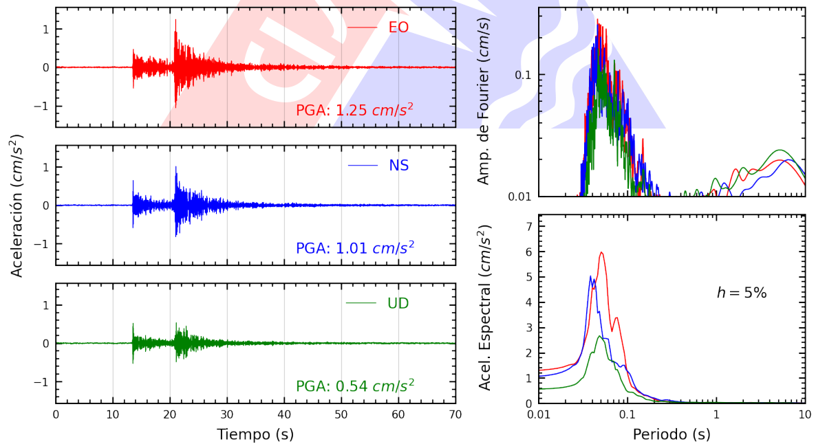
Figura A.10: Registros tiempo-historia, espectros de Fourier y de respuesta en las direcciones EO, NS y vertical de la estación UCSS. Sismo de Chilca, Cañete - Lima del 2024-08-04, 13:39:32 (Hora local)
