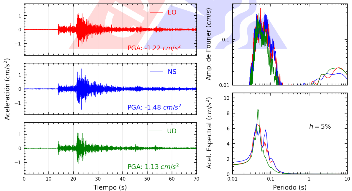
Figura A.8: Registros tiempo-historia, espectros de Fourier y de respuesta en las direcciones EO, NS y vertical de la estación JOSEO. Sismo de Chilca, Cañete - Lima del 2024-08-04, 13:39:32 (Hora local)
