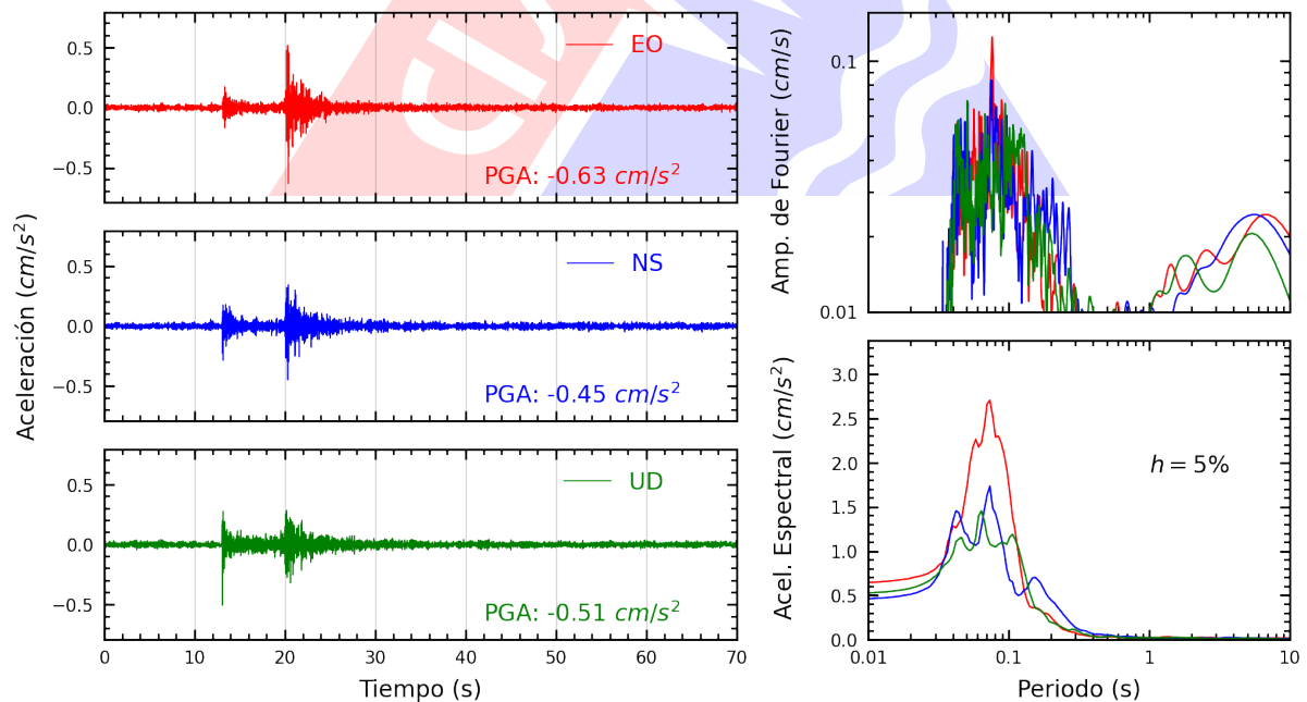
Figura A.24: Registros tiempo-historia, espectros de Fourier y de respuesta en las direcciones EO, NS y vertical de la estación BONDY. Sismo de Chilca, Cañete - Lima del 2024-08-04, 13:39:32 (Hora local)
