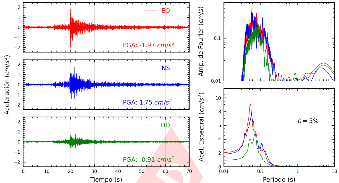
Figura A.5: Registros tiempo-historia, espectros de Fourier y de respuesta en las direcciones EO, NS y vertical de la estación USILM. Sismo de Chilca, Cañete - Lima del 2024-08-04, 13:39:32 (Hora local)
