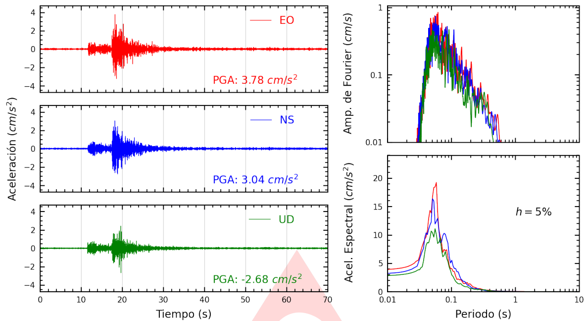
Figura A.1: Registros tiempo-historia, espectros de Fourier y de respuesta en las direcciones EO, NS y vertical de la estación UNTEL. Sismo de Chilca, Cañete - Lima del 2024-08-04, 13:39:32 (Hora local)
