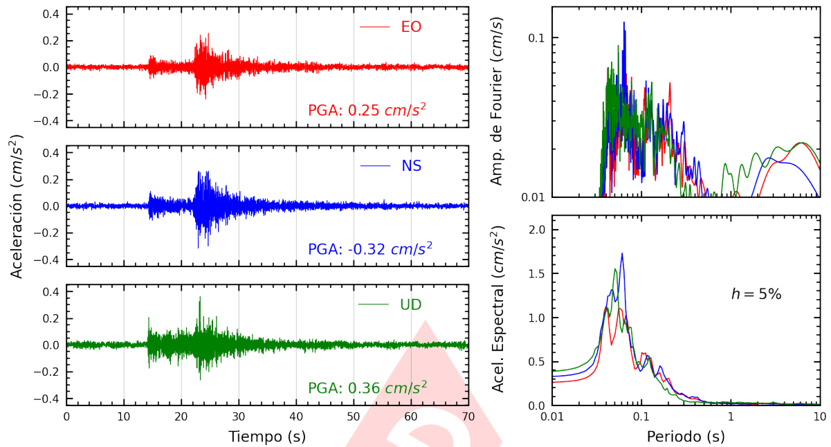
Figura A.29: Registros tiempo-historia, espectros de Fourier y de respuesta en las direcciones EO, NS y vertical de la estación VHAYA. Sismo de Chilca, Cañete - Lima del 2024-08-04, 13:39:32 (Hora local)
