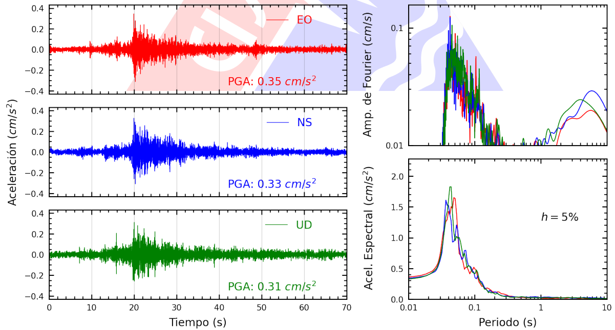
Figura A.30: Registros tiempo-historia, espectros de Fourier y de respuesta en las direcciones EO, NS y vertical de la estación USMP. Sismo de Chilca, Cañete - Lima del 2024-08-04, 13:39:32 (Hora local)
