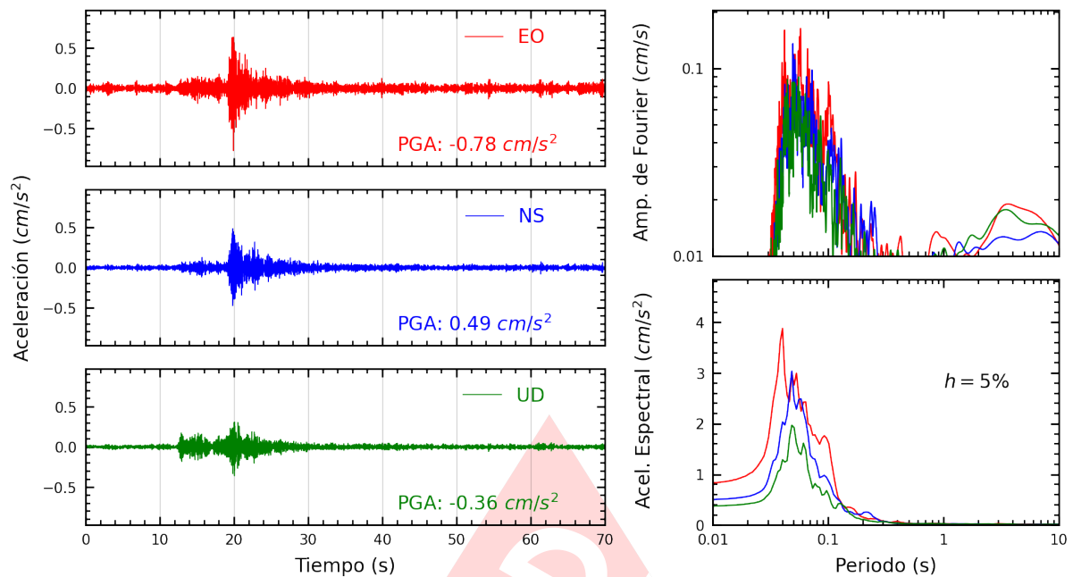
Figura A.19: Registros tiempo-historia, espectros de Fourier y de respuesta en las direcciones EO, NS y vertical de la estación INICT. Sismo de Chilca, Cañete - Lima del 2024-08-04, 13:39:32 (Hora local)
