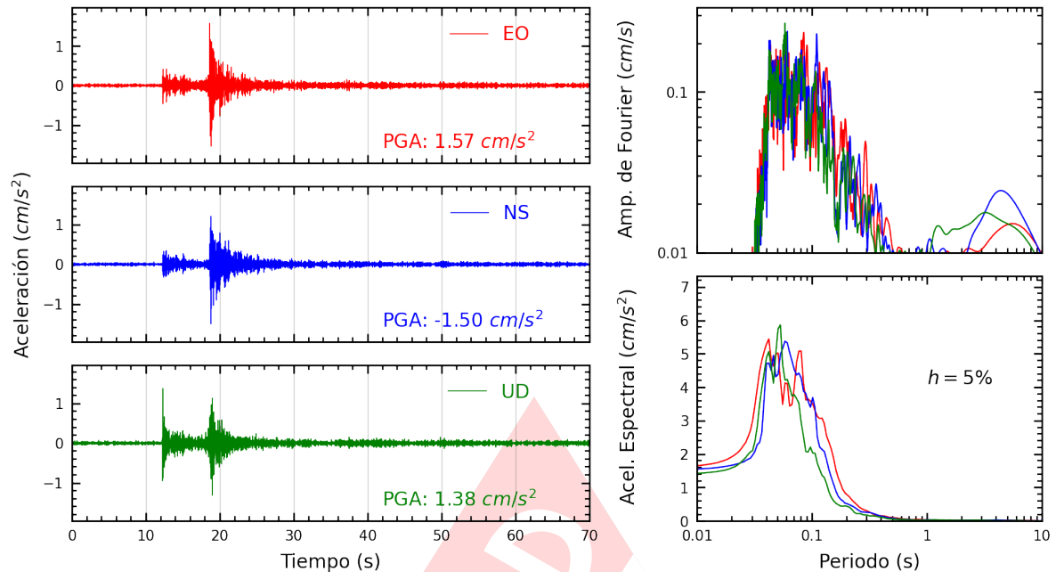
Figura A.7: Registros tiempo-historia, espectros de Fourier y de respuesta en las direcciones EO, NS y vertical de la estación URPE. Sismo de Chilca, Cañete - Lima del 2024-08-04, 13:39:32 (Hora local)
