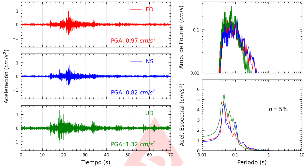
Figura A.9: Registros tiempo-historia, espectros de Fourier y de respuesta en las direcciones EO, NS y vertical de la estación SCOLI. Sismo de Chilca, Cañete - Lima del 2024-08-04, 13:39:32 (Hora local)
