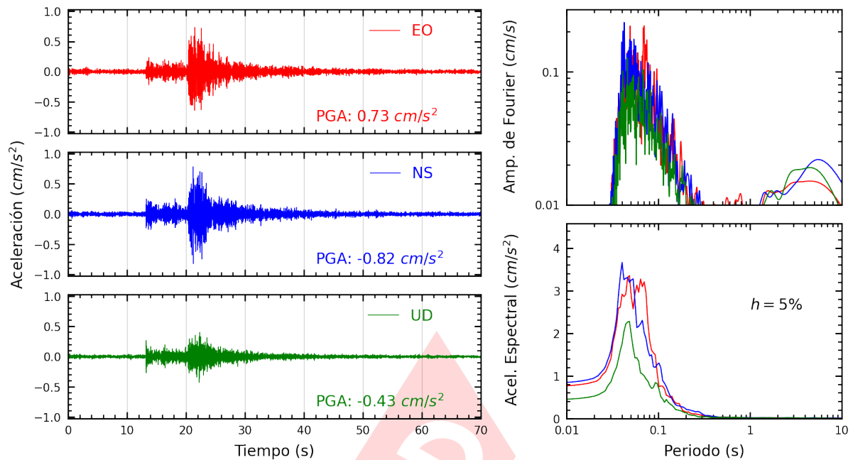
Figura A.17: Registros tiempo-historia, espectros de Fourier y de respuesta en las direcciones EO, NS y vertical de la estación FICPE. Sismo de Chilca, Cañete - Lima del 2024-08-04, 13:39:32 (Hora local)
