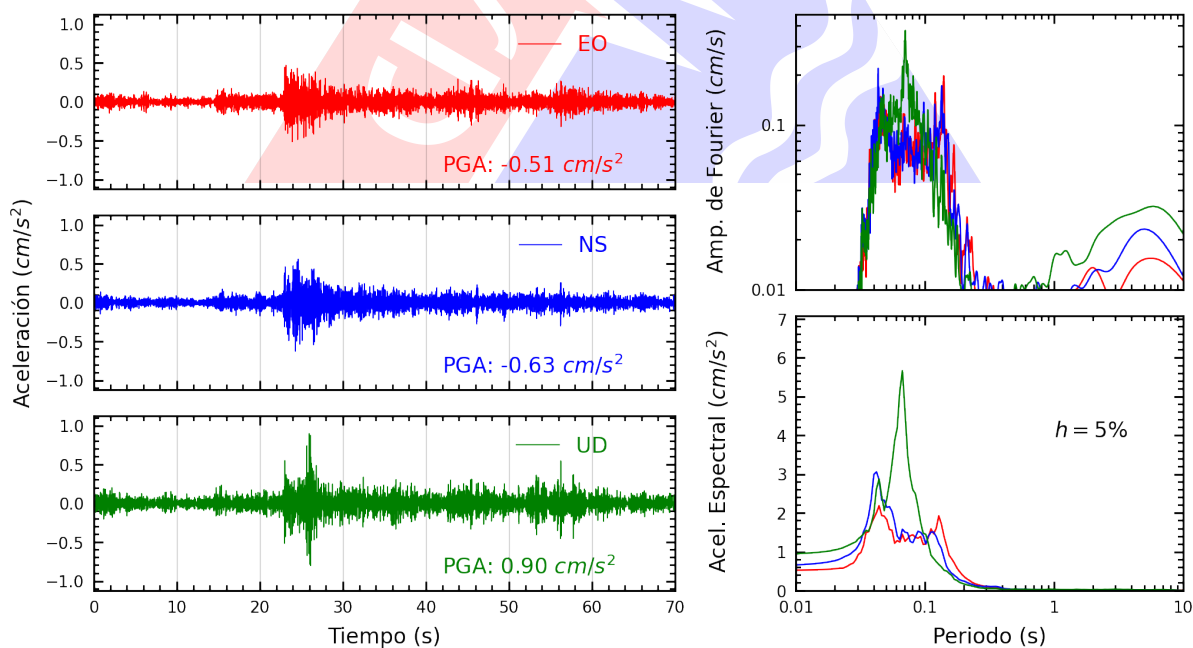
Figura A.16: Registros tiempo-historia, espectros de Fourier y de respuesta en las direcciones EO, NS y vertical de la estación CARAB. Sismo de Chilca, Cañete - Lima del 2024-08-04, 13:39:32 (Hora local)
