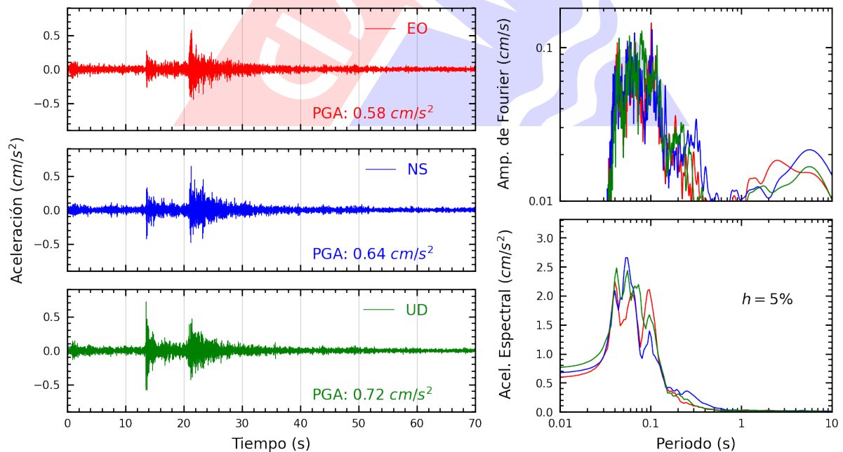
Figura A.20: Registros tiempo-historia, espectros de Fourier y de respuesta en las direcciones EO, NS y vertical de la estación MADRE. Sismo de Chilca, Cañete - Lima del 2024-08-04, 13:39:32 (Hora local)
