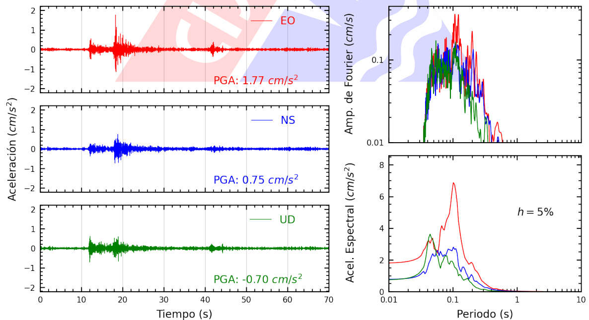
Figura A.6: Registros tiempo-historia, espectros de Fourier y de respuesta en las direcciones EO, NS y vertical de la estación SCCHO. Sismo de Chilca, Cañete - Lima del 2024-08-04, 13:39:32 (Hora local)
