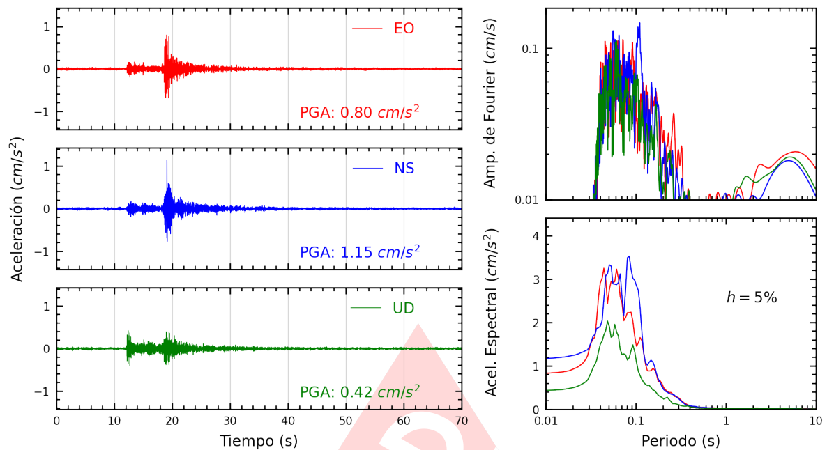
Figura A.11: Registros tiempo-historia, espectros de Fourier y de respuesta en las direcciones EO, NS y vertical de la estación SERVI. Sismo de Chilca, Cañete - Lima del 2024-08-04, 13:39:32 (Hora local)
