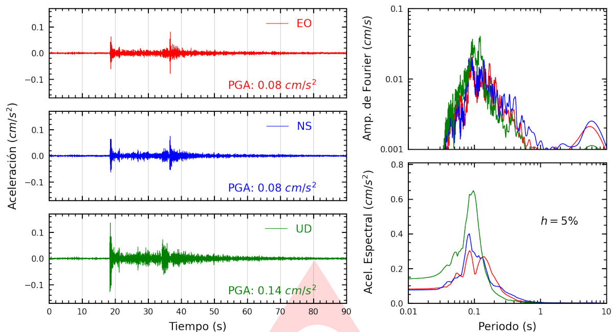
Figura A.1: Registros tiempo-historia, espectros de Fourier y de respuesta en las direcciones EO, NS y vertical de la estación UNIA. Sismo de Puerto Inca, Puerto Inca - Huanuco del 2024-08-05, 00:00:34 (Hora local)
