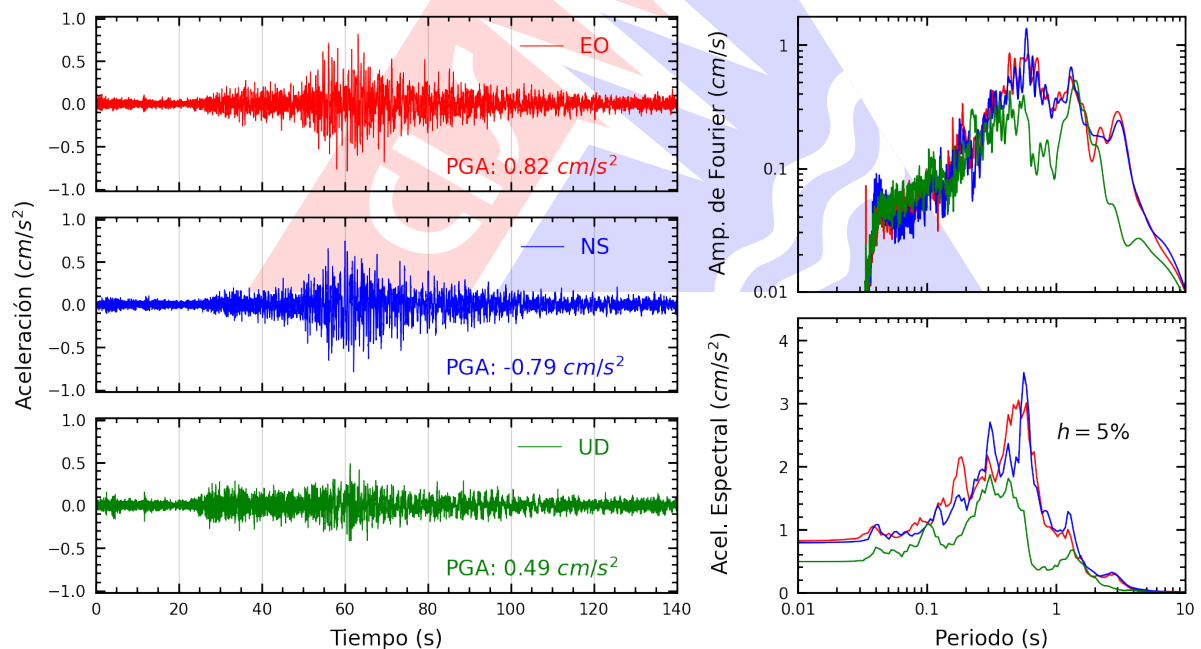
Figura A.2: Registros tiempo-historia, espectros de Fourier y de respuesta en las direcciones EO, NS y vertical de la estación SCICA. Sismo de Lomas, Caraveli - Arequipa del 2024-08-13, 21:55:25 (Hora local)
