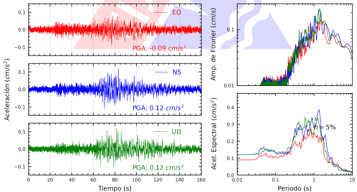
Figura A.4: Registros tiempo-historia, espectros de Fourier y de respuesta en las direcciones EO, NS y vertical de la estación UNSCH. Sismo de Lomas, Caraveli - Arequipa del 2024-08-13, 21:55:25 (Hora local)
