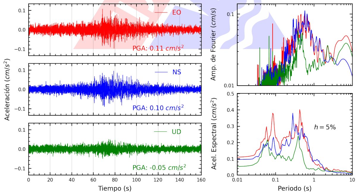
Figura A.6: Registros tiempo-historia, espectros de Fourier y de respuesta en las direcciones EO, NS y vertical de la estación USILP. Sismo de Lomas, Caraveli - Arequipa del 2024-08-13, 21:55:25 (Hora local)
