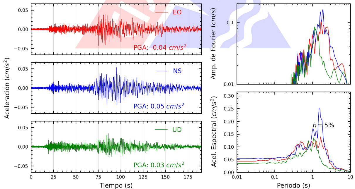
Figura A.8: Registros tiempo-historia, espectros de Fourier y de respuesta en las direcciones EO, NS y vertical de la estación UNCP. Sismo de Lomas, Caraveli - Arequipa del 2024-08-13, 21:55:25 (Hora local)
