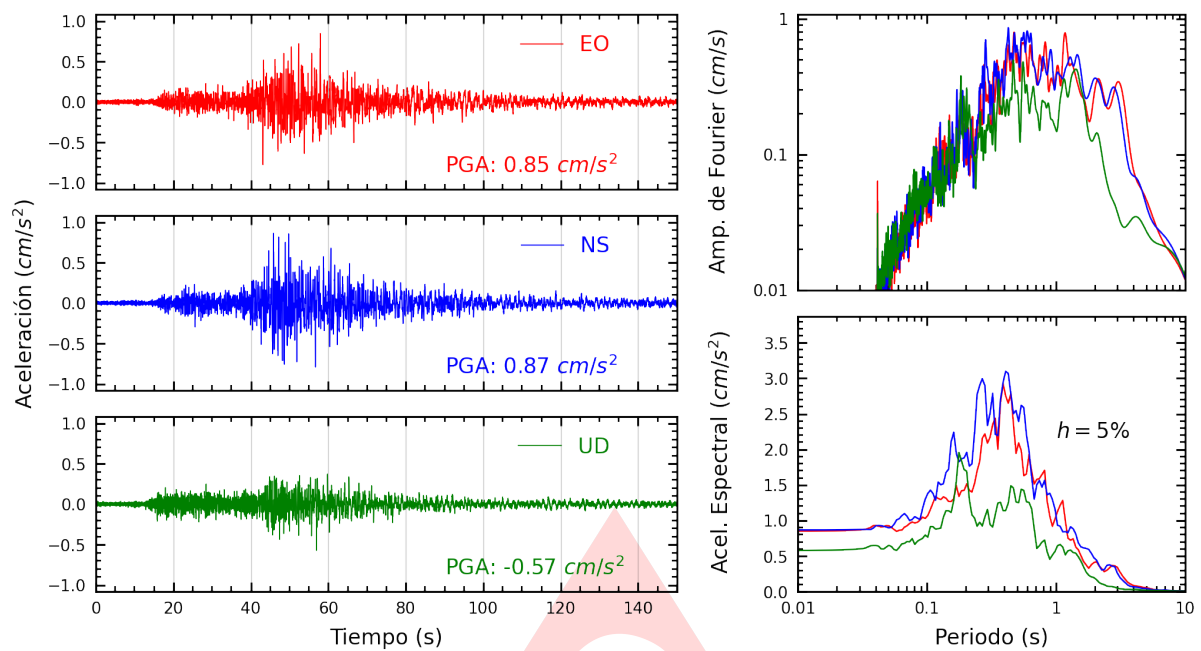
Figura A.1: Registros tiempo-historia, espectros de Fourier y de respuesta en las direcciones EO, NS y vertical de la estación UNICA. Sismo de Lomas, Caraveli - Arequipa del 2024-08-13, 21:55:25 (Hora local)
