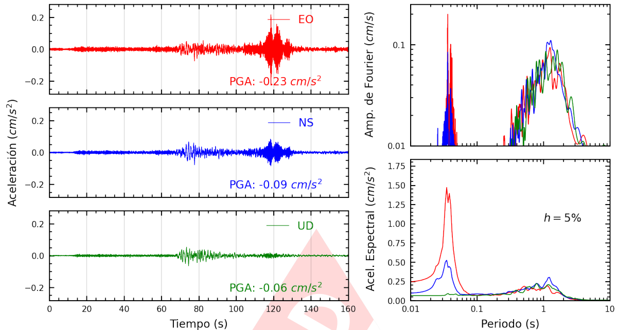
Figura A.3: Registros tiempo-historia, espectros de Fourier y de respuesta en las direcciones EO, NS y vertical de la estación UNAM. Sismo de Lomas, Caraveli - Arequipa del 2024-08-13, 21:55:25 (Hora local)
