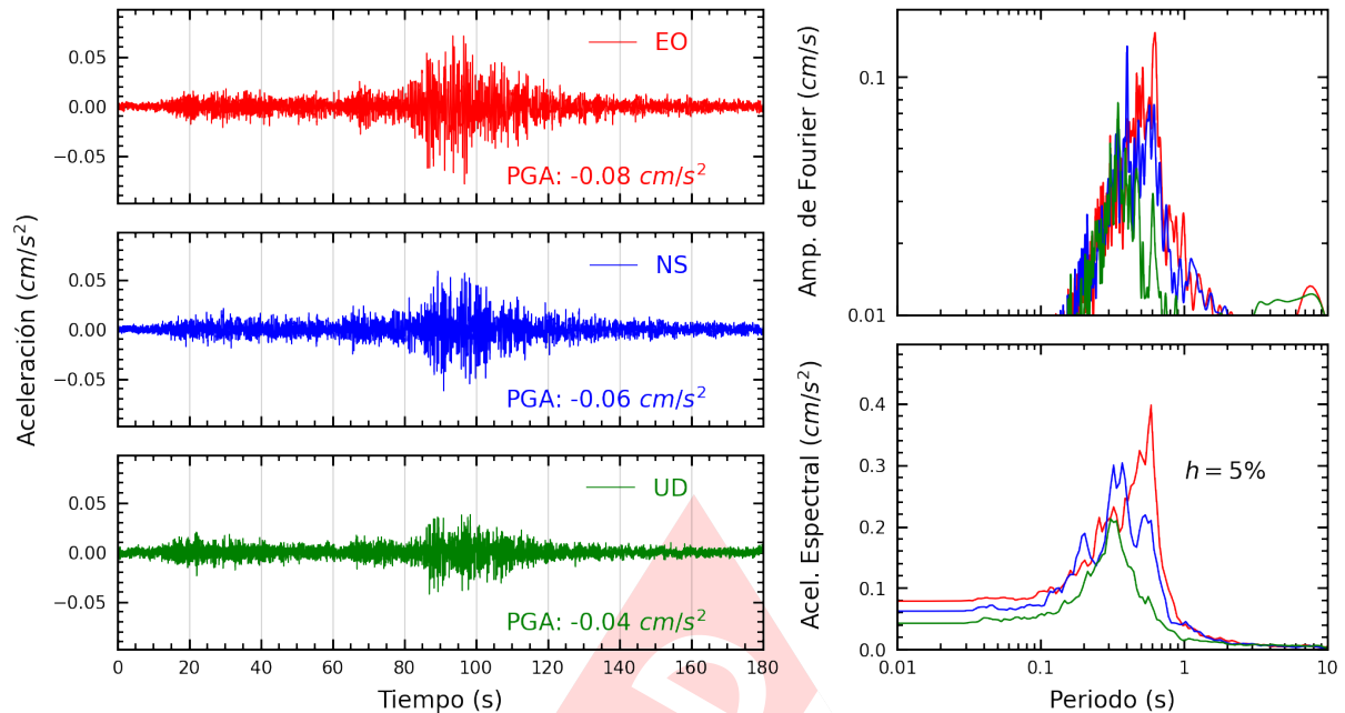
Figura A.7: Registros tiempo-historia, espectros de Fourier y de respuesta en las direcciones EO, NS y vertical de la estación CARAL. Sismo de Lomas, Caraveli - Arequipa del 2024-08-13, 21:55:25 (Hora local)
