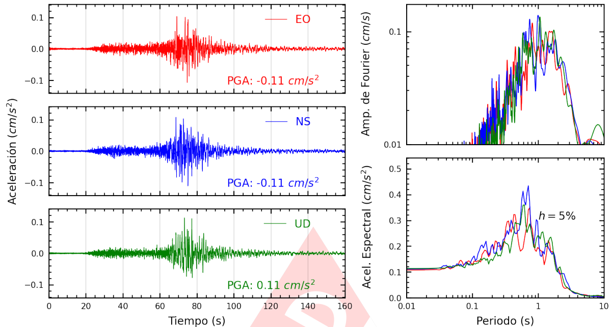
Figura A.5: Registros tiempo-historia, espectros de Fourier y de respuesta en las direcciones EO, NS y vertical de la estación UNSA2. Sismo de Lomas, Caraveli - Arequipa del 2024-08-13, 21:55:25 (Hora local)
