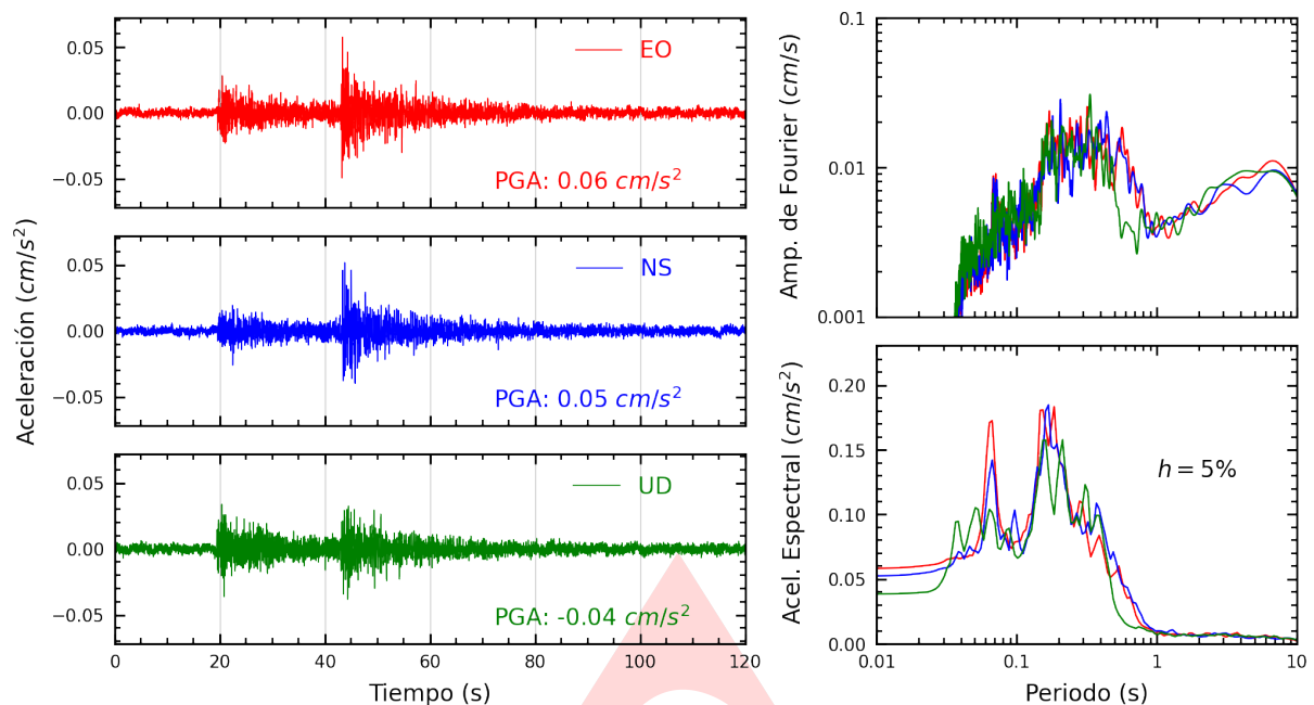
Figura A.1: Registros tiempo-historia, espectros de Fourier y de respuesta en las direcciones EO, NS y vertical de la estación CARAL. Sismo de Huancabamba, Oxapampa - Pasco del 2024-08-13, 23:41:35 (Hora local)
