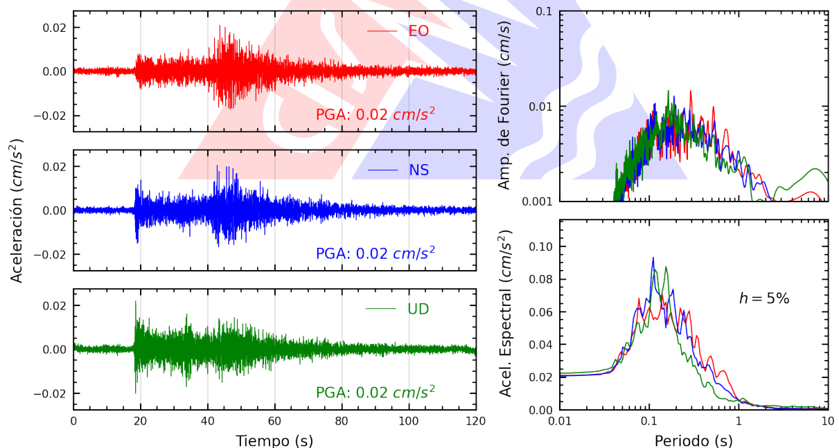
Figura A.2: Registros tiempo-historia, espectros de Fourier y de respuesta en las direcciones EO, NS y vertical de la estación UNCP. Sismo de Huancabamba, Oxapampa - Pasco del 2024-08-13, 23:41:35 (Hora local)
