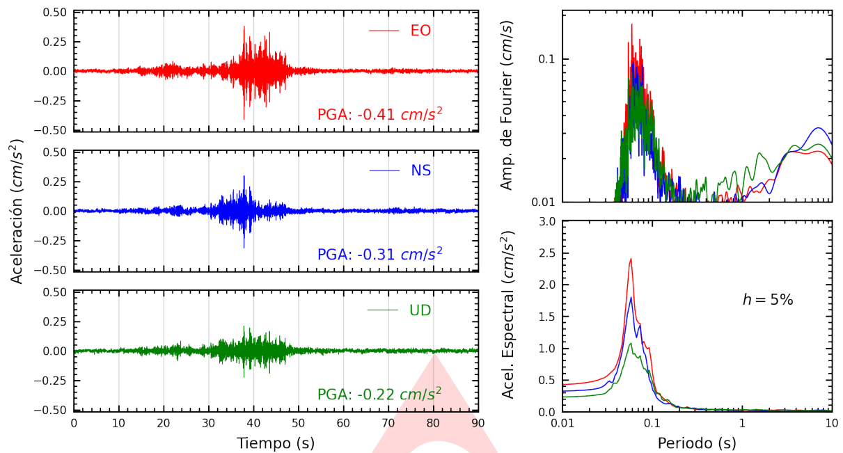
Figura A.1: Registros tiempo-historia, espectros de Fourier y de respuesta en las direcciones EO, NS y vertical de la estación UNTRM. Sismo de Puerto Inca, Puerto Inca - Huanuco del 2024-08-16, 22:09:39 (Hora local)
