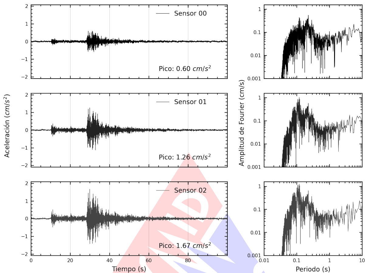
Figura A.2: Registros tiempo-historia y espectros de Fourier en la dirección NS de la edificación Vivienda. Sismo de Chinchipe Alta, Chinchipe - Ica del 2024-08-21, 23:22:14 (Hora local)
