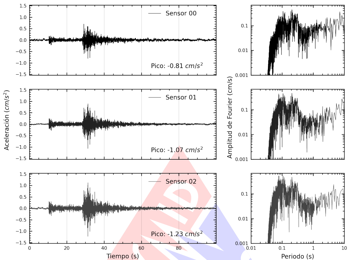
Figura A.1: Registros tiempo-historia y espectros de Fourier en la dirección EW de la edificación Vivienda. Sismo de Chinchipe Alta, Chinchipe - Ica del 2024-08-21, 23:22:14 (Hora local)
