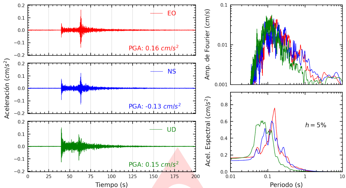
Figura A.1: Registros tiempo-historia, espectros de Fourier y de respuesta en las direcciones EO, NS y vertical de la estación UNIA. Sismo de Puerto Inca, Puerto Inca - Huanuco del 2024-09-03, 04:18:49 (Hora local)
