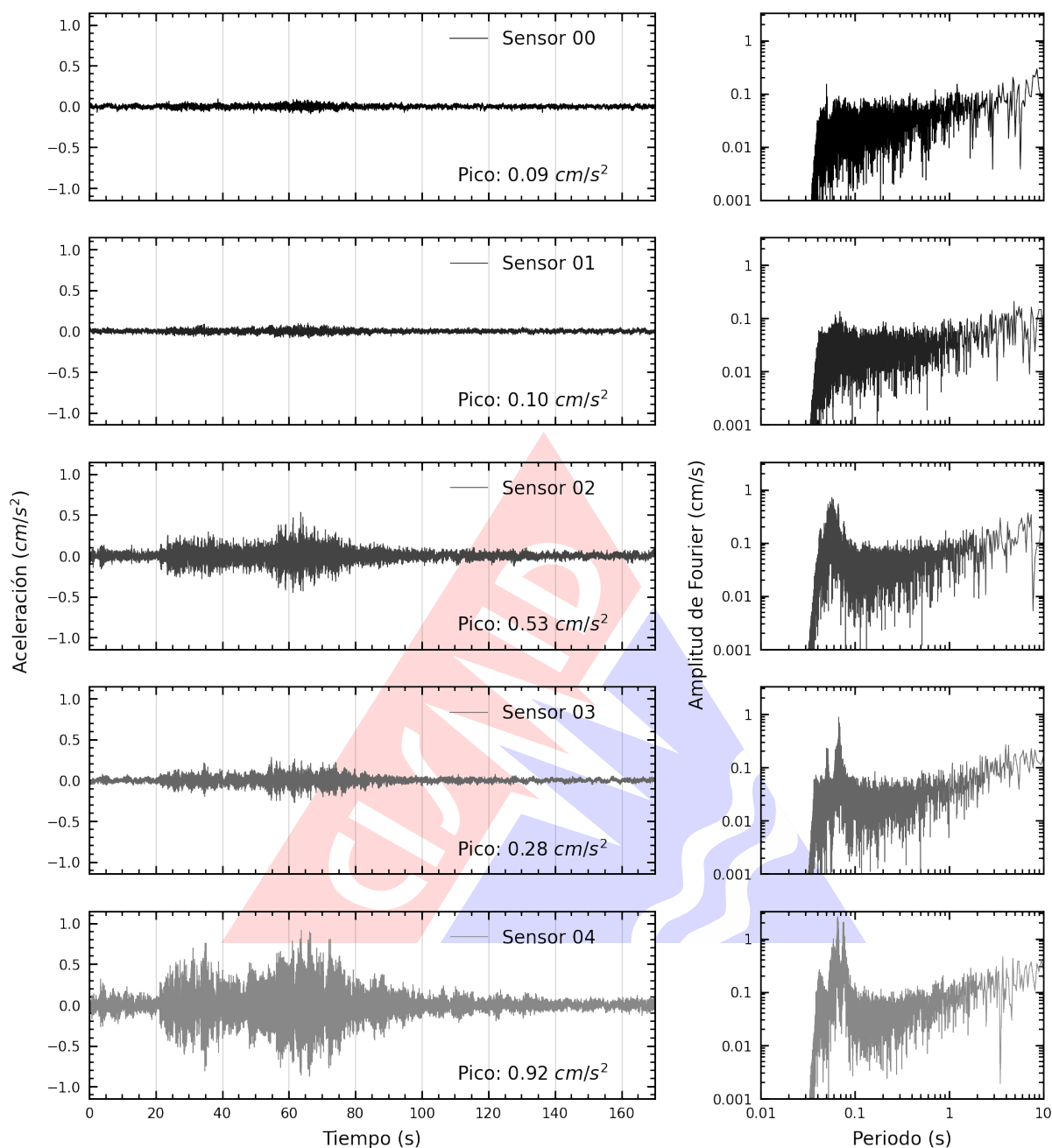
Figura A.3: Registros tiempo-historia y espectros de Fourier en la dirección vertical de la edificación Centro de Observación para la Ingeniería Sísmica del CISMID-FIC-UNI. Sismo de Ica, Ica - Ica del 2024-09-03, 05:08:35 (Hora local)
