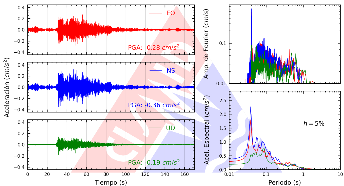
Figura A.5: Registros tiempo-historia, espectros de Fourier y de respuesta en las direcciones EO, NS y vertical de la estación UNAM. Sismo de Tacna, Tacna - Tacna del 2024-09-03, 20:37:17 (Hora local)
