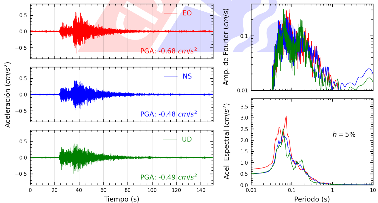
Figura A.4: Registros tiempo-historia, espectros de Fourier y de respuesta en las direcciones EO, NS y vertical de la estación CREY. Sismo de Tacna, Tacna - Tacna del 2024-09-03, 20:37:17 (Hora local)
