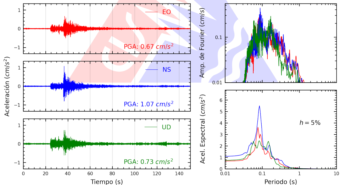
Figura A.2: Registros tiempo-historia, espectros de Fourier y de respuesta en las direcciones EO, NS y vertical de la estación UJBG2. Sismo de Tacna, Tacna - Tacna del 2024-09-03, 20:37:17 (Hora local)
