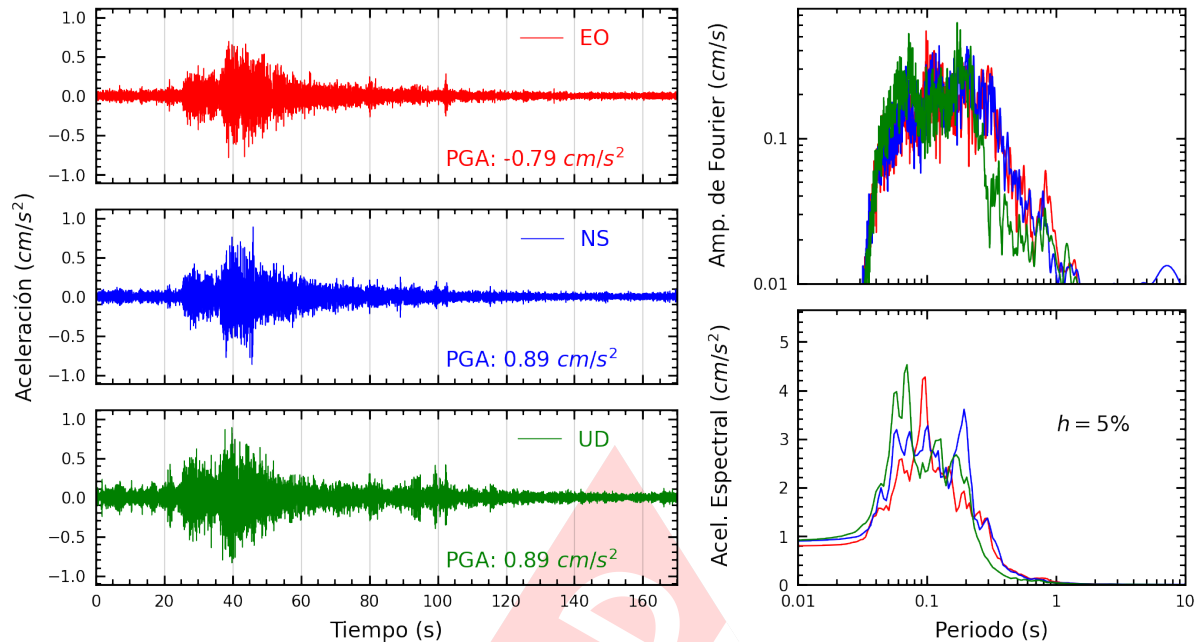
Figura A.3: Registros tiempo-historia, espectros de Fourier y de respuesta en las direcciones EO, NS y vertical de la estación SCTAC. Sismo de Tacna, Tacna - Tacna del 2024-09-03, 20:37:17 (Hora local)
