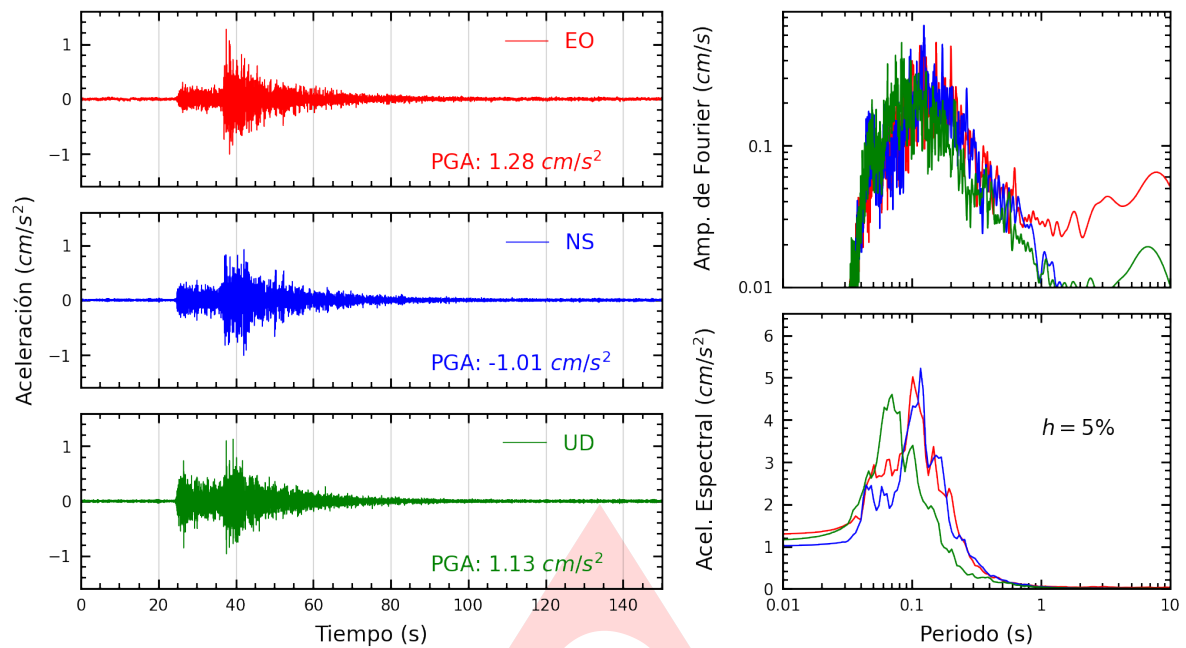
Figura A.1: Registros tiempo-historia, espectros de Fourier y de respuesta en las direcciones EO, NS y vertical de la estación UJBG3. Sismo de Tacna, Tacna - Tacna del 2024-09-03, 20:37:17 (Hora local)
