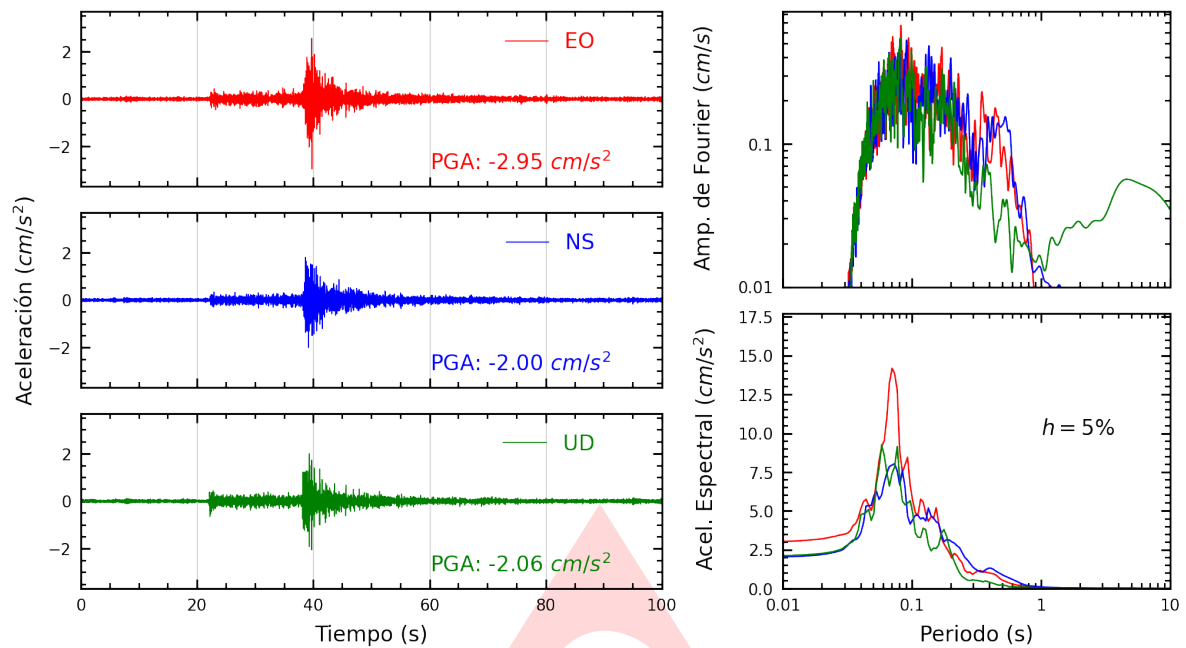
Figura A.1: Registros tiempo-historia, espectros de Fourier y de respuesta en las direcciones EO, NS y vertical de la estación SCARQ. Sismo de Camana, Camana - Arequipa del 2024-09-04, 09:44:19 (Hora local)
