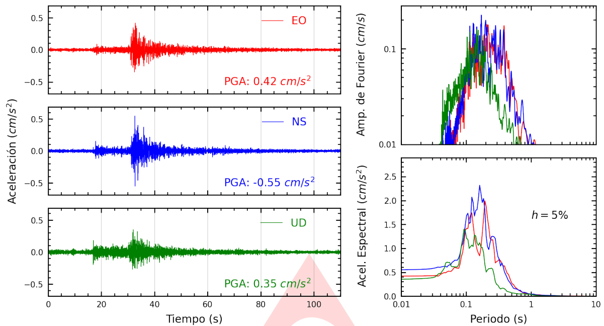
Figura A.1: Registros tiempo-historia, espectros de Fourier y de respuesta en las direcciones EO, NS y vertical de la estación UNP. Sismo de Sullana, Sullana - Piura del 2024-09-05, 09:58:27 (Hora local)
