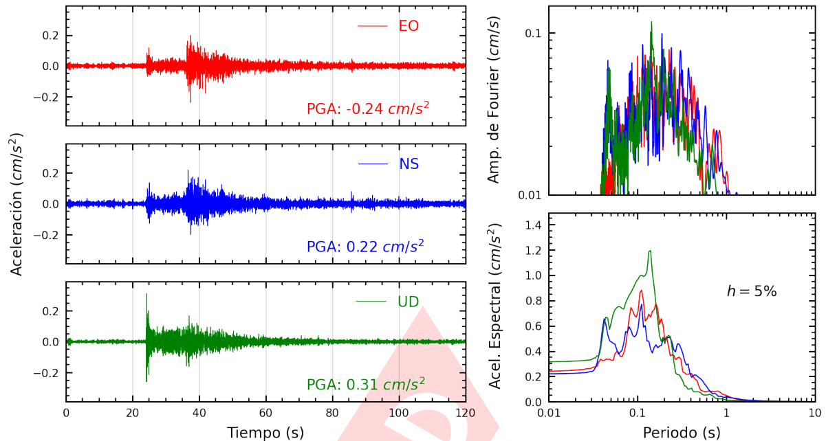
Figura A.3: Registros tiempo-historia, espectros de Fourier y de respuesta en las direcciones EO, NS y vertical de la estación UNF. Sismo de Sullana, Sullana - Piura del 2024-09-05, 09:58:27 (Hora local)
