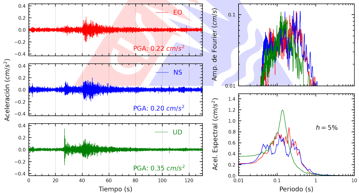
Figura A.2: Registros tiempo-historia, espectros de Fourier y de respuesta en las direcciones EO, NS y vertical de la estación UPAOP. Sismo de Sullana, Sullana - Piura del 2024-09-05, 09:58:27 (Hora local)
