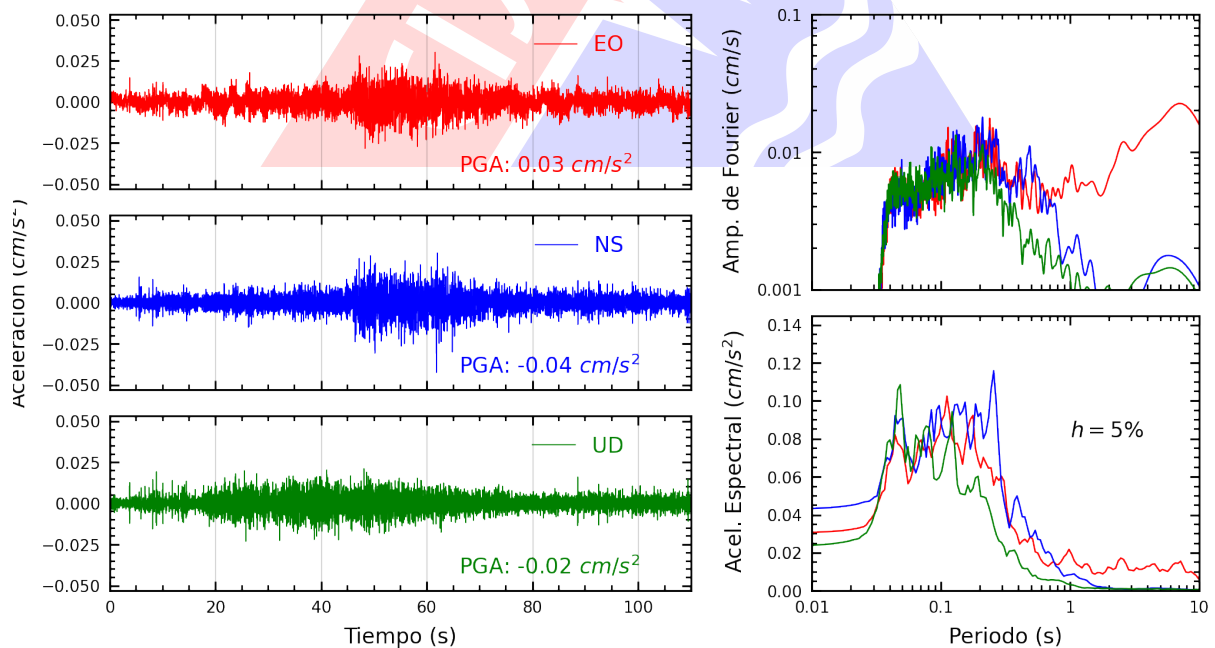
Figura A.4: Registros tiempo-historia, espectros de Fourier y de respuesta en las direcciones EO, NS y vertical de la estación SCCHI. Sismo de Sullana, Sullana - Piura del 2024-09-05, 09:58:27 (Hora local)
