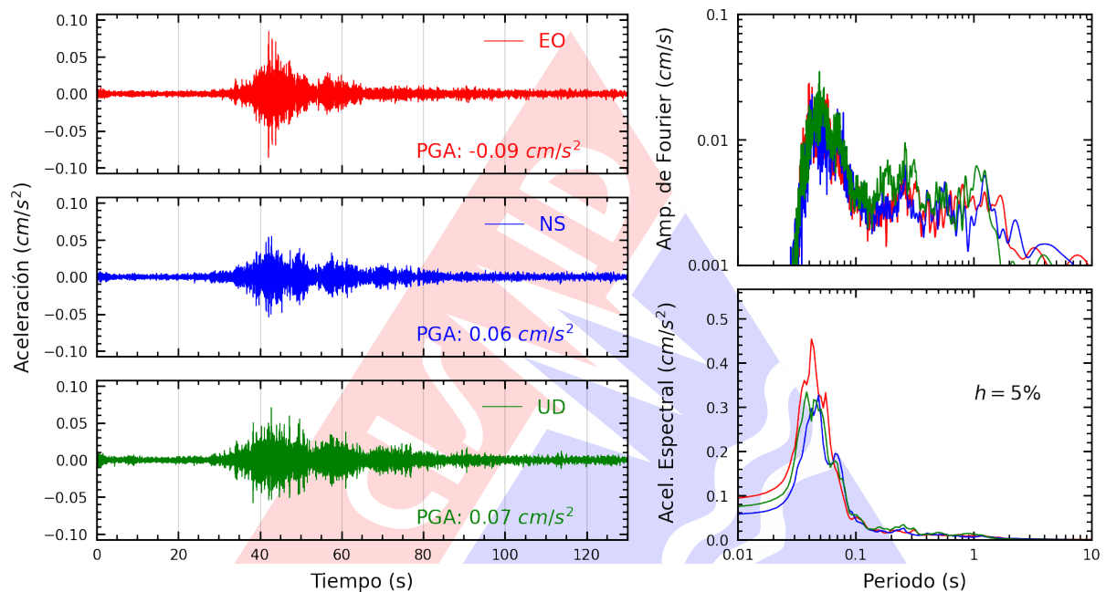
Figura A.7: Registros tiempo-historia, espectros de Fourier y de respuesta en las direcciones EO, NS y vertical de la estación UNCP. Sismo de Santiago De Chuco, Santiago De Chuco - La Libertad del 2024-09-12, 18:27:13 (Hora local)
