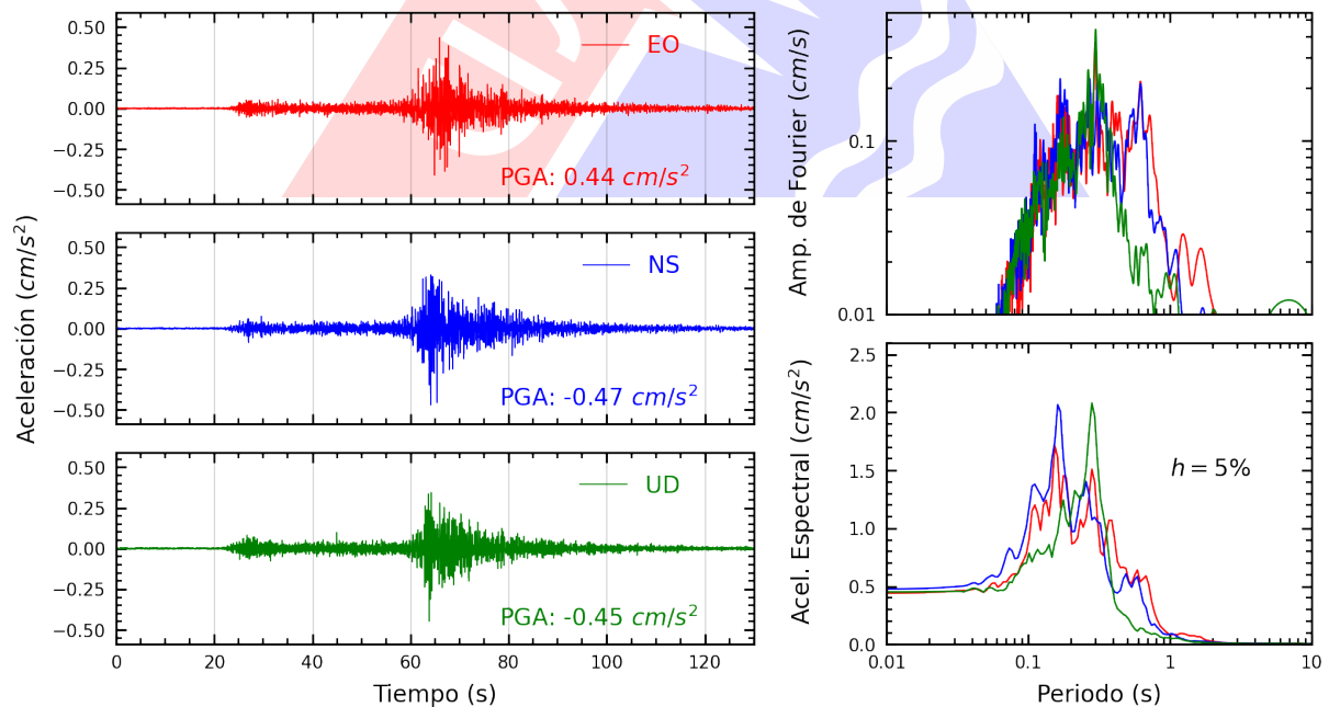
Figura A.4: Registros tiempo-historia, espectros de Fourier y de respuesta en las direcciones EO, NS y vertical de la estación CARAL. Sismo de Santiago De Chuco, Santiago De Chuco - La Libertad del 2024-09-12, 18:27:13 (Hora local)
