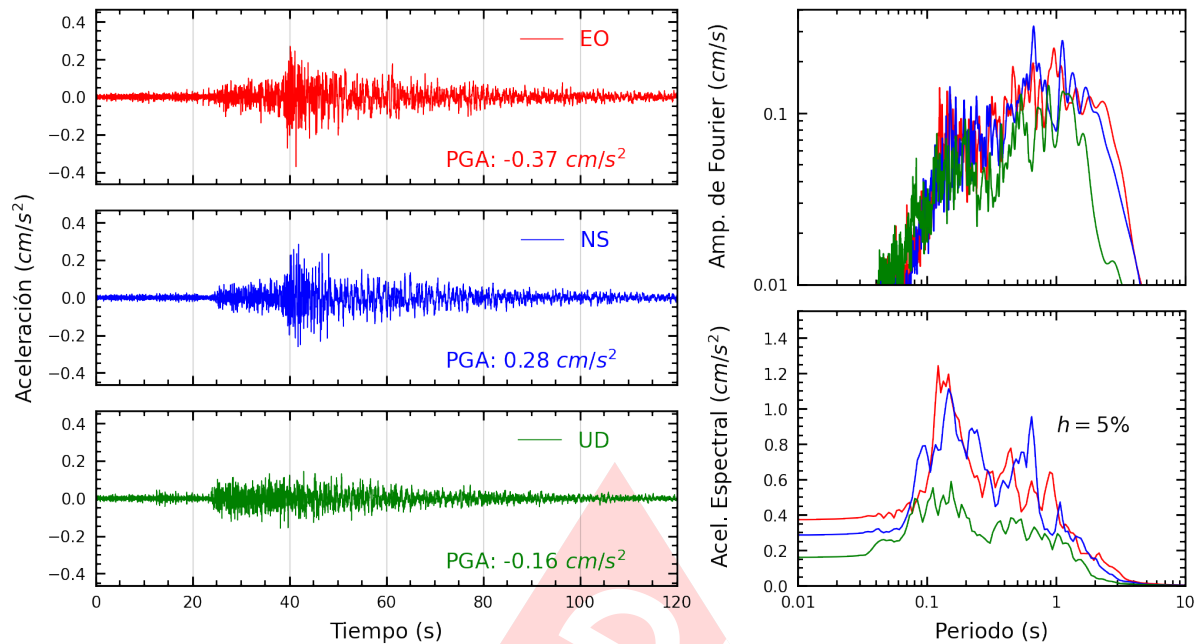
Figura A.5: Registros tiempo-historia, espectros de Fourier y de respuesta en las direcciones EO, NS y vertical de la estación UNC. Sismo de Santiago De Chuco, Santiago De Chuco - La Libertad del 2024-09-12, 18:27:13 (Hora local)
