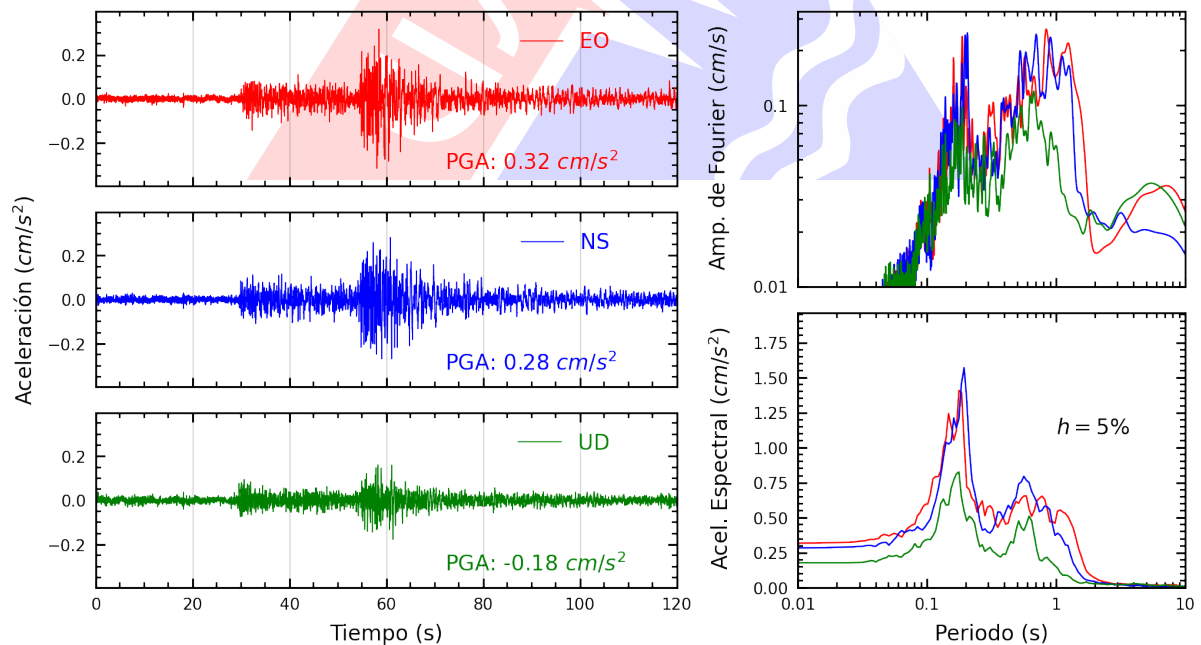
Figura A.6: Registros tiempo-historia, espectros de Fourier y de respuesta en las direcciones EO, NS y vertical de la estación UNTRM. Sismo de Santiago De Chuco, Santiago De Chuco - La Libertad del 2024-09-12, 18:27:13 (Hora local)
