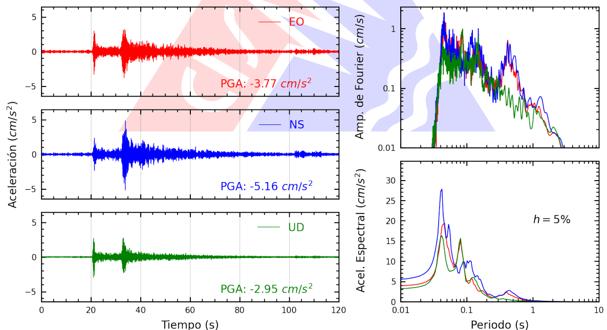
Figura A.2: Registros tiempo-historia, espectros de Fourier y de respuesta en las direcciones EO, NS y vertical de la estación SCTRU. Sismo de Santiago De Chuco, Santiago De Chuco - La Libertad del 2024-09-12, 18:27:13 (Hora local)
