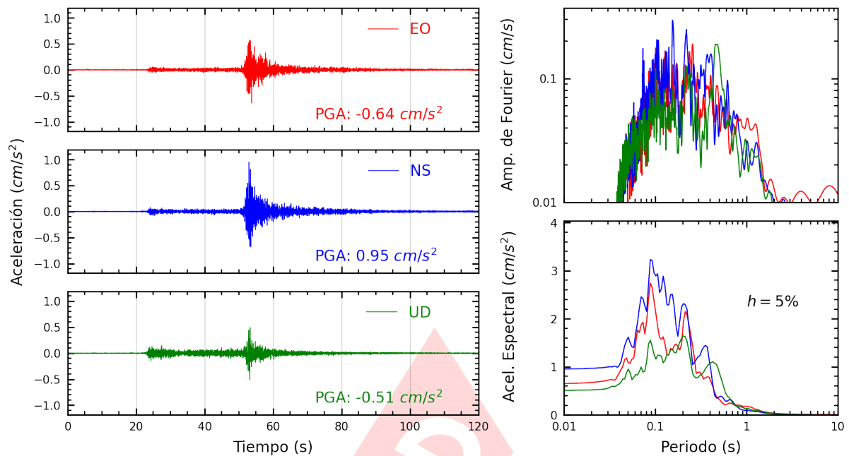
Figura A.3: Registros tiempo-historia, espectros de Fourier y de respuesta en las direcciones EO, NS y vertical de la estación SCCHI. Sismo de Santiago De Chuco, Santiago De Chuco - La Libertad del 2024-09-12, 18:27:13 (Hora local)
