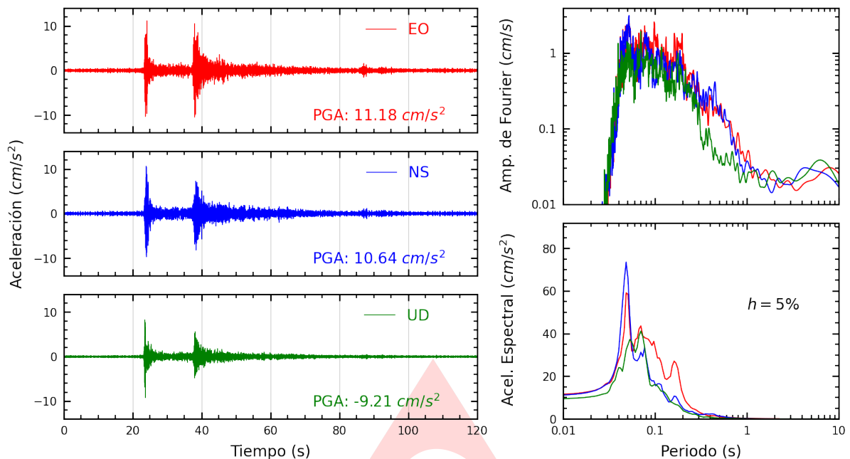
Figura A.1: Registros tiempo-historia, espectros de Fourier y de respuesta en las direcciones EO, NS y vertical de la estación USP. Sismo de Santiago De Chuco, Santiago De Chuco - La Libertad del 2024-09-12, 18:27:13 (Hora local)
