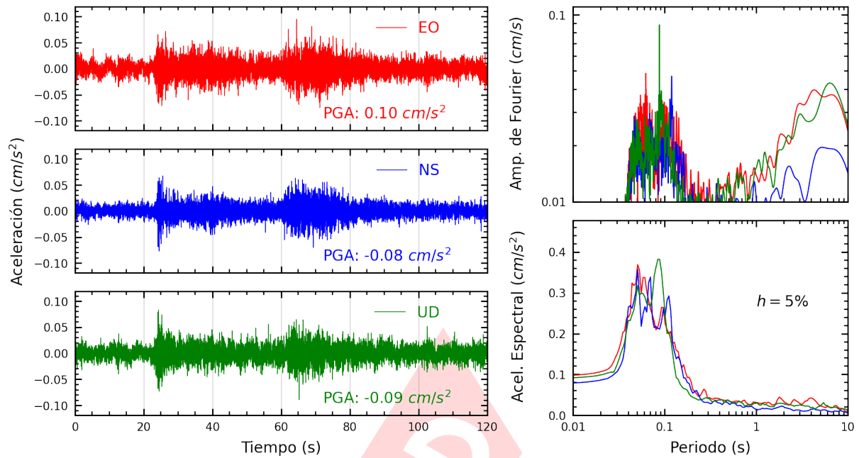
Figura A.3: Registros tiempo-historia, espectros de Fourier y de respuesta en las direcciones EO, NS y vertical de la estación AMORE. Sismo de Aguaytia, Padre Abad - Ucayali del 2024-09-19, 12:11:30 (Hora local)
