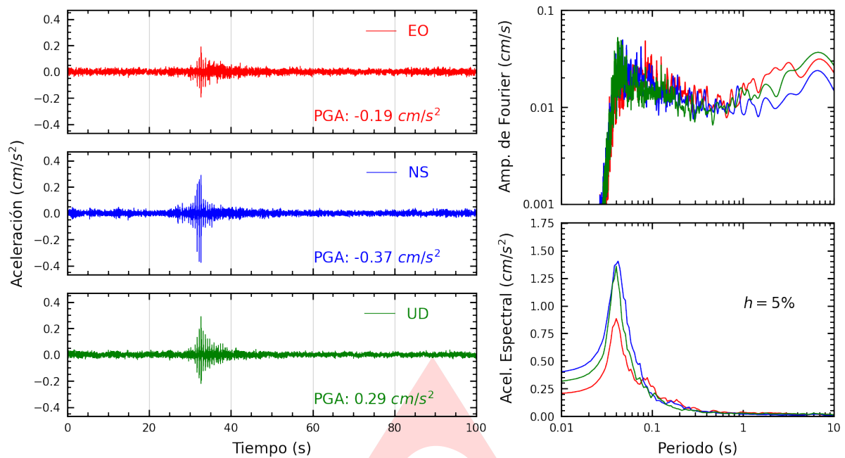
Figura A.1: Registros tiempo-historia, espectros de Fourier y de respuesta en las direcciones EO, NS y vertical de la estación USILP. Sismo de Aguaytia, Padre Abad - Ucayali del 2024-09-19, 12:11:30 (Hora local)
