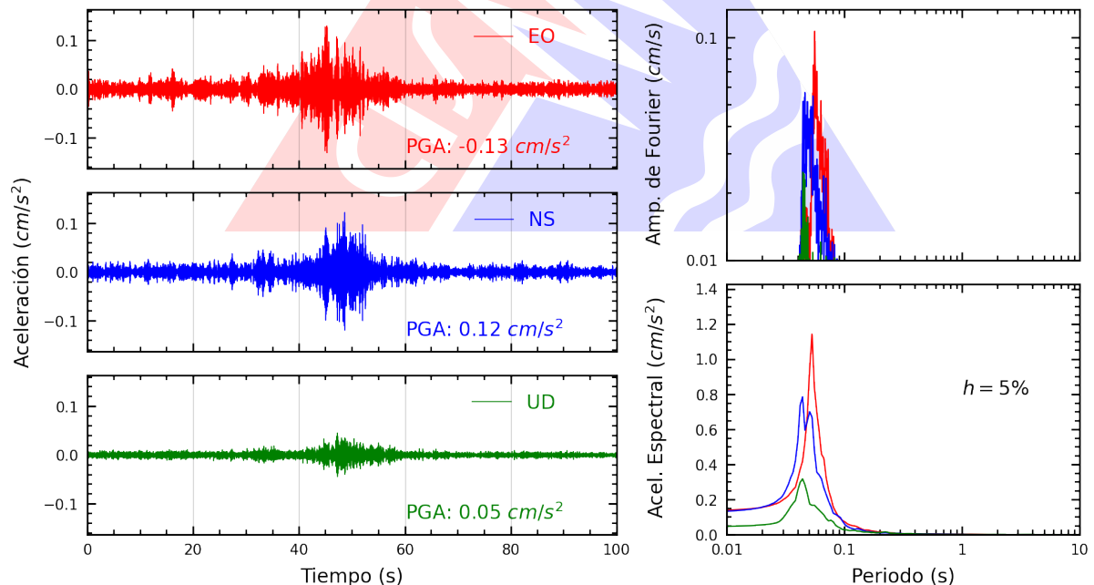
Figura A.2: Registros tiempo-historia, espectros de Fourier y de respuesta en las direcciones EO, NS y vertical de la estación UNMBA. Sismo de Aguaytia, Padre Abad - Ucayali del 2024-09-19, 12:11:30 (Hora local)
