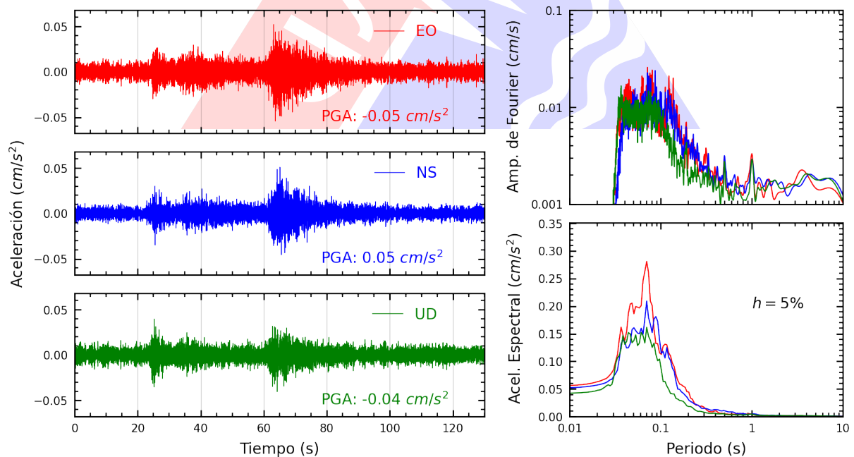
Figura A.4: Registros tiempo-historia, espectros de Fourier y de respuesta en las direcciones EO, NS y vertical de la estación ATARJ. Sismo de Aguaytia, Padre Abad - Ucayali del 2024-09-19, 12:11:30 (Hora local)
