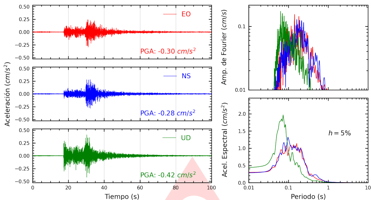
Figura A.1: Registros tiempo-historia, espectros de Fourier y de respuesta en las direcciones EO, NS y vertical de la estación UNAAA. Sismo de Moyobamba, Moyobamba - San Martín del 2024-09-24, 04:26:49 (Hora local)
