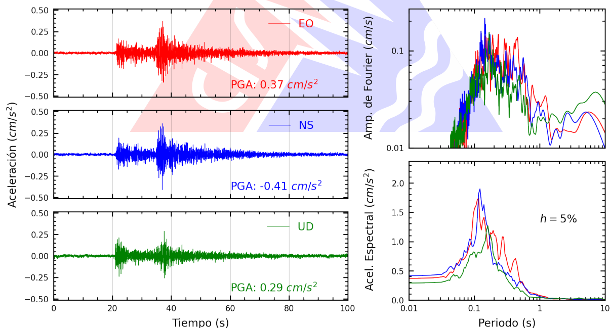
Figura A.2: Registros tiempo-historia, espectros de Fourier y de respuesta en las direcciones EO, NS y vertical de la estación UNTRM. Sismo de Moyobamba, Moyobamba - San Martín del 2024-09-24, 04:26:49 (Hora local)
