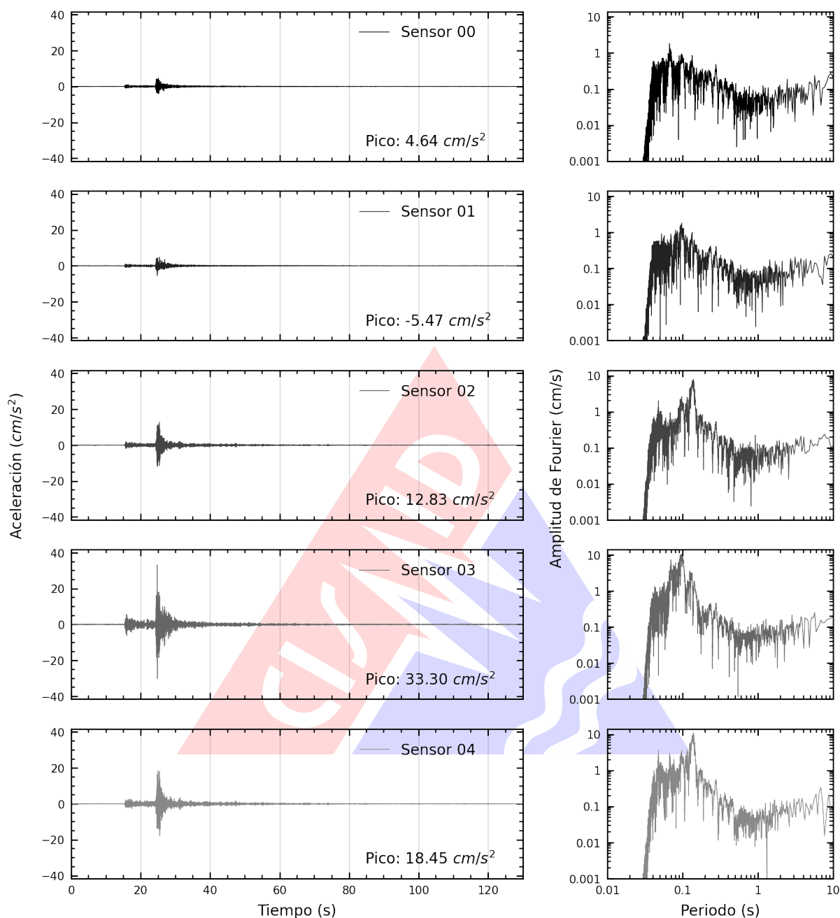
Figura A.1: Registros tiempo-historia y espectros de Fourier en la dirección EW de la edificación Centro de Observación para la Ingeniería Sísmica del CISMID-FIC-UNI. Sismo de Ancon, Lima - Lima del 2024-09-26, 09:38:13 (Hora local)
