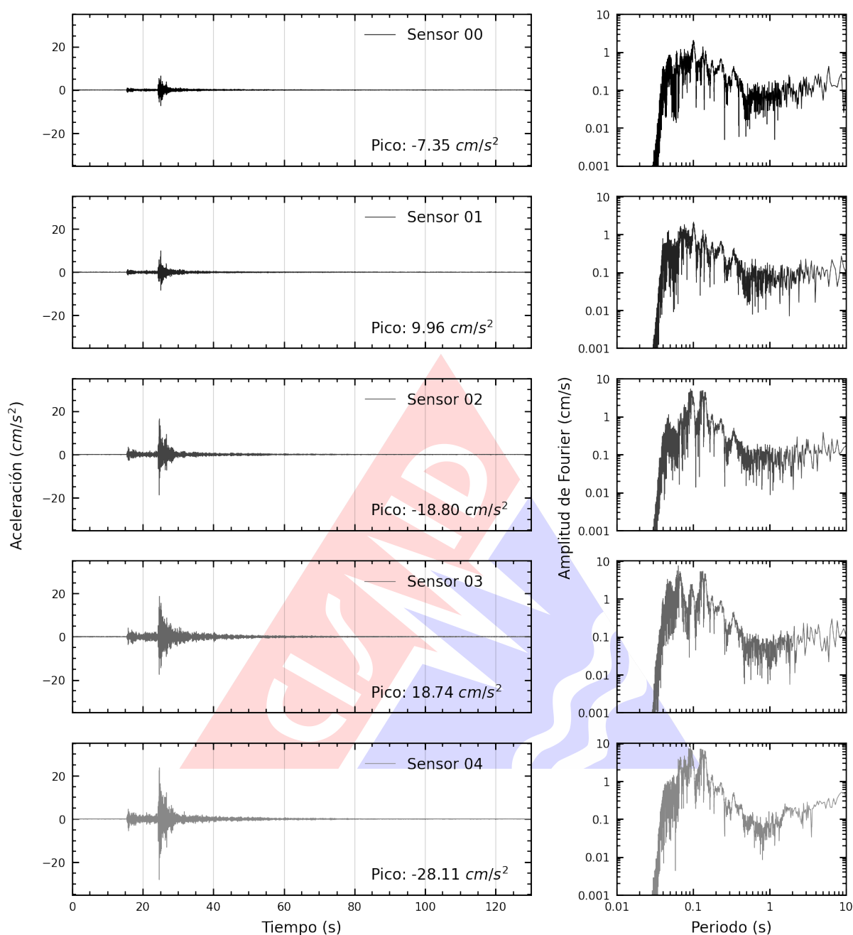
Figura A.2: Registros tiempo-historia y espectros de Fourier en la dirección NS de la edificación Centro de Observación para la Ingeniería Sísmica del CISMID-FIC-UNI. Sismo de Ancon, Lima - Lima del 2024-09-26, 09:38:13 (Hora local)
