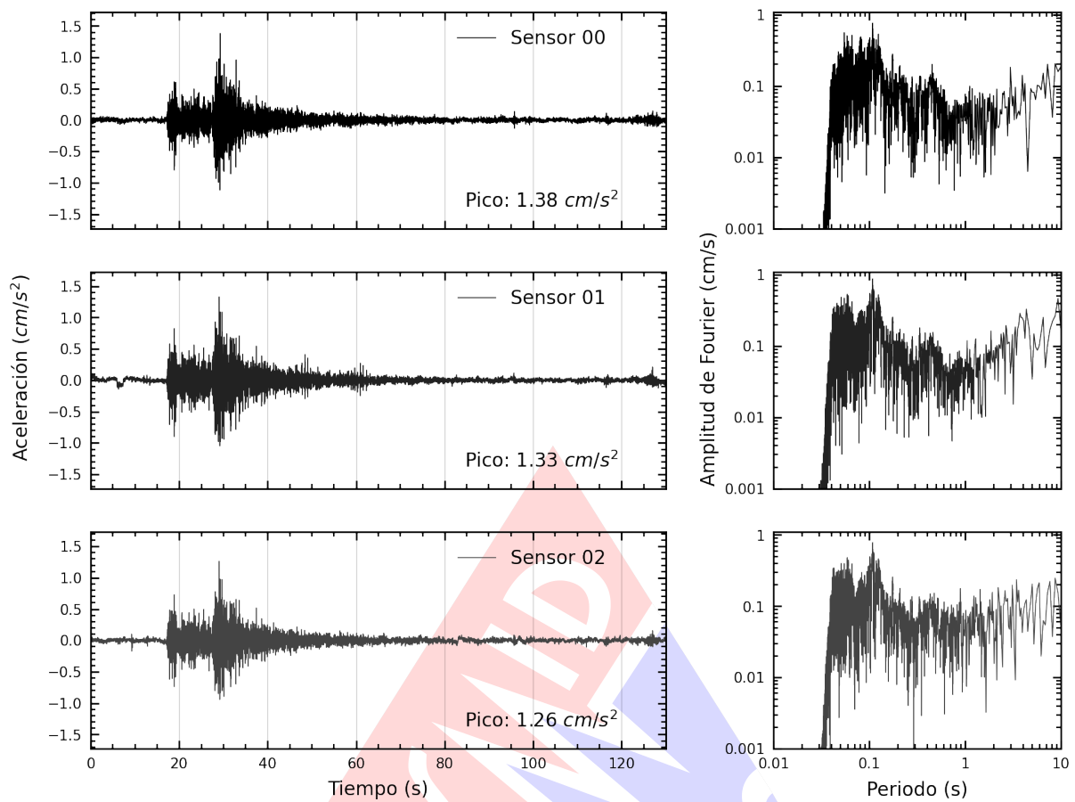
Figura A.3: Registros tiempo-historia y espectros de Fourier en la dirección vertical de la edificación Vivienda. Sismo de Ancon, Lima - Lima del 2024-09-26, 09:38:13 (Hora local)
