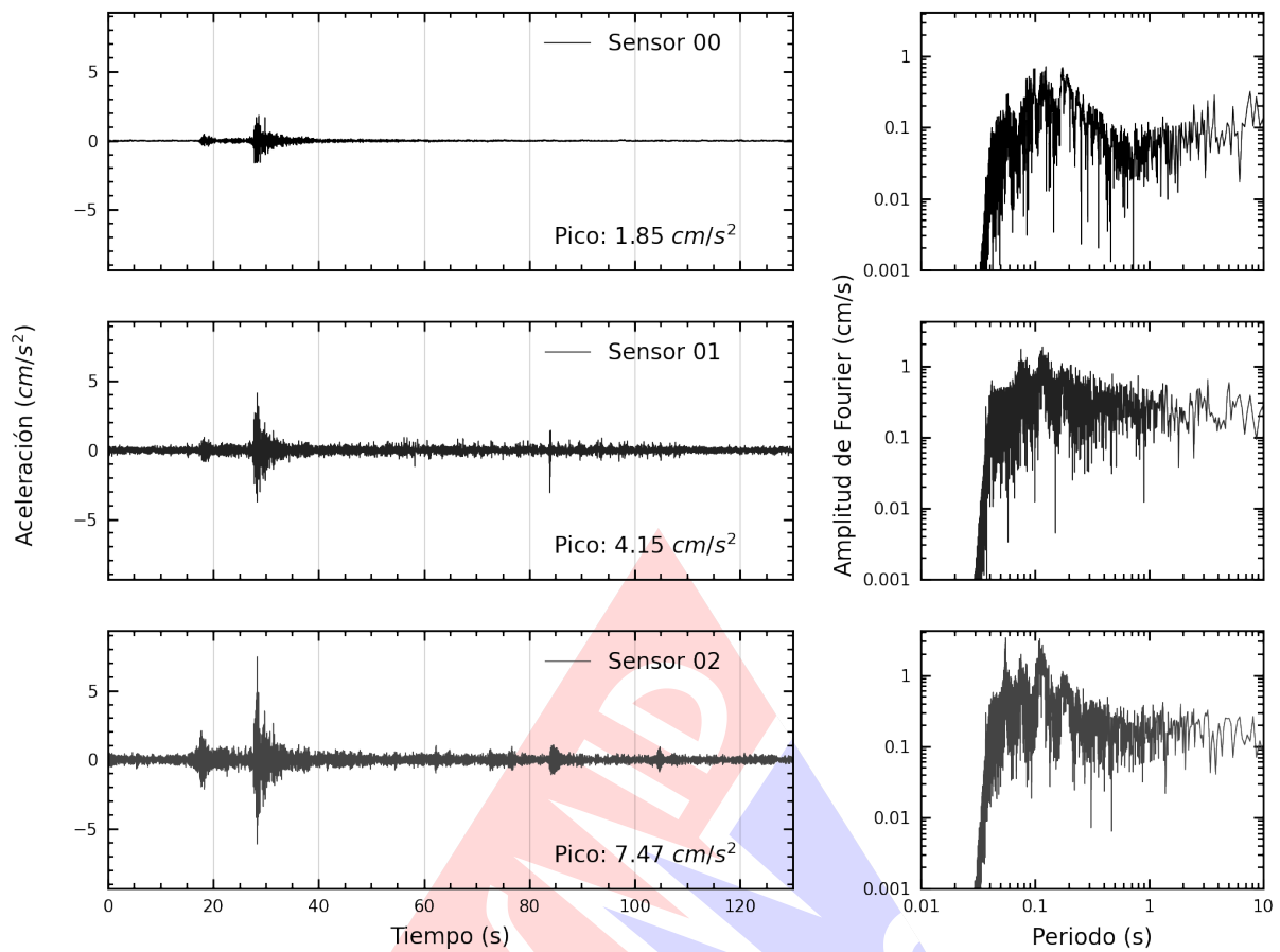
Figura A.2: Registros tiempo-historia y espectros de Fourier en la dirección NS de la edificación Instituto Nacional de Rehabilitación (INR), Chorrillos. Sismo de Ancon, Lima - Lima del 2024-09-26, 09:38:13 (Hora local)
