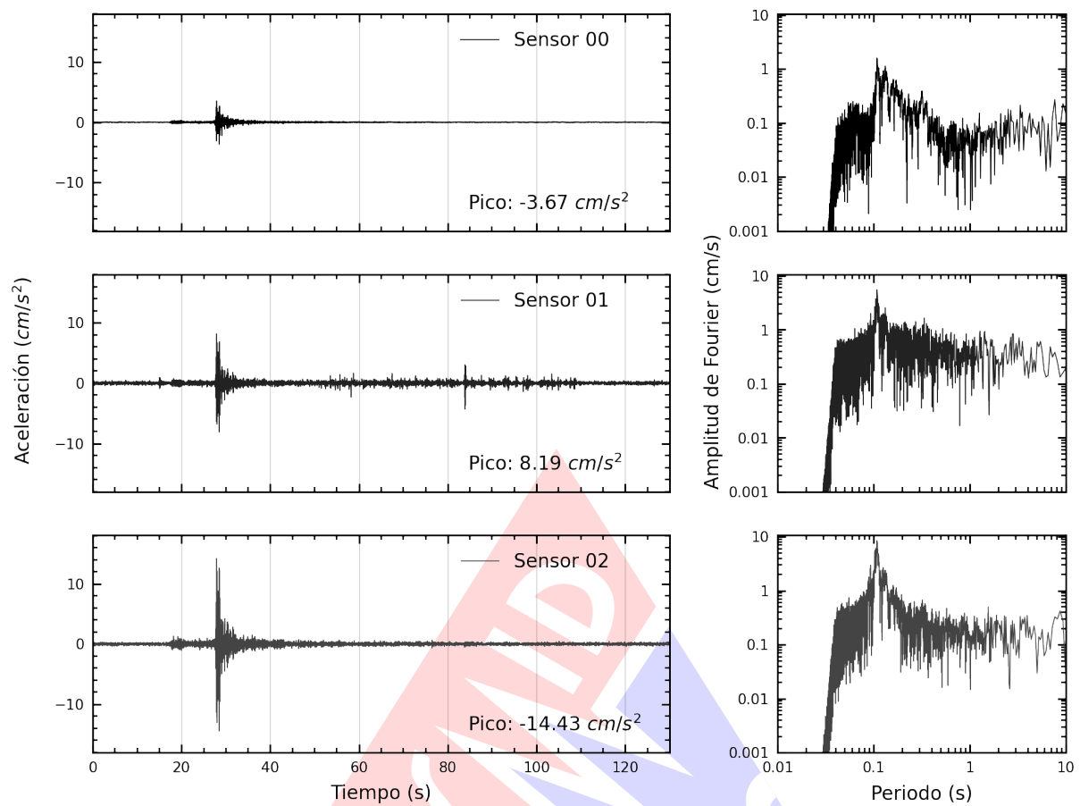
Figura A.1: Registros tiempo-historia y espectros de Fourier en la dirección EW de la edificación Instituto Nacional de Rehabilitación (INR), Chorrillos. Sismo de Ancon, Lima - Lima del 2024-09-26, 09:38:13 (Hora local)
