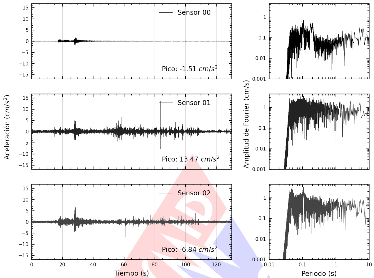
Figura A.3: Registros tiempo-historia y espectros de Fourier en la dirección vertical de la edificación Instituto Nacional de Rehabilitación (INR), Chorrillos. Sismo de Ancon, Lima - Lima del 2024-09-26, 09:38:13 (Hora local)
