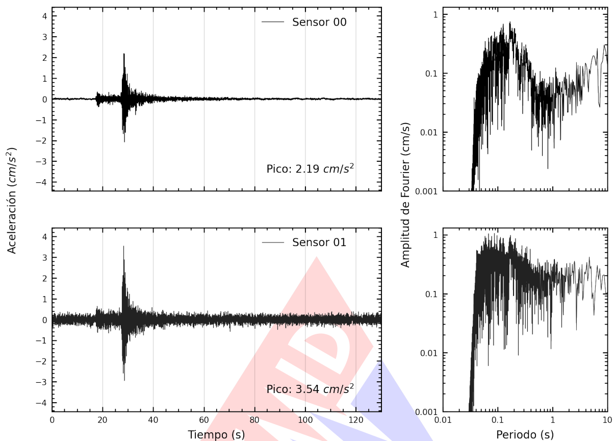
Figura A.2: Registros tiempo-historia y espectros de Fourier en la dirección NS de la edificación Instituto Nacional de Rehabilitación (INR), Chorrillos. Sismo de Ancon, Lima - Lima del 2024-09-26, 09:38:13 (Hora local)
