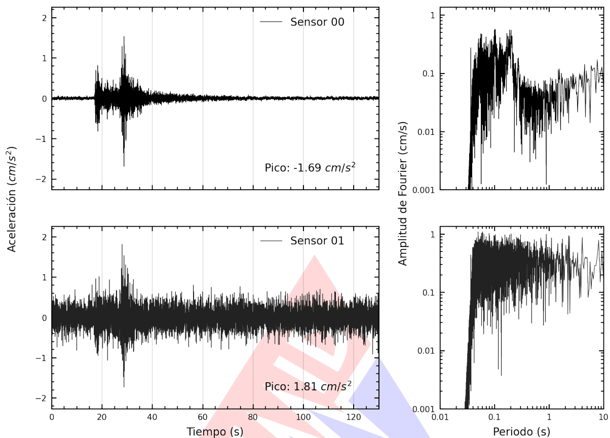
Figura A.3: Registros tiempo-historia y espectros de Fourier en la dirección vertical de la edificación Instituto Nacional de Rehabilitación (INR), Chorrillos. Sismo de Ancon, Lima - Lima del 2024-09-26, 09:38:13 (Hora local)
