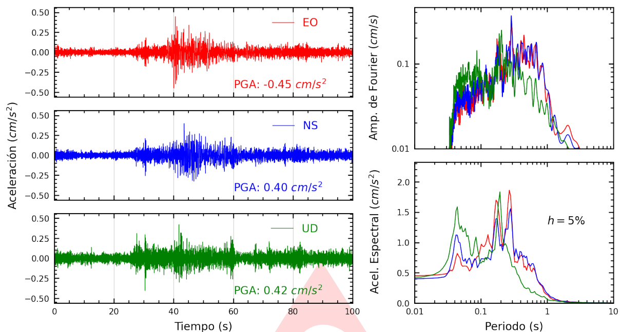
Figura A.1: Registros tiempo-historia, espectros de Fourier y de respuesta en las direcciones EO, NS y vertical de la estación UNICA. Sismo de Marcona, Nazca - Ica del 2024-09-26, 13:49:07 (Hora local)
