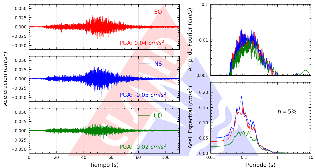
Figura A.3: Registros tiempo-historia, espectros de Fourier y de respuesta en las direcciones EO, NS y vertical de la estación UNSA2. Sismo de Chala, Caraveli - Arequipa del 2024-09-29, 02:02:30 (Hora local)
