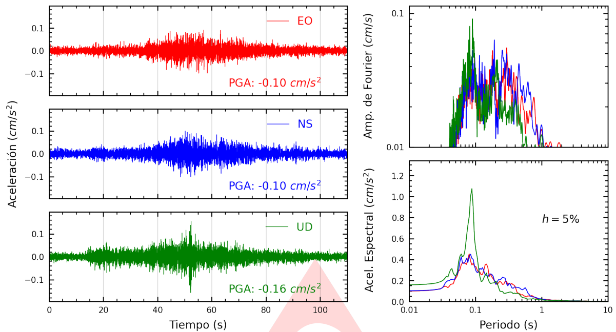
Figura A.1: Registros tiempo-historia, espectros de Fourier y de respuesta en las direcciones EO, NS y vertical de la estación UNICA. Sismo de Chala, Caraveli - Arequipa del 2024-09-29, 02:02:30 (Hora local)
