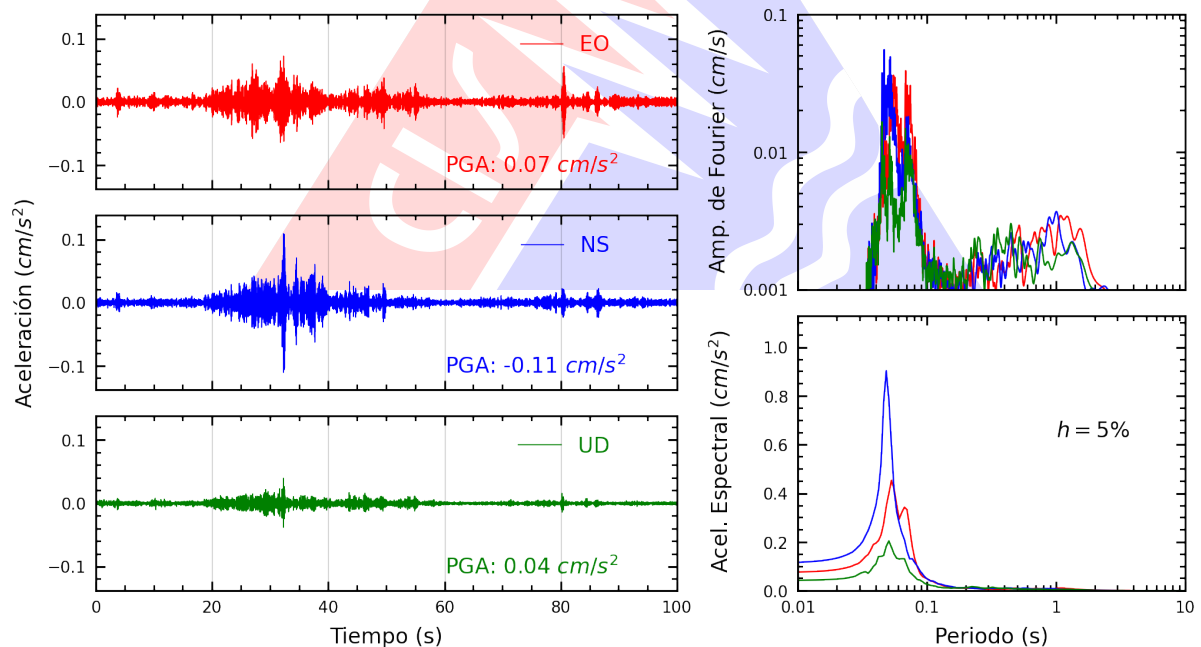
Figura A.2: Registros tiempo-historia, espectros de Fourier y de respuesta en las direcciones EO, NS y vertical de la estación UNMBA. Sismo de Chala, Caraveli - Arequipa del 2024-09-29, 02:02:30 (Hora local)
