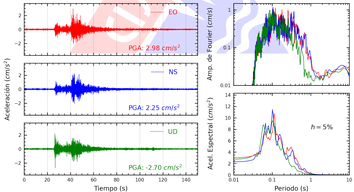
Figura A.30: Registros tiempo-historia, espectros de Fourier y de respuesta en las direcciones EO, NS y vertical de la estación MADRE. Sismo de Yauyos, Yauyos - Lima del 2024-09-30, 06:36:46 (Hora local)
