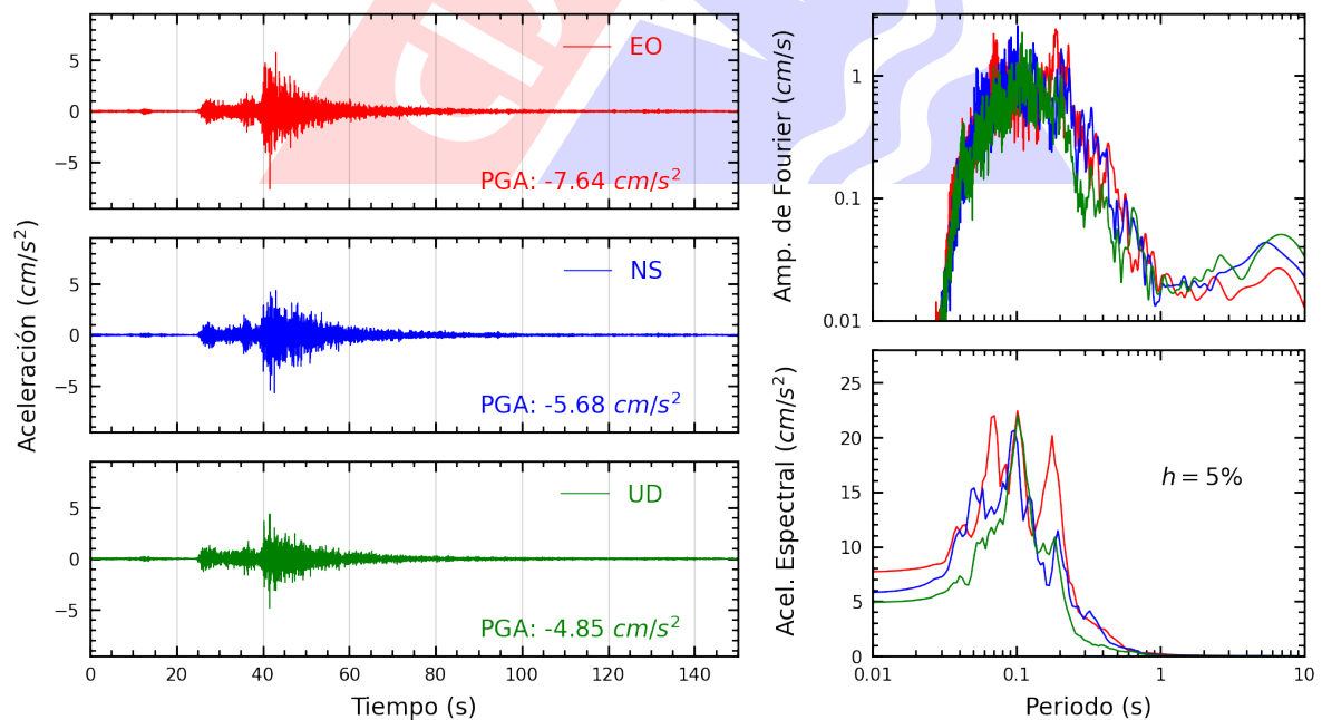
Figura A.8: Registros tiempo-historia, espectros de Fourier y de respuesta en las direcciones EO, NS y vertical de la estación INDEP. Sismo de Yauyos, Yauyos - Lima del 2024-09-30, 06:36:46 (Hora local)
