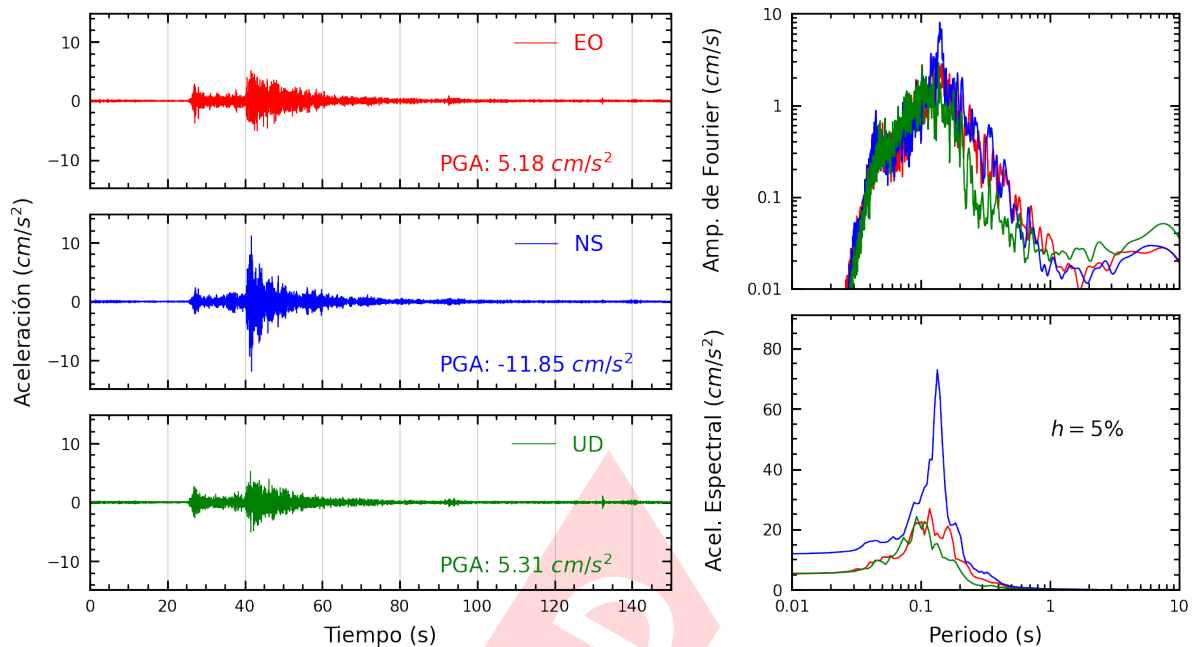
Figura A.3: Registros tiempo-historia, espectros de Fourier y de respuesta en las direcciones EO, NS y vertical de la estación CARAB. Sismo de Yauyos, Yauyos - Lima del 2024-09-30, 06:36:46 (Hora local)
