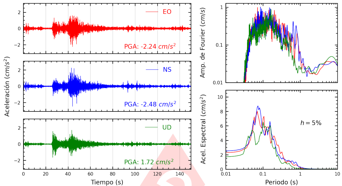
Figura A.33: Registros tiempo-historia, espectros de Fourier y de respuesta en las direcciones EO, NS y vertical de la estación UPCS. Sismo de Yauyos, Yauyos - Lima del 2024-09-30, 06:36:46 (Hora local)
