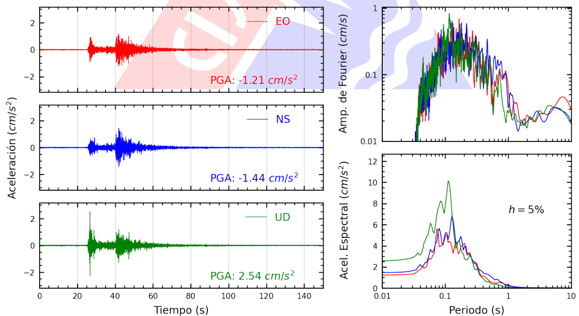
Figura A.32: Registros tiempo-historia, espectros de Fourier y de respuesta en las direcciones EO, NS y vertical de la estación BONDY. Sismo de Yauyos, Yauyos - Lima del 2024-09-30, 06:36:46 (Hora local)
