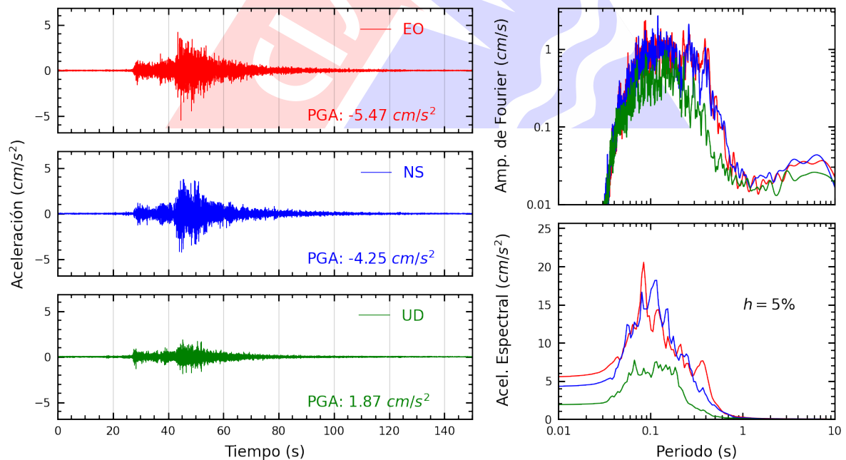
Figura A.12: Registros tiempo-historia, espectros de Fourier y de respuesta en las direcciones EO, NS y vertical de la estación DEFEN. Sismo de Yauyos, Yauyos - Lima del 2024-09-30, 06:36:46 (Hora local)
