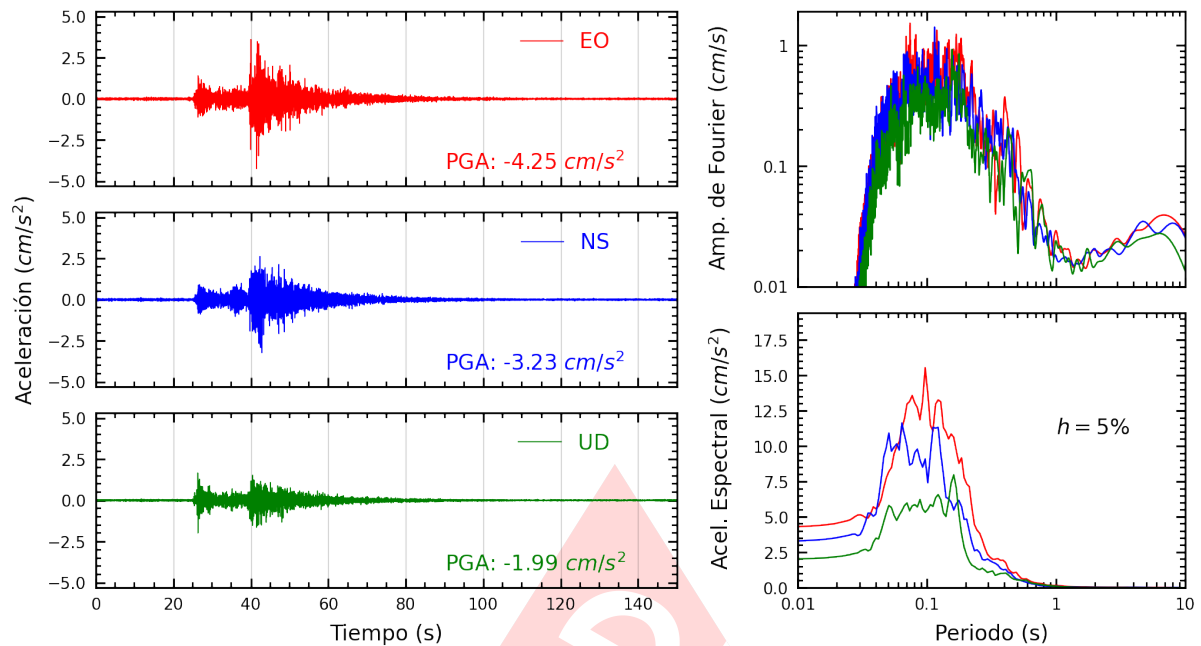
Figura A.19: Registros tiempo-historia, espectros de Fourier y de respuesta en las direcciones EO, NS y vertical de la estación FICPE. Sismo de Yauyos, Yauyos - Lima del 2024-09-30, 06:36:46 (Hora local)
