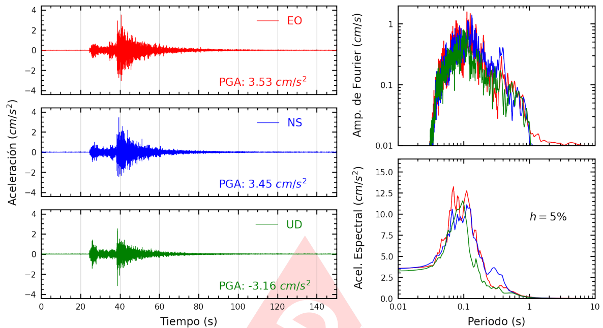
Figura A.25: Registros tiempo-historia, espectros de Fourier y de respuesta en las direcciones EO, NS y vertical de la estación ATARJ. Sismo de Yauyos, Yauyos - Lima del 2024-09-30, 06:36:46 (Hora local)
