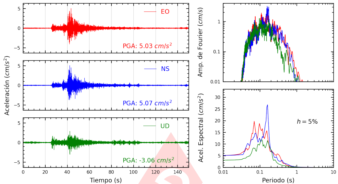
Figura A.15: Registros tiempo-historia, espectros de Fourier y de respuesta en las direcciones EO, NS y vertical de la estación SCOLI. Sismo de Yauyos, Yauyos - Lima del 2024-09-30, 06:36:46 (Hora local)
