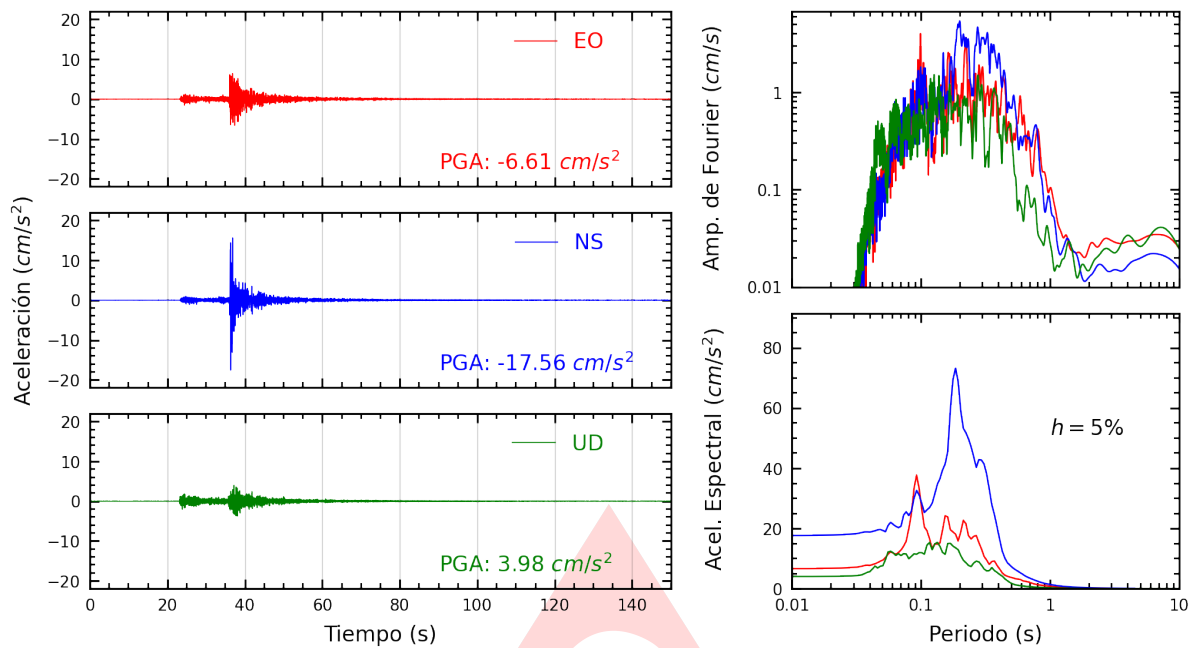
Figura A.1: Registros tiempo-historia, espectros de Fourier y de respuesta en las direcciones EO, NS y vertical de la estación USILP. Sismo de Yauyos, Yauyos - Lima del 2024-09-30, 06:36:46 (Hora local)
