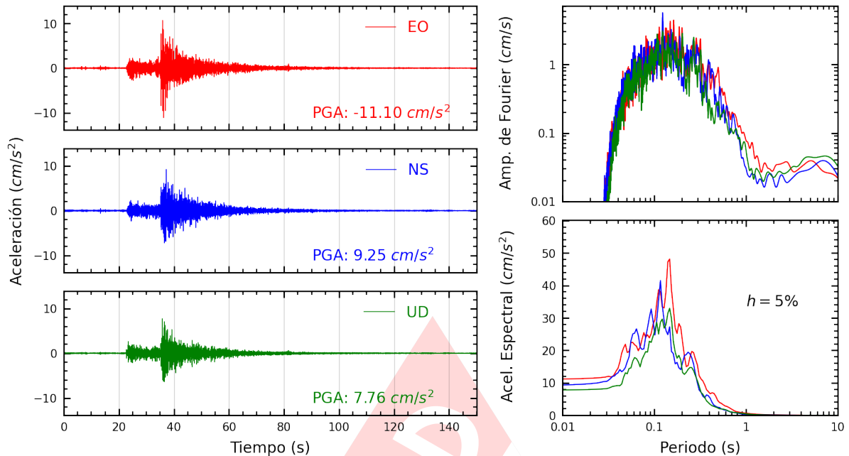
Figura A.5: Registros tiempo-historia, espectros de Fourier y de respuesta en las direcciones EO, NS y vertical de la estación PHERM. Sismo de Yauyos, Yauyos - Lima del 2024-09-30, 06:36:46 (Hora local)
