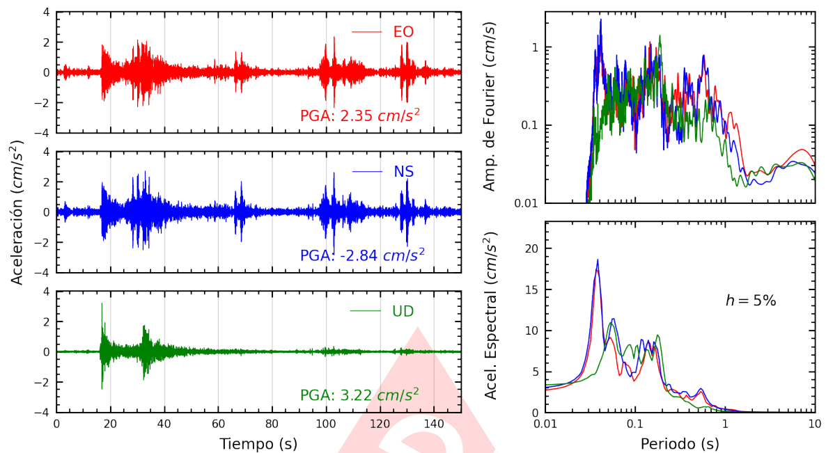
Figura A.27: Registros tiempo-historia, espectros de Fourier y de respuesta en las direcciones EO, NS y vertical de la estación DHNPE. Sismo de Yauyos, Yauyos - Lima del 2024-09-30, 06:36:46 (Hora local)
