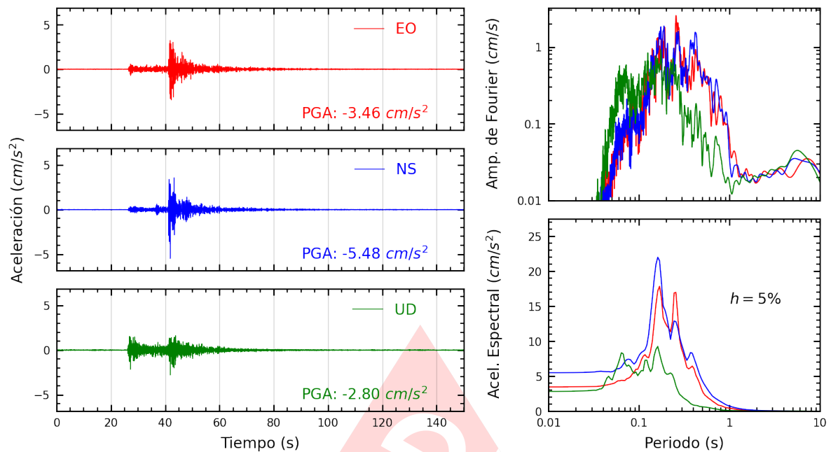
Figura A.11: Registros tiempo-historia, espectros de Fourier y de respuesta en las direcciones EO, NS y vertical de la estación ACAPU. Sismo de Yauyos, Yauyos - Lima del 2024-09-30, 06:36:46 (Hora local)
