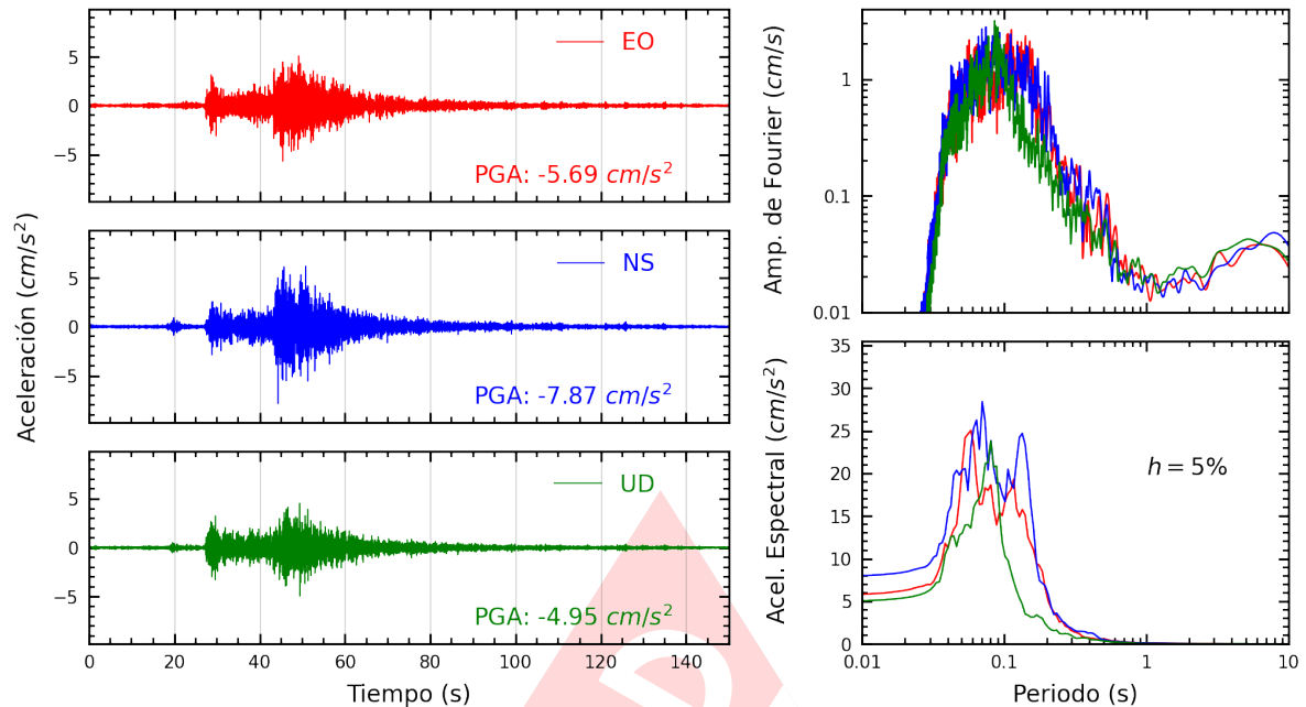
Figura A.7: Registros tiempo-historia, espectros de Fourier y de respuesta en las direcciones EO, NS y vertical de la estación SROSA. Sismo de Yauyos, Yauyos - Lima del 2024-09-30, 06:36:46 (Hora local)
