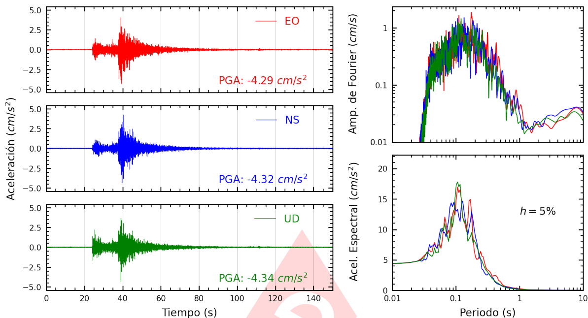
Figura A.17: Registros tiempo-historia, espectros de Fourier y de respuesta en las direcciones EO, NS y vertical de la estación USMP. Sismo de Yauyos, Yauyos - Lima del 2024-09-30, 06:36:46 (Hora local)
