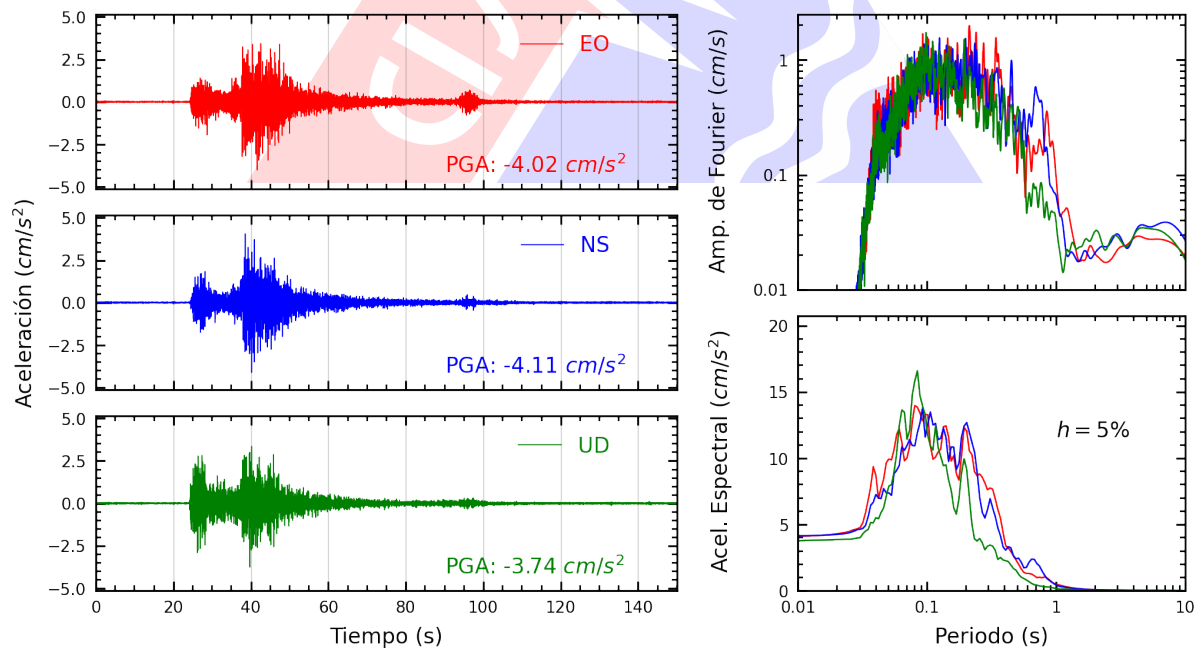
Figura A.22: Registros tiempo-historia, espectros de Fourier y de respuesta en las direcciones EO, NS y vertical de la estación UCVAT. Sismo de Yauyos, Yauyos - Lima del 2024-09-30, 06:36:46 (Hora local)
