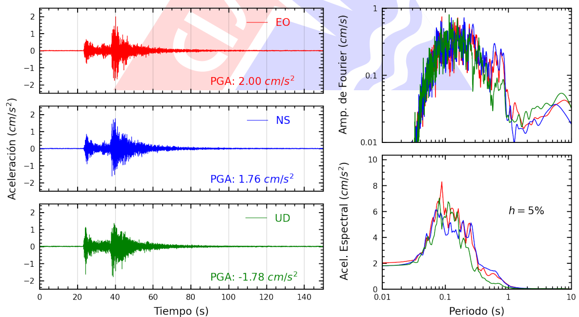
Figura A.38: Registros tiempo-historia, espectros de Fourier y de respuesta en las direcciones EO, NS y vertical de la estación UNMSM. Sismo de Yauyos, Yauyos - Lima del 2024-09-30, 06:36:46 (Hora local)
