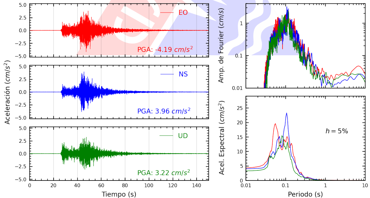
Figura A.20: Registros tiempo-historia, espectros de Fourier y de respuesta en las direcciones EO, NS y vertical de la estación AMORE. Sismo de Yauyos, Yauyos - Lima del 2024-09-30, 06:36:46 (Hora local)
