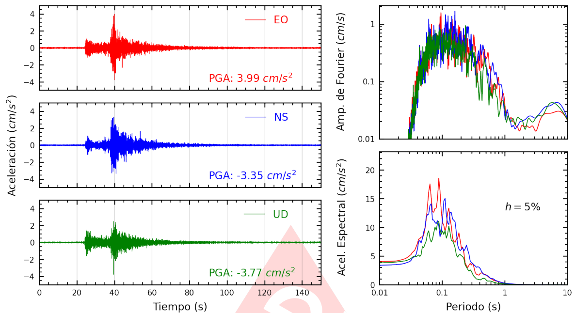
Figura A.23: Registros tiempo-historia, espectros de Fourier y de respuesta en las direcciones EO, NS y vertical de la estación URPE. Sismo de Yauyos, Yauyos - Lima del 2024-09-30, 06:36:46 (Hora local)
