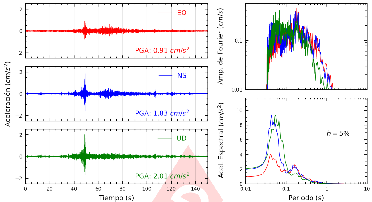
Figura A.37: Registros tiempo-historia, espectros de Fourier y de respuesta en las direcciones EO, NS y vertical de la estación SCICA. Sismo de Yauyos, Yauyos - Lima del 2024-09-30, 06:36:46 (Hora local)
