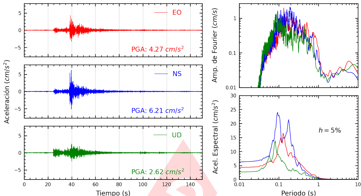
Figura A.9: Registros tiempo-historia, espectros de Fourier y de respuesta en las direcciones EO, NS y vertical de la estación SOCHO. Sismo de Yauyos, Yauyos - Lima del 2024-09-30, 06:36:46 (Hora local)
