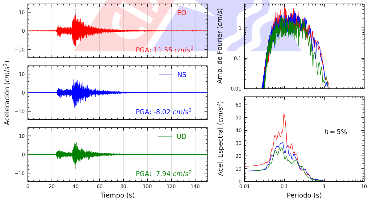
Figura A.4: Registros tiempo-historia, espectros de Fourier y de respuesta en las direcciones EO, NS y vertical de la estación UNTEL. Sismo de Yauyos, Yauyos - Lima del 2024-09-30, 06:36:46 (Hora local)
