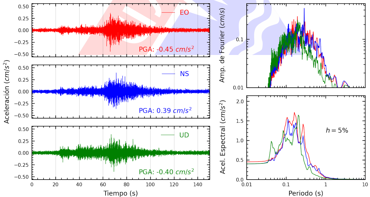
Figura A.42: Registros tiempo-historia, espectros de Fourier y de respuesta en las direcciones EO, NS y vertical de la estación UNICA. Sismo de Yauyos, Yauyos - Lima del 2024-09-30, 06:36:46 (Hora local)
