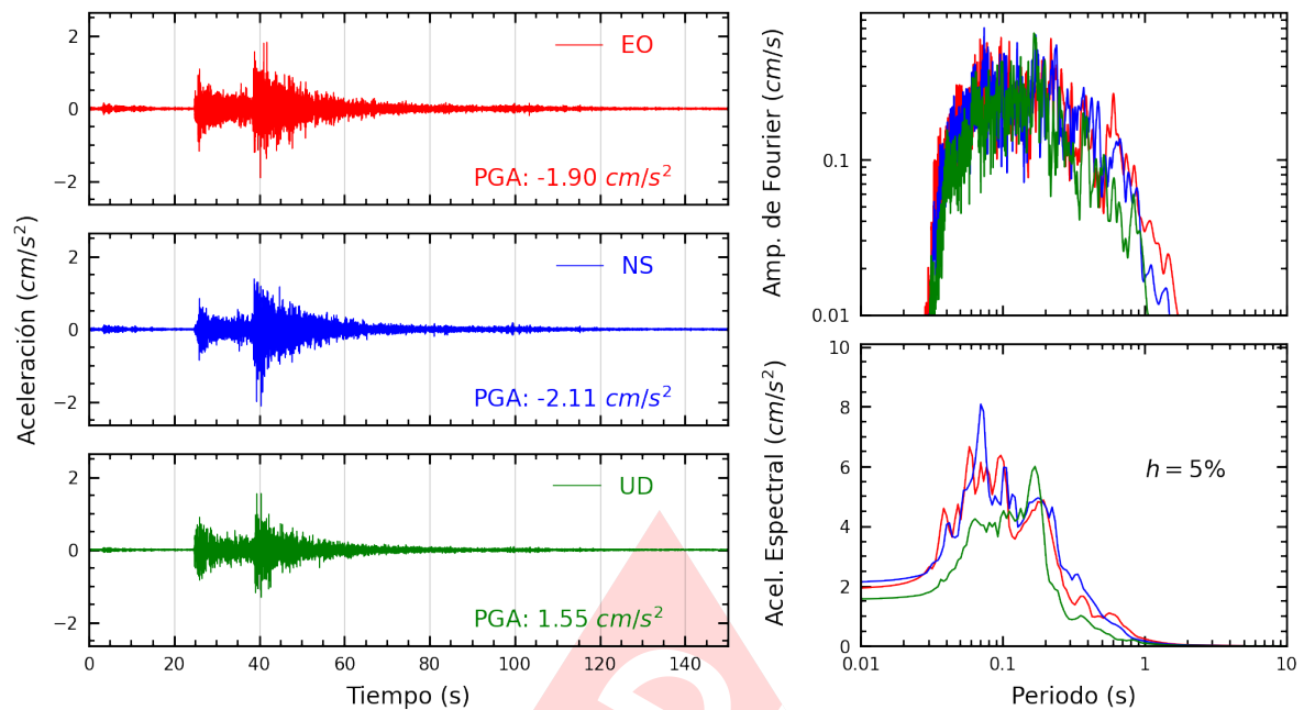
Figura A.35: Registros tiempo-historia, espectros de Fourier y de respuesta en las direcciones EO, NS y vertical de la estación BORJA. Sismo de Yauyos, Yauyos - Lima del 2024-09-30, 06:36:46 (Hora local)
