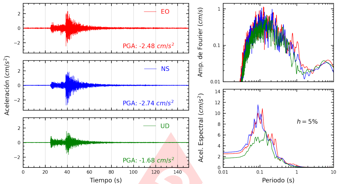
Figura A.31: Registros tiempo-historia, espectros de Fourier y de respuesta en las direcciones EO, NS y vertical de la estación INICT. Sismo de Yauyos, Yauyos - Lima del 2024-09-30, 06:36:46 (Hora local)
