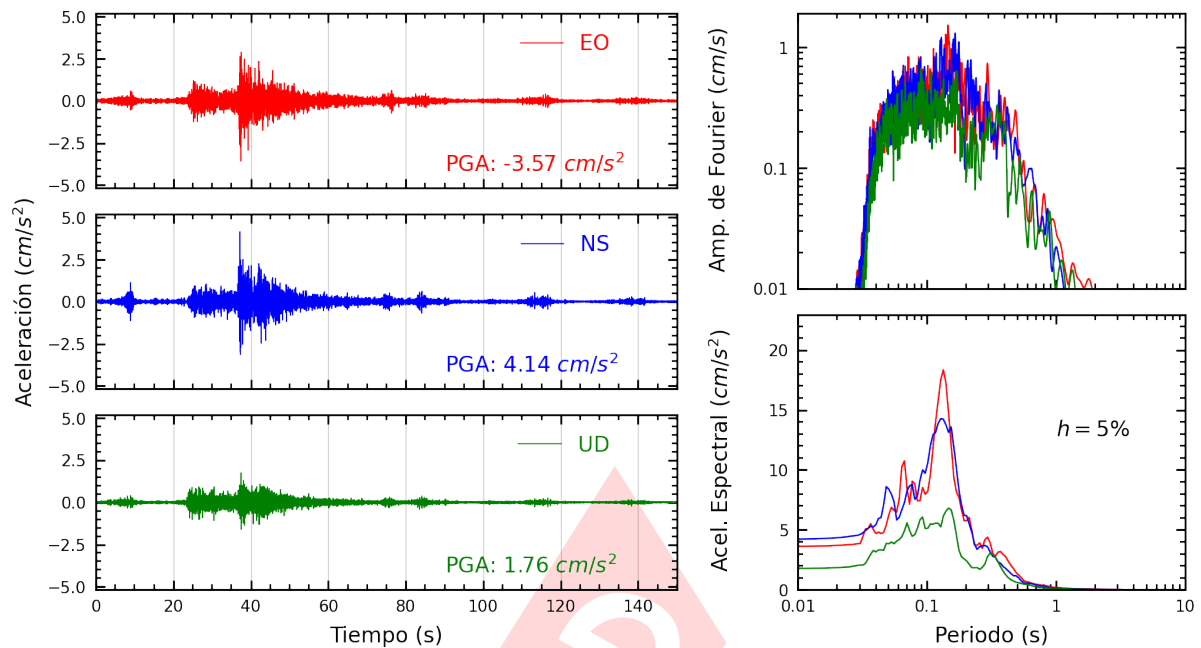
Figura A.21: Registros tiempo-historia, espectros de Fourier y de respuesta en las direcciones EO, NS y vertical de la estación PACHA. Sismo de Yauyos, Yauyos - Lima del 2024-09-30, 06:36:46 (Hora local)
