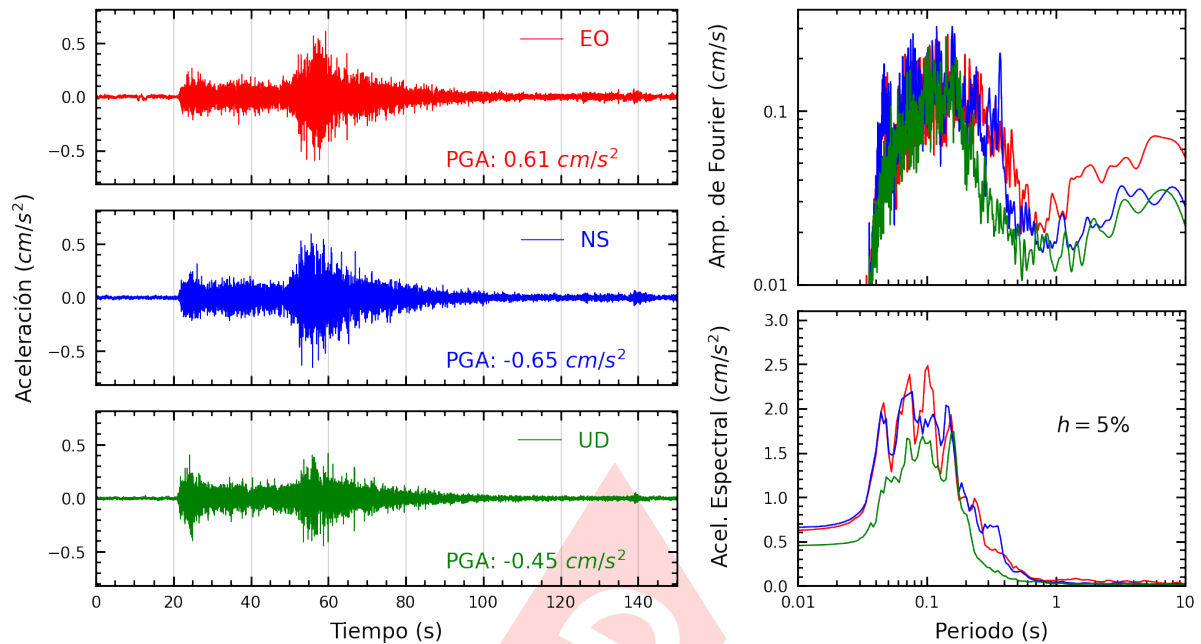
Figura A.41: Registros tiempo-historia, espectros de Fourier y de respuesta en las direcciones EO, NS y vertical de la estación UNAB. Sismo de Yauyos, Yauyos - Lima del 2024-09-30, 06:36:46 (Hora local)
