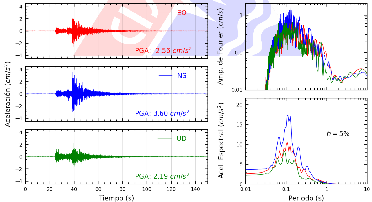
Figura A.24: Registros tiempo-historia, espectros de Fourier y de respuesta en las direcciones EO, NS y vertical de la estación SERVI. Sismo de Yauyos, Yauyos - Lima del 2024-09-30, 06:36:46 (Hora local)
