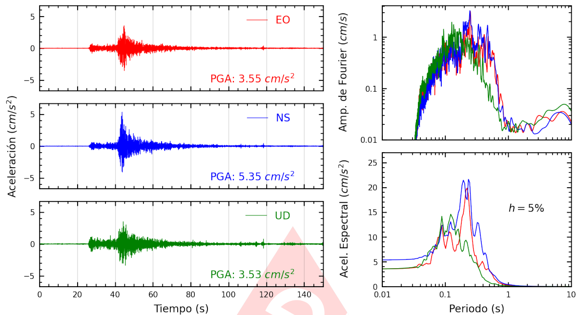
Figura A.13: Registros tiempo-historia, espectros de Fourier y de respuesta en las direcciones EO, NS y vertical de la estación MDPP. Sismo de Yauyos, Yauyos - Lima del 2024-09-30, 06:36:46 (Hora local)
