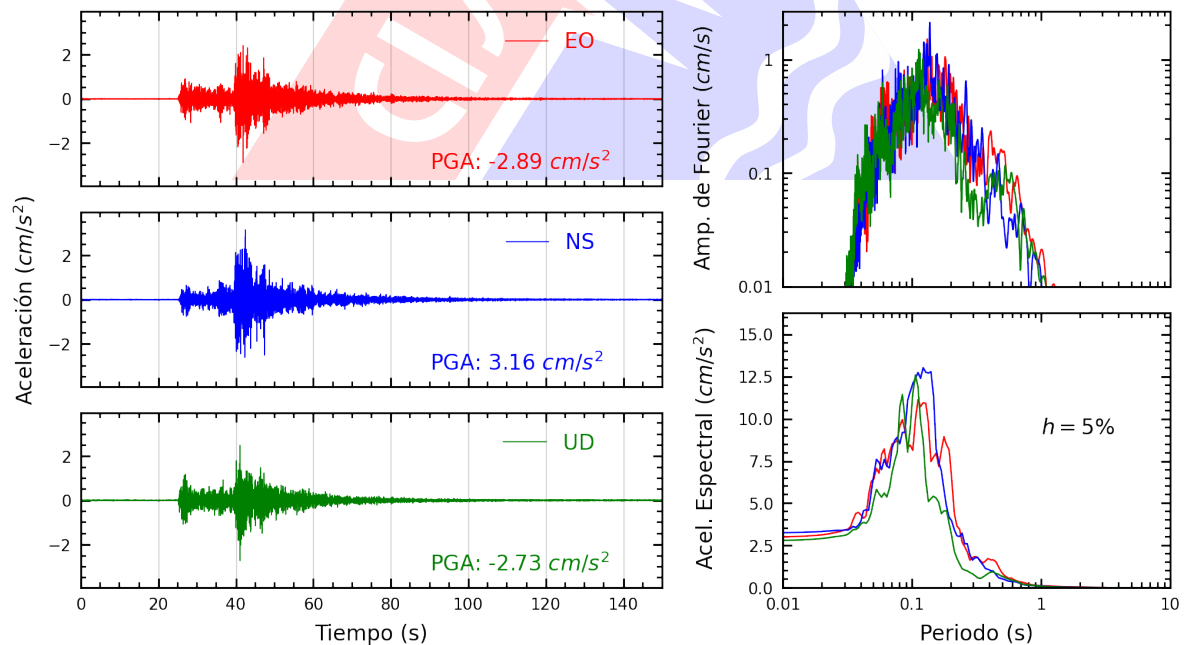
Figura A.28: Registros tiempo-historia, espectros de Fourier y de respuesta en las direcciones EO, NS y vertical de la estación JALV2. Sismo de Yauyos, Yauyos - Lima del 2024-09-30, 06:36:46 (Hora local)
