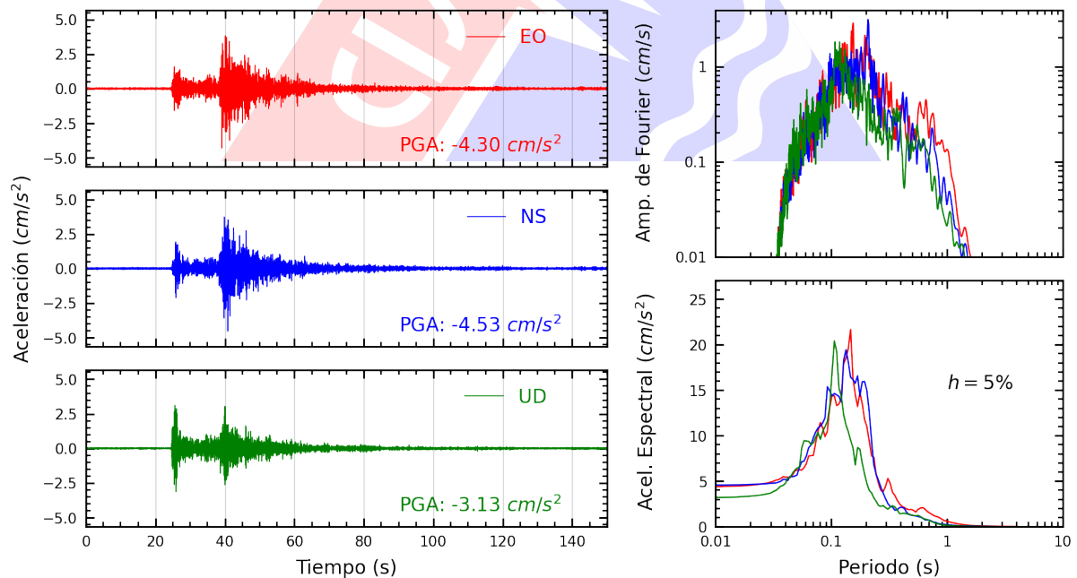
Figura A.16: Registros tiempo-historia, espectros de Fourier y de respuesta en las direcciones EO, NS y vertical de la estación SCCHO. Sismo de Yauyos, Yauyos - Lima del 2024-09-30, 06:36:46 (Hora local)
