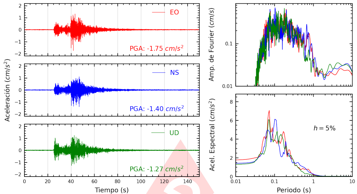
Figura A.39: Registros tiempo-historia, espectros de Fourier y de respuesta en las direcciones EO, NS y vertical de la estación UNFV. Sismo de Yauyos, Yauyos - Lima del 2024-09-30, 06:36:46 (Hora local)
