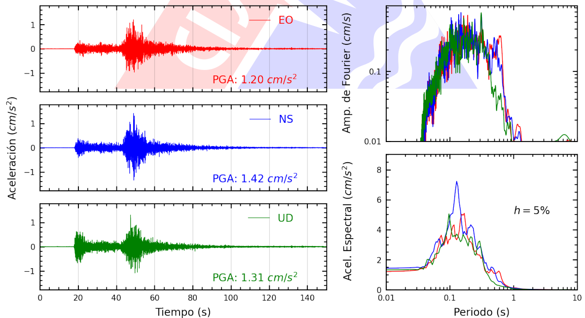
Figura A.40: Registros tiempo-historia, espectros de Fourier y de respuesta en las direcciones EO, NS y vertical de la estación CARAL. Sismo de Yauyos, Yauyos - Lima del 2024-09-30, 06:36:46 (Hora local)
