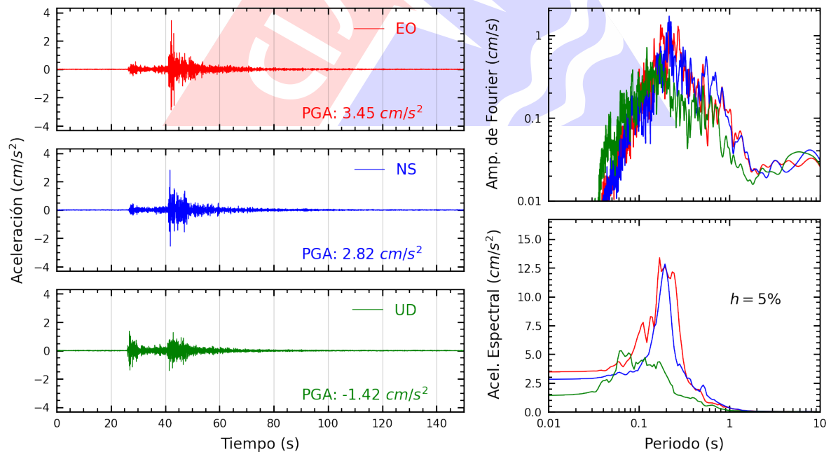
Figura A.26: Registros tiempo-historia, espectros de Fourier y de respuesta en las direcciones EO, NS y vertical de la estación DSMI. Sismo de Yauyos, Yauyos - Lima del 2024-09-30, 06:36:46 (Hora local)
