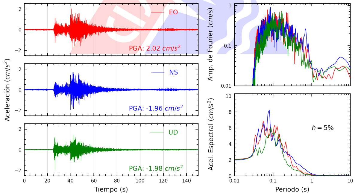
Figura A.36: Registros tiempo-historia, espectros de Fourier y de respuesta en las direcciones EO, NS y vertical de la estación CEPRE. Sismo de Yauyos, Yauyos - Lima del 2024-09-30, 06:36:46 (Hora local)
