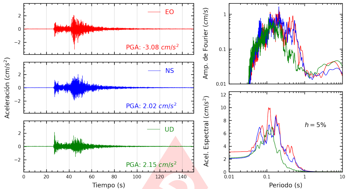
Figura A.29: Registros tiempo-historia, espectros de Fourier y de respuesta en las direcciones EO, NS y vertical de la estación VHAYA. Sismo de Yauyos, Yauyos - Lima del 2024-09-30, 06:36:46 (Hora local)
