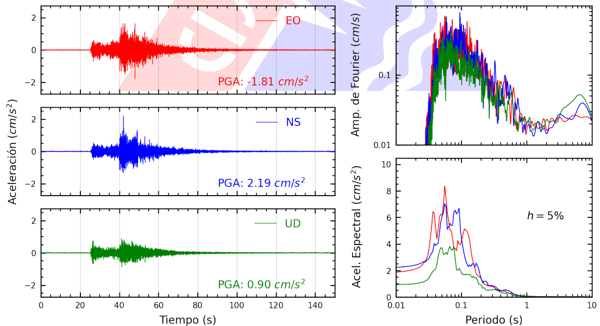
Figura A.34: Registros tiempo-historia, espectros de Fourier y de respuesta en las direcciones EO, NS y vertical de la estación UCSS. Sismo de Yauyos, Yauyos - Lima del 2024-09-30, 06:36:46 (Hora local)
