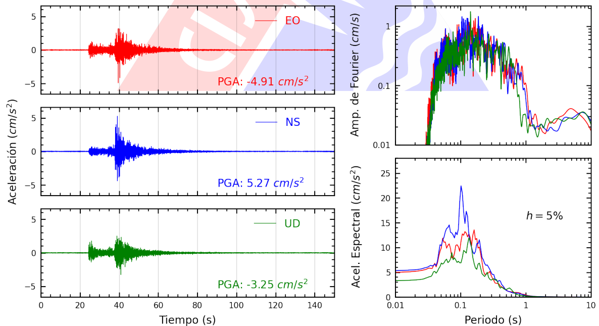
Figura A.14: Registros tiempo-historia, espectros de Fourier y de respuesta en las direcciones EO, NS y vertical de la estación IMCA. Sismo de Yauyos, Yauyos - Lima del 2024-09-30, 06:36:46 (Hora local)
