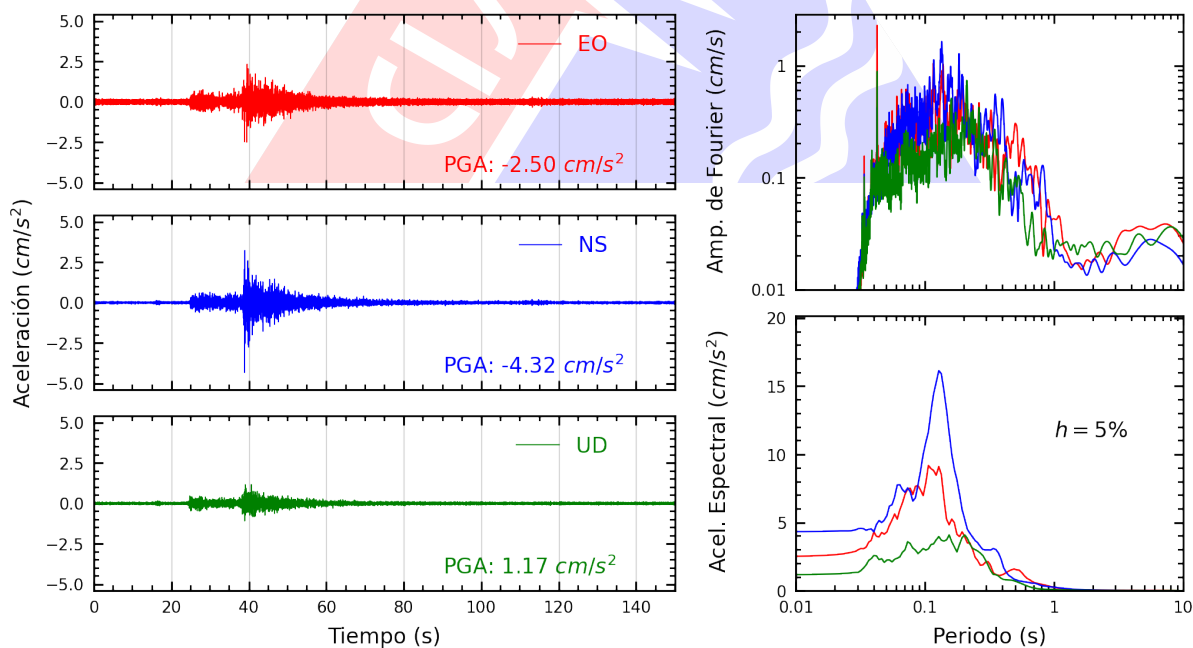
Figura A.18: Registros tiempo-historia, espectros de Fourier y de respuesta en las direcciones EO, NS y vertical de la estación UPCVI. Sismo de Yauyos, Yauyos - Lima del 2024-09-30, 06:36:46 (Hora local)
