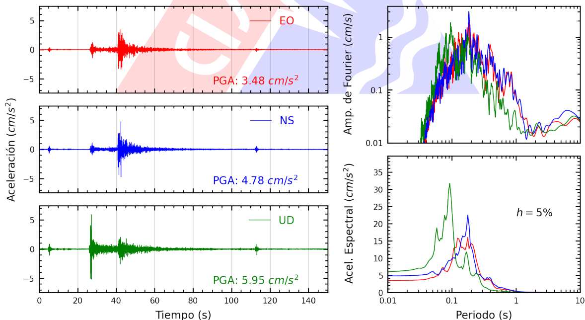
Figura A.10: Registros tiempo-historia, espectros de Fourier y de respuesta en las direcciones EO, NS y vertical de la estación RAMON. Sismo de Yauyos, Yauyos - Lima del 2024-09-30, 06:36:46 (Hora local)
