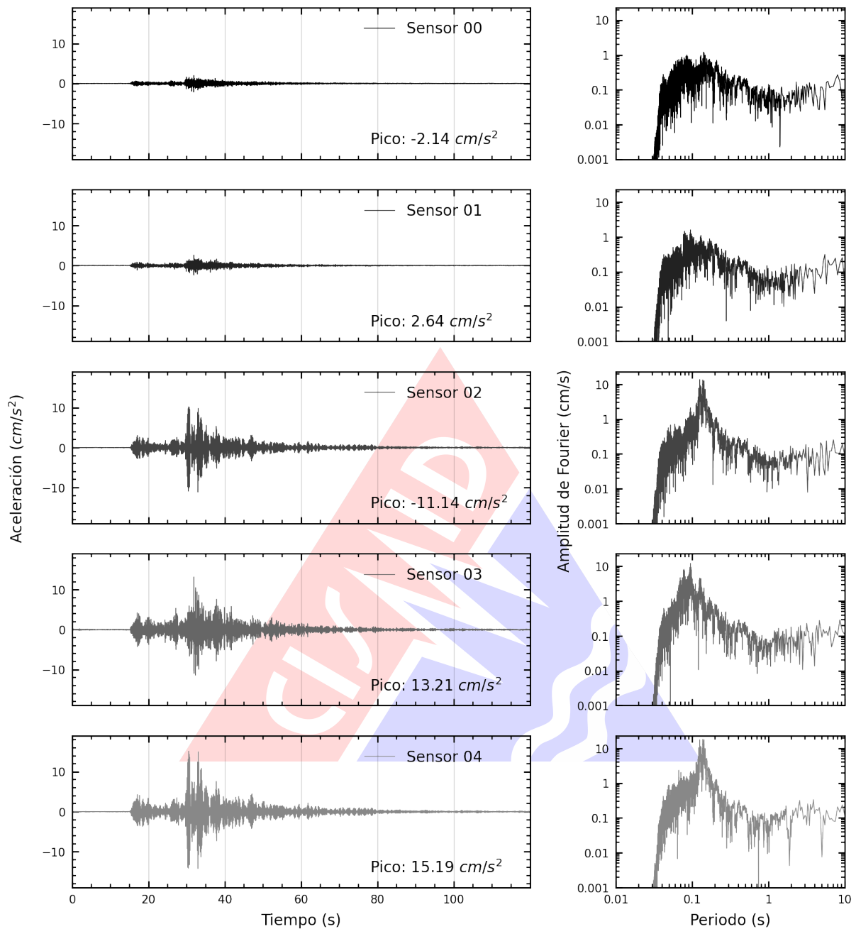
Figura A.1: Registros tiempo-historia y espectros de Fourier en la dirección EW de la edificación Centro de Observación para la Ingeniería Sísmica del CISMID-FIC-UNI. Sismo de Yauyos, Yauyos - Lima del 2024-09-30, 06:36:46 (Hora local)
