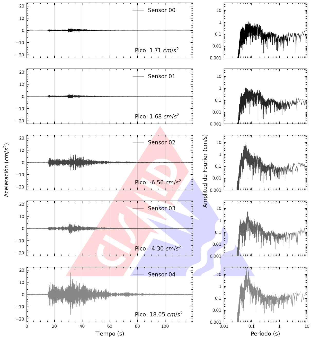
Figura A.3: Registros tiempo-historia y espectros de Fourier en la dirección vertical de la edificación Centro de Observación para la Ingeniería Sísmica del CISMID-FIC-UNI. Sismo de Yauyos, Yauyos - Lima del 2024-09-30, 06:36:46 (Hora local)
