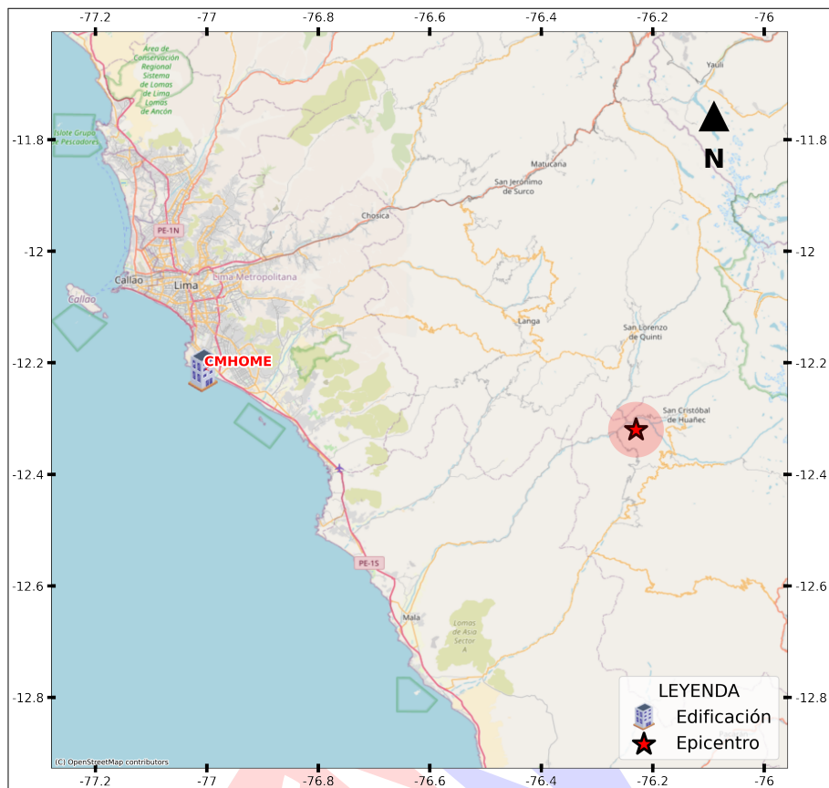
Figura 2: Mapa de ubicación de la edificación monitoreada a nivel nacional correspondiente(s) al Sismo de Yauyos, Yauyos - Lima del 30 de setiembre de 2024 a las 06:36:46 (hora local)
