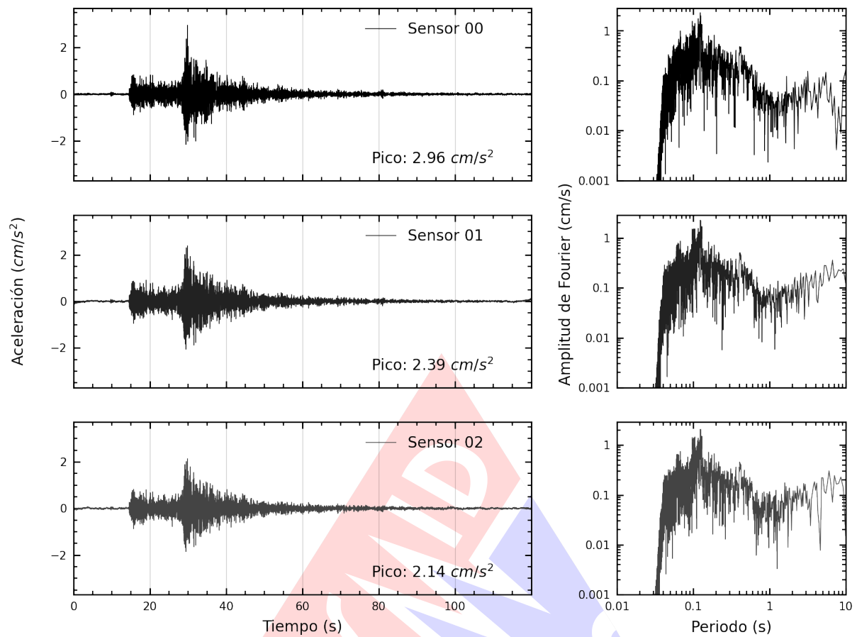
Figura A.3: Registros tiempo-historia y espectros de Fourier en la dirección vertical de la edificación Vivienda. Sismo de Yauyos, Yauyos - Lima del 2024-09-30, 06:36:46 (Hora local)
