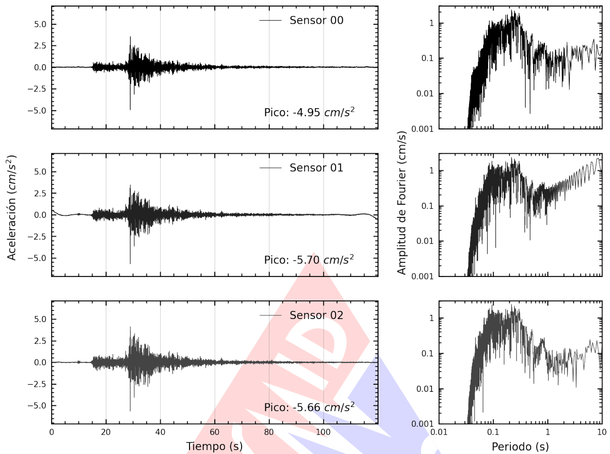
Figura A.1: Registros tiempo-historia y espectros de Fourier en la dirección EW de la edificación Vivienda. Sismo de Yauyos, Yauyos - Lima del 2024-09-30, 06:36:46 (Hora local)
