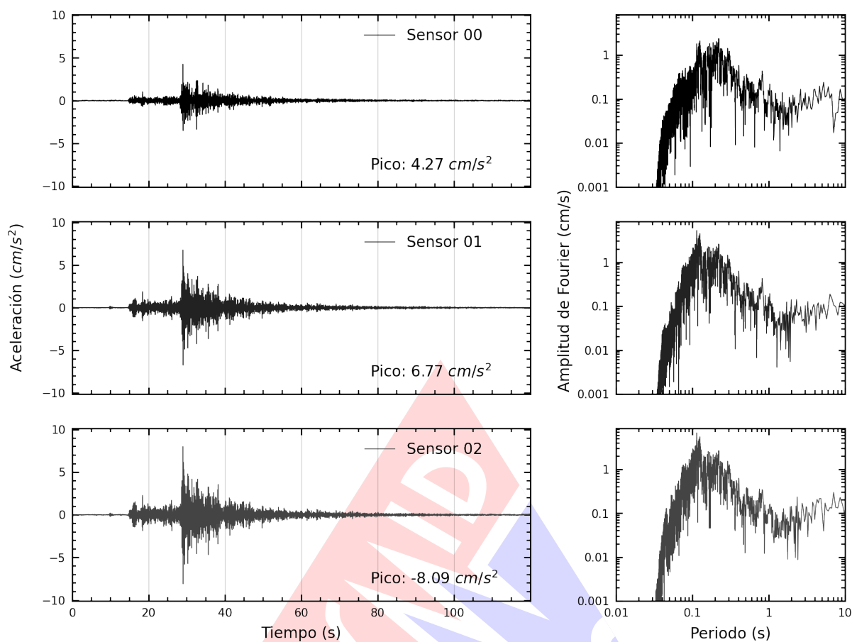
Figura A.2: Registros tiempo-historia y espectros de Fourier en la dirección NS de la edificación Vivienda. Sismo de Yauyos, Yauyos - Lima del 2024-09-30, 06:36:46 (Hora local)
