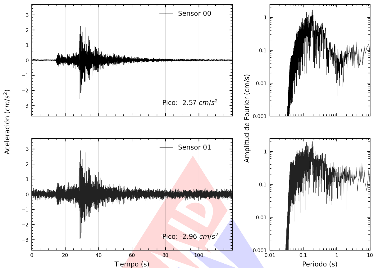
Figura A.2: Registros tiempo-historia y espectros de Fourier en la dirección NS de la edificación Instituto Nacional de Rehabilitación (INR), Chorrillos. Sismo de Yauyos, Yauyos - Lima del 2024-09-30, 06:36:46 (Hora local)
