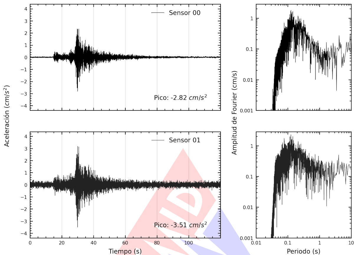
Figura A.1: Registros tiempo-historia y espectros de Fourier en la dirección EW de la edificación Instituto Nacional de Rehabilitación (INR), Chorrillos. Sismo de Yauyos, Yauyos - Lima del 2024-09-30, 06:36:46 (Hora local)
