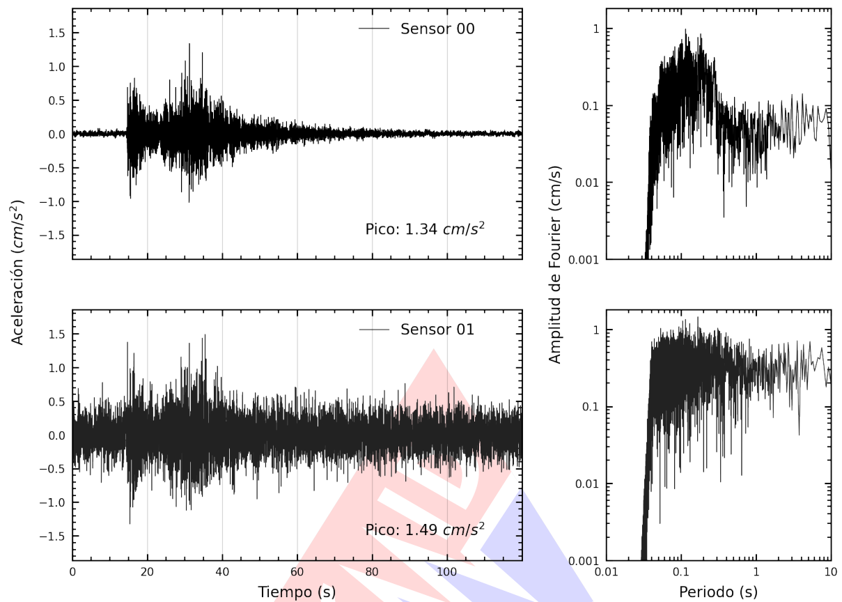
Figura A.3: Registros tiempo-historia y espectros de Fourier en la dirección vertical de la edificación Instituto Nacional de Rehabilitación (INR), Chorrillos. Sismo de Yauyos, Yauyos - Lima del 2024-09-30, 06:36:46 (Hora local)
