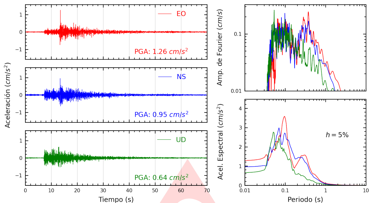
Figura A.1: Registros tiempo-historia, espectros de Fourier y de respuesta en las direcciones EO, NS y vertical de la estación UPAOP. Sismo de Sullana, Sullana - Piura del 2024-10-01, 20:40:28 (Hora local)
