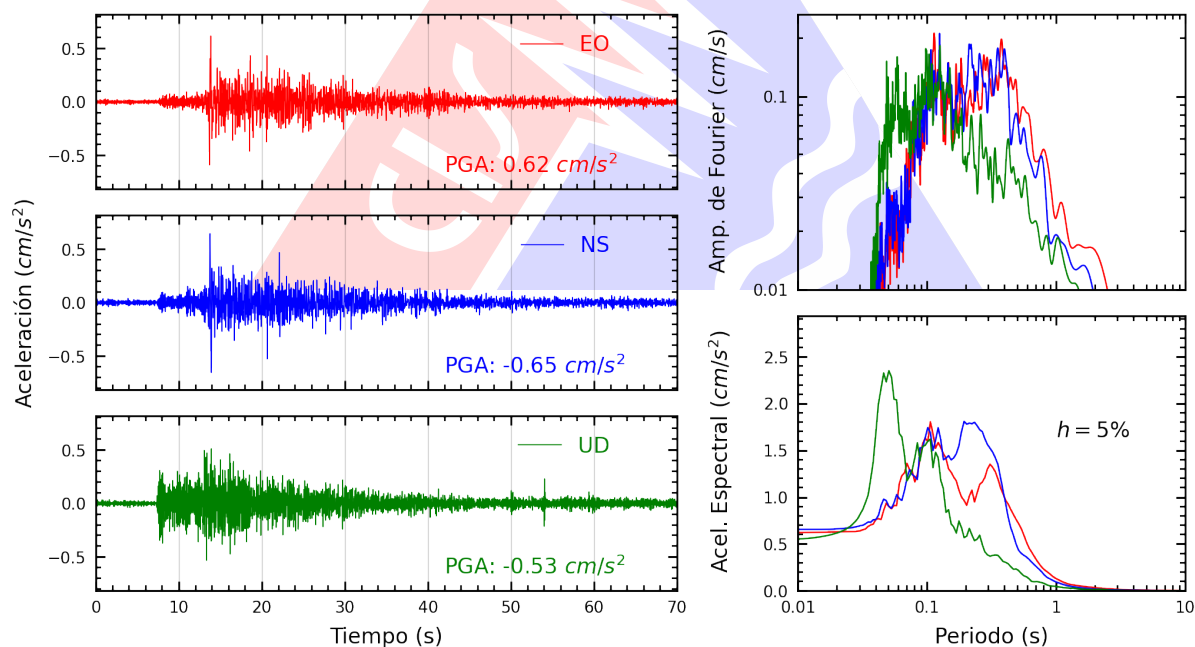
Figura A.2: Registros tiempo-historia, espectros de Fourier y de respuesta en las direcciones EO, NS y vertical de la estación UNP. Sismo de Sullana, Sullana - Piura del 2024-10-01, 20:40:28 (Hora local)
