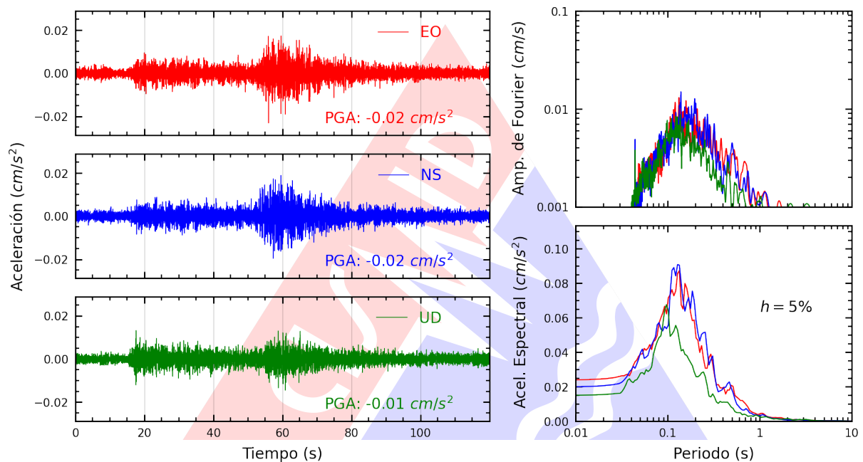
Figura A.3: Registros tiempo-historia, espectros de Fourier y de respuesta en las direcciones EO, NS y vertical de la estación JALV2. Sismo de Tingo Maria, Leoncio Prado - Huanuco del 2024-10-10, 03:39:26 (Hora local)
