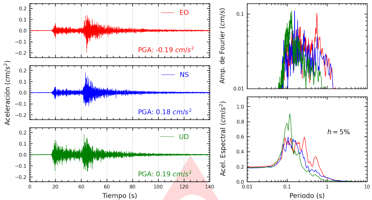
Figura A.1: Registros tiempo-historia, espectros de Fourier y de respuesta en las direcciones EO, NS y vertical de la estación UNIA. Sismo de Tingo Maria, Leoncio Prado - Huanuco del 2024-10-10, 03:39:26 (Hora local)
