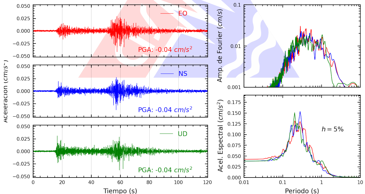
Figura A.2: Registros tiempo-historia, espectros de Fourier y de respuesta en las direcciones EO, NS y vertical de la estación UNCP. Sismo de Tingo Maria, Leoncio Prado - Huanuco del 2024-10-10, 03:39:26 (Hora local)
