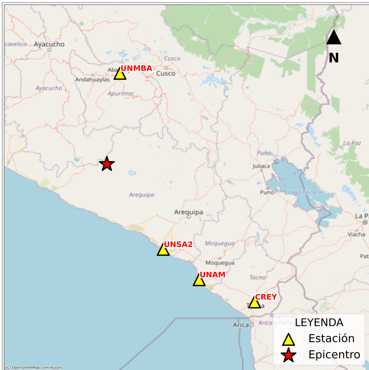
Figura 2: Mapa de ubicación de la(s) estación(es) acelerográfica(s) correspondiente(s) al Sismo de Pausa, Paucar Del Sara Sara - Ayacucho del 12 de octubre de 2024 a las 03:55:00 (hora local)
