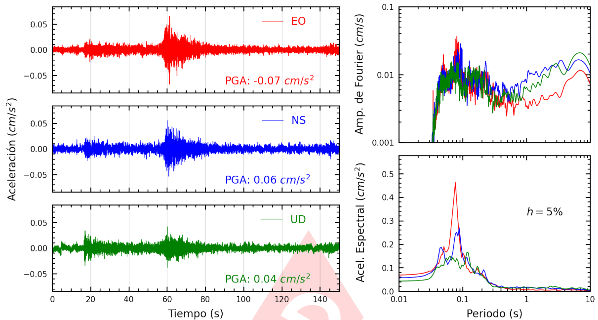
Figura A.3: Registros tiempo-historia, espectros de Fourier y de respuesta en las direcciones EO, NS y vertical de la estación CREY. Sismo de Pausa, Paucar Del Sara Sara - Ayacucho del 2024-10-12, 03:55:00 (Hora local)
