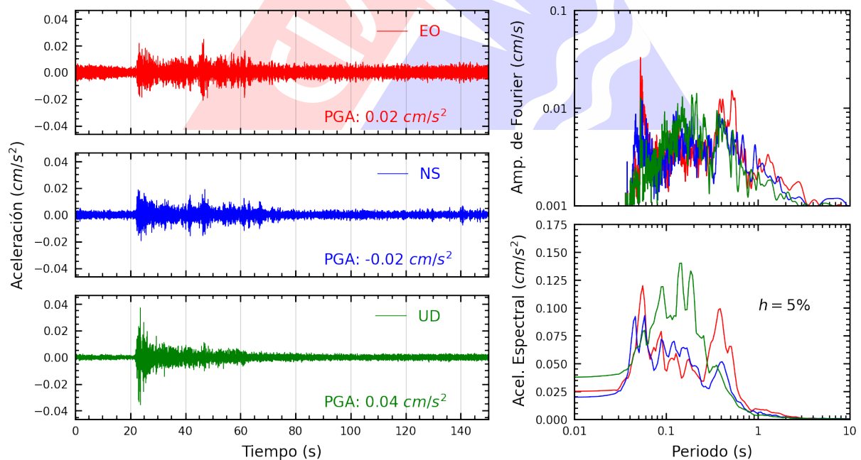
Figura A.4: Registros tiempo-historia, espectros de Fourier y de respuesta en las direcciones EO, NS y vertical de la estación UNMBA. Sismo de Pausa, Paucar Del Sara Sara - Ayacucho del 2024-10-12, 03:55:00 (Hora local)
