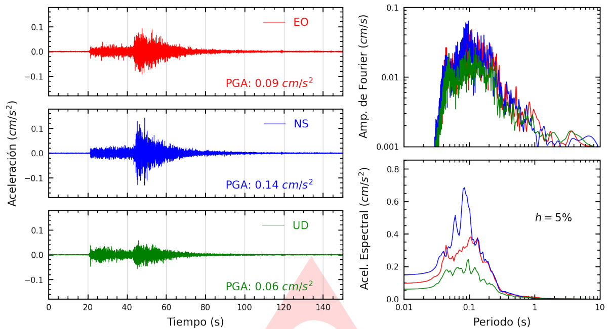
Figura A.1: Registros tiempo-historia, espectros de Fourier y de respuesta en las direcciones EO, NS y vertical de la estación UNSA2. Sismo de Pausa, Paucar Del Sara Sara - Ayacucho del 2024-10-12, 03:55:00 (Hora local)
