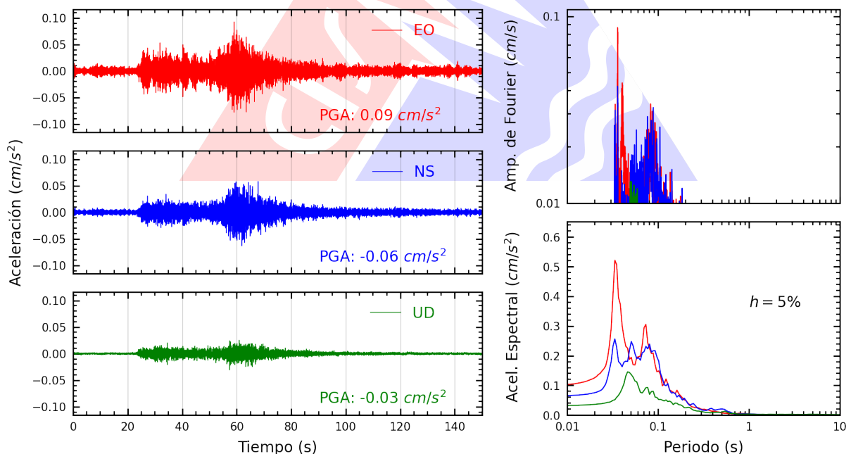
Figura A.2: Registros tiempo-historia, espectros de Fourier y de respuesta en las direcciones EO, NS y vertical de la estación UNAM. Sismo de Pausa, Paucar Del Sara Sara - Ayacucho del 2024-10-12, 03:55:00 (Hora local)
