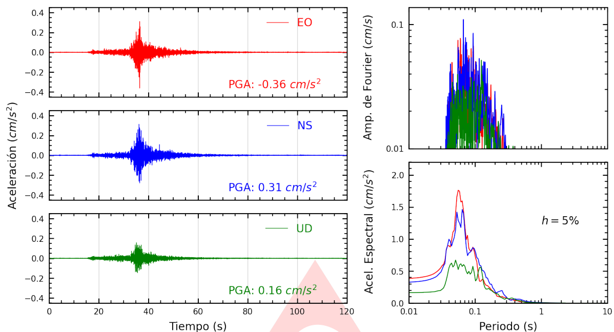
Figura A.1: Registros tiempo-historia, espectros de Fourier y de respuesta en las direcciones EO, NS y vertical de la estación UNSA2. Sismo de Chuquibamba, Condesuyos - Arequipa del 2024-10-12, 19:43:31 (Hora local)
