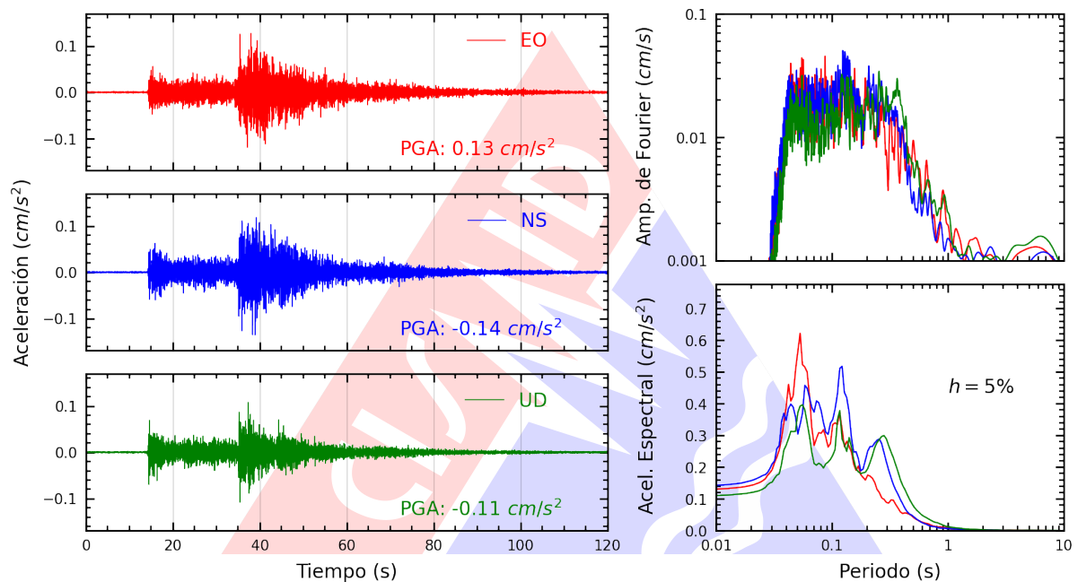
Figura A.7: Registros tiempo-historia, espectros de Fourier y de respuesta en las direcciones EO, NS y vertical de la estación UNSA2. Sismo de Locumba, Jorge Basadre - Tacna del 2024-10-13, 03:50:55 (Hora local)
