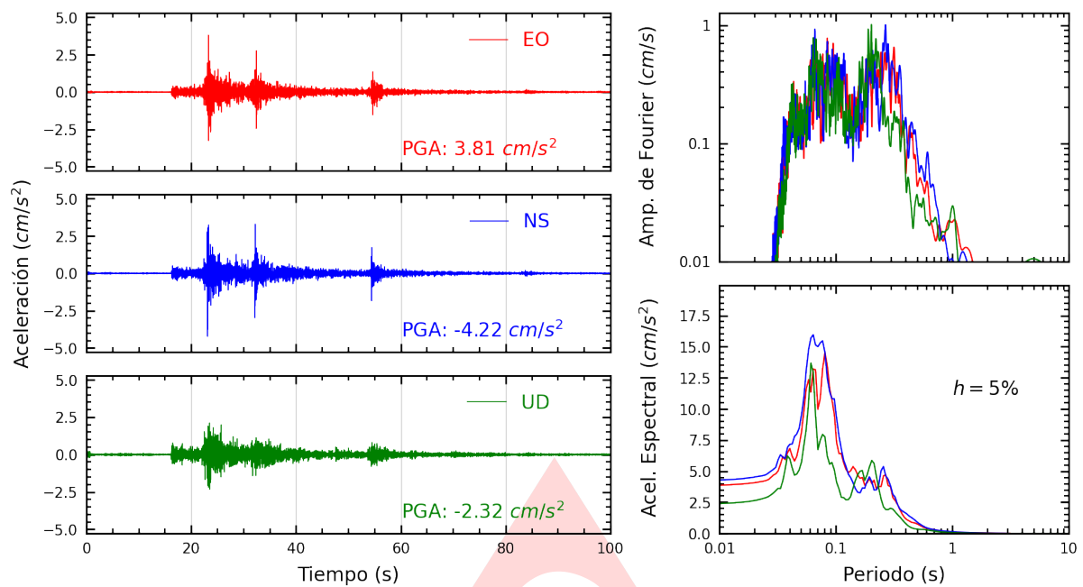
Figura A.1: Registros tiempo-historia, espectros de Fourier y de respuesta en las direcciones EO, NS y vertical de la estación SCTAC. Sismo de Locumba, Jorge Basadre - Tacna del 2024-10-13, 03:50:55 (Hora local)
