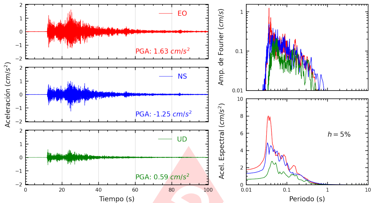
Figura A.5: Registros tiempo-historia, espectros de Fourier y de respuesta en las direcciones EO, NS y vertical de la estación UNAM. Sismo de Locumba, Jorge Basadre - Tacna del 2024-10-13, 03:50:55 (Hora local)
