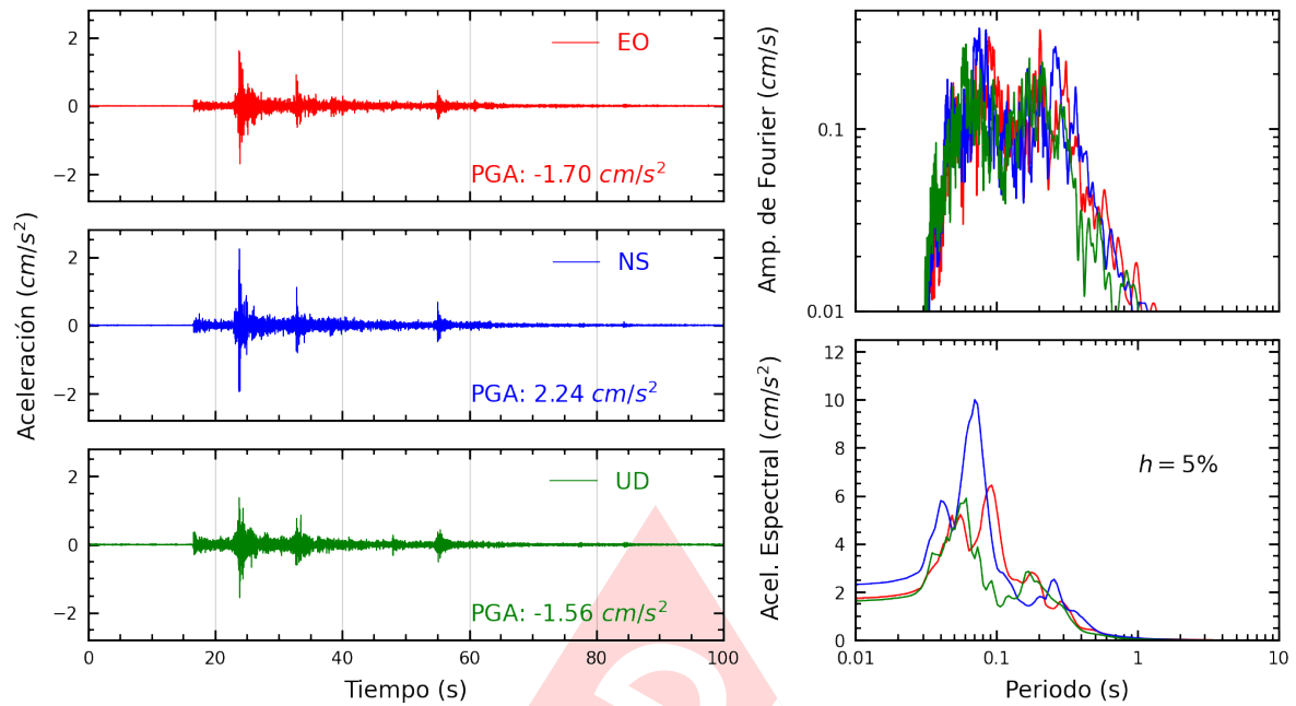
Figura A.3: Registros tiempo-historia, espectros de Fourier y de respuesta en las direcciones EO, NS y vertical de la estación UJBG2. Sismo de Locumba, Jorge Basadre - Tacna del 2024-10-13, 03:50:55 (Hora local)
