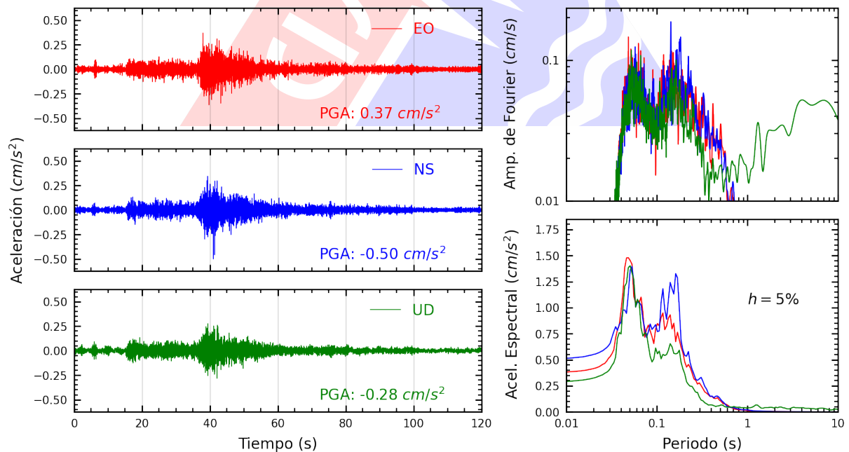
Figura A.6: Registros tiempo-historia, espectros de Fourier y de respuesta en las direcciones EO, NS y vertical de la estación SCARQ. Sismo de Locumba, Jorge Basadre - Tacna del 2024-10-13, 03:50:55 (Hora local)
