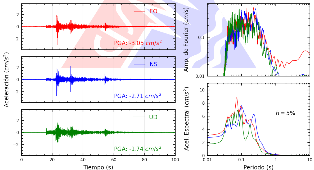
Figura A.2: Registros tiempo-historia, espectros de Fourier y de respuesta en las direcciones EO, NS y vertical de la estación UJBG3. Sismo de Locumba, Jorge Basadre - Tacna del 2024-10-13, 03:50:55 (Hora local)
