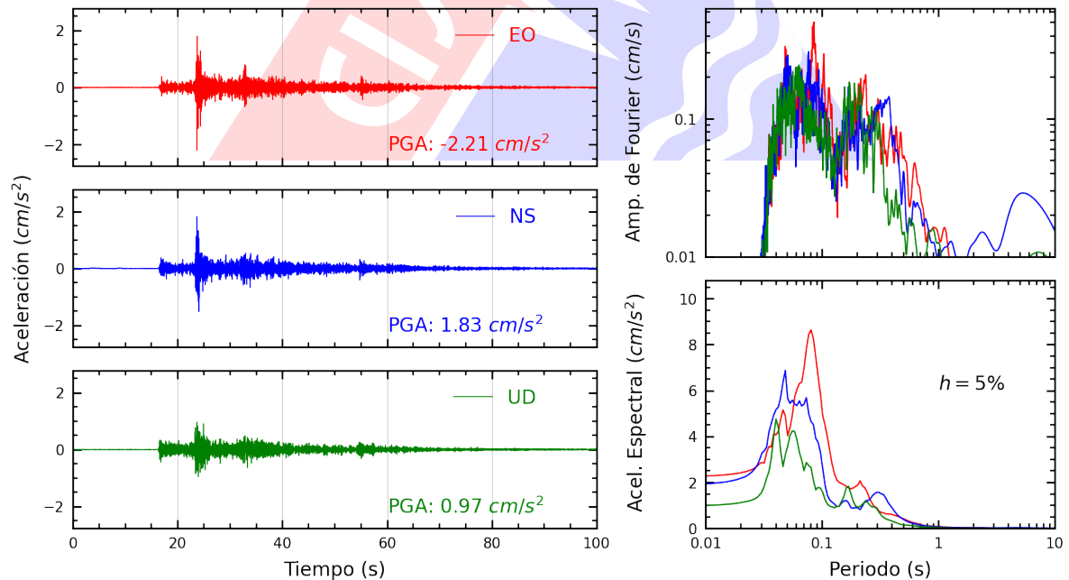
Figura A.4: Registros tiempo-historia, espectros de Fourier y de respuesta en las direcciones EO, NS y vertical de la estación CREY. Sismo de Locumba, Jorge Basadre - Tacna del 2024-10-13, 03:50:55 (Hora local)
