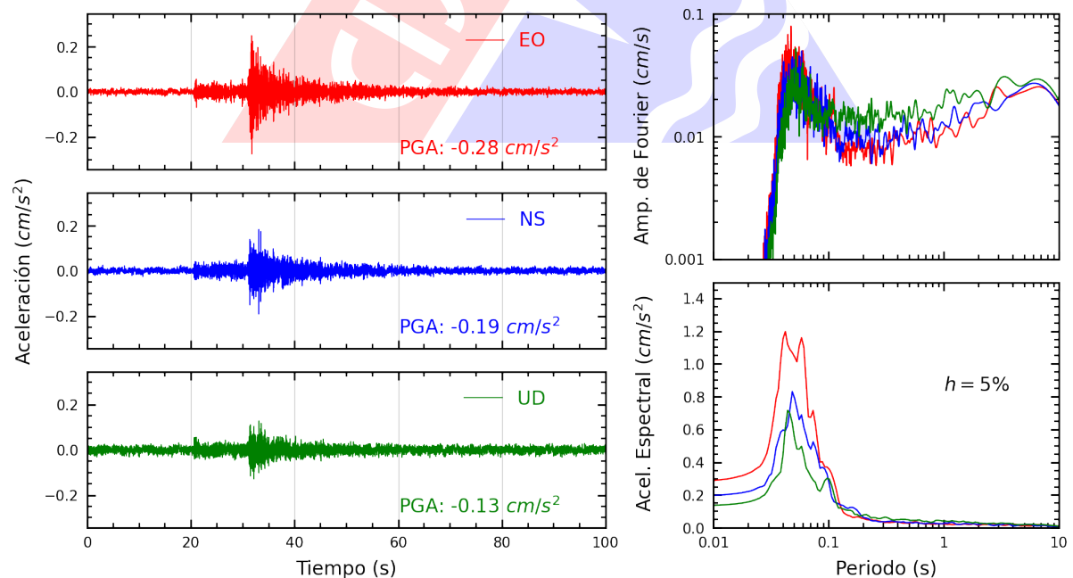
Figura A.16: Registros tiempo-historia, espectros de Fourier y de respuesta en las direcciones EO, NS y vertical de la estación UCSS. Sismo de Mala, Cañete - Lima del 2024-10-15, 02:30:34 (Hora local)
