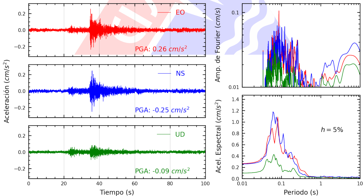
Figura A.18: Registros tiempo-historia, espectros de Fourier y de respuesta en las direcciones EO, NS y vertical de la estación DEFEN. Sismo de Mala, Cañete - Lima del 2024-10-15, 02:30:34 (Hora local)
