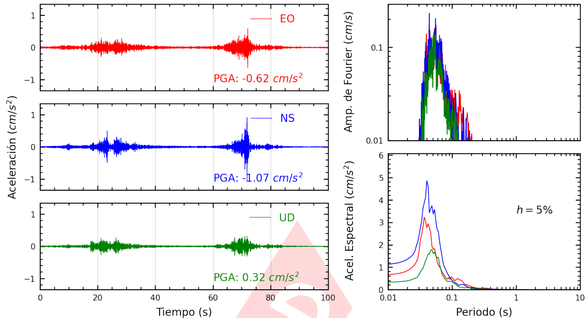
Figura A.3: Registros tiempo-historia, espectros de Fourier y de respuesta en las direcciones EO, NS y vertical de la estación PACHA. Sismo de Mala, Cañete - Lima del 2024-10-15, 02:30:34 (Hora local)
