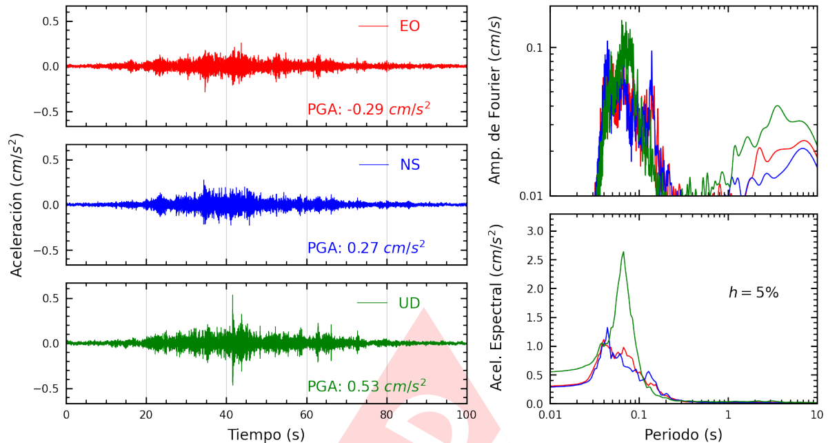
Figura A.5: Registros tiempo-historia, espectros de Fourier y de respuesta en las direcciones EO, NS y vertical de la estación CARAB. Sismo de Mala, Cañete - Lima del 2024-10-15, 02:30:34 (Hora local)
