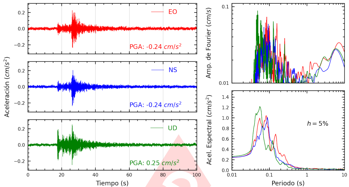
Figura A.19: Registros tiempo-historia, espectros de Fourier y de respuesta en las direcciones EO, NS y vertical de la estación USILP. Sismo de Mala, Cañete - Lima del 2024-10-15, 02:30:34 (Hora local)
