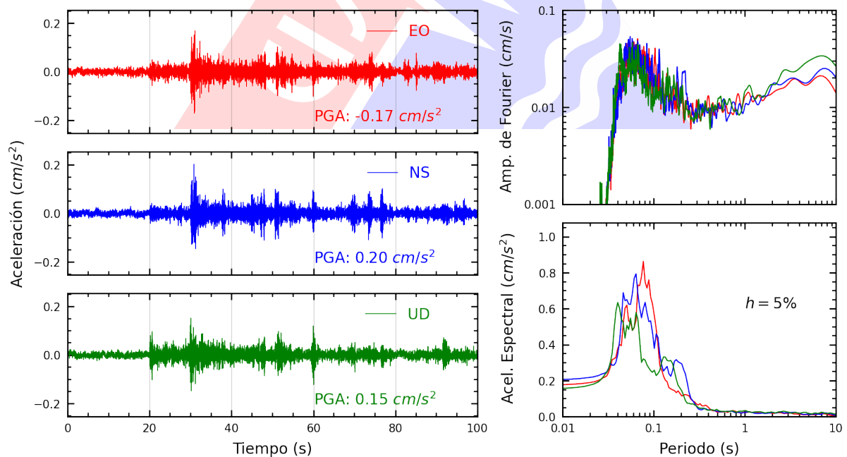
Figura A.22: Registros tiempo-historia, espectros de Fourier y de respuesta en las direcciones EO, NS y vertical de la estación UPCSM. Sismo de Mala, Cañete - Lima del 2024-10-15, 02:30:34 (Hora local)
