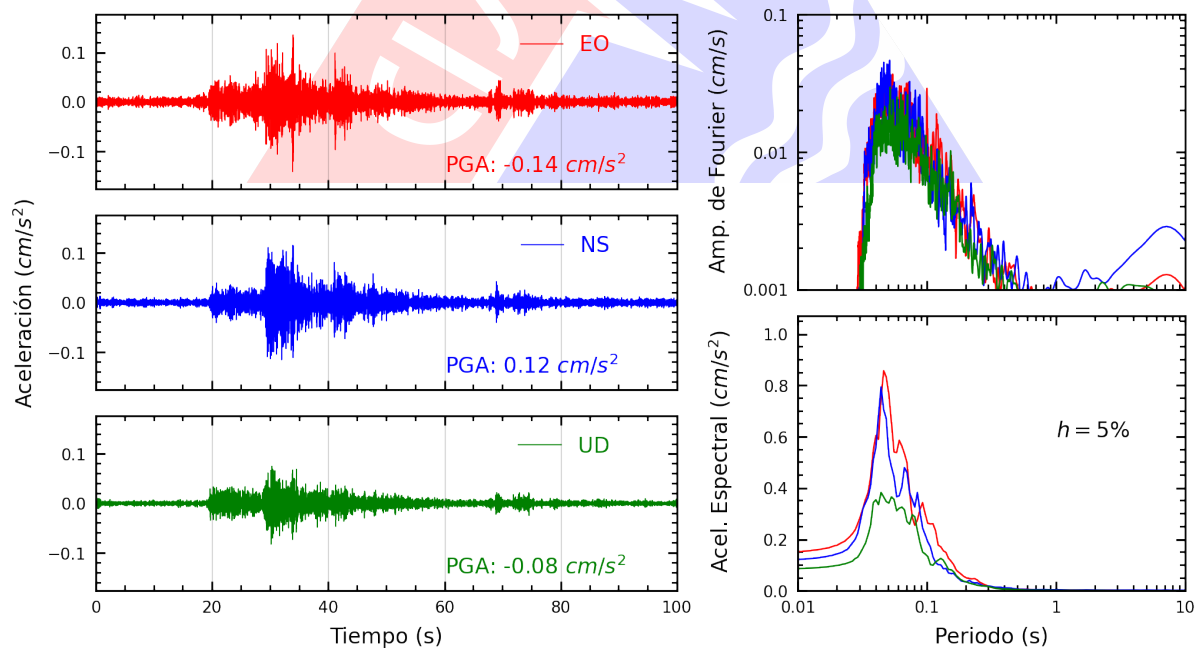
Figura A.26: Registros tiempo-historia, espectros de Fourier y de respuesta en las direcciones EO, NS y vertical de la estación BORJA. Sismo de Mala, Cañete - Lima del 2024-10-15, 02:30:34 (Hora local)
