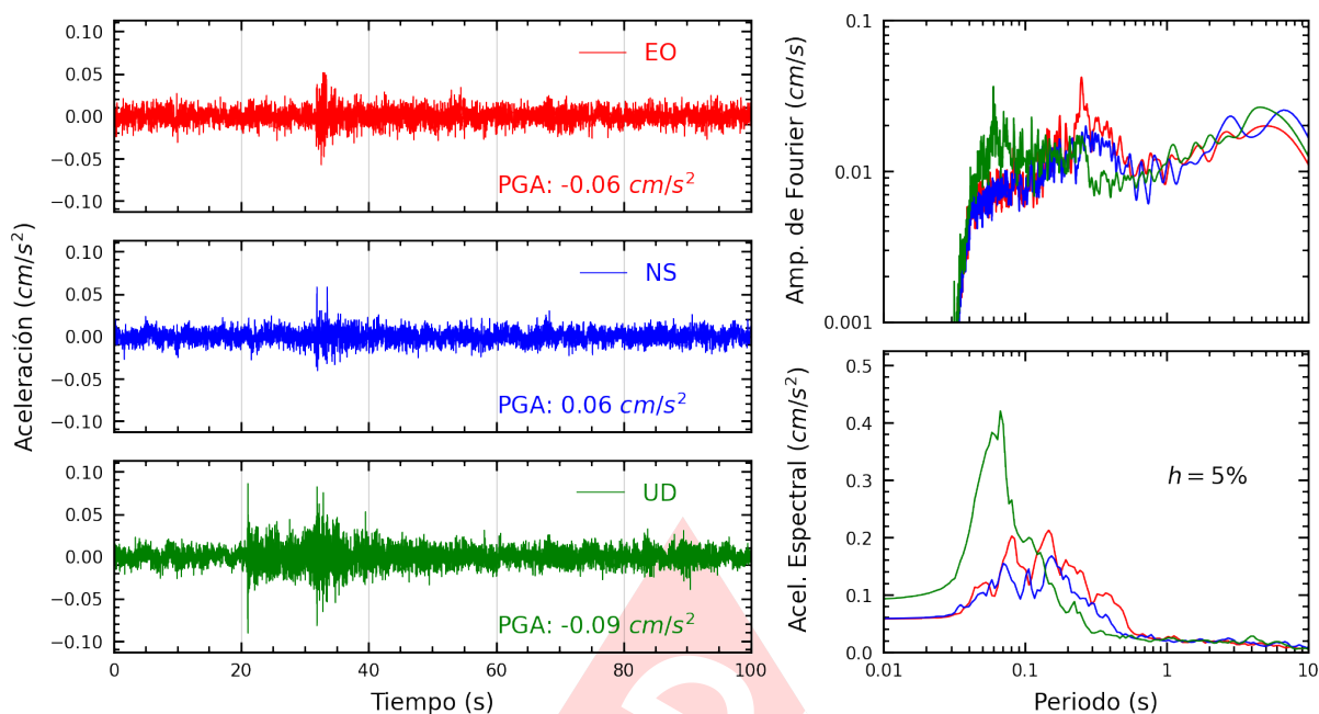
Figura A.33: Registros tiempo-historia, espectros de Fourier y de respuesta en las direcciones EO, NS y vertical de la estación ACAPU. Sismo de Mala, Cañete - Lima del 2024-10-15, 02:30:34 (Hora local)
