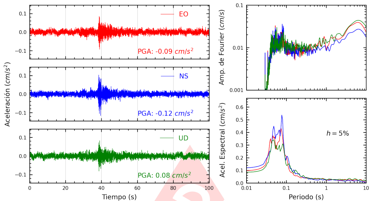
Figura A.29: Registros tiempo-historia, espectros de Fourier y de respuesta en las direcciones EO, NS y vertical de la estación UNMSM. Sismo de Mala, Cañete - Lima del 2024-10-15, 02:30:34 (Hora local)
