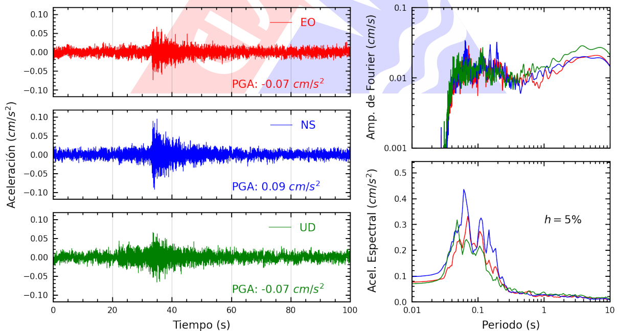
Figura A.32: Registros tiempo-historia, espectros de Fourier y de respuesta en las direcciones EO, NS y vertical de la estación VHAYA. Sismo de Mala, Cañete - Lima del 2024-10-15, 02:30:34 (Hora local)
