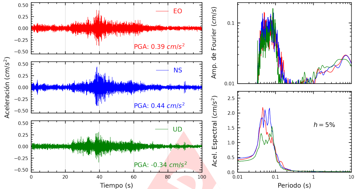
Figura A.7: Registros tiempo-historia, espectros de Fourier y de respuesta en las direcciones EO, NS y vertical de la estación SROSA. Sismo de Mala, Cañete - Lima del 2024-10-15, 02:30:34 (Hora local)
