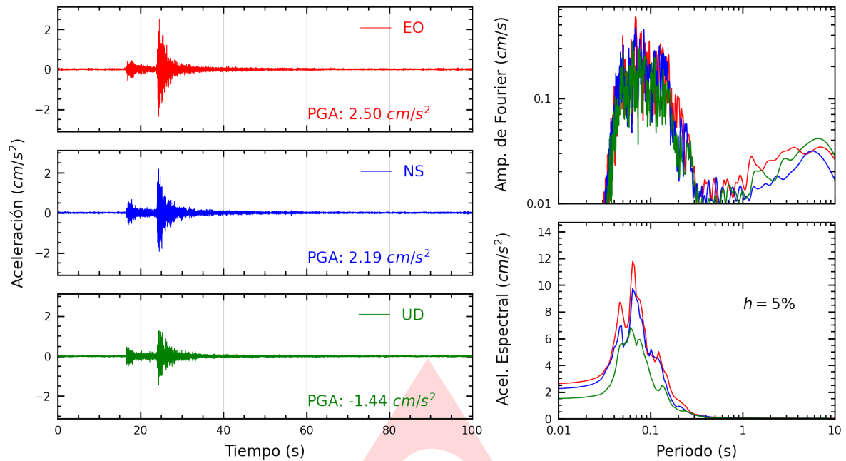
Figura A.1: Registros tiempo-historia, espectros de Fourier y de respuesta en las direcciones EO, NS y vertical de la estación PHERM. Sismo de Mala, Cañete - Lima del 2024-10-15, 02:30:34 (Hora local)
