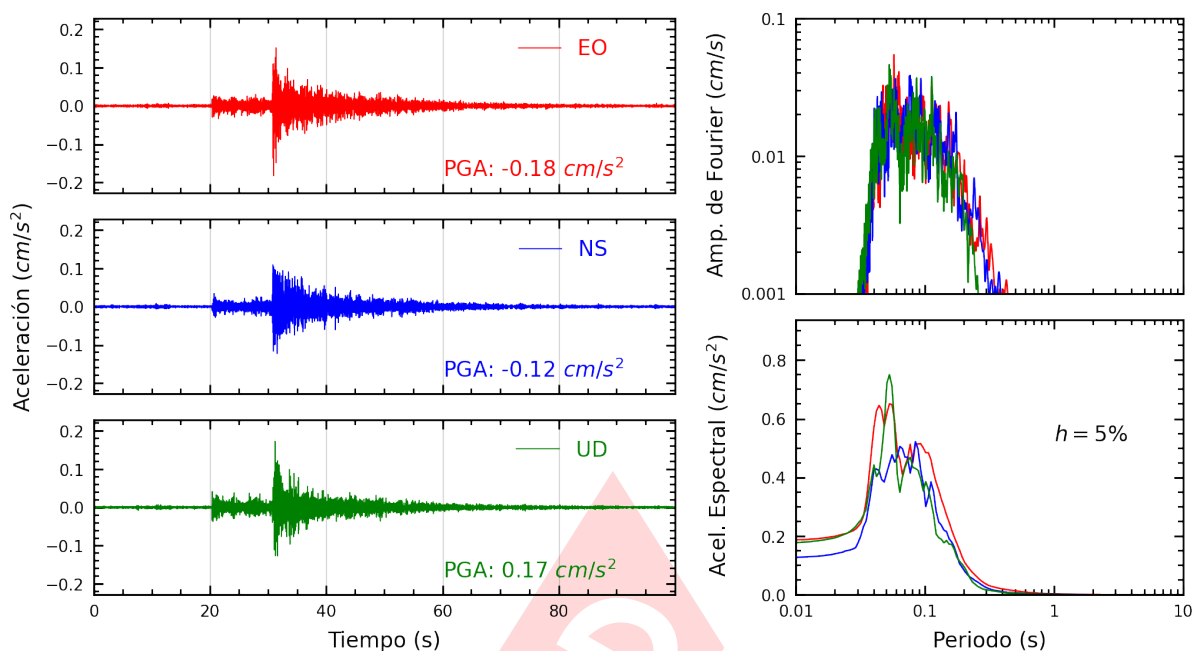
Figura A.23: Registros tiempo-historia, espectros de Fourier y de respuesta en las direcciones EO, NS y vertical de la estación JALV2. Sismo de Mala, Cañete - Lima del 2024-10-15, 02:30:34 (Hora local)
