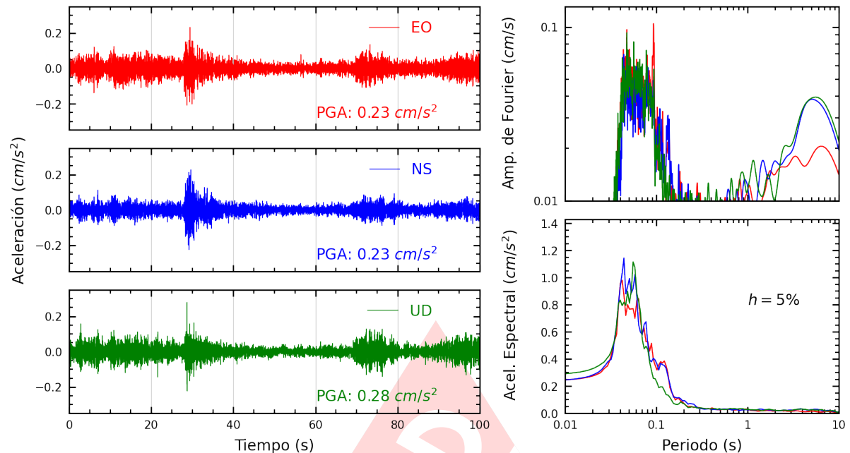
Figura A.15: Registros tiempo-historia, espectros de Fourier y de respuesta en las direcciones EO, NS y vertical de la estación URPE. Sismo de Mala, Cañete - Lima del 2024-10-15, 02:30:34 (Hora local)
