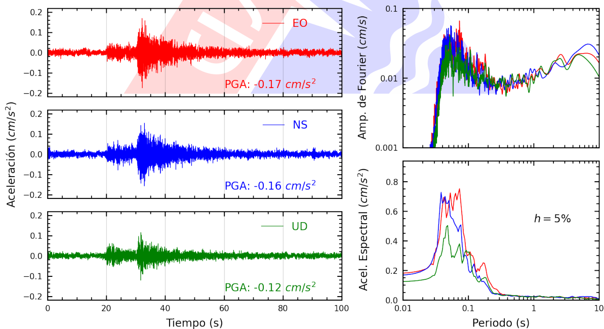
Figura A.24: Registros tiempo-historia, espectros de Fourier y de respuesta en las direcciones EO, NS y vertical de la estación FICPE. Sismo de Mala, Cañete - Lima del 2024-10-15, 02:30:34 (Hora local)
