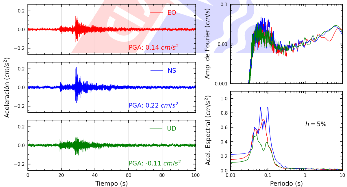
Figura A.20: Registros tiempo-historia, espectros de Fourier y de respuesta en las direcciones EO, NS y vertical de la estación SERVI. Sismo de Mala, Cañete - Lima del 2024-10-15, 02:30:34 (Hora local)
