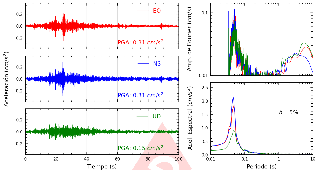
Figura A.13: Registros tiempo-historia, espectros de Fourier y de respuesta en las direcciones EO, NS y vertical de la estación USMP. Sismo de Mala, Cañete - Lima del 2024-10-15, 02:30:34 (Hora local)
