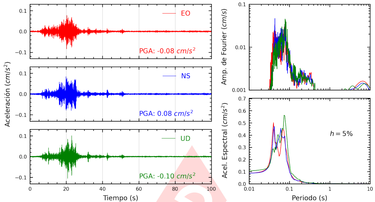
Figura A.31: Registros tiempo-historia, espectros de Fourier y de respuesta en las direcciones EO, NS y vertical de la estación SCAYA. Sismo de Mala, Cañete - Lima del 2024-10-15, 02:30:34 (Hora local)
