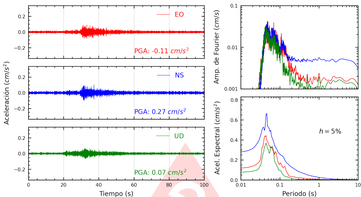
Figura A.17: Registros tiempo-historia, espectros de Fourier y de respuesta en las direcciones EO, NS y vertical de la estación ATARJ. Sismo de Mala, Cañete - Lima del 2024-10-15, 02:30:34 (Hora local)
