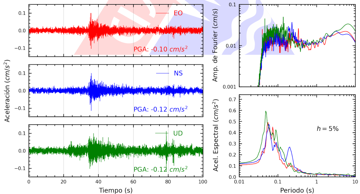
Figura A.28: Registros tiempo-historia, espectros de Fourier y de respuesta en las direcciones EO, NS y vertical de la estación MDPP. Sismo de Mala, Cañete - Lima del 2024-10-15, 02:30:34 (Hora local)
