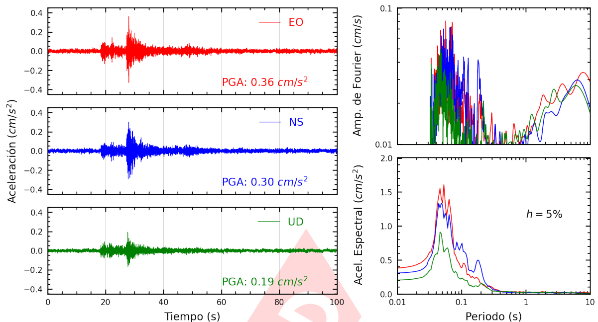
Figura A.9: Registros tiempo-historia, espectros de Fourier y de respuesta en las direcciones EO, NS y vertical de la estación UPCVI. Sismo de Mala, Cañete - Lima del 2024-10-15, 02:30:34 (Hora local)
