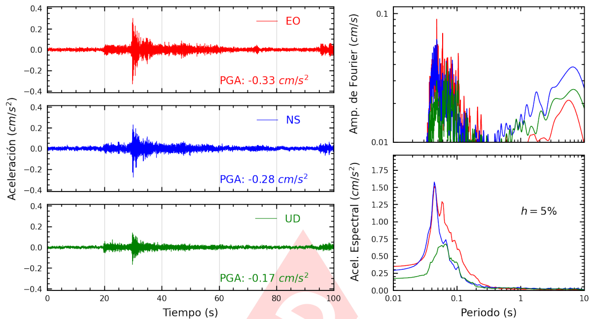
Figura A.11: Registros tiempo-historia, espectros de Fourier y de respuesta en las direcciones EO, NS y vertical de la estación CEPRE. Sismo de Mala, Cañete - Lima del 2024-10-15, 02:30:34 (Hora local)
