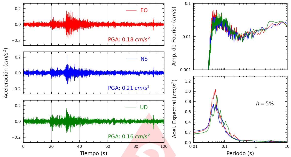
Figura A.21: Registros tiempo-historia, espectros de Fourier y de respuesta en las direcciones EO, NS y vertical de la estación UCVAT. Sismo de Mala, Cañete - Lima del 2024-10-15, 02:30:34 (Hora local)
