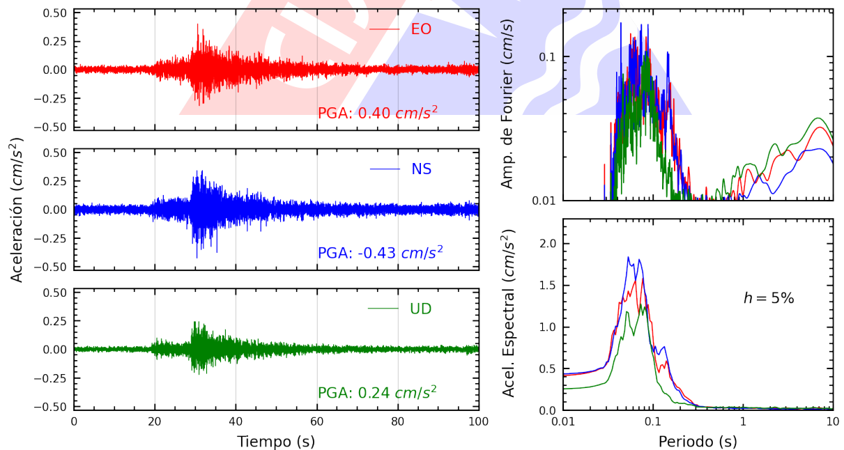
Figura A.8: Registros tiempo-historia, espectros de Fourier y de respuesta en las direcciones EO, NS y vertical de la estación USILM. Sismo de Mala, Cañete - Lima del 2024-10-15, 02:30:34 (Hora local)
