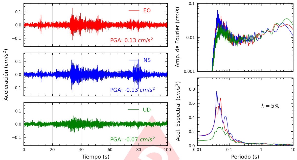
Figura A.27: Registros tiempo-historia, espectros de Fourier y de respuesta en las direcciones EO, NS y vertical de la estación COMAS. Sismo de Mala, Cañete - Lima del 2024-10-15, 02:30:34 (Hora local)
