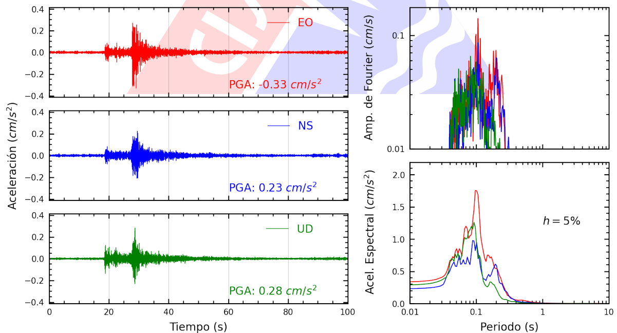
Figura A.12: Registros tiempo-historia, espectros de Fourier y de respuesta en las direcciones EO, NS y vertical de la estación SCCHO. Sismo de Mala, Cañete - Lima del 2024-10-15, 02:30:34 (Hora local)
