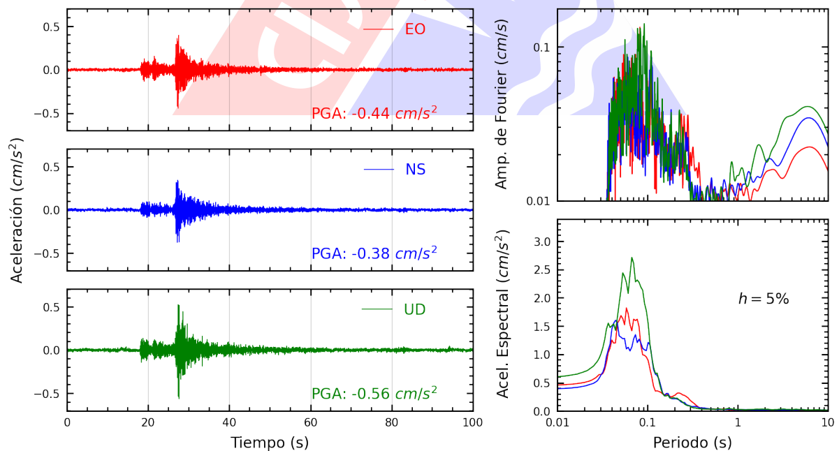
Figura A.4: Registros tiempo-historia, espectros de Fourier y de respuesta en las direcciones EO, NS y vertical de la estación SOVES. Sismo de Mala, Cañete - Lima del 2024-10-15, 02:30:34 (Hora local)
