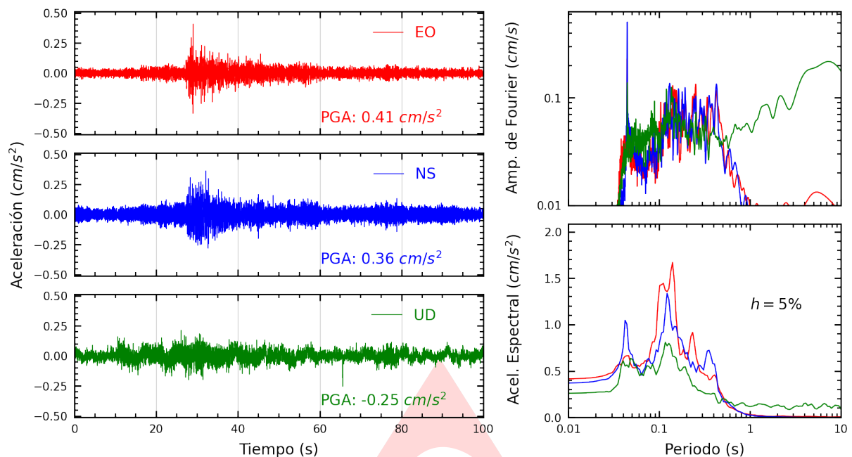
Figura A.1: Registros tiempo-historia, espectros de Fourier y de respuesta en las direcciones EO, NS y vertical de la estación SCPIU. Sismo de Zorritos, Contralmirante Villar - Tumbes del 2024-10-15, 09:13:55 (Hora local)
