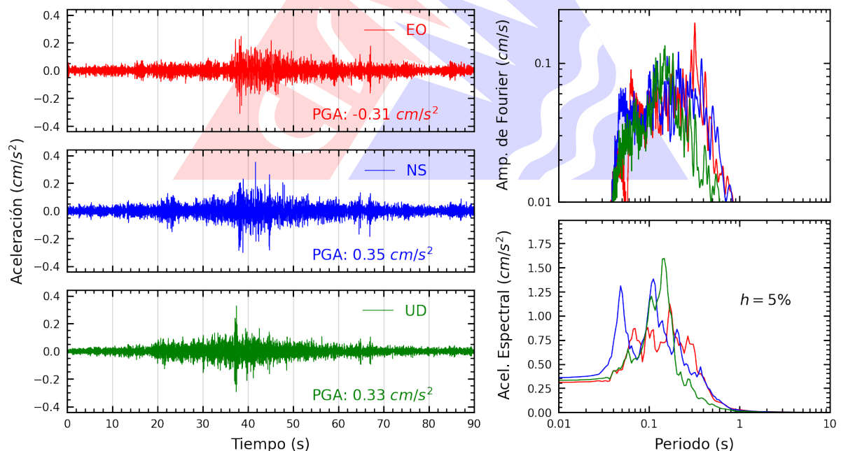
Figura A.2: Registros tiempo-historia, espectros de Fourier y de respuesta en las direcciones EO, NS y vertical de la estación UPAOP. Sismo de Zorritos, Contralmirante Villar - Tumbes del 2024-10-15, 09:13:55 (Hora local)
