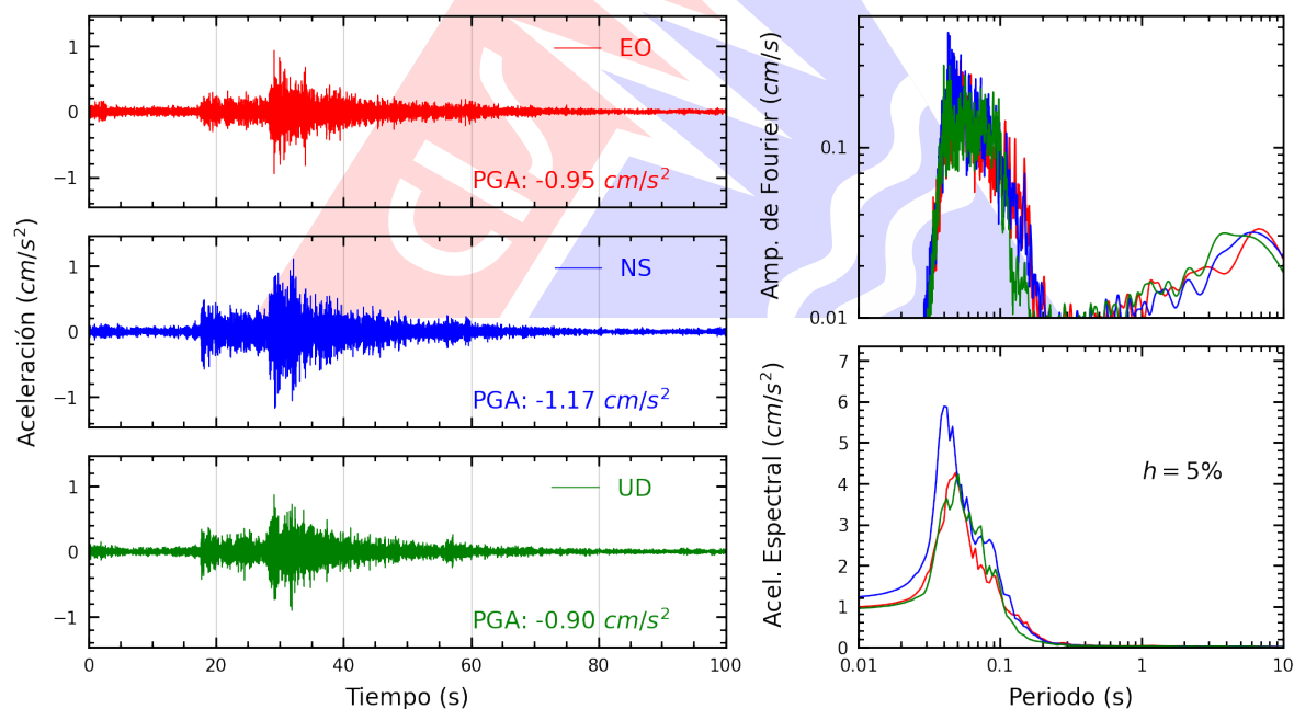
Figura A.2: Registros tiempo-historia, espectros de Fourier y de respuesta en las direcciones EO, NS y vertical de la estación SROSA. Sismo de Huacho, Huaura - Lima del 2024-10-18, 02:09:02 (Hora local)
