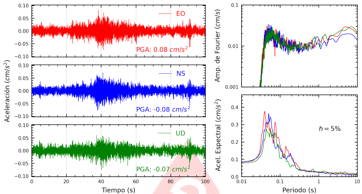
Figura A.27: Registros tiempo-historia, espectros de Fourier y de respuesta en las direcciones EO, NS y vertical de la estación IMCA. Sismo de Huacho, Huaura - Lima del 2024-10-18, 02:09:02 (Hora local)
