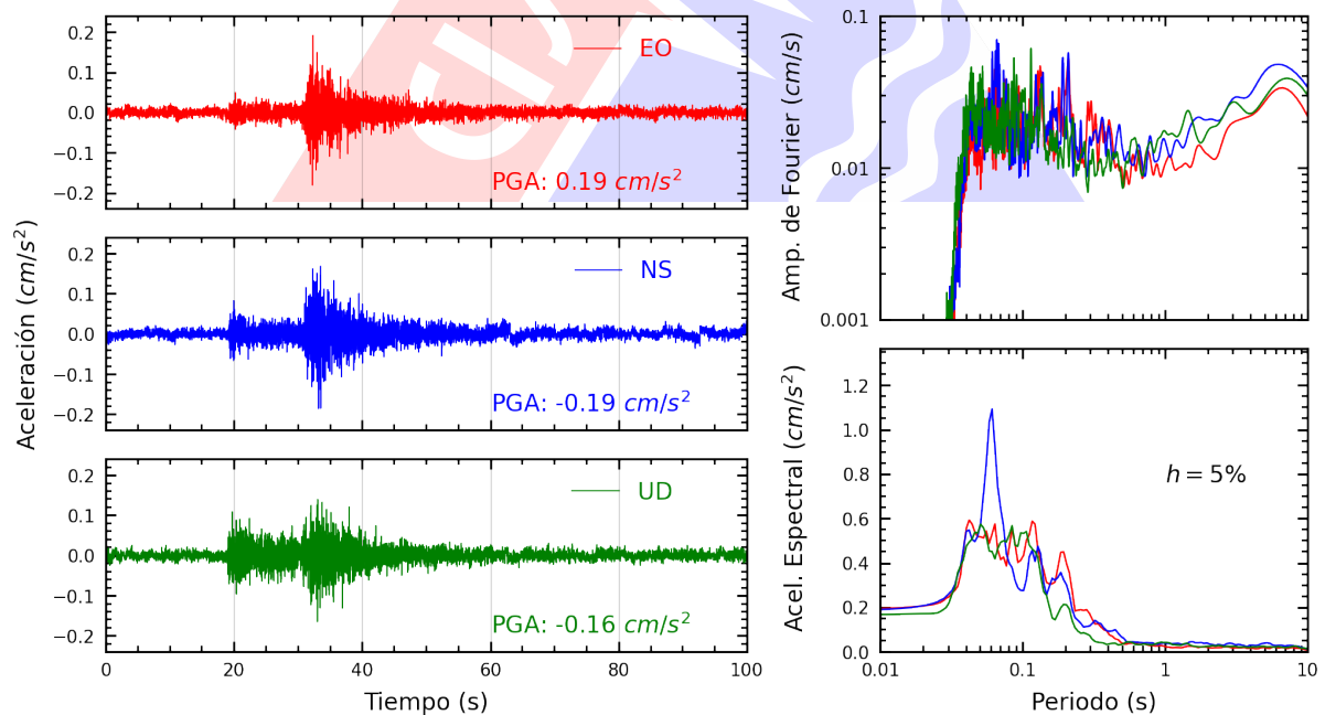
Figura A.14: Registros tiempo-historia, espectros de Fourier y de respuesta en las direcciones EO, NS y vertical de la estación VHAYA. Sismo de Huacho, Huaura - Lima del 2024-10-18, 02:09:02 (Hora local)
