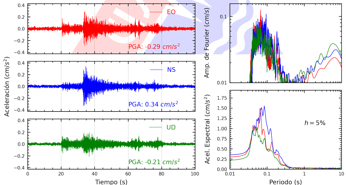
Figura A.10: Registros tiempo-historia, espectros de Fourier y de respuesta en las direcciones EO, NS y vertical de la estación INDEP. Sismo de Huacho, Huaura - Lima del 2024-10-18, 02:09:02 (Hora local)
