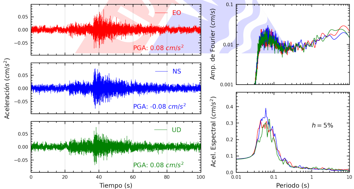
Figura A.28: Registros tiempo-historia, espectros de Fourier y de respuesta en las direcciones EO, NS y vertical de la estación SERVI. Sismo de Huacho, Huaura - Lima del 2024-10-18, 02:09:02 (Hora local)
