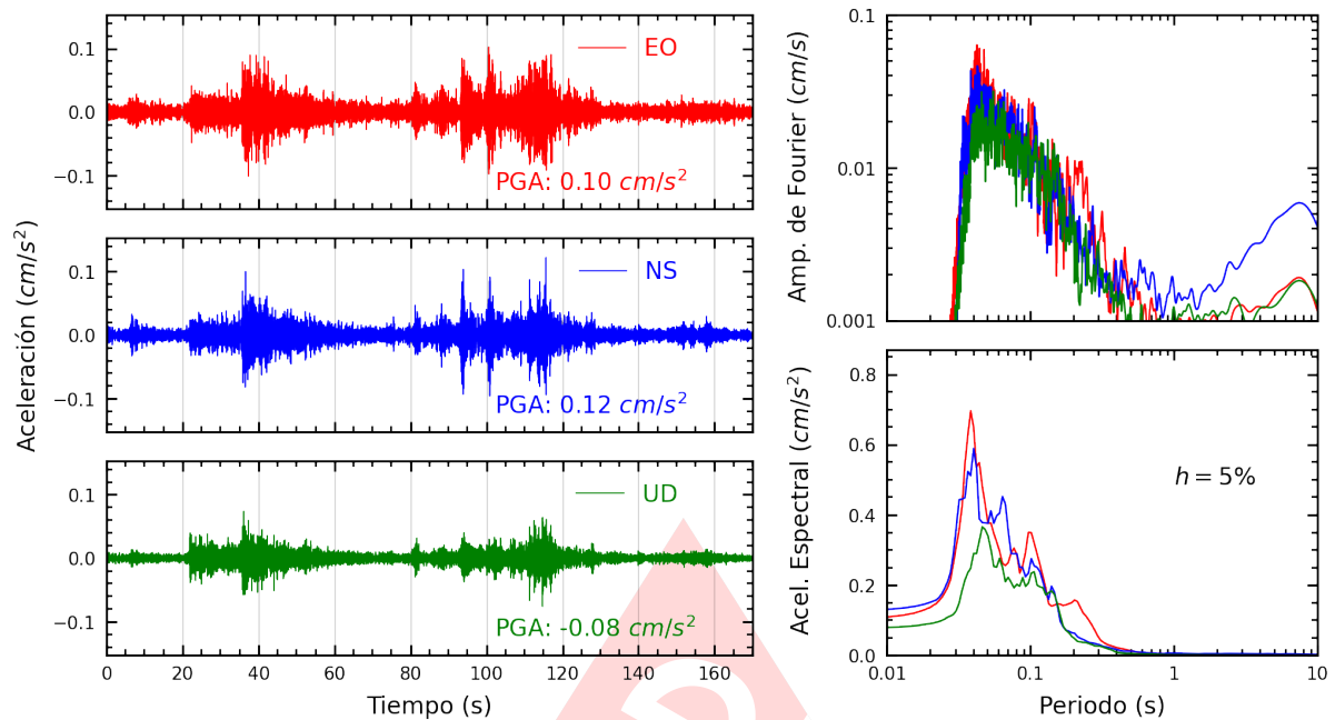
Figura A.21: Registros tiempo-historia, espectros de Fourier y de respuesta en las direcciones EO, NS y vertical de la estación BORJA. Sismo de Huacho, Huaura - Lima del 2024-10-18, 02:09:02 (Hora local)
