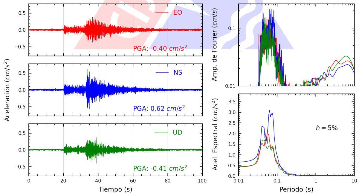
Figura A.4: Registros tiempo-historia, espectros de Fourier y de respuesta en las direcciones EO, NS y vertical de la estación JOSEO. Sismo de Huacho, Huaura - Lima del 2024-10-18, 02:09:02 (Hora local)
