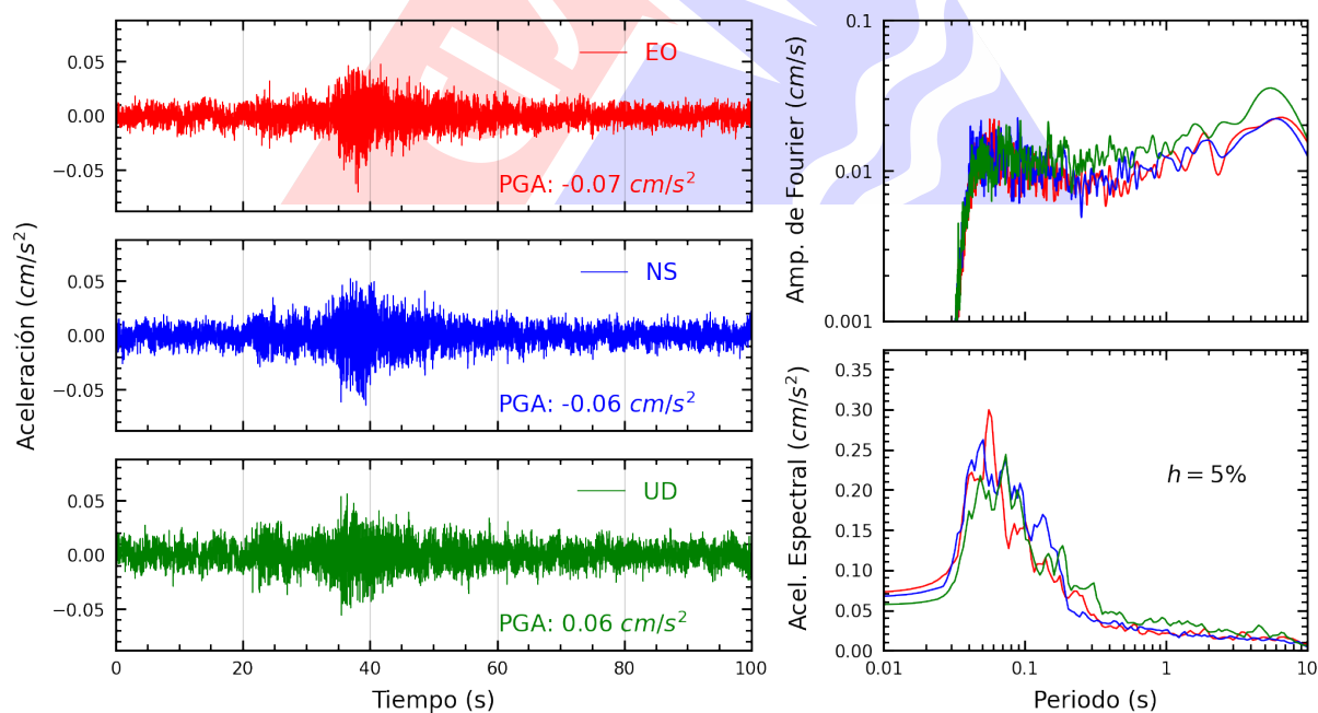
Figura A.30: Registros tiempo-historia, espectros de Fourier y de respuesta en las direcciones EO, NS y vertical de la estación UNFV. Sismo de Huacho, Huaura - Lima del 2024-10-18, 02:09:02 (Hora local)
