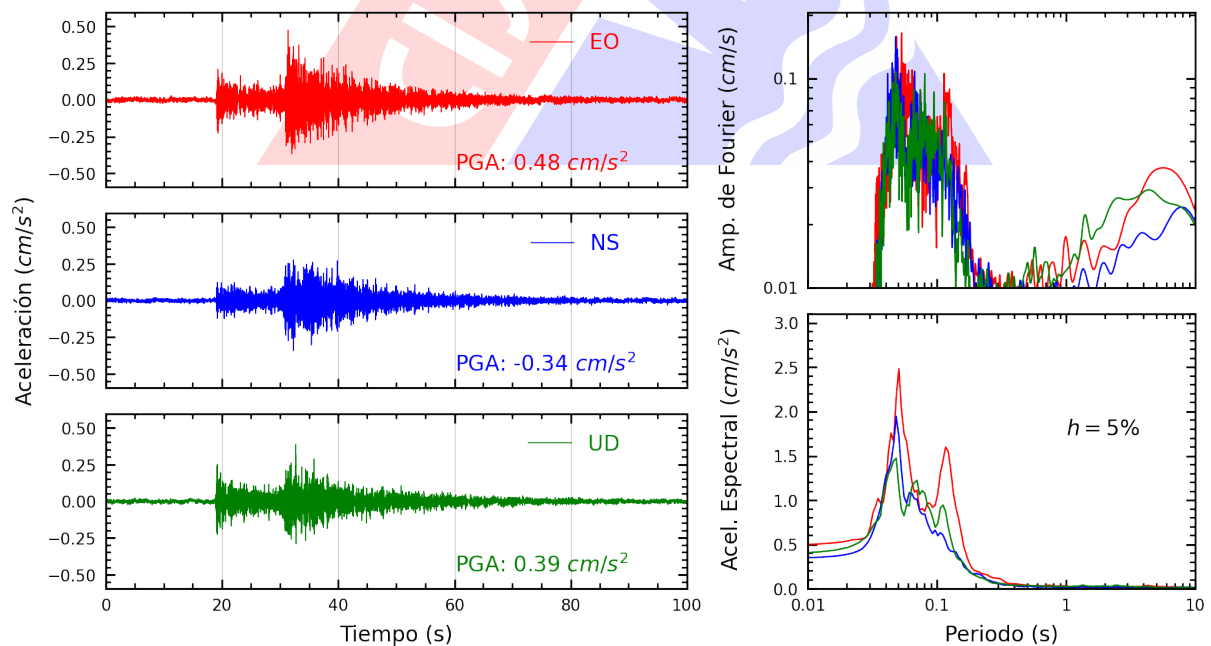
Figura A.6: Registros tiempo-historia, espectros de Fourier y de respuesta en las direcciones EO, NS y vertical de la estación AMORE. Sismo de Huacho, Huaura - Lima del 2024-10-18, 02:09:02 (Hora local)
