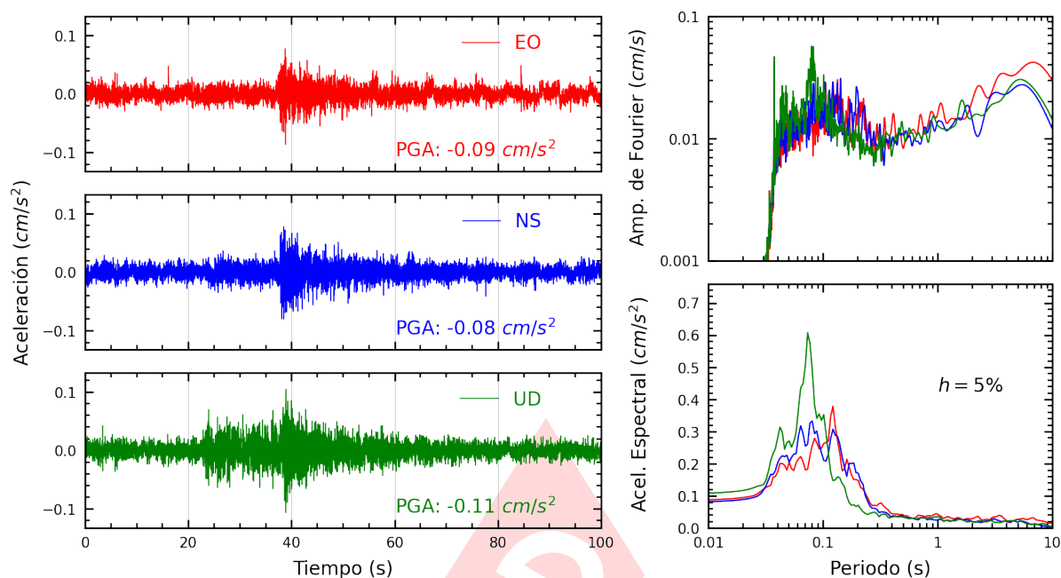
Figura A.25: Registros tiempo-historia, espectros de Fourier y de respuesta en las direcciones EO, NS y vertical de la estación SOCHO. Sismo de Huacho, Huaura - Lima del 2024-10-18, 02:09:02 (Hora local)
