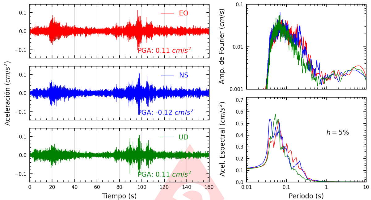
Figura A.23: Registros tiempo-historia, espectros de Fourier y de respuesta en las direcciones EO, NS y vertical de la estación SCCHO. Sismo de Huacho, Huaura - Lima del 2024-10-18, 02:09:02 (Hora local)
