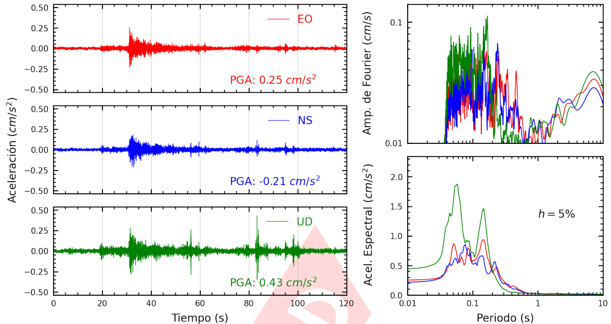
Figura A.7: Registros tiempo-historia, espectros de Fourier y de respuesta en las direcciones EO, NS y vertical de la estación MDPP. Sismo de Huacho, Huaura - Lima del 2024-10-18, 02:09:02 (Hora local)
