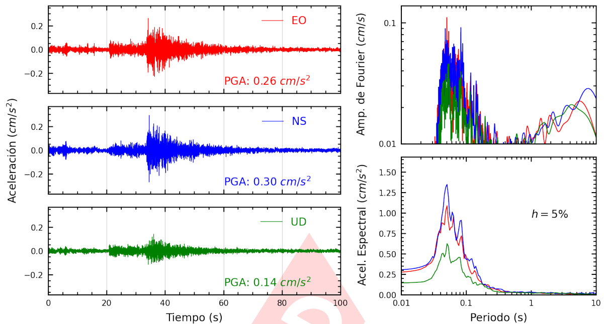
Figura A.11: Registros tiempo-historia, espectros de Fourier y de respuesta en las direcciones EO, NS y vertical de la estación FICPE. Sismo de Huacho, Huaura - Lima del 2024-10-18, 02:09:02 (Hora local)
