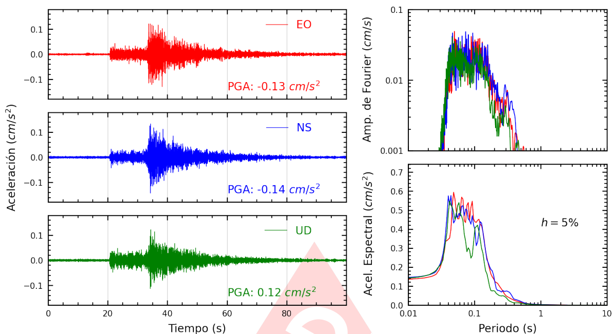
Figura A.19: Registros tiempo-historia, espectros de Fourier y de respuesta en las direcciones EO, NS y vertical de la estación JALV2. Sismo de Huacho, Huaura - Lima del 2024-10-18, 02:09:02 (Hora local)
