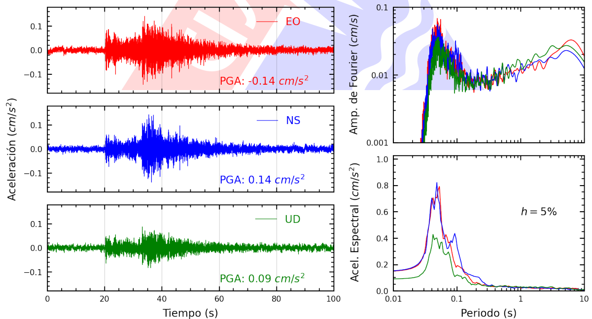
Figura A.18: Registros tiempo-historia, espectros de Fourier y de respuesta en las direcciones EO, NS y vertical de la estación UCSS. Sismo de Huacho, Huaura - Lima del 2024-10-18, 02:09:02 (Hora local)
