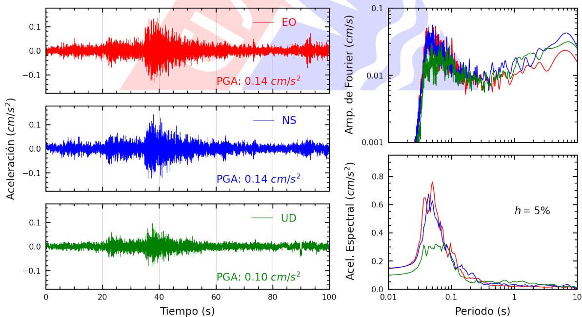
Figura A.20: Registros tiempo-historia, espectros de Fourier y de respuesta en las direcciones EO, NS y vertical de la estación CEPRE. Sismo de Huacho, Huaura - Lima del 2024-10-18, 02:09:02 (Hora local)
