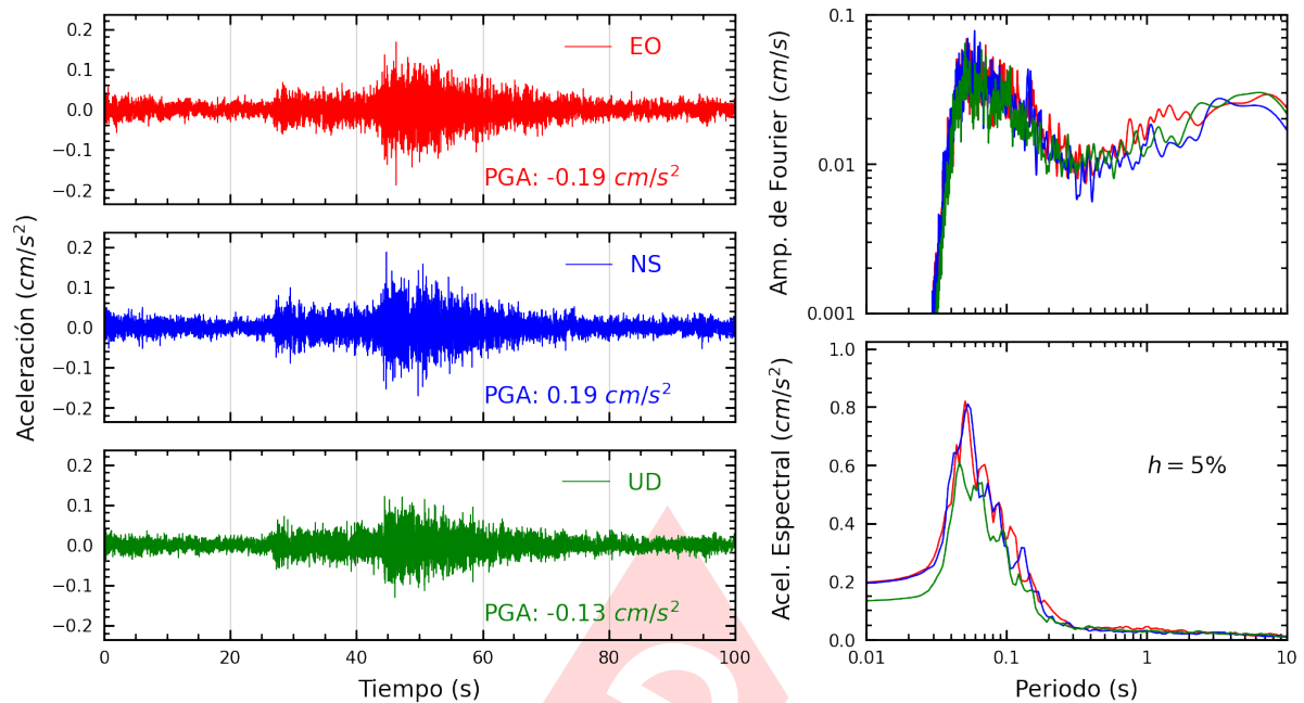
Figura A.15: Registros tiempo-historia, espectros de Fourier y de respuesta en las direcciones EO, NS y vertical de la estación PHERM. Sismo de Huacho, Huaaura - Lima del 2024-10-18, 02:09:02 (Hora local)
