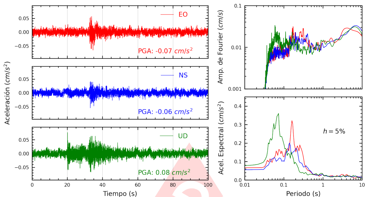
Figura A.29: Registros tiempo-historia, espectros de Fourier y de respuesta en las direcciones EO, NS y vertical de la estación ACAPU. Sismo de Huacho, Huaura - Lima del 2024-10-18, 02:09:02 (Hora local)
