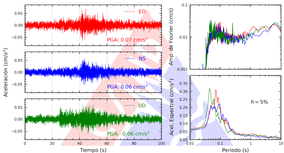
Figura A.31: Registros tiempo-historia, espectros de Fourier y de respuesta en las direcciones EO, NS y vertical de la estación USILP. Sismo de Huacho, Huaura - Lima del 2024-10-18, 02:09:02 (Hora local)
