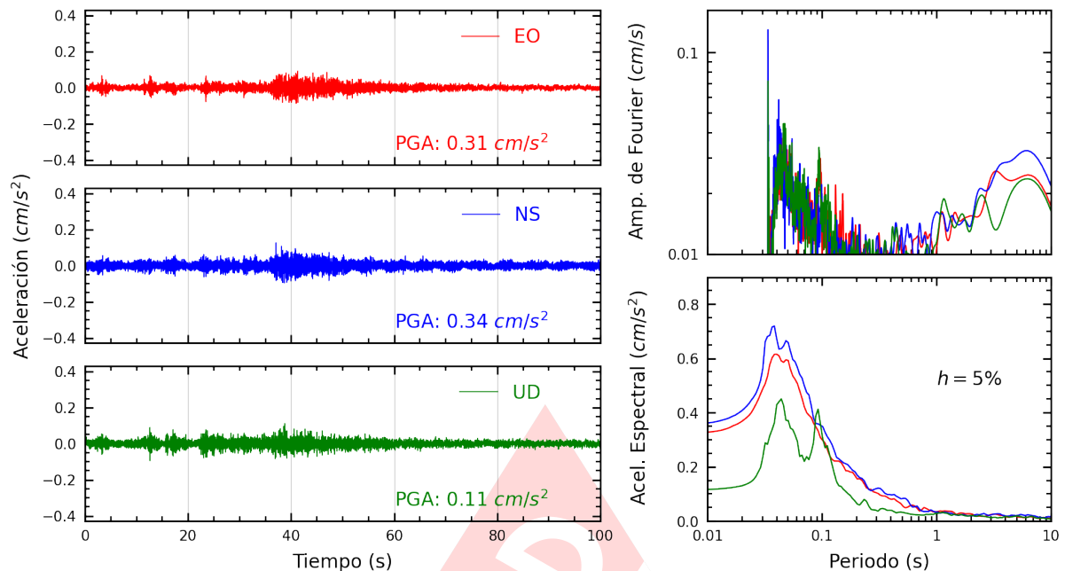
Figura A.9: Registros tiempo-historia, espectros de Fourier y de respuesta en las direcciones EO, NS y vertical de la estación USMP. Sismo de Huacho, Huaura - Lima del 2024-10-18, 02:09:02 (Hora local)
