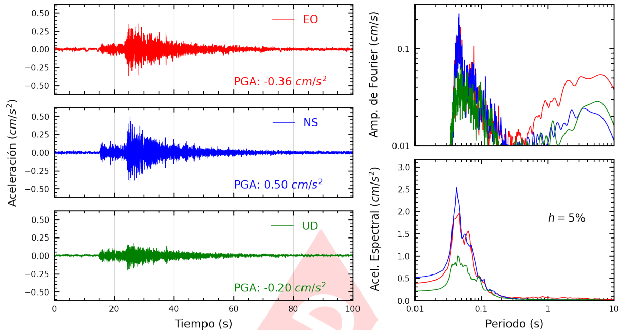
Figura A.5: Registros tiempo-historia, espectros de Fourier y de respuesta en las direcciones EO, NS y vertical de la estación UNAB. Sismo de Huacho, Huaura - Lima del 2024-10-18, 02:09:02 (Hora local)
