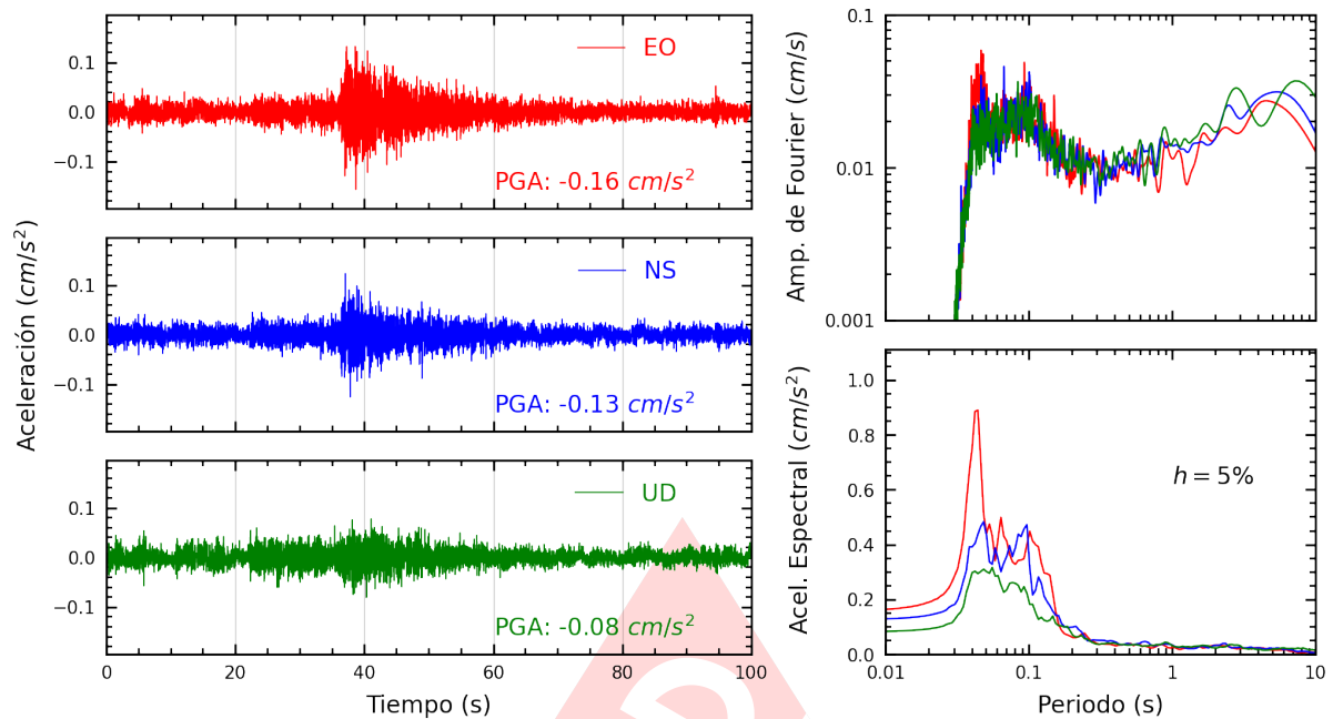
Figura A.17: Registros tiempo-historia, espectros de Fourier y de respuesta en las direcciones EO, NS y vertical de la estación UCVAT. Sismo de Huacho, Huaura - Lima del 2024-10-18, 02:09:02 (Hora local)
