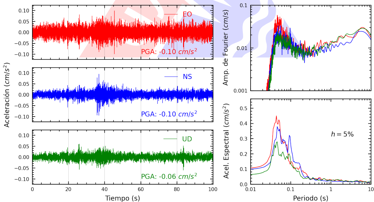
Figura A.26: Registros tiempo-historia, espectros de Fourier y de respuesta en las direcciones EO, NS y vertical de la estación INICT. Sismo de Huacho, Huaura - Lima del 2024-10-18, 02:09:02 (Hora local)
