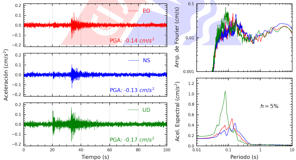
Figura A.16: Registros tiempo-historia, espectros de Fourier y de respuesta en las direcciones EO, NS y vertical de la estación RAMON. Sismo de Huacho, Huaaura - Lima del 2024-10-18, 02:09:02 (Hora local)
