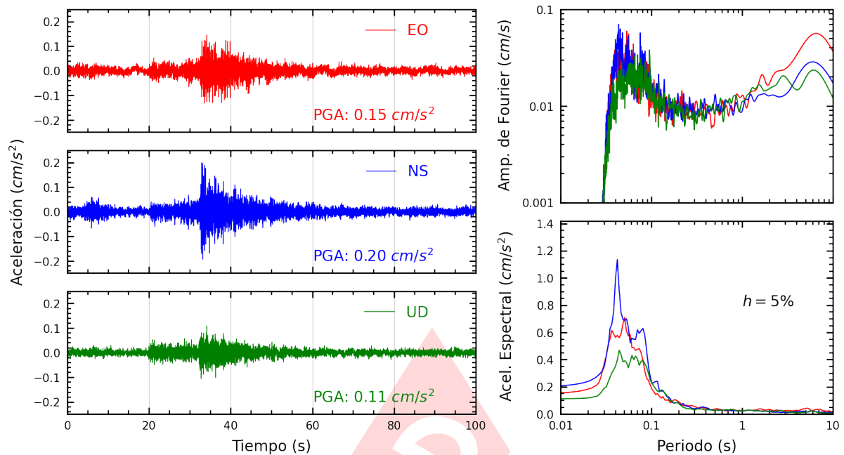
Figura A.13: Registros tiempo-historia, espectros de Fourier y de respuesta en las direcciones EO, NS y vertical de la estación COMAS. Sismo de Huacho, Huaura - Lima del 2024-10-18, 02:09:02 (Hora local)
