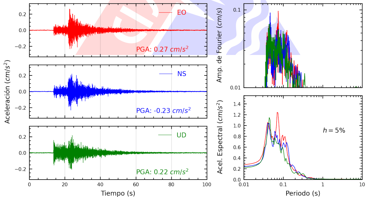
Figura A.12: Registros tiempo-historia, espectros de Fourier y de respuesta en las direcciones EO, NS y vertical de la estación CARAL. Sismo de Huacho, Huaura - Lima del 2024-10-18, 02:09:02 (Hora local)
