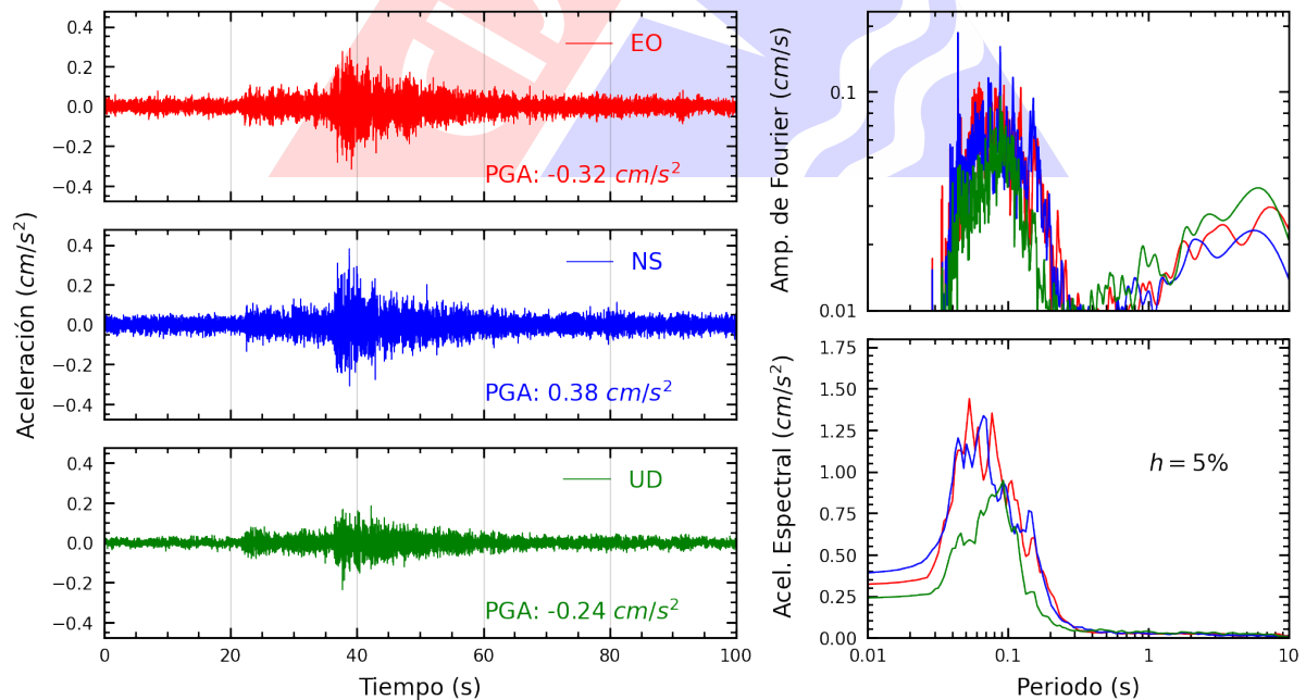
Figura A.8: Registros tiempo-historia, espectros de Fourier y de respuesta en las direcciones EO, NS y vertical de la estación USILM. Sismo de Huacho, Huaura - Lima del 2024-10-18, 02:09:02 (Hora local)
