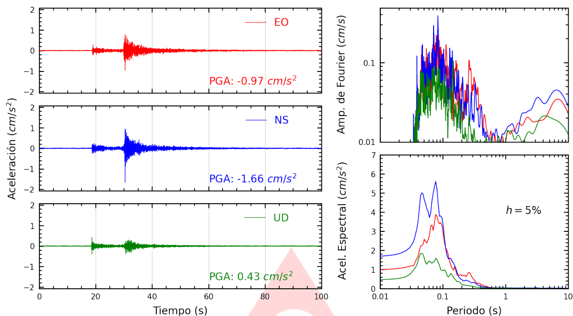
Figura A.1: Registros tiempo-historia, espectros de Fourier y de respuesta en las direcciones EO, NS y vertical de la estación DEFEN. Sismo de Huacho, Huaura - Lima del 2024-10-18, 02:09:02 (Hora local)
