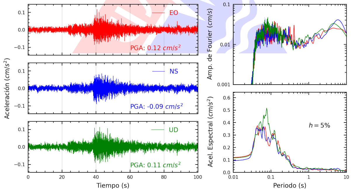
Figura A.22: Registros tiempo-historia, espectros de Fourier y de respuesta en las direcciones EO, NS y vertical de la estación SOVES. Sismo de Huacho, Huaura - Lima del 2024-10-18, 02:09:02 (Hora local)
