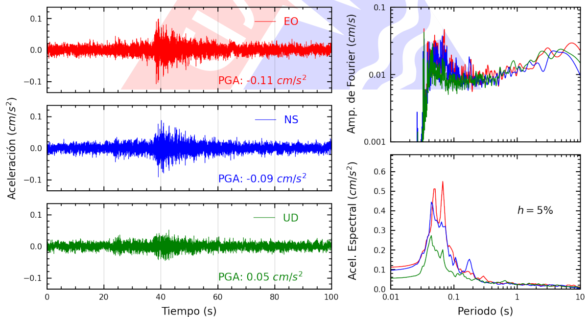
Figura A.24: Registros tiempo-historia, espectros de Fourier y de respuesta en las direcciones EO, NS y vertical de la estación UPCVI. Sismo de Huacho, Huaura - Lima del 2024-10-18, 02:09:02 (Hora local)
