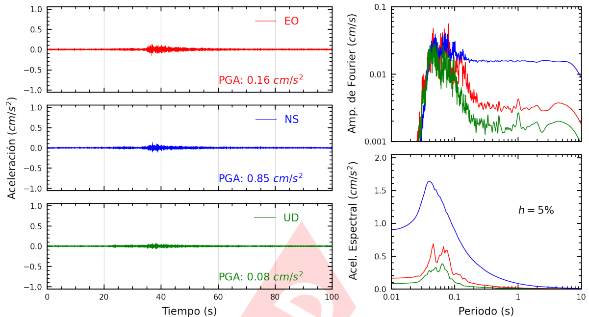
Figura A.3: Registros tiempo-historia, espectros de Fourier y de respuesta en las direcciones EO, NS y vertical de la estación ATARJ. Sismo de Huacho, Huaura - Lima del 2024-10-18, 02:09:02 (Hora local)
