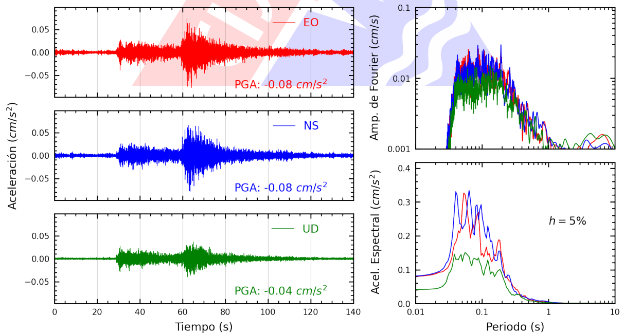
Figura A.4: Registros tiempo-historia, espectros de Fourier y de respuesta en las direcciones EO, NS y vertical de la estación UNSA2. Sismo de Calana, Tacna - Tacna del 2024-10-20, 15:20:38 (Hora local)
