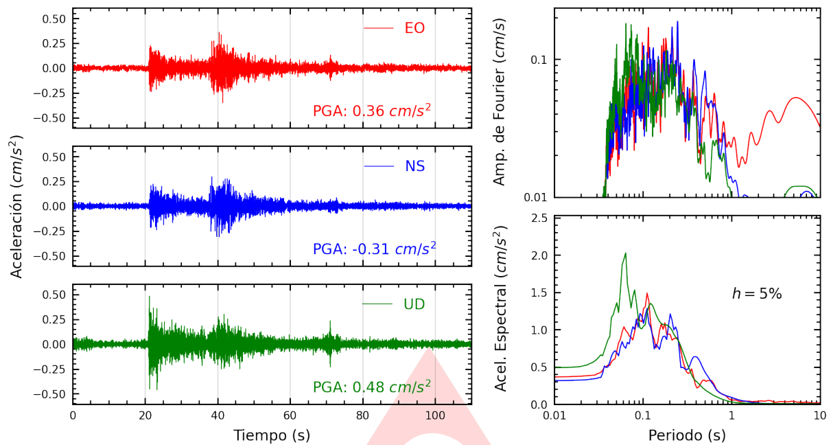
Figura A.1: Registros tiempo-historia, espectros de Fourier y de respuesta en las direcciones EO, NS y vertical de la estación UJBG3. Sismo de Calana, Tacna - Tacna del 2024-10-20, 15:20:38 (Hora local)
