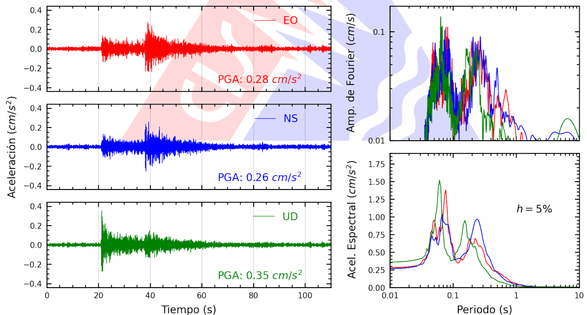
Figura A.2: Registros tiempo-historia, espectros de Fourier y de respuesta en las direcciones EO, NS y vertical de la estación CREY. Sismo de Calana, Tacna - Tacna del 2024-10-20, 15:20:38 (Hora local)
