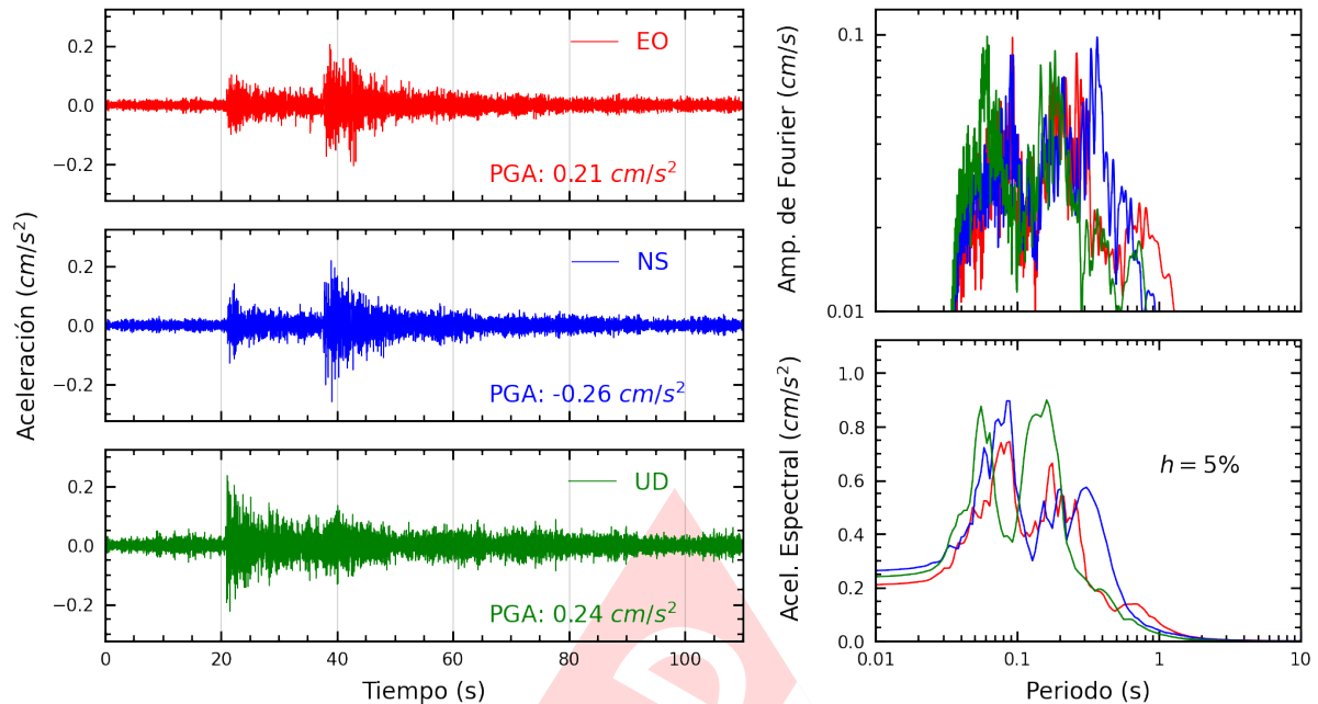
Figura A.3: Registros tiempo-historia, espectros de Fourier y de respuesta en las direcciones EO, NS y vertical de la estación UJBG2. Sismo de Calana, Tacna - Tacna del 2024-10-20, 15:20:38 (Hora local)
