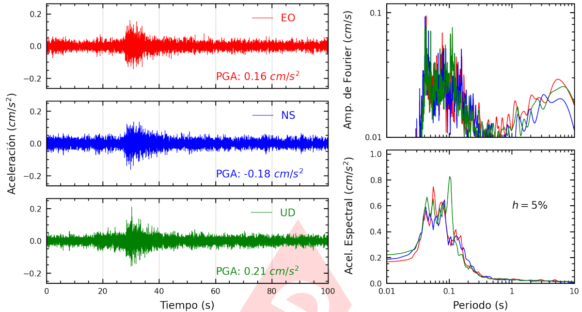
Figura A.35: Registros tiempo-historia, espectros de Fourier y de respuesta en las direcciones EO, NS y vertical de la estación BONDY. Sismo de Mala, Cañete - Lima del 2024-10-25, 09:22:30 (Hora local)
