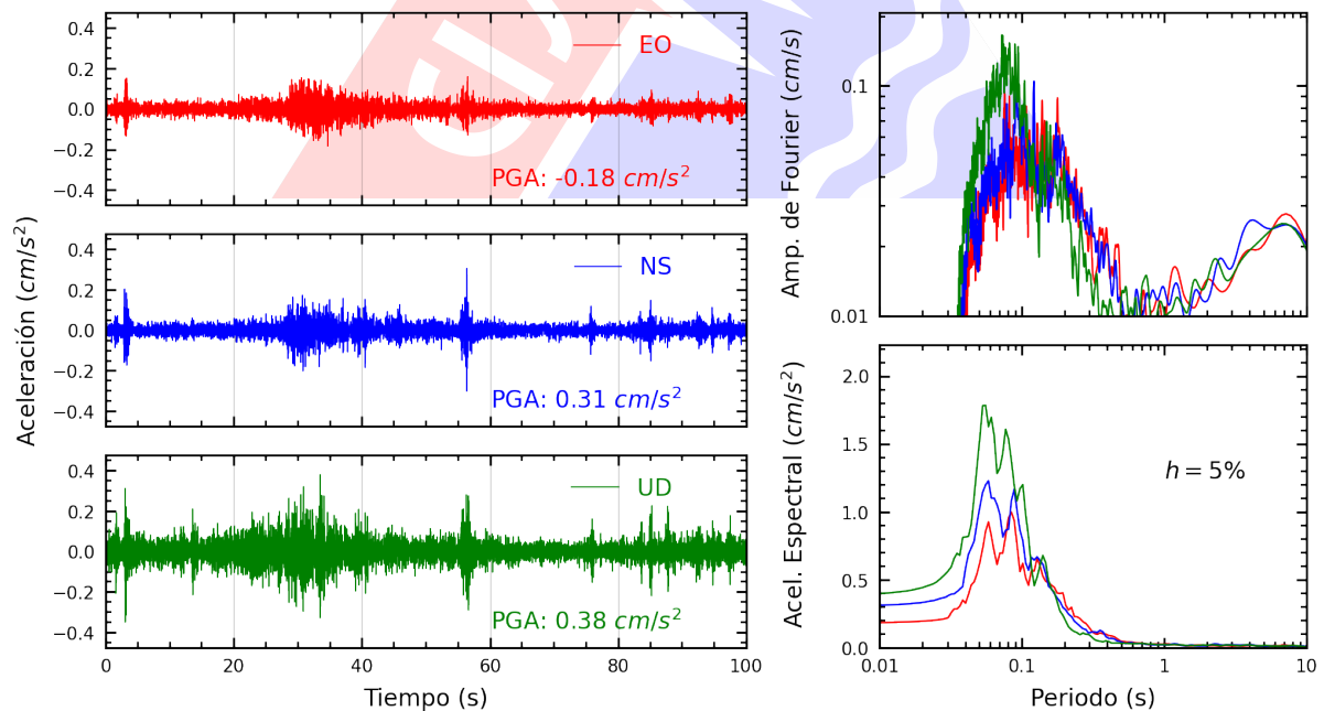
Figura A.30: Registros tiempo-historia, espectros de Fourier y de respuesta en las direcciones EO, NS y vertical de la estación RAMON. Sismo de Mala, Cañete - Lima del 2024-10-25, 09:22:30 (Hora local)
