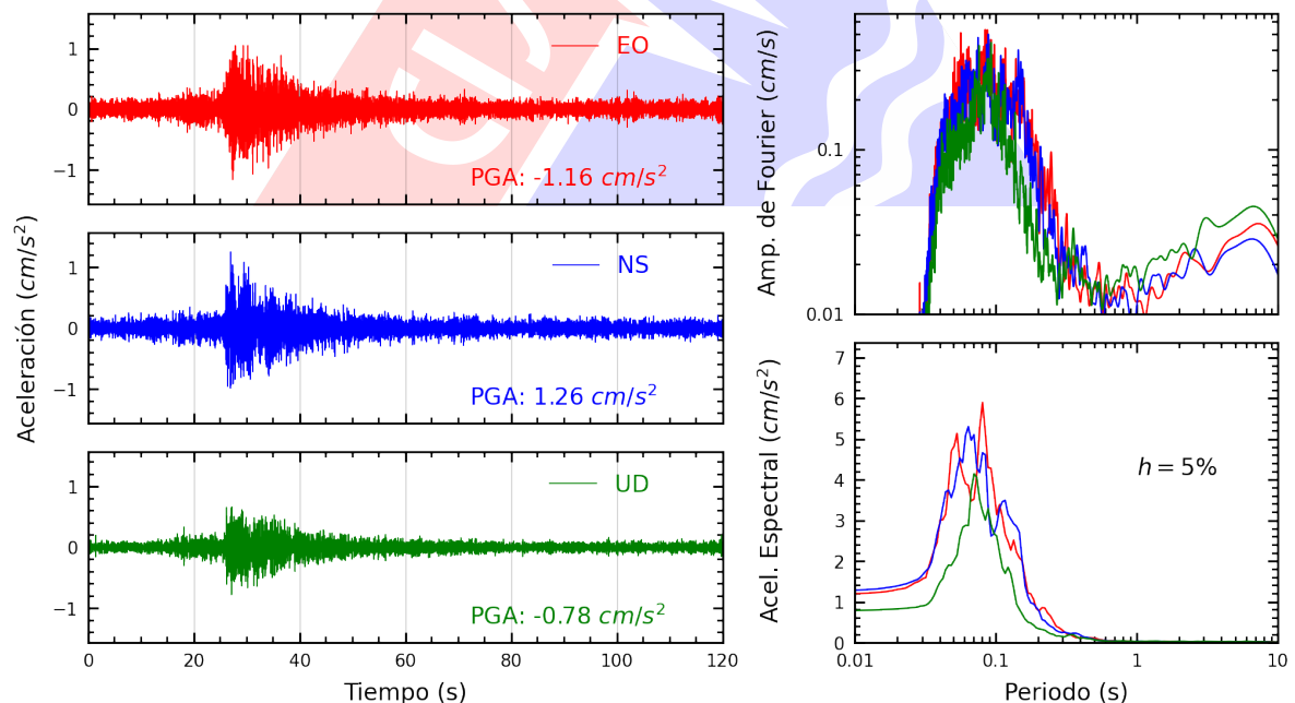
Figura A.10: Registros tiempo-historia, espectros de Fourier y de respuesta en las direcciones EO, NS y vertical de la estación USILM. Sismo de Mala, Cañete - Lima del 2024-10-25, 09:22:30 (Hora local)
