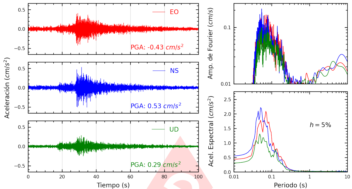
Figura A.21: Registros tiempo-historia, espectros de Fourier y de respuesta en las direcciones EO, NS y vertical de la estación FICPE. Sismo de Mala, Cañete - Lima del 2024-10-25, 09:22:30 (Hora local)
