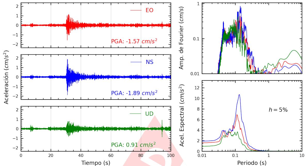
Figura A.3: Registros tiempo-historia, espectros de Fourier y de respuesta en las direcciones EO, NS y vertical de la estación CARAB. Sismo de Mala, Cañete - Lima del 2024-10-25, 09:22:30 (Hora local)
