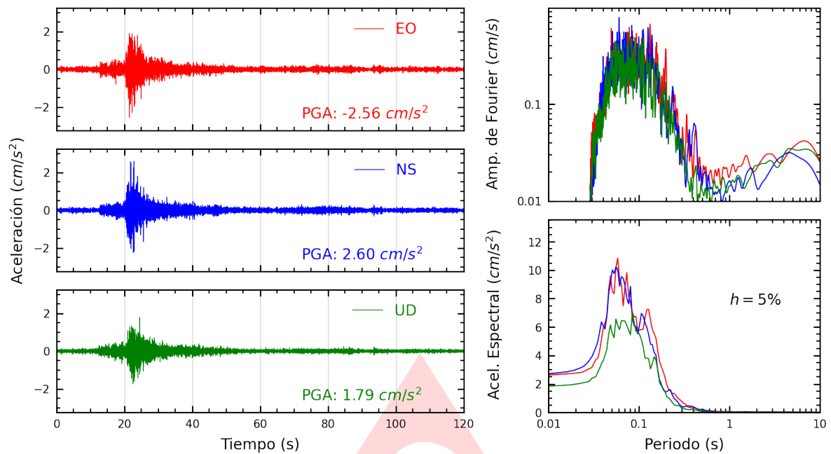
Figura A.1: Registros tiempo-historia, espectros de Fourier y de respuesta en las direcciones EO, NS y vertical de la estación PHERM. Sismo de Mala, Cañete - Lima del 2024-10-25, 09:22:30 (Hora local)
