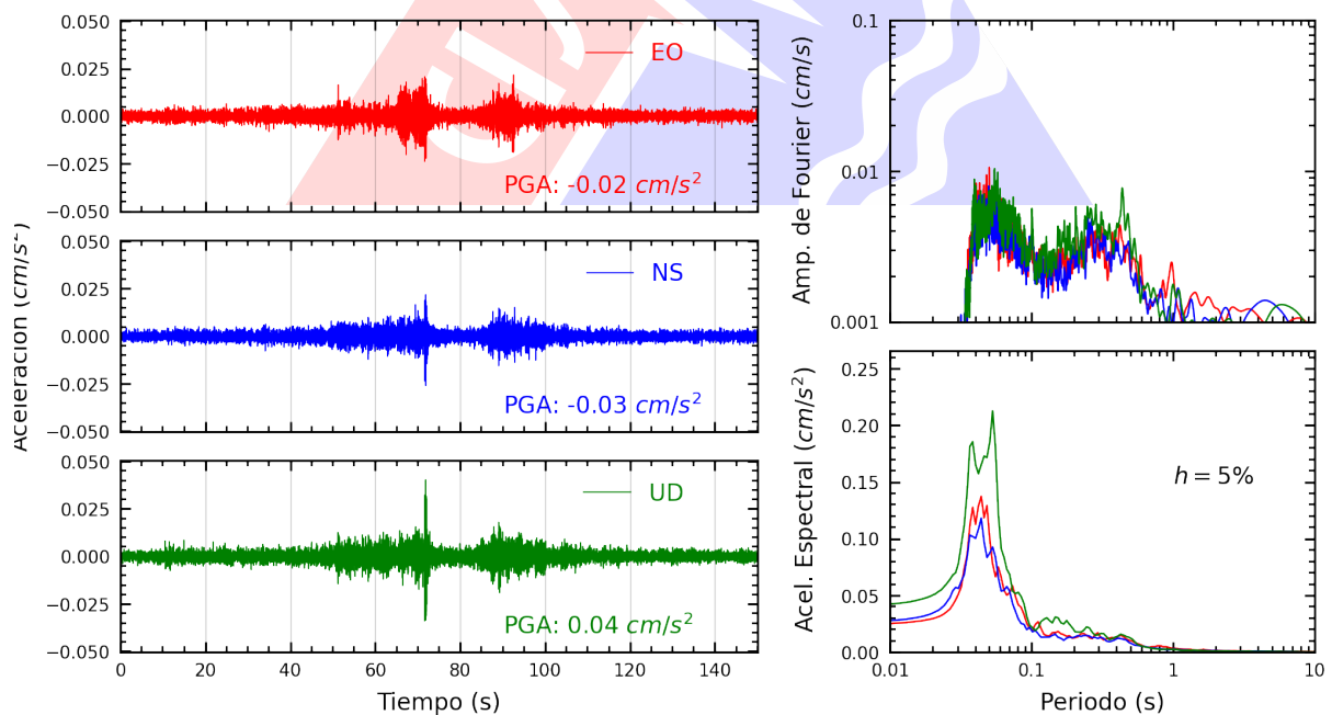
Figura A.38: Registros tiempo-historia, espectros de Fourier y de respuesta en las direcciones EO, NS y vertical de la estación UNCP. Sismo de Mala, Cañete - Lima del 2024-10-25, 09:22:30 (Hora local)
