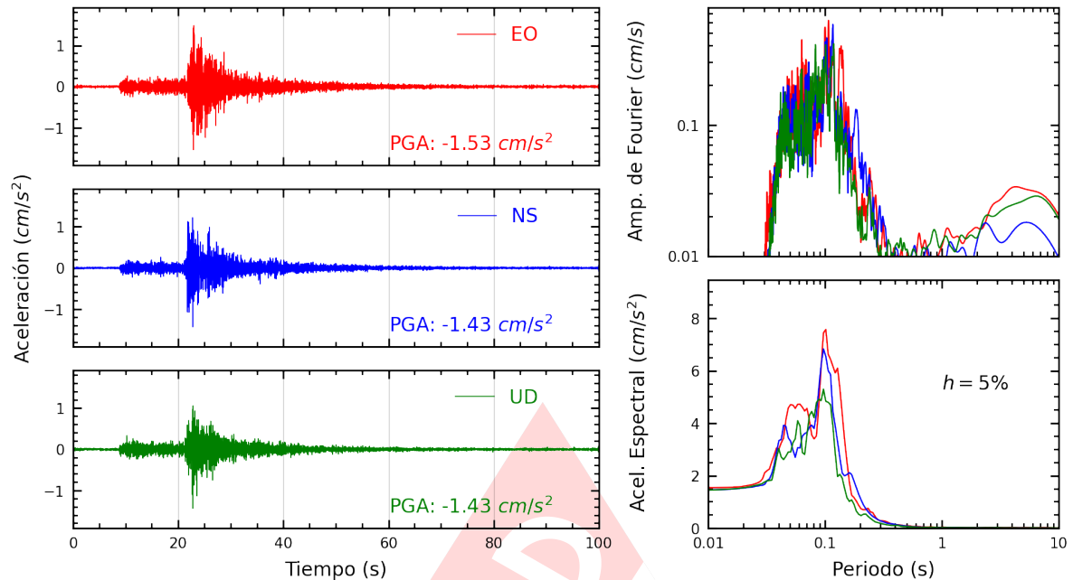
Figura A.5: Registros tiempo-historia, espectros de Fourier y de respuesta en las direcciones EO, NS y vertical de la estación AMORE. Sismo de Mala, Cañete - Lima del 2024-10-25, 09:22:30 (Hora local)
