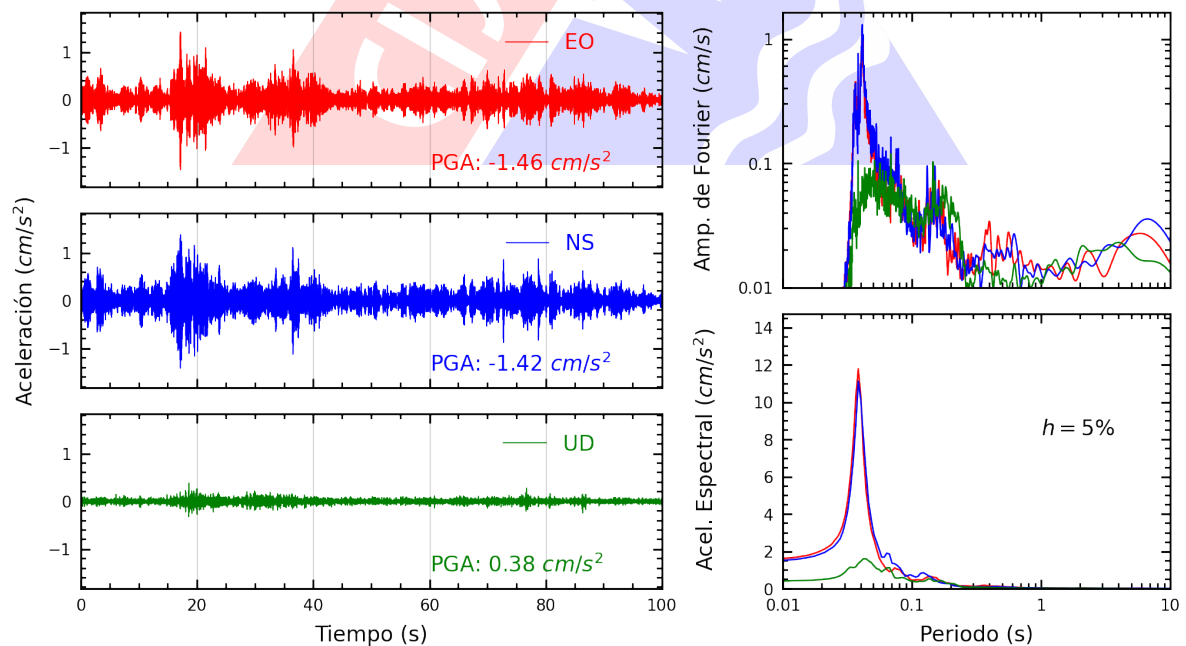
Figura A.6: Registros tiempo-historia, espectros de Fourier y de respuesta en las direcciones EO, NS y vertical de la estación DHNPE. Sismo de Mala, Cañete - Lima del 2024-10-25, 09:22:30 (Hora local)
