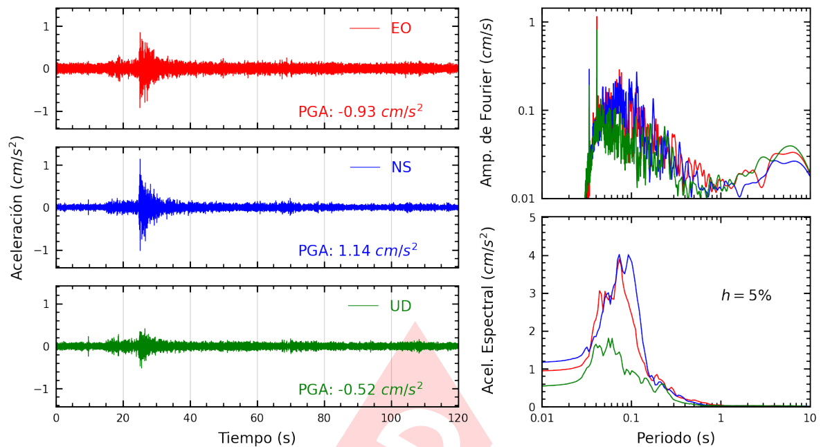
Figura A.11: Registros tiempo-historia, espectros de Fourier y de respuesta en las direcciones EO, NS y vertical de la estación UPCVI. Sismo de Mala, Cañete - Lima del 2024-10-25, 09:22:30 (Hora local)
