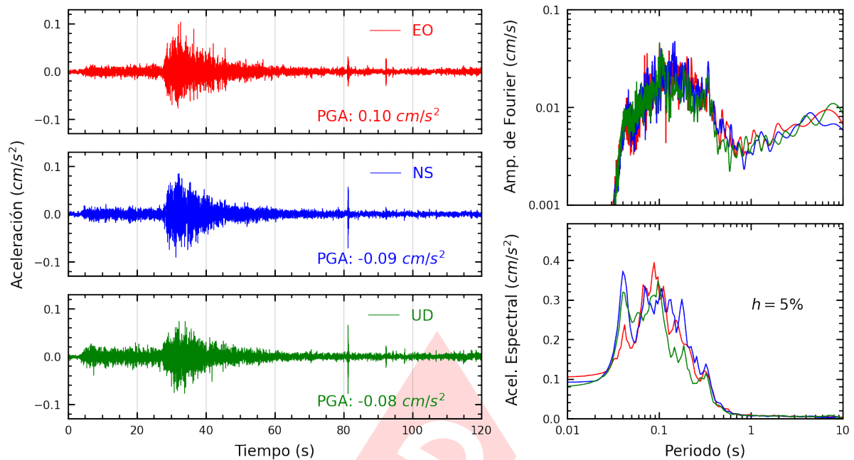
Figura A.37: Registros tiempo-historia, espectros de Fourier y de respuesta en las direcciones EO, NS y vertical de la estación CARAL. Sismo de Mala, Cañete - Lima del 2024-10-25, 09:22:30 (Hora local)
