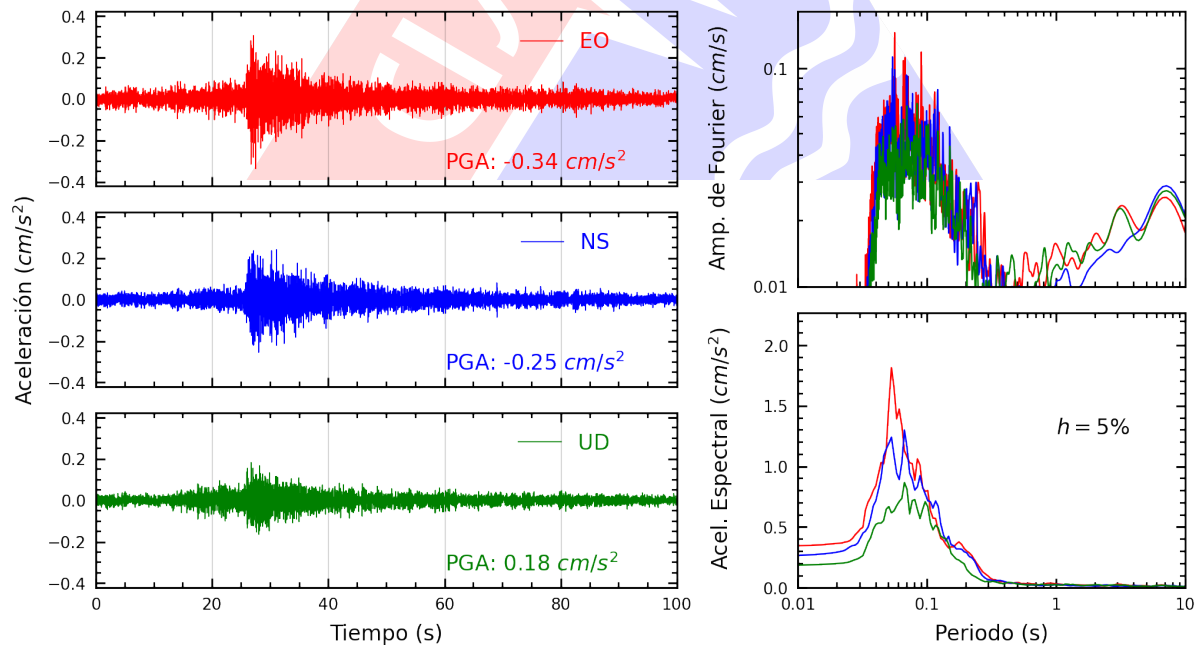
Figura A.32: Registros tiempo-historia, espectros de Fourier y de respuesta en las direcciones EO, NS y vertical de la estación INICT. Sismo de Mala, Cañete - Lima del 2024-10-25, 09:22:30 (Hora local)
