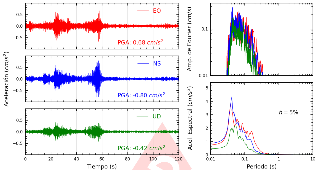
Figura A.17: Registros tiempo-historia, espectros de Fourier y de respuesta en las direcciones EO, NS y vertical de la estación PACHA. Sismo de Mala, Cañete - Lima del 2024-10-25, 09:22:30 (Hora local)
