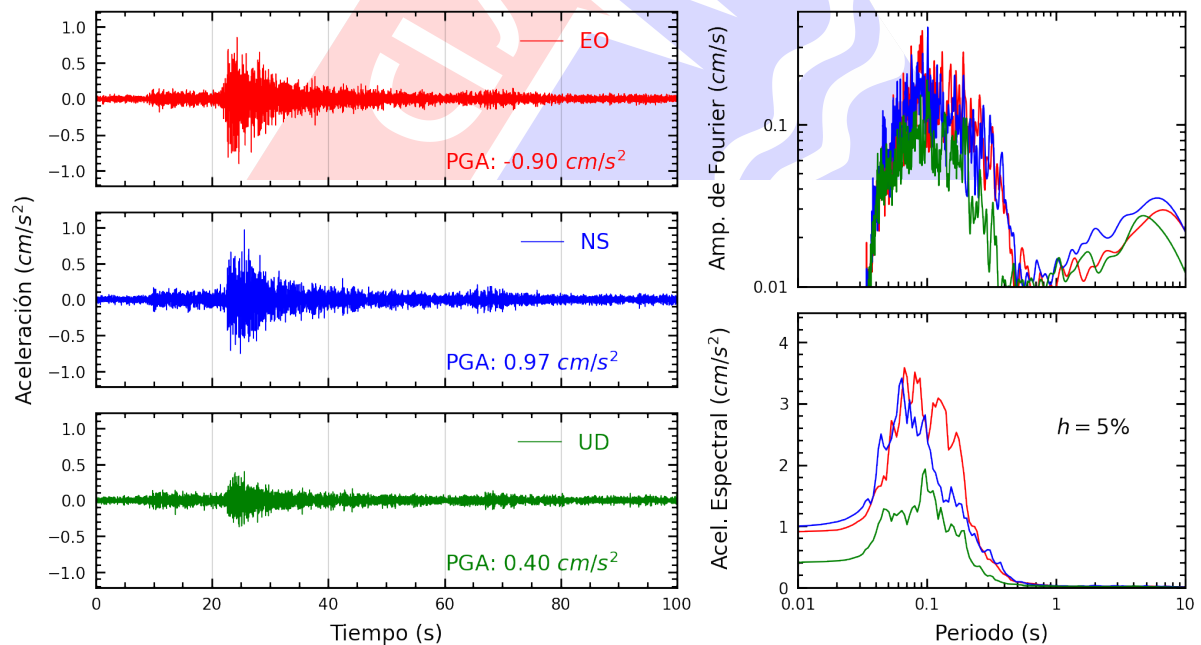
Figura A.16: Registros tiempo-historia, espectros de Fourier y de respuesta en las direcciones EO, NS y vertical de la estación DEFEN. Sismo de Mala, Cañete - Lima del 2024-10-25, 09:22:30 (Hora local)
