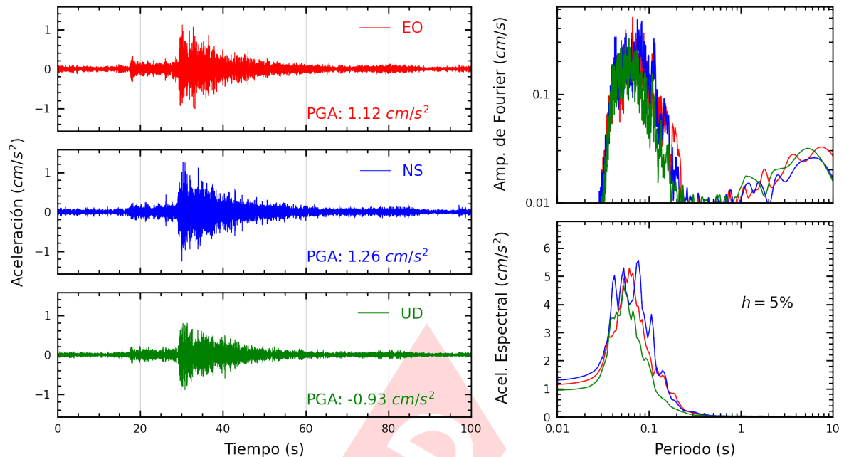
Figura A.9: Registros tiempo-historia, espectros de Fourier y de respuesta en las direcciones EO, NS y vertical de la estación JOSEO. Sismo de Mala, Cañete - Lima del 2024-10-25, 09:22:30 (Hora local)
