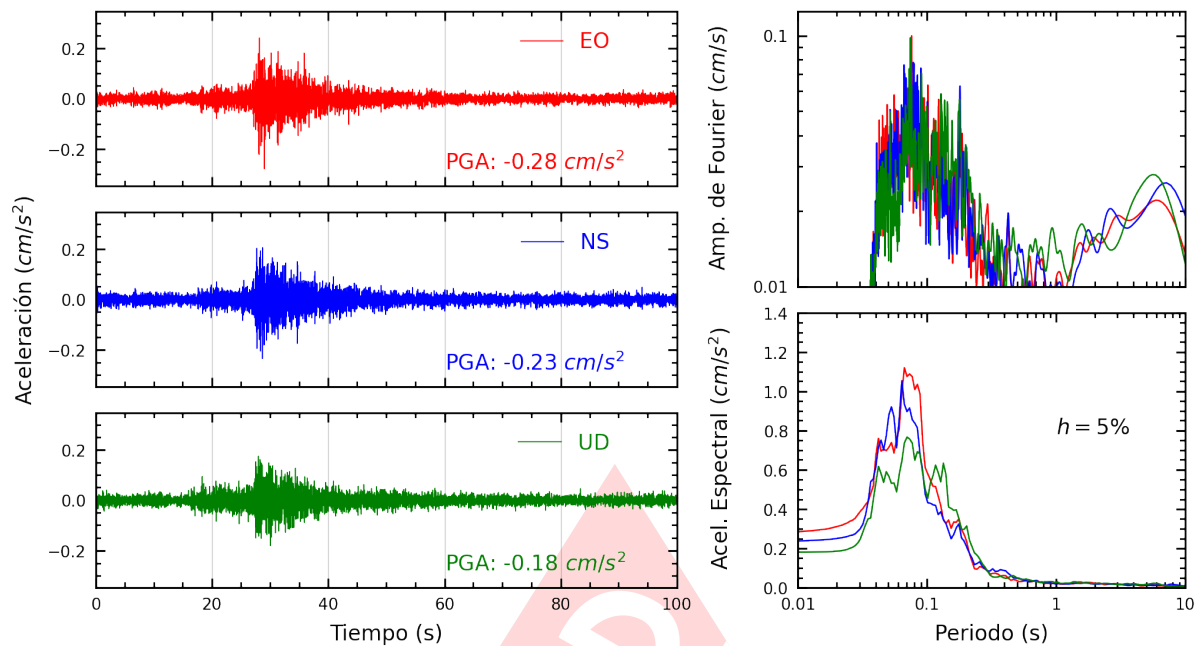
Figura A.33: Registros tiempo-historia, espectros de Fourier y de respuesta en las direcciones EO, NS y vertical de la estación UNFV. Sismo de Mala, Cañete - Lima del 2024-10-25, 09:22:30 (Hora local)
