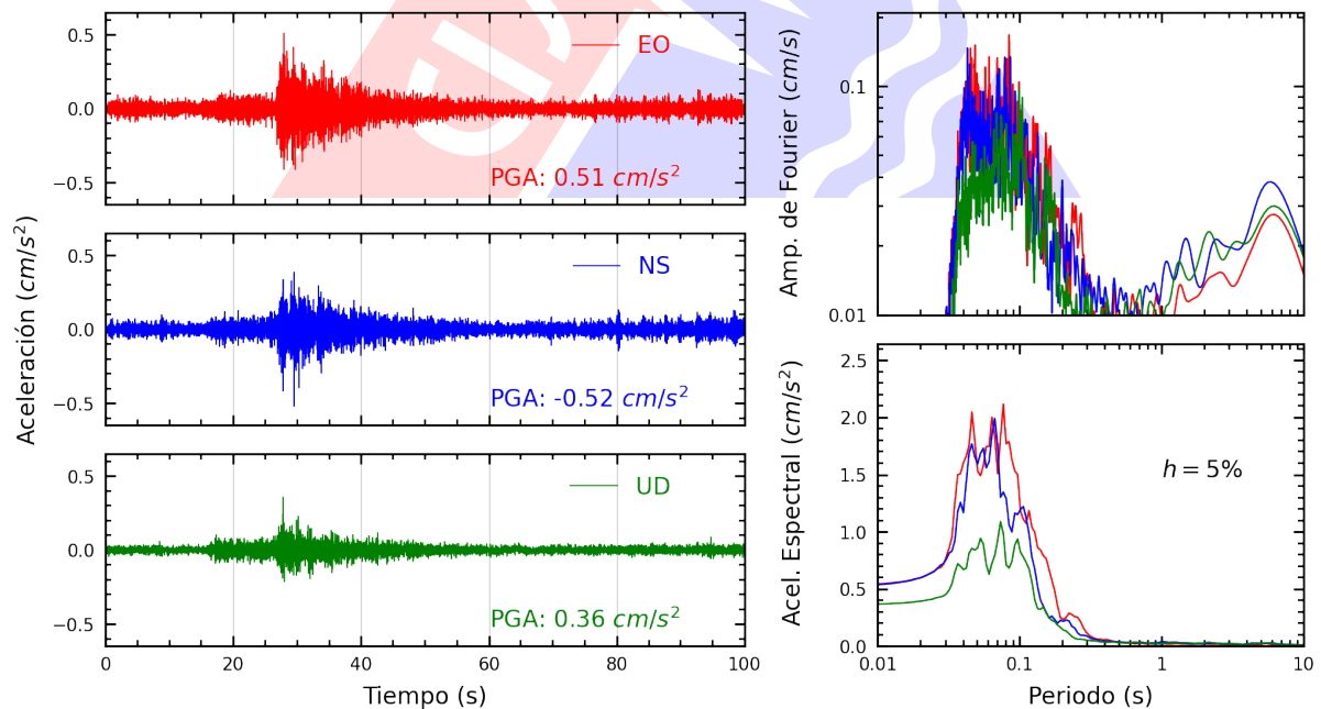
Figura A.22: Registros tiempo-historia, espectros de Fourier y de respuesta en las direcciones EO, NS y vertical de la estación CEPRE. Sismo de Mala, Cañete - Lima del 2024-10-25, 09:22:30 (Hora local)
