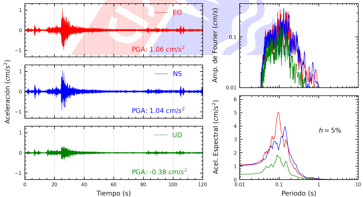
Figura A.12: Registros tiempo-historia, espectros de Fourier y de respuesta en las direcciones EO, NS y vertical de la estación BRISA. Sismo de Mala, Cañete - Lima del 2024-10-25, 09:22:30 (Hora local)
