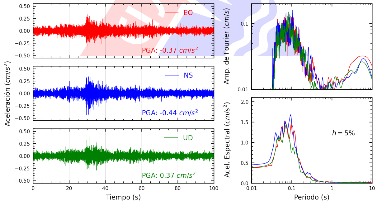
Figura A.26: Registros tiempo-historia, espectros de Fourier y de respuesta en las direcciones EO, NS y vertical de la estación MADRE. Sismo de Mala, Cañete - Lima del 2024-10-25, 09:22:30 (Hora local)
