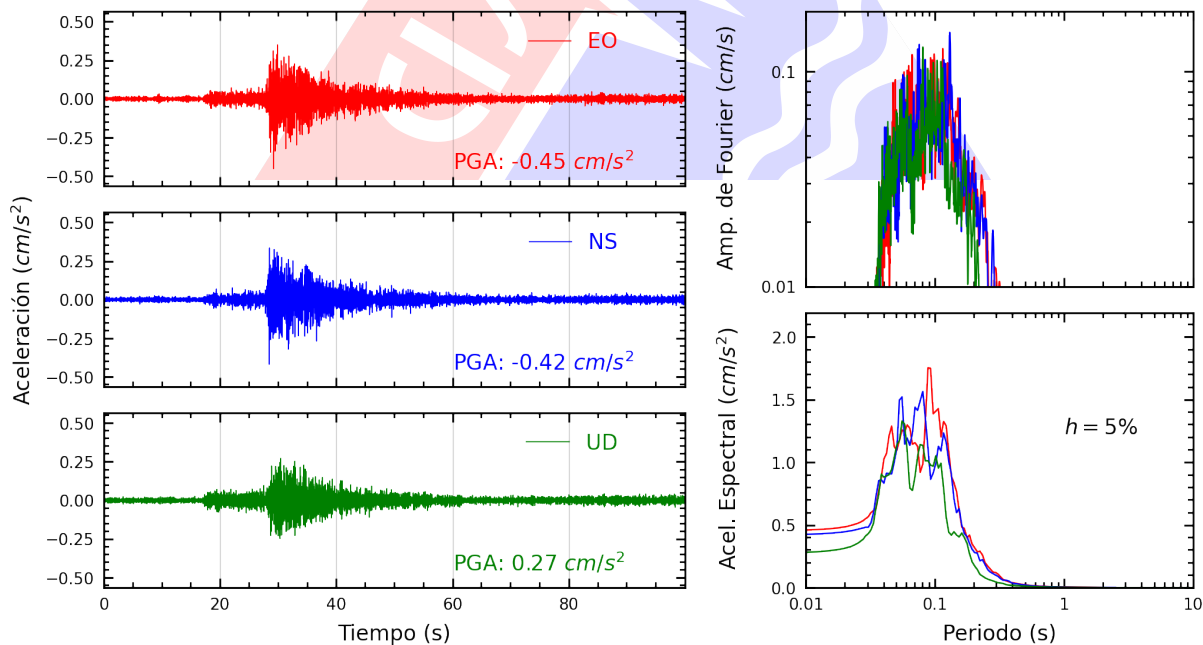
Figura A.24: Registros tiempo-historia, espectros de Fourier y de respuesta en las direcciones EO, NS y vertical de la estación JALV2. Sismo de Mala, Cañete - Lima del 2024-10-25, 09:22:30 (Hora local)
