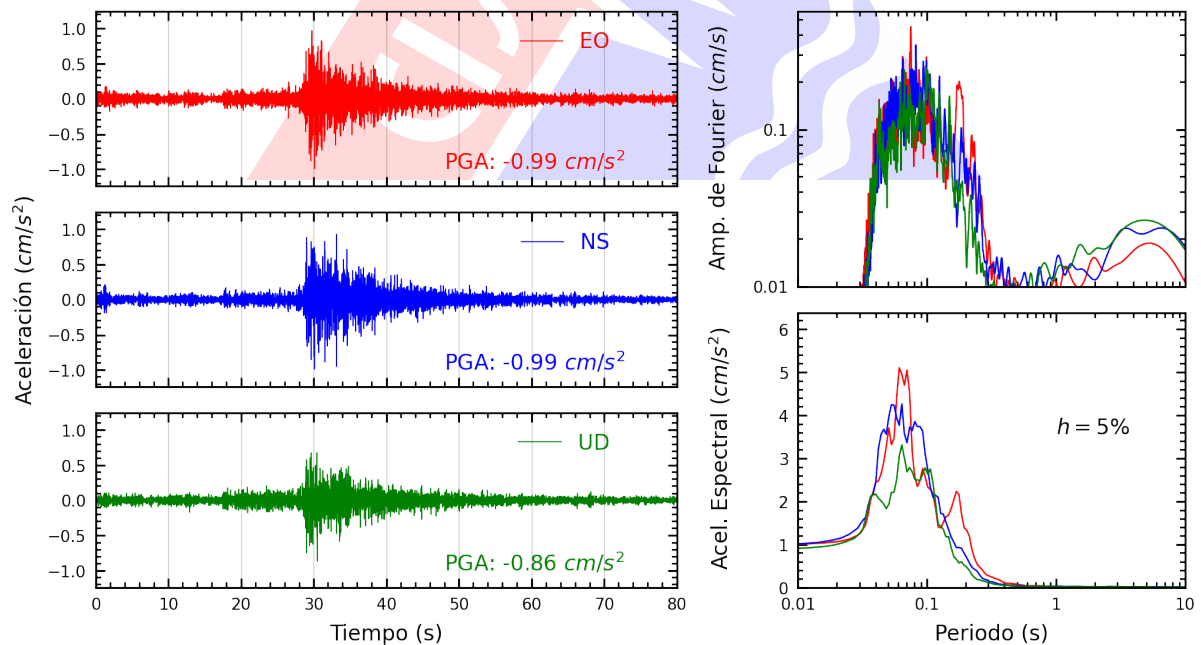
Figura A.14: Registros tiempo-historia, espectros de Fourier y de respuesta en las direcciones EO, NS y vertical de la estación INDEP. Sismo de Mala, Cañete - Lima del 2024-10-25, 09:22:30 (Hora local)
