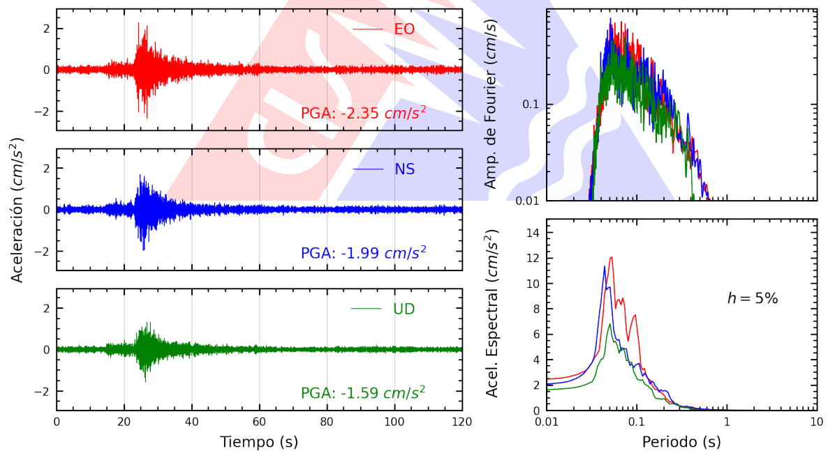
Figura A.2: Registros tiempo-historia, espectros de Fourier y de respuesta en las direcciones EO, NS y vertical de la estación UNTEL. Sismo de Mala, Cañete - Lima del 2024-10-25, 09:22:30 (Hora local)
