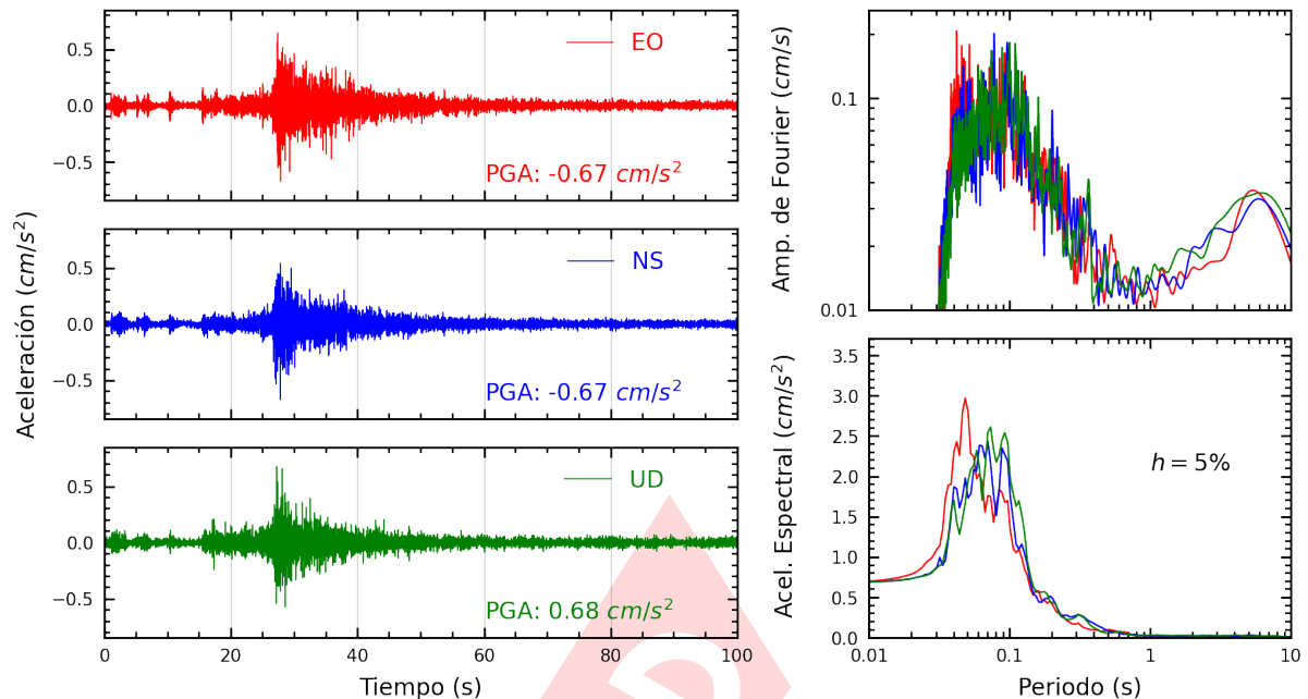
Figura A.19: Registros tiempo-historia, espectros de Fourier y de respuesta en las direcciones EO, NS y vertical de la estación UCVAT. Sismo de Mala, Cañete - Lima del 2024-10-25, 09:22:30 (Hora local)
