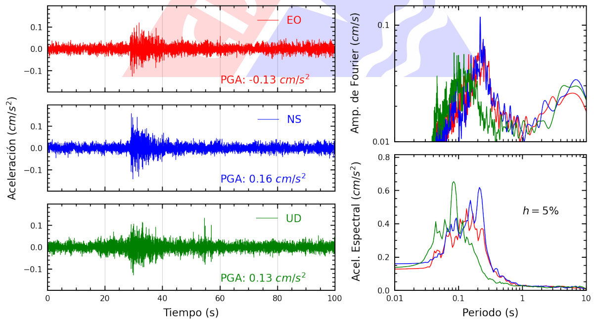
Figura A.36: Registros tiempo-historia, espectros de Fourier y de respuesta en las direcciones EO, NS y vertical de la estación DSMI. Sismo de Mala, Cañete - Lima del 2024-10-25, 09:22:30 (Hora local)
