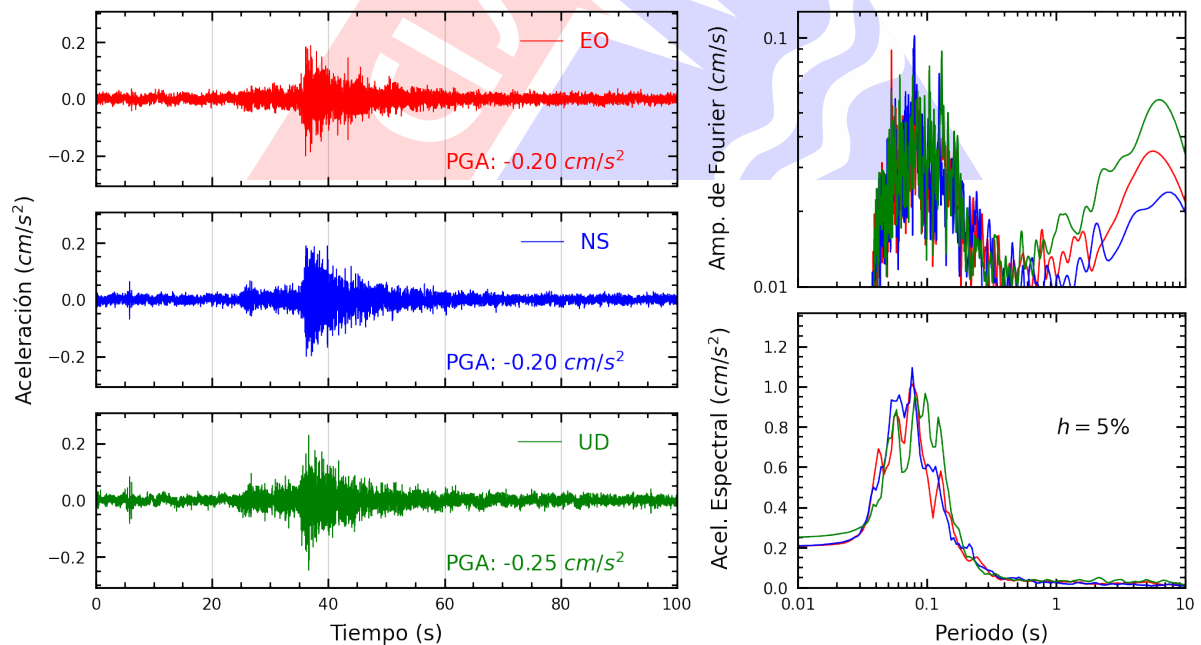
Figura A.34: Registros tiempo-historia, espectros de Fourier y de respuesta en las direcciones EO, NS y vertical de la estación UNMSM. Sismo de Mala, Cañete - Lima del 2024-10-25, 09:22:30 (Hora local)
