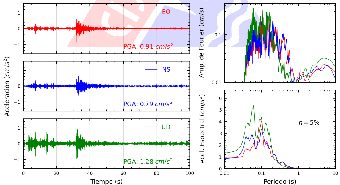
Figura A.8: Registros tiempo-historia, espectros de Fourier y de respuesta en las direcciones EO, NS y vertical de la estación MDPP. Sismo de Mala, Cañete - Lima del 2024-10-25, 09:22:30 (Hora local)
