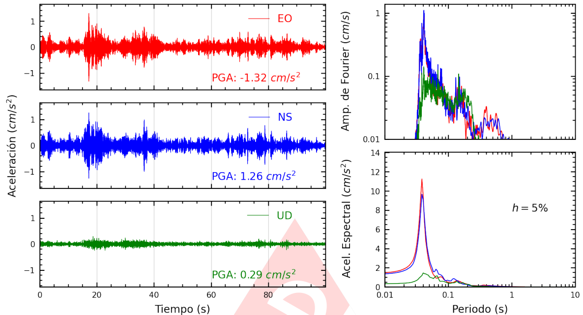
Figura A.7: Registros tiempo-historia, espectros de Fourier y de respuesta en las direcciones EO, NS y vertical de la estación DHN2. Sismo de Mala, Cañete - Lima del 2024-10-25, 09:22:30 (Hora local)
