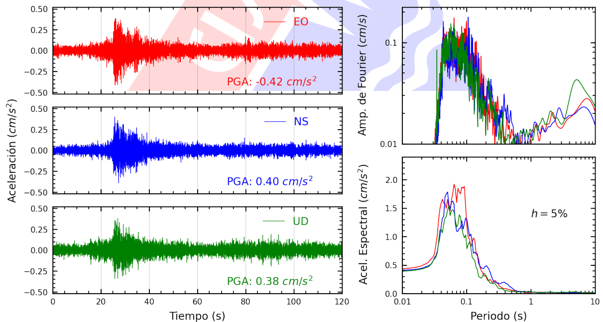
Figura A.28: Registros tiempo-historia, espectros de Fourier y de respuesta en las direcciones EO, NS y vertical de la estación URPE. Sismo de Mala, Cañete - Lima del 2024-10-25, 09:22:30 (Hora local)
