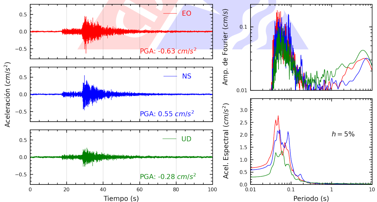
Figura A.20: Registros tiempo-historia, espectros de Fourier y de respuesta en las direcciones EO, NS y vertical de la estación UCSS. Sismo de Mala, Cañete - Lima del 2024-10-25, 09:22:30 (Hora local)
