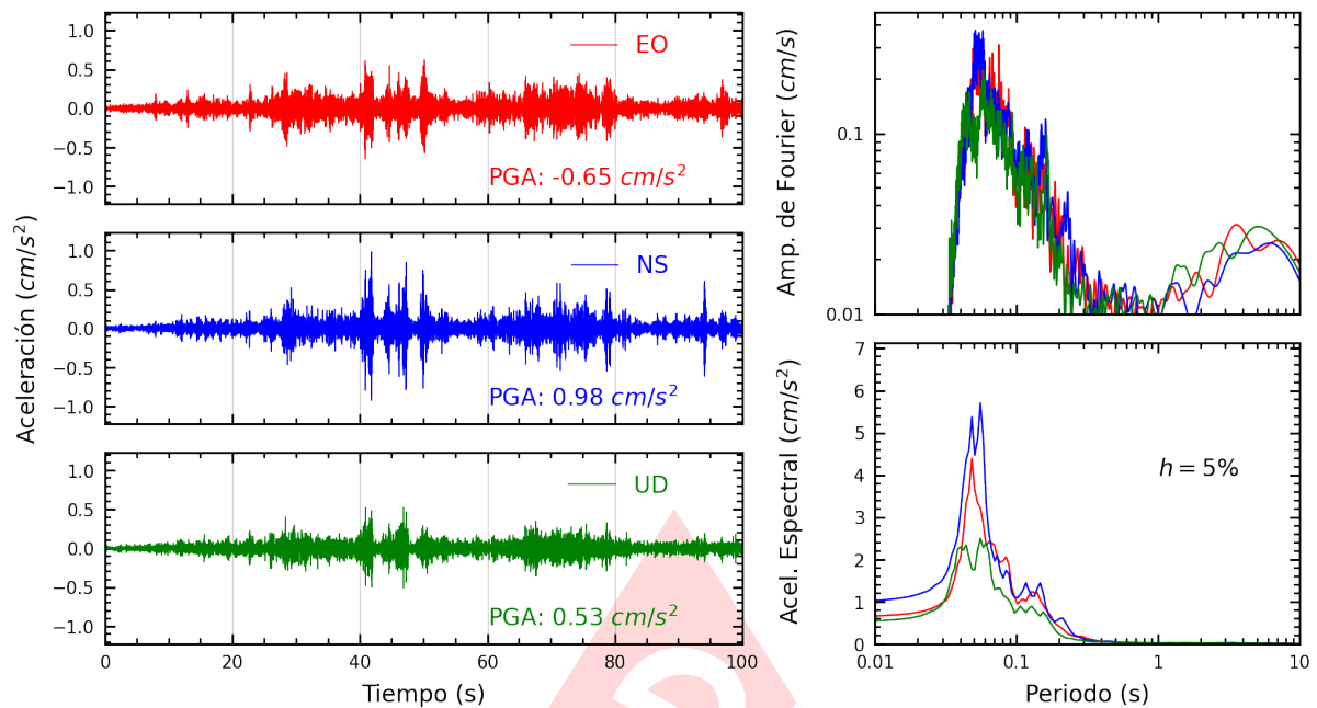
Figura A.15: Registros tiempo-historia, espectros de Fourier y de respuesta en las direcciones EO, NS y vertical de la estación UPCSM. Sismo de Mala, Cañete - Lima del 2024-10-25, 09:22:30 (Hora local)
