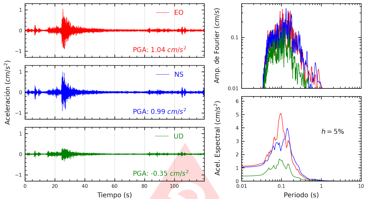
Figura A.13: Registros tiempo-historia, espectros de Fourier y de respuesta en las direcciones EO, NS y vertical de la estación BRIS2. Sismo de Mala, Cañete - Lima del 2024-10-25, 09:22:30 (Hora local)
