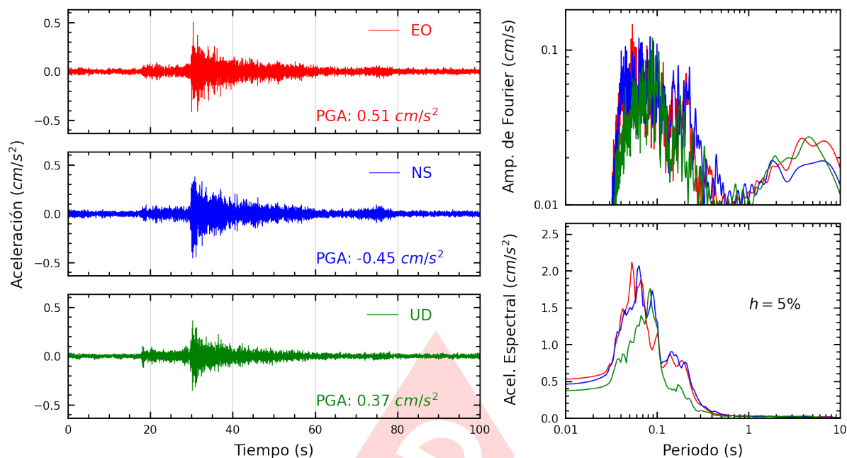
Figura A.23: Registros tiempo-historia, espectros de Fourier y de respuesta en las direcciones EO, NS y vertical de la estación COMAS. Sismo de Mala, Cañete - Lima del 2024-10-25, 09:22:30 (Hora local)
