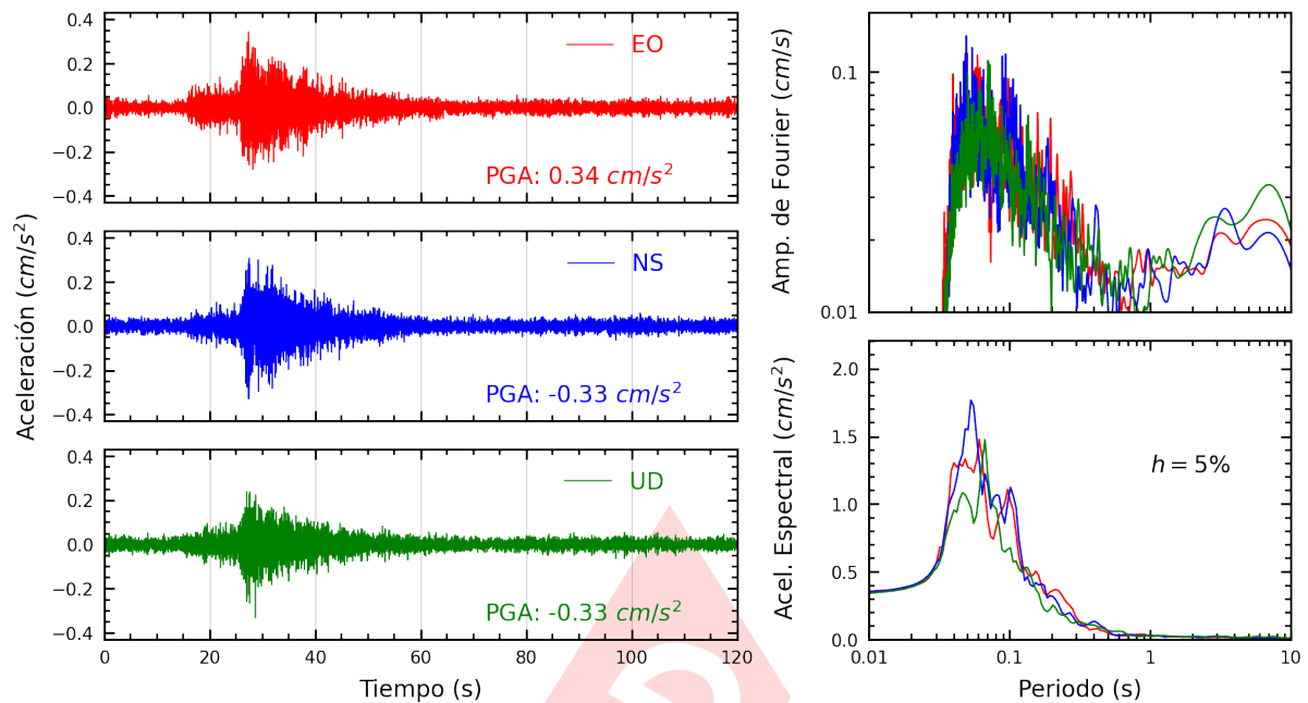
Figura A.31: Registros tiempo-historia, espectros de Fourier y de respuesta en las direcciones EO, NS y vertical de la estación IMCA. Sismo de Mala, Cañete - Lima del 2024-10-25, 09:22:30 (Hora local)
