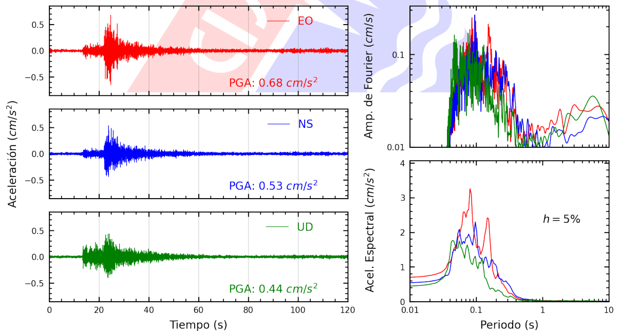
Figura A.18: Registros tiempo-historia, espectros de Fourier y de respuesta en las direcciones EO, NS y vertical de la estación USILP. Sismo de Mala, Cañete - Lima del 2024-10-25, 09:22:30 (Hora local)
