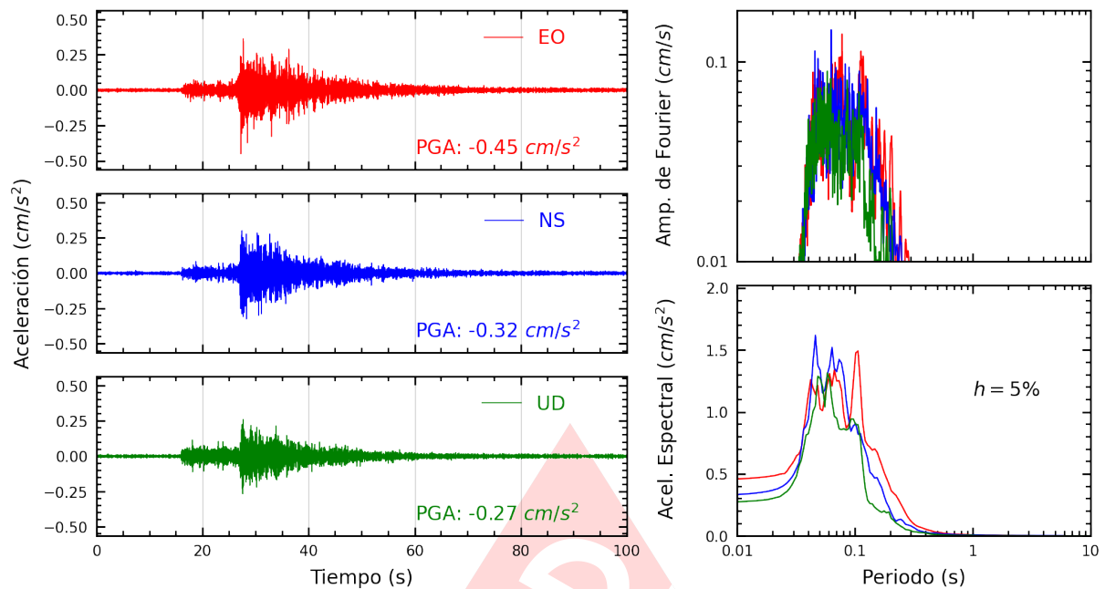
Figura A.25: Registros tiempo-historia, espectros de Fourier y de respuesta en las direcciones EO, NS y vertical de la estación ATARJ. Sismo de Mala, Cañete - Lima del 2024-10-25, 09:22:30 (Hora local)
