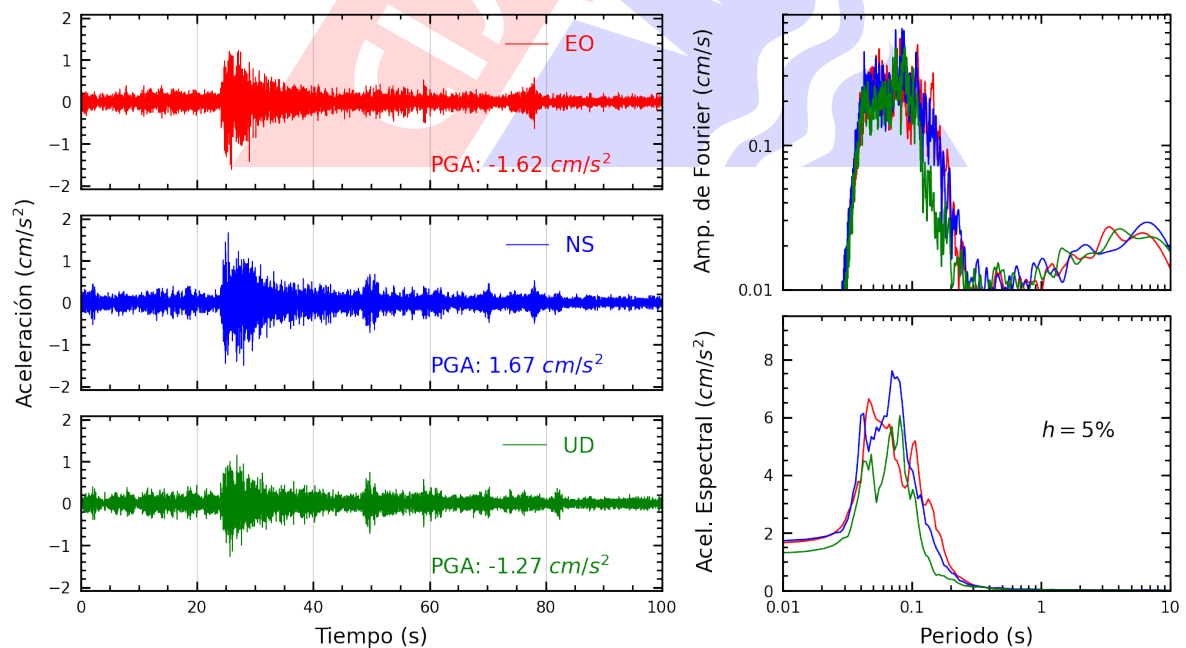
Figura A.4: Registros tiempo-historia, espectros de Fourier y de respuesta en las direcciones EO, NS y vertical de la estación SROSA. Sismo de Mala, Cañete - Lima del 2024-10-25, 09:22:30 (Hora local)
