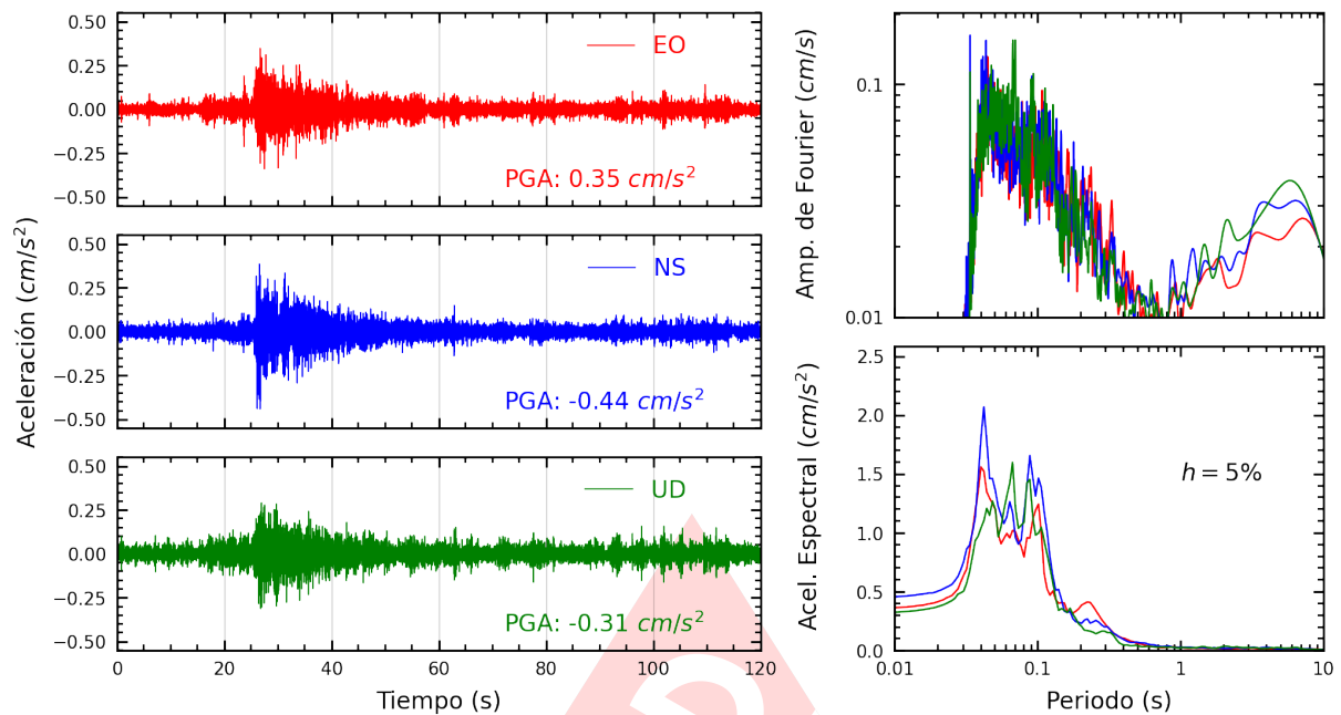
Figura A.27: Registros tiempo-historia, espectros de Fourier y de respuesta en las direcciones EO, NS y vertical de la estación USMP. Sismo de Mala, Cañete - Lima del 2024-10-25, 09:22:30 (Hora local)
