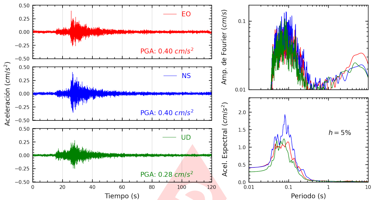
Figura A.29: Registros tiempo-historia, espectros de Fourier y de respuesta en las direcciones EO, NS y vertical de la estación SERVI. Sismo de Mala, Cañete - Lima del 2024-10-25, 09:22:30 (Hora local)
