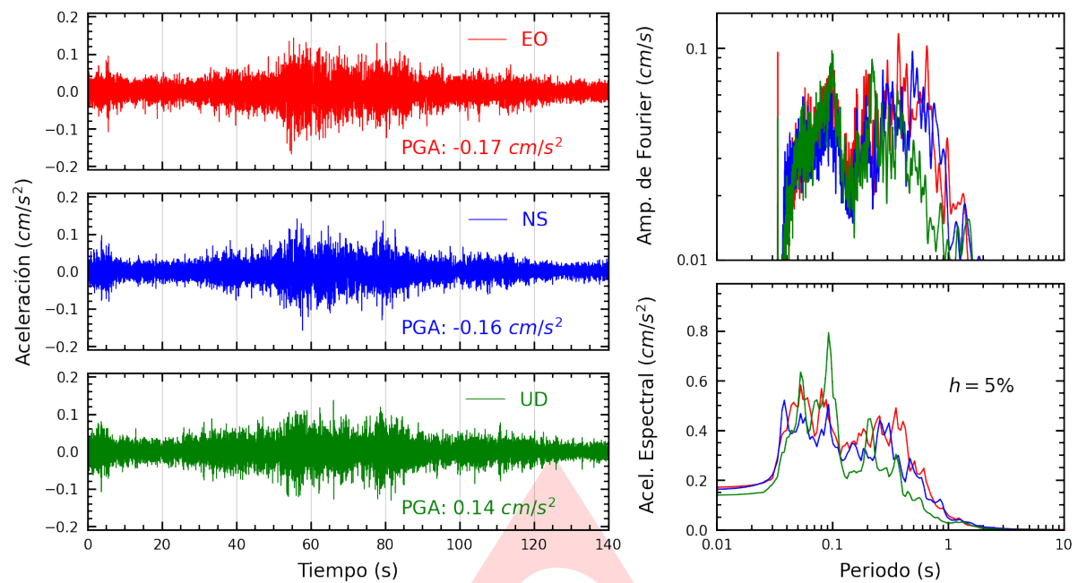
Figura A.1: Registros tiempo-historia, espectros de Fourier y de respuesta en las direcciones EO, NS y vertical de la estación SCICA. Sismo de Lomas, Caraveli - Arequipa del 2024-07-19, 01:54:08 (Hora local)
