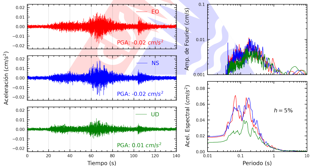
Figura A.2: Registros tiempo-historia, espectros de Fourier y de respuesta en las direcciones EO, NS y vertical de la estación UNSA2. Sismo de Lomas, Caraveli - Arequipa del 2024-07-19, 01:54:08 (Hora local)
