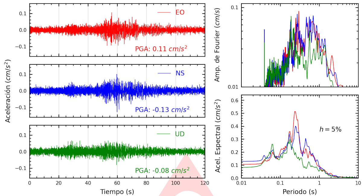
Figura A.1: Registros tiempo-historia, espectros de Fourier y de respuesta en las direcciones EO, NS y vertical de la estación UNICA. Sismo de Lomas, Caraveli - Arequipa del 2024-09-16, 00:08:53 (Hora local)
