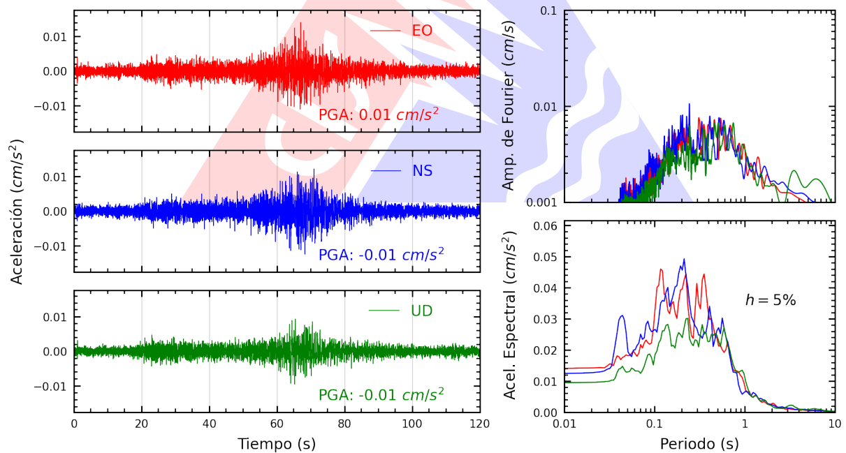
Figura A.2: Registros tiempo-historia, espectros de Fourier y de respuesta en las direcciones EO, NS y vertical de la estación UNSA2. Sismo de Lomas, Caraveli - Arequipa del 2024-09-16, 00:08:53 (Hora local)
